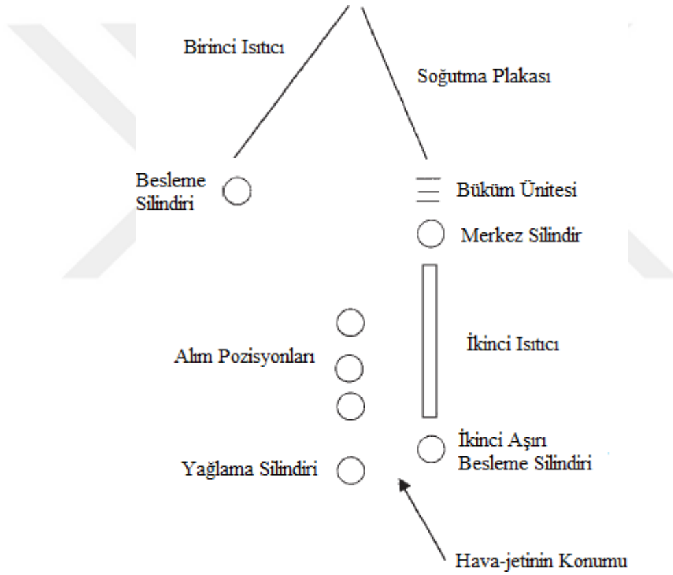
Şekil 2.4. M profilli bir yalancı büküm tekstüre makinesinin şematik gösterimi (Hearle et al., 2001)
