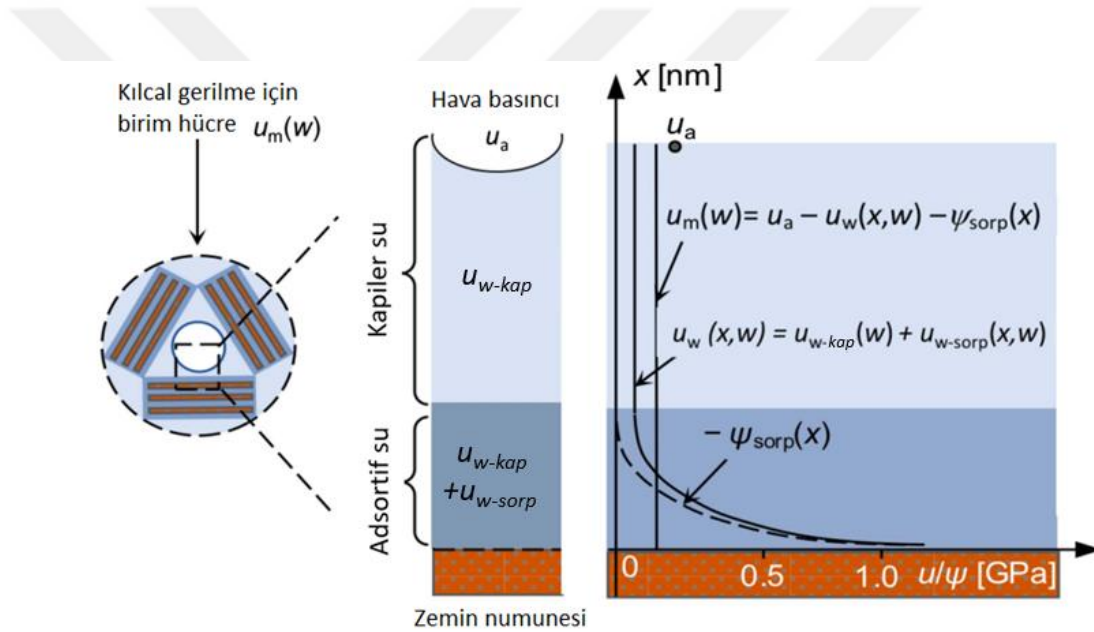
Şekil 4.4. Genelleştirilmiş kılcal gerilme tanımının gösterimi.
