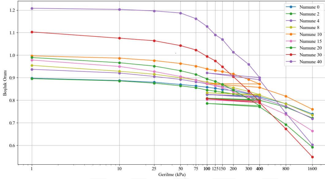
Şekil 6.2. Mevcut ( e-\sigma(\log) ) eğrileri (tek grafik).
