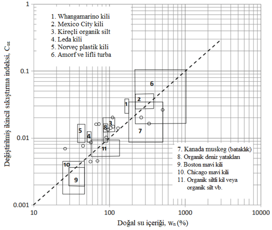
Şekil 2.23. Normal konsolide killeri için doğal su içeriğine karşı modifiye ikincil sıkışma indisi.
