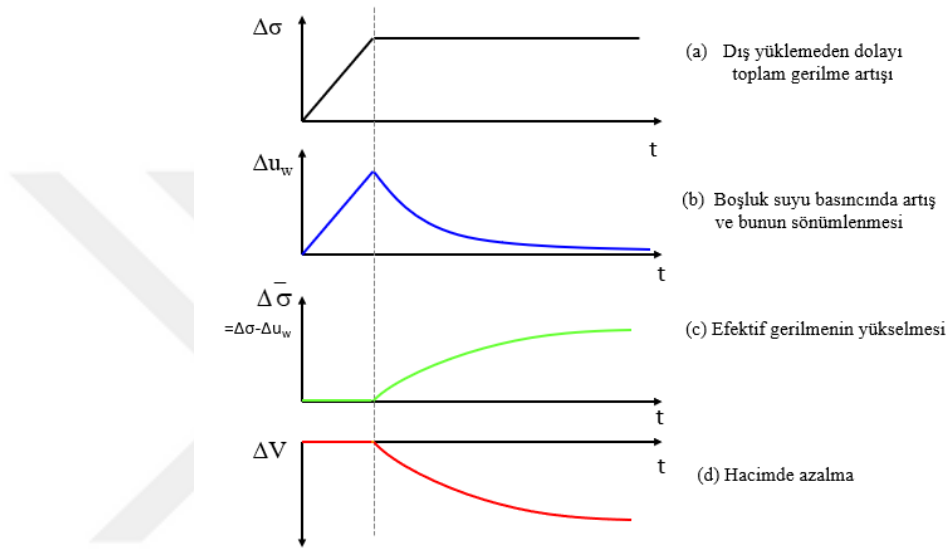
Şekil 2.4. Konsolidasyon süreci: Toplam gerilmenin zaman içinde efektif gerilmeye dönüşmesi [6].
