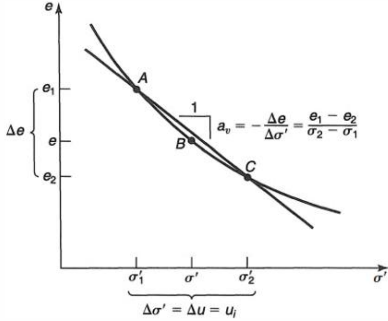
Şekil 2.7. Laboratuvar sıkışma eğrisi.
