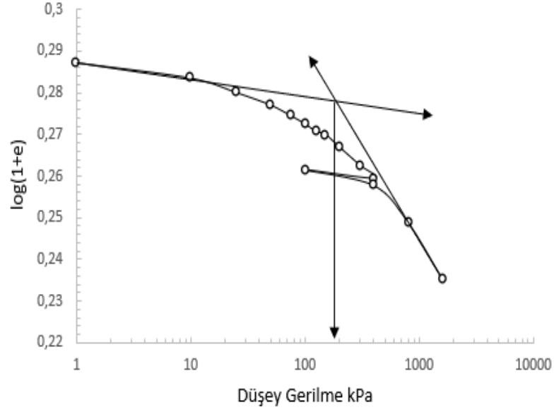
Şekil 2.11. Oikawa-Sridharan yöntemi ile ön konsolidasyon basıncının bulunuşu.
