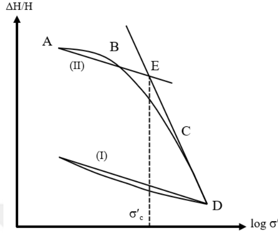
Şekil 2.18. Van Zelts yöntemi ile ön konsolidasyon basıncının bulunuşu.
