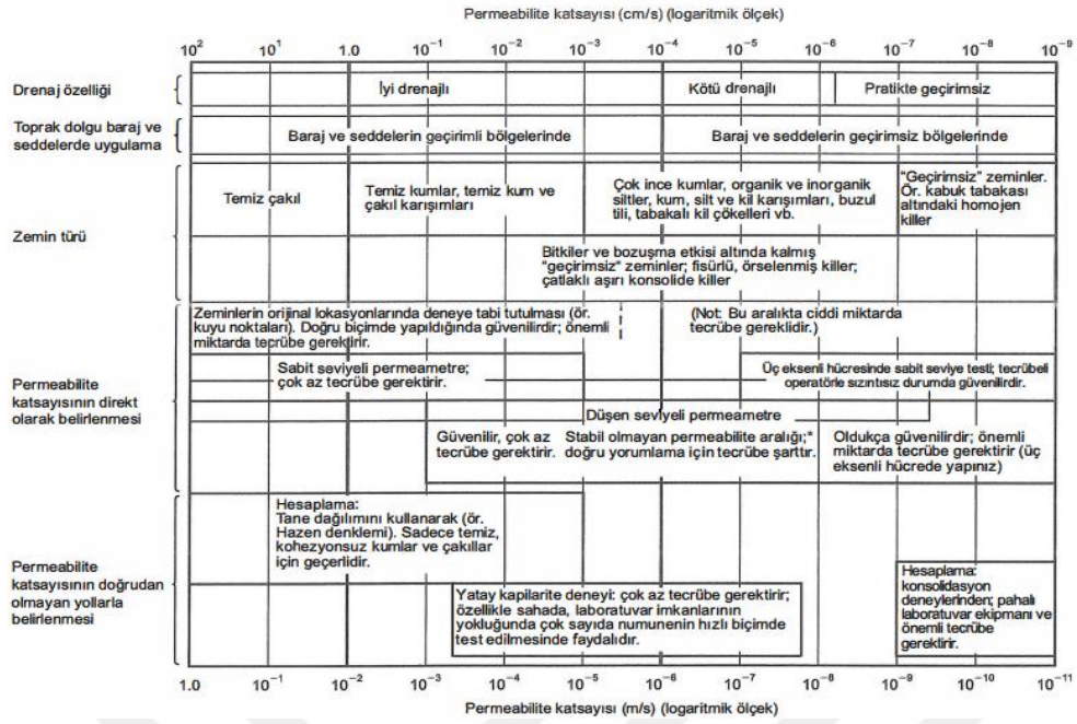
Şekil 3.2. Zemin sınıflarına göre geçirimlilik aralıkları.
