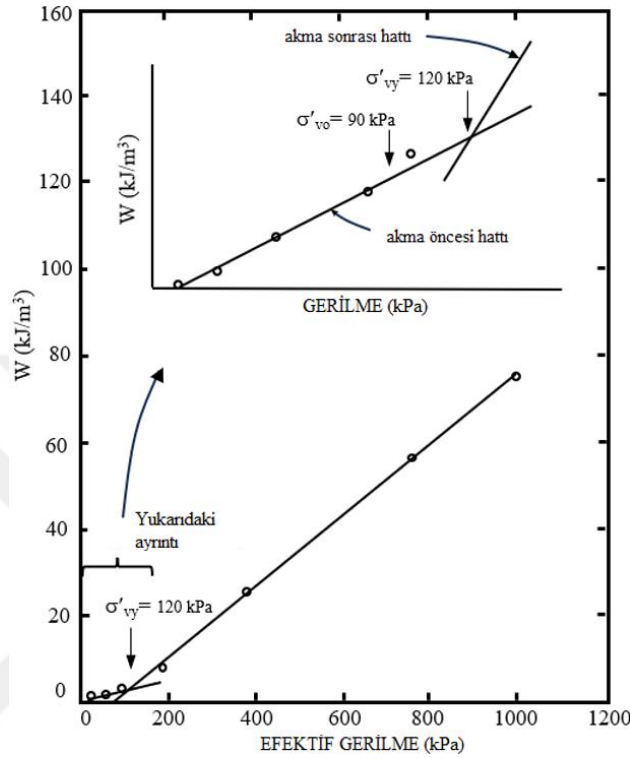
Şekil 2.20. Becker yöntemi ile ön konsolidasyon basıncının bulunuşu.
