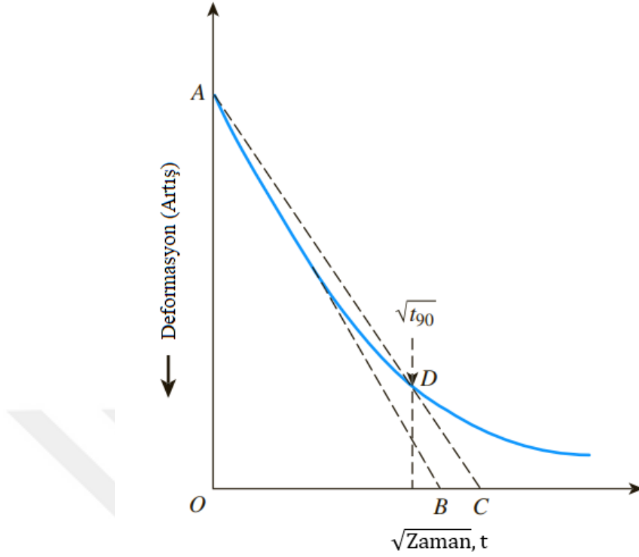
Şekil 2.22. Konsolidasyon katsayısı karekök-zaman yöntemi grafiği [10].
