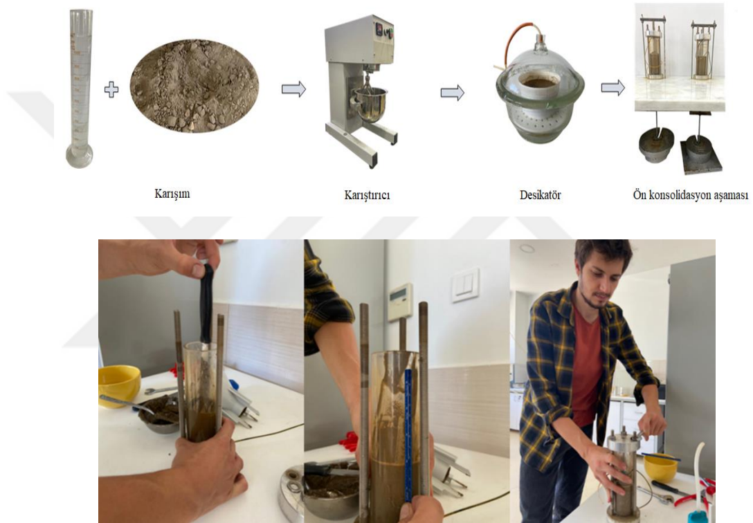
Şekil 5.19. Bulamaç (slurry) yöntemi şematik gösterimi.
