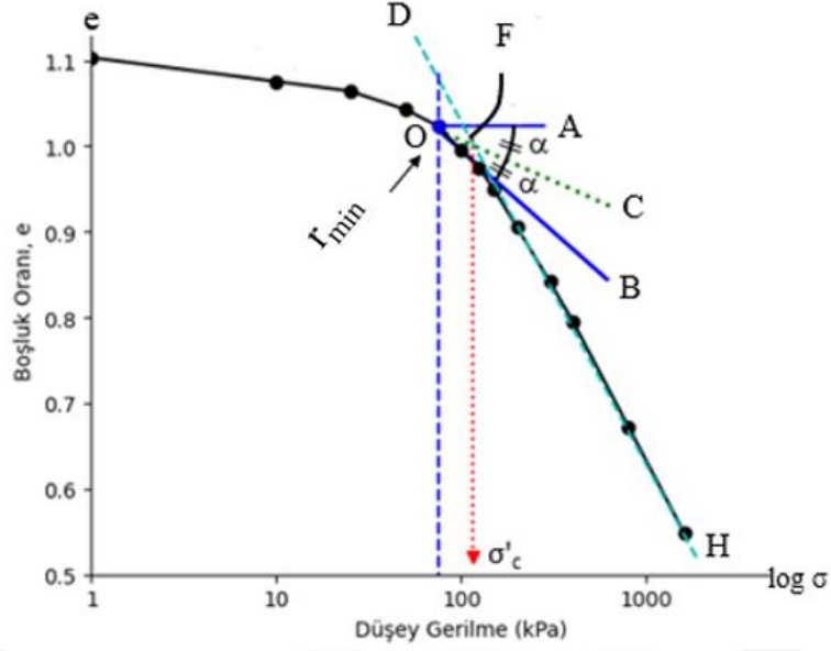
Şekil 2.9. Casagrande yöntemi ile ön konsolidasyon basıncının bulunuşu.
