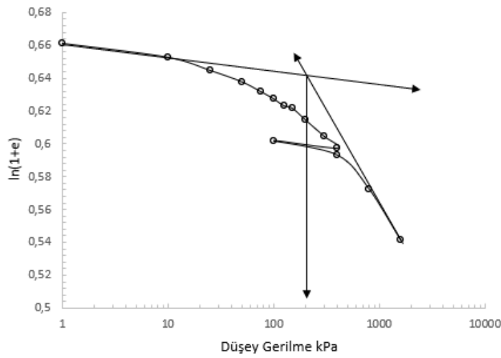
Şekil 2.10. Onitsuka yöntemi ile ön konsolidasyon basıncının bulunuşu.
