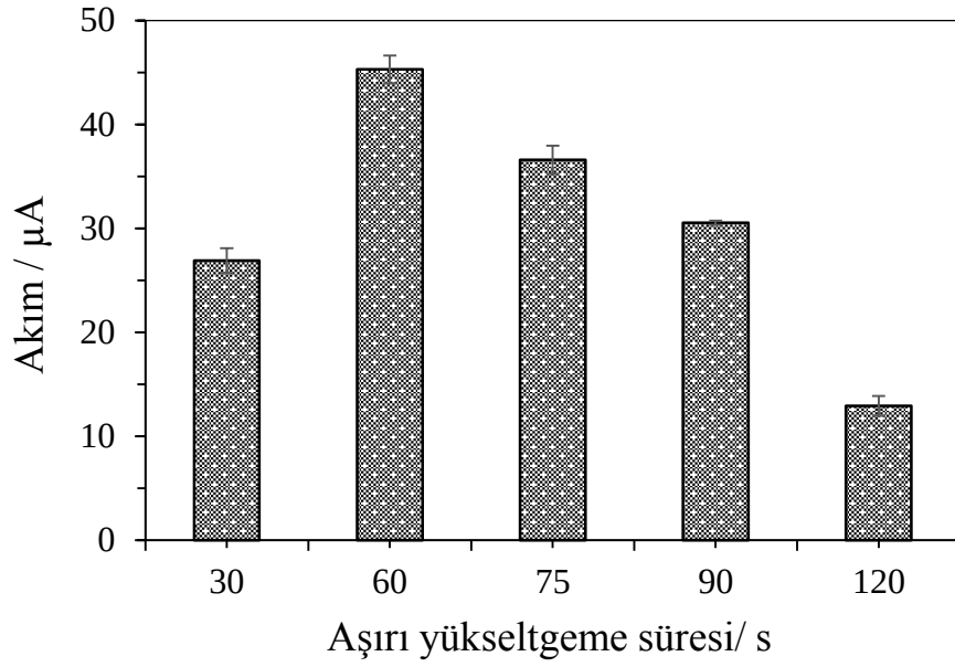
Şekil 4.10. Farklı sürelerde aşırı yükseltgeme işlemi uygulanmış PEDOT-nf/KUG elektrotlar kullanılarak 0,1 M fosfat tamponunda (pH 2) 5,0 \mu M ürik asit varlığında elde edilen yükseltgenme pik akımları
