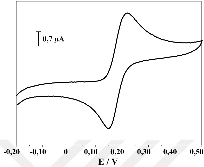
Şekil 4.44. Dopaminin (5 \mu\text{M} ) 0,1 M fosfat tamponunda (pH 5) KUG elektrot ile alınan dönüşümlü voltamogramı
