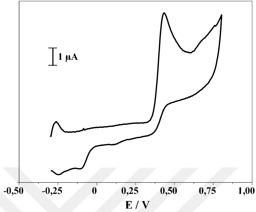
Şekil 4.25. Serotoninin (5 \mu\text{M} ) 0,1 M fosfat tamponunda (pH 5) KUG elektrot ile alınan dönüşümlü voltamogramı (Tarama hızı: 50 \text{mVs}^{-1} , bekleme süresi: 60 s)
