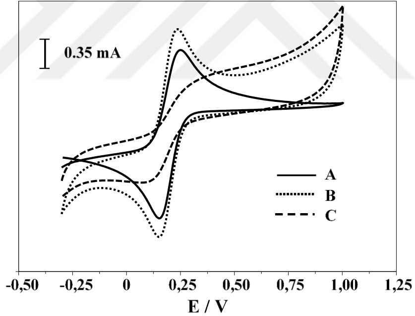
Şekil 4.56. (A) KUG, (B) AY-KUG ve (C) p(P3KA)/AY-KUG elektrolarına ait 0,1M KCl çözeltisinde 2,5 mM \text{Fe}(\text{CN})_6^{3-/4-} varlığında elde edilen dönüşümlü voltamogramlar
