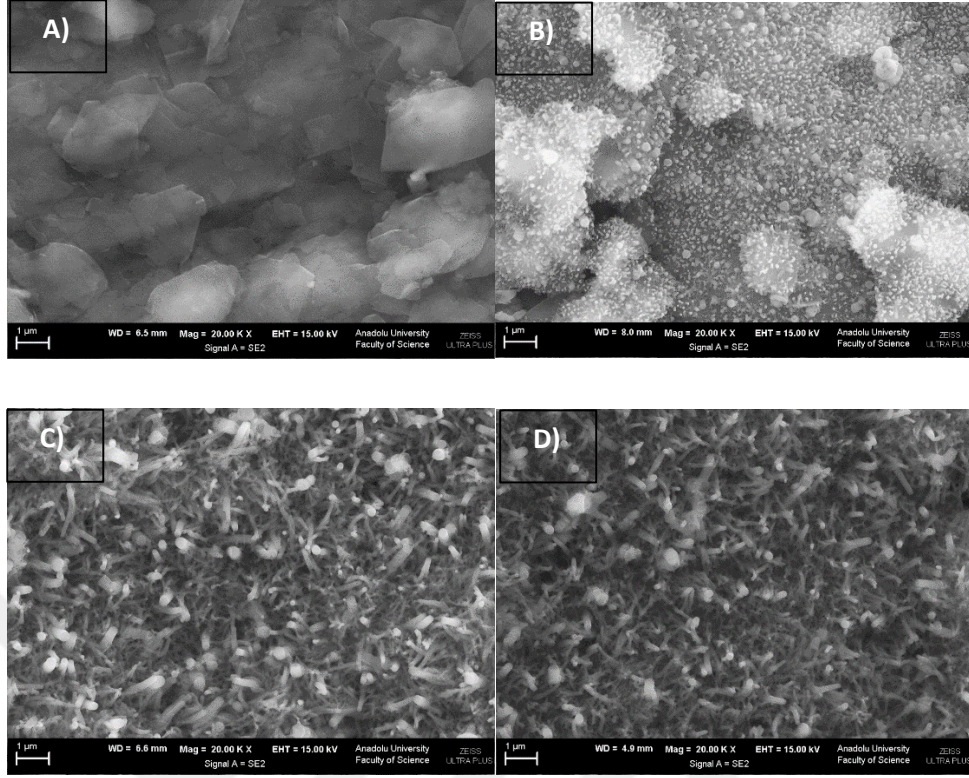
Şekil 4.17. KUG (A), 3 döngü ile hazırlanan PEDOT-nf/KUG (B), 20 döngü ile hazırlanan PEDOT-nf/KUG (C) ve 2V gerilim değerinde 60 saniye aşırı yükseltgeme ile hazırlanan AY-PEDOT-nf/KUG (D) elektrotlarının SEM görüntüleri
