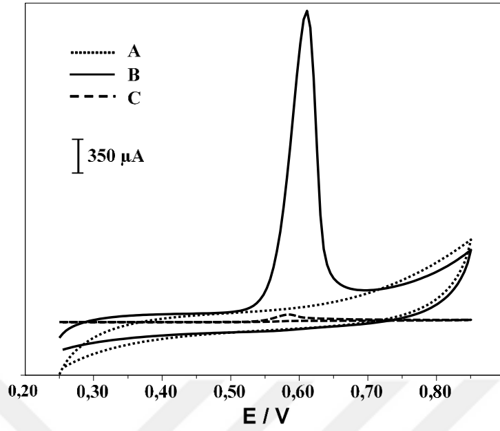
Şekil 4.5. AY-PEDOT-nf/KUG elektrodun ürik asit yokluğunda (A), AY-PEDOT-nf/KUG (B) ve KUG (C) elektrodun 50 \mu\text{M} ürik asit varlığında 0,1 M fosfat tamponunda (pH 2) elde edilen dönüşümlü voltamogramları
