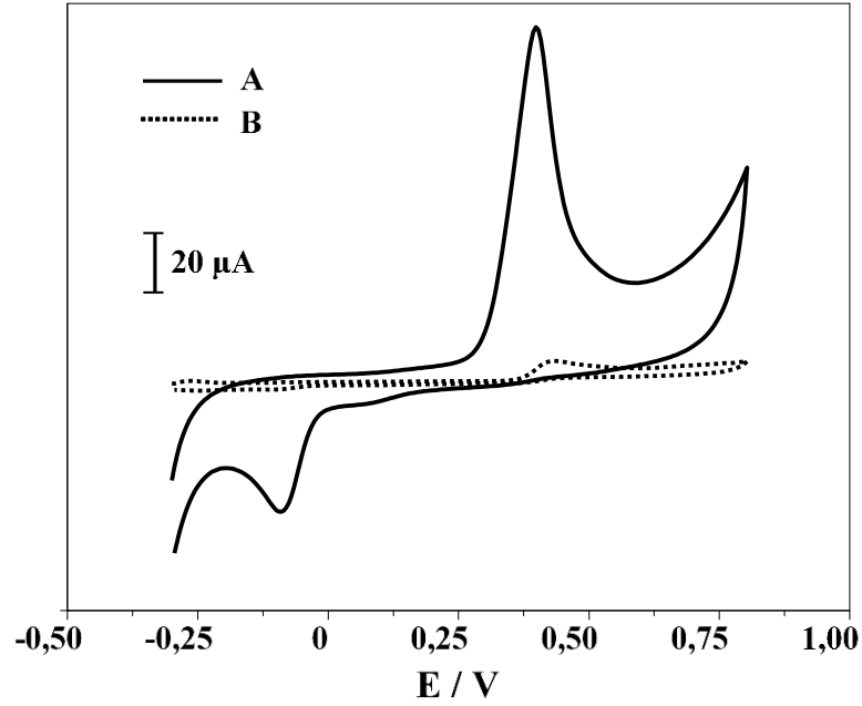
Şekil 4.28. p(P3KA)/KUG (A) ve KUG (B) elektrotlarının fosfat tamponunda (pH 5) 5,0 \mu M serotonin varlığında elde edilen dönüşümlü voltamogramları
