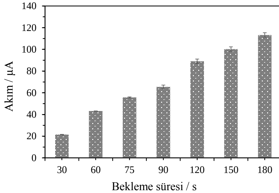
Şekil 4.20. AY-PEDOT-nf/KUG elektrotlar ile pH 2'de farklı bekleme sürelerinde elde edilen 5,0 \mu\text{M} ürik asite ait yükseltgenme pik akımları
