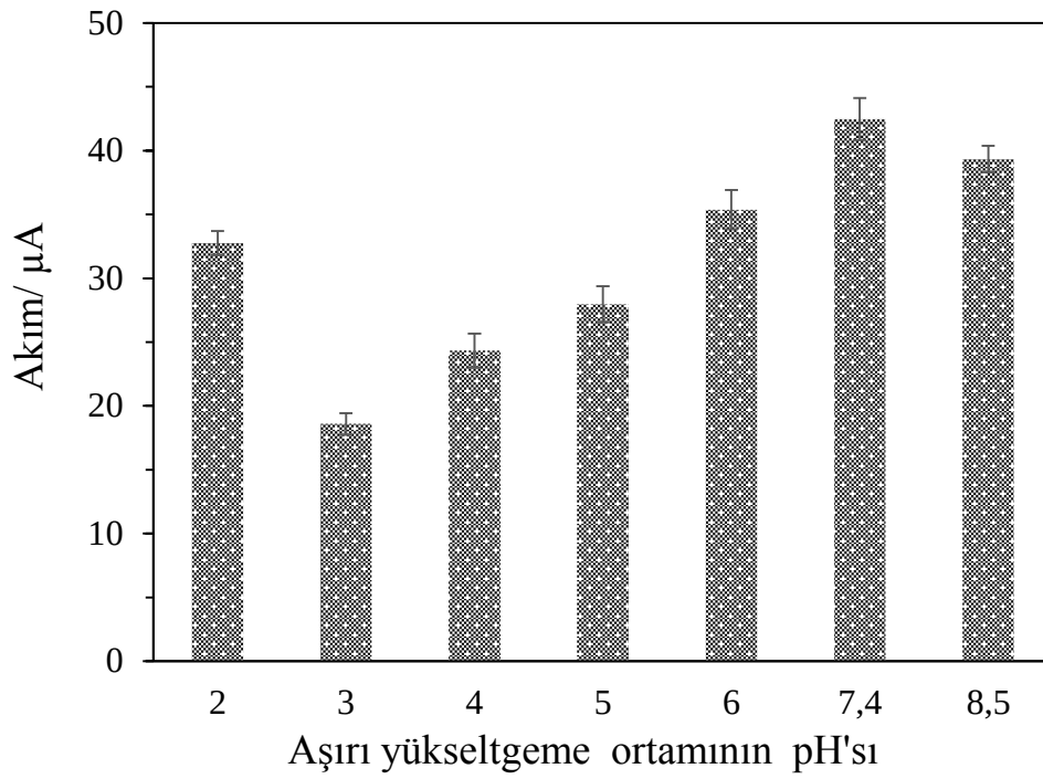
Şekil 4.11. Farklı pH değerlerinde aşırı yükseltgenmiş PEDOT-nf/KUG elektrotlar kullanılarak 0,1 M fosfat tamponunda elde edilen 5,0 \mu\text{M} ürik asite ait yükseltgenme pik akımları
