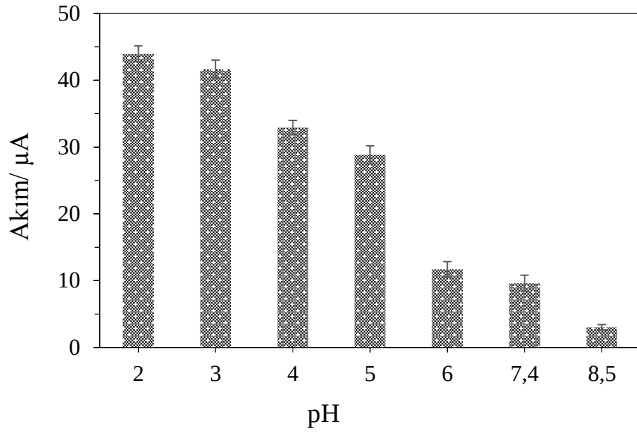
Şekil 4.18. AY-PEDOT-nf/KUG elektrotların farklı pH değerlerinde elde edilen 5,0 \mu\text{M} ürik asite ait yükseltgenme pik akımları (Bekleme süresi: 60 s)
