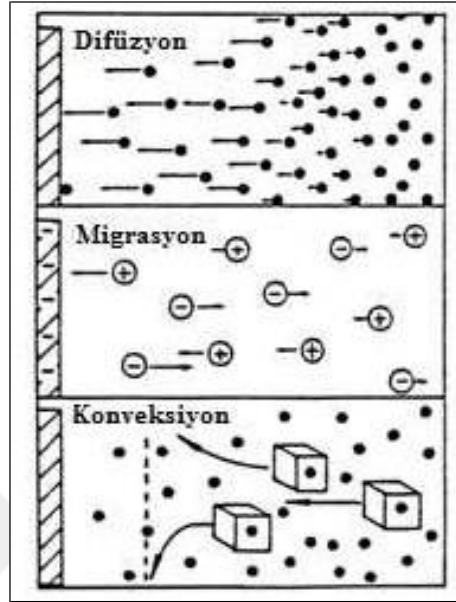
Şekil 2.13. Elektrokimyasal hücrede gerçekleşen kütle aktarım türleri
