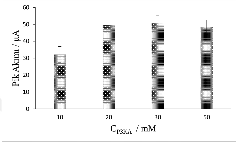
Şekil 4.52. Farklı derişimlerde P3KA monomeri içeren polimerizasyon çözeltisinde hazırlanan p(P3KA)/AY-KUG elektrotlar ile fosfat tamponunda (pH 7,4) elde edilen 5,0 \mu\text{M} dopaminin yükseltgenme pik akımları
