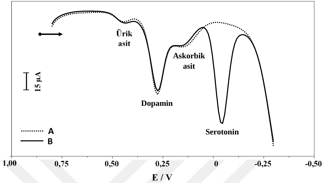
Şekil 4.40. p(P3KA)/KUG elektrotlar ile 500,0 \mu\text{M} askorbik asit, 5,0 \mu\text{M} dopamin ve 5,0 \mu\text{M} ürik asit içeren fosfat tamponunda (pH 5) serotonin yokluğunda (A) ve 5,0 \mu\text{M} serotonin varlığında (B) elde edilen diferansiyel puls voltamogramları
