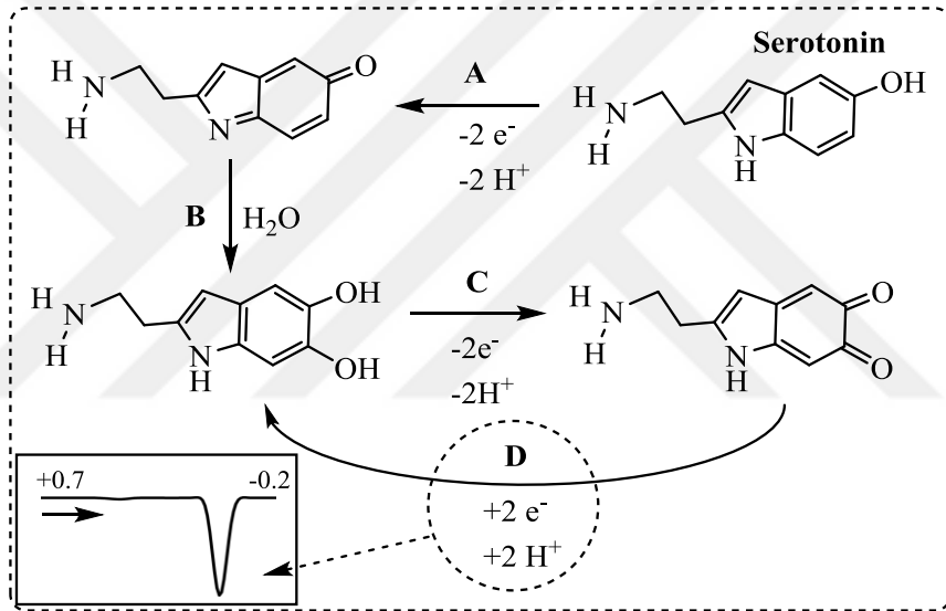
Şekil 4.31. p(P3KA)/KUG elektrot ile 5,0 \mu\text{M} serotonin içeren fosfat tamponunda (pH 5) 0,70 ile -0,20 V gerilim aralığında katodik yönde gerilim taraması esnasında gerçekleşen dönüşümleri
