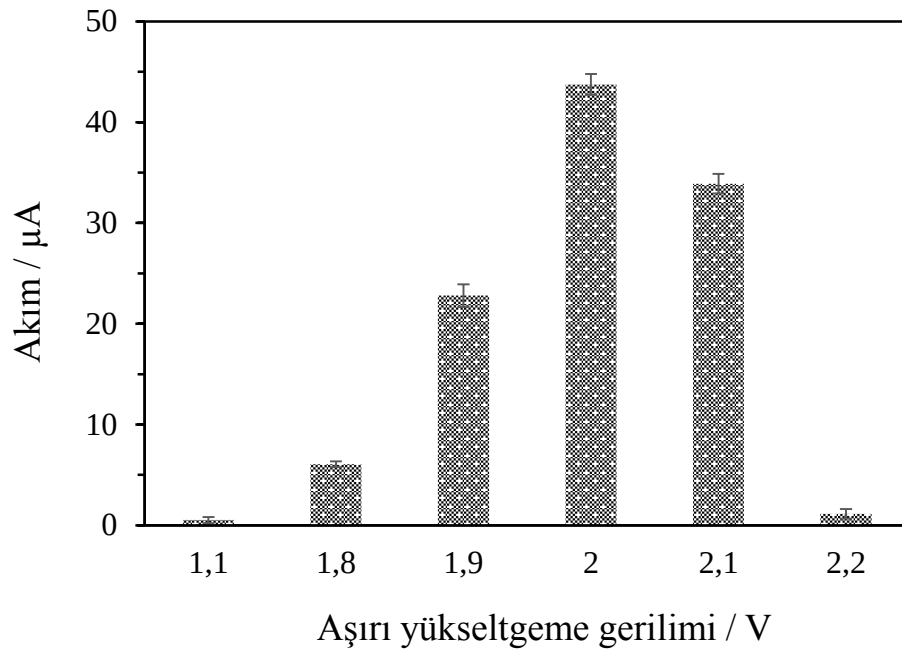
Şekil 4.9. Farklı gerilimlerde aşırı yükseltgenmiş AY-PEDOT-nf/KUG elektrotların 0,1 M fosfat tamponunda (pH 2) elde edilen 5,0 µM ürik asite ait yükseltgenme pik akımları
