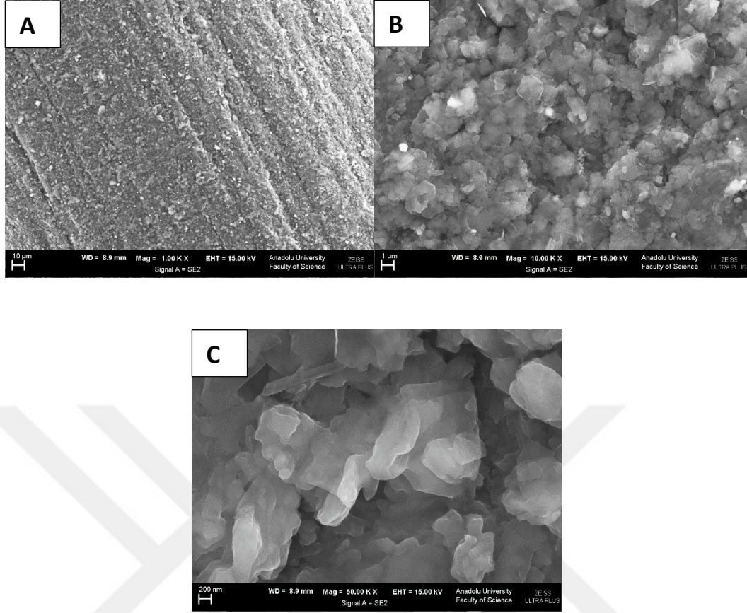
Şekil 4.59. p(P3KA)/AY-KUG elektrodunun farklı büyütme oranlarında alınan SEM görüntüleri (A: 1,5X, B: 10000X ve C: 50000X)
