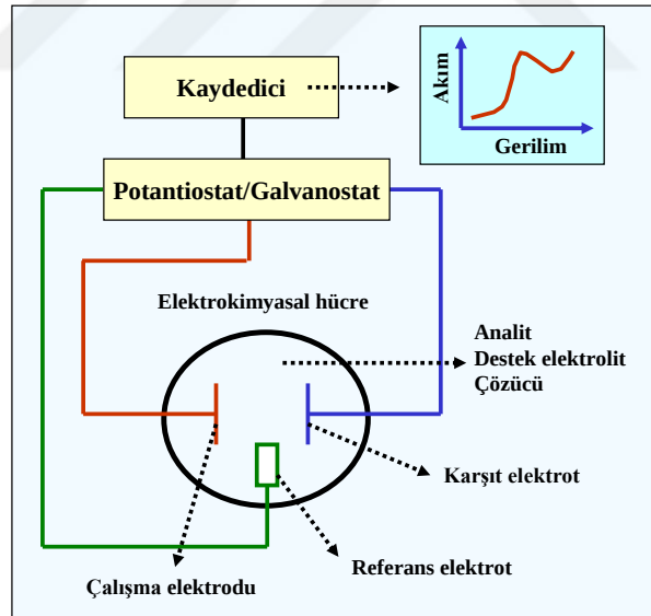
Şekil 2.7. Voltametrik ölçümlerin gerçekleştirildiği bir analiz sisteminin şematik görünümü
