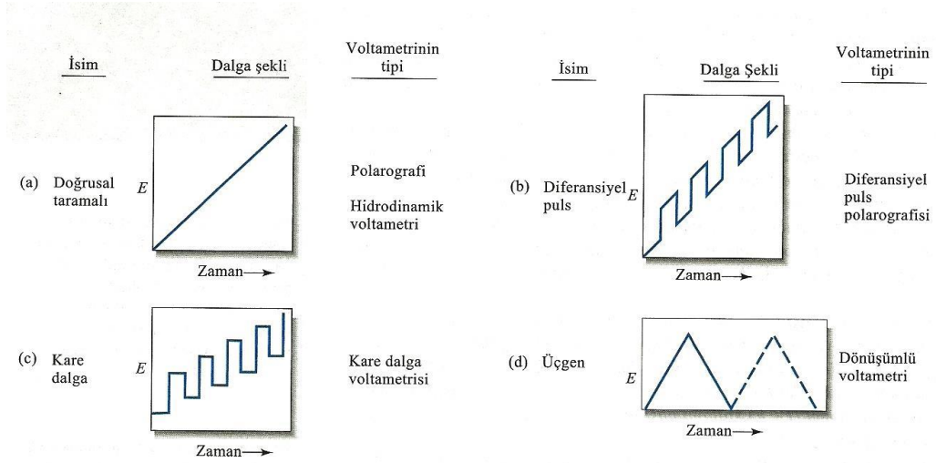
Şekil 2.14. Voltametrik çalışmalarda kullanılan uyarma sinyalleri ve gerçekleştirilebilecek farklı voltmetri tipleri
