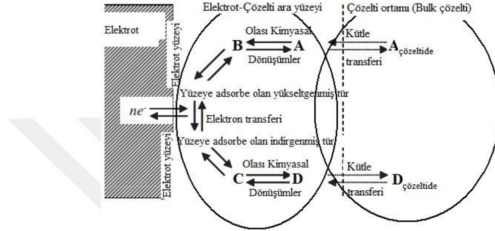
Şekil 2.12. Elektrokimyasal çalışmalarda pik şeklini ve pik akımını etkileyen olası sistem dönüşümleri [134]
