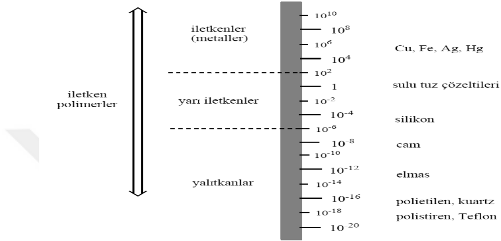
Şekil 2.2. İletken polimerlerin iletkenliklerinin iletken, yarı iletken ve yalıtkanlar ile karşılaştırılması
