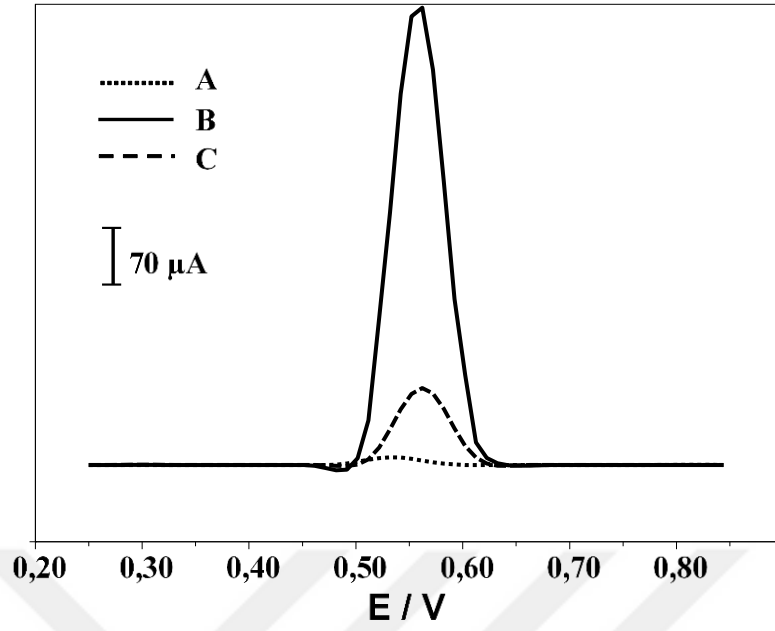
Şekil 4.8. KUG(A), AY-PEDOT/KUG (B) ve AY-PPy/KUG (C) elektrotlarının 5,0 \mu\text{M} ürik asit içeren fosfat tamponunda (pH 2) elde edilen diferansiyel puls voltamogramları (Bekleme süresi: 120 s; Karıştırma hızı: 250 rpm)
