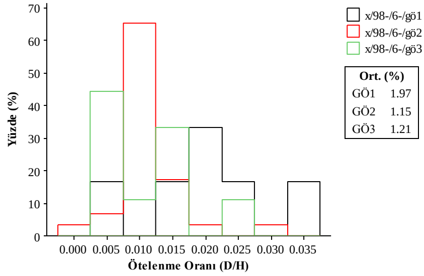
Şekil B.52: Orta Yükseklikteki Eski Binaların GÖ Performans Seviyesi Dağılımları
