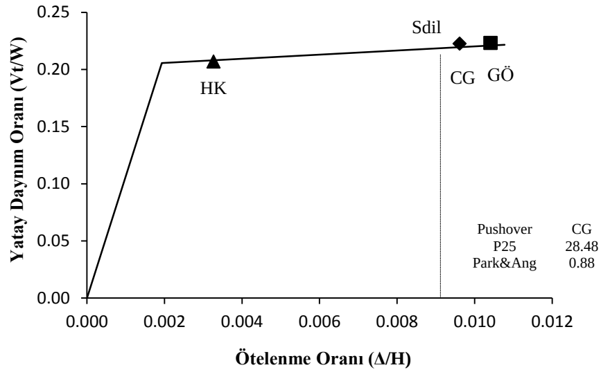
Şekil B.75: Bina#1 Performans Sonuçları (X Yönü)
