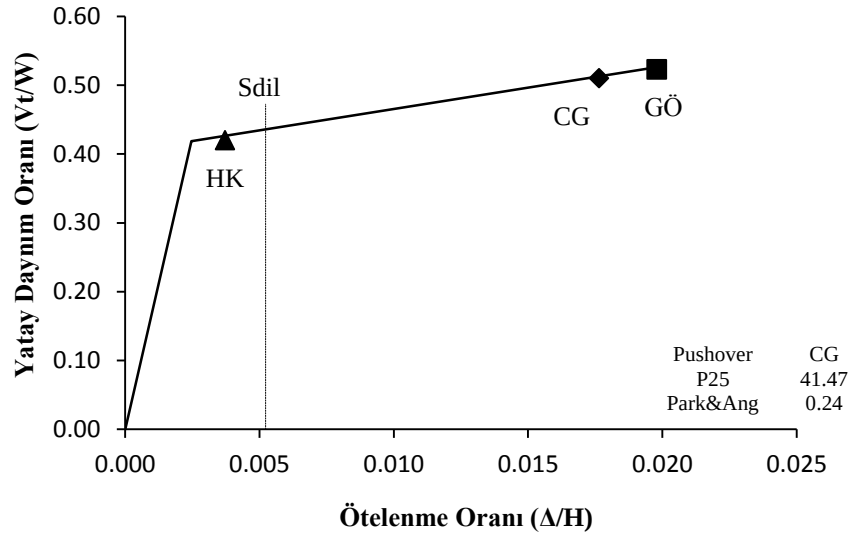
Şekil B.81: Bina#28 Performans Sonuçları (X Yönü)
