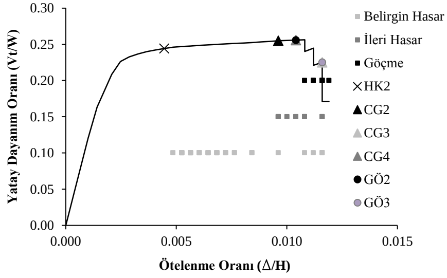
Şekil B.1: Bina#1'e Ait Kolon Hasar Dağılımları (X Yönü)
