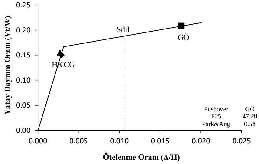
Şekil B.85:Bina#34 Performans Sonuçları (X Yönü)
