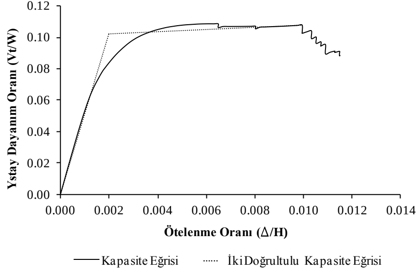
Şekil 4.9: Bina#16'ya Ait İki Doğrultulu Hale Getirilmiş Kapasite Eğrisi
