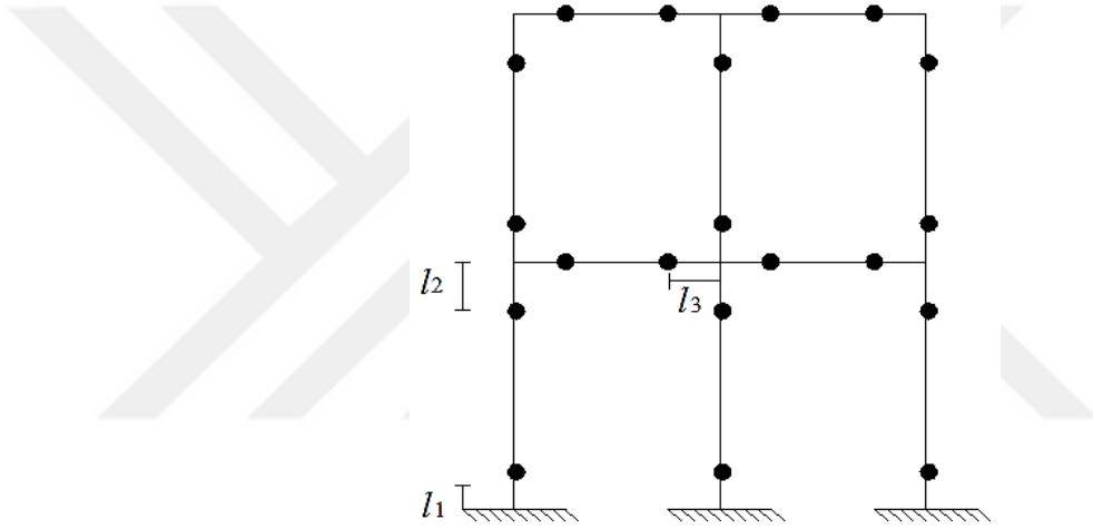
Şekil 4.8: Eğilme Mafsallarının Yeri ve Boyu
