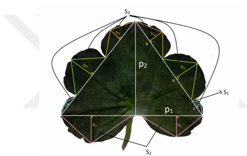
Şekil 4.4 : Beş loblu yaprak üzerinde Arşimet Teoremi'nin uygulanması.
