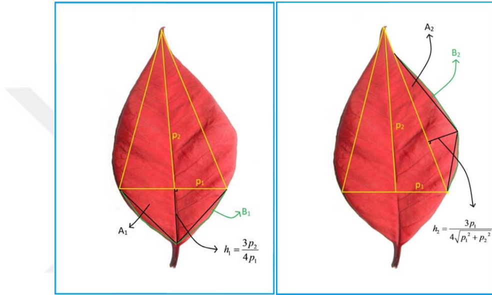
Şekil 4.3: Eliptik tipi yaprak üzerinde Arşimet Teoremi'nin uygulanması.
