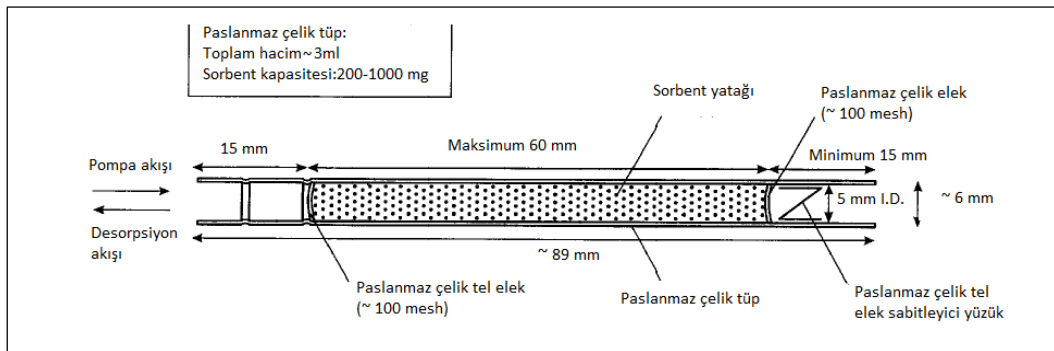
Şekil 2.3. Sorbent tüpünün şematik gösterimi
