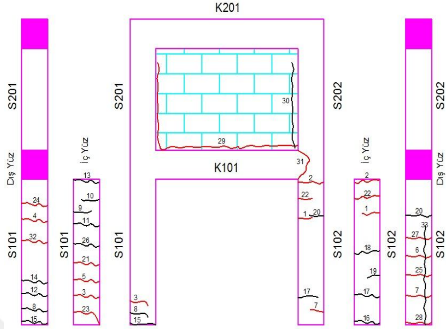
Şekil 4.16. Yumuşak katlı çerçeve numunesinde (DN2-YKÇ) meydana gelen çatlaklar ve numaraları.
