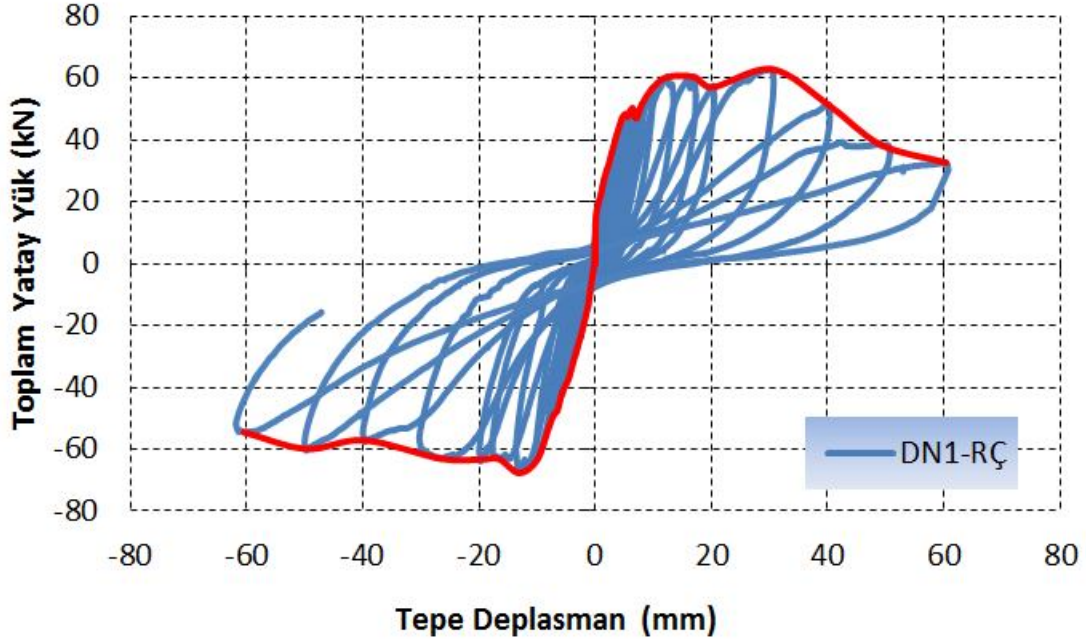
Şekil 4.8. Referans numuneye (DN1-RÇ) ait yatay yük-tepe deplasmanı çevrimsel histeresis eğrisi ve zarfı eğrisi.
