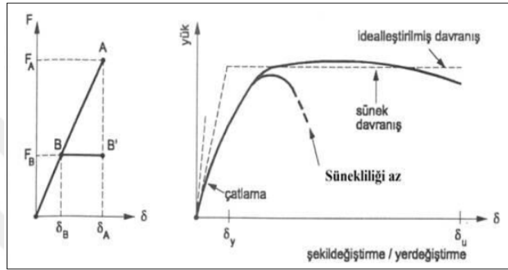
Şekil 1.7. Elastik olan ve olmayan kuvvet-yer değiştirme grafiği ve betonarme elemanda yük-yer Değiştirme Eğrisi (Celep ve Kumbasar, 2004)
