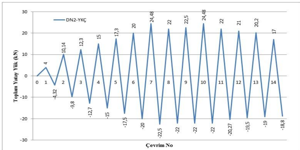
Şekil 4.11. Yumuşak katlı çerçevenin (DN2-YKÇ) yatay yük geçmişi.
