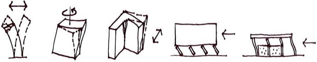
Şekil 1.2. Mimari tasarım açısından hatalı ve eksik tasarım kararlarına bağlı olası hasar ve yıkım nedenleri (Zacek, 2002b)
