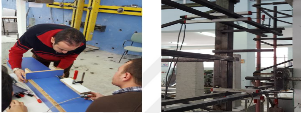
Şekil 3.24. Deneylerde kullanılan LVDT'lerin kalibrasyonu ve yerleşimi.
