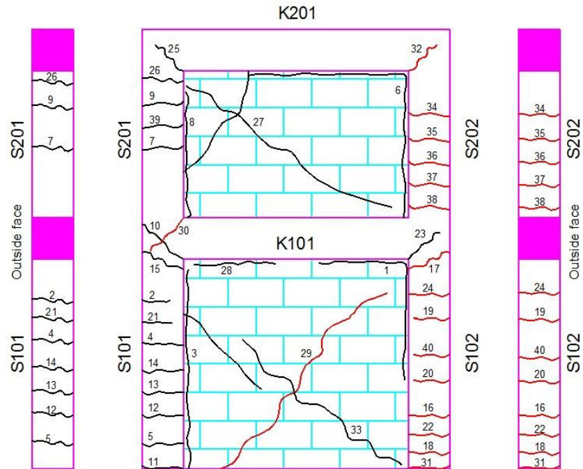
Şekil 4.7. Referans çerçeve numunesinde (DN1-RÇ) meydana gelen çatlaklar ve numaraları.
