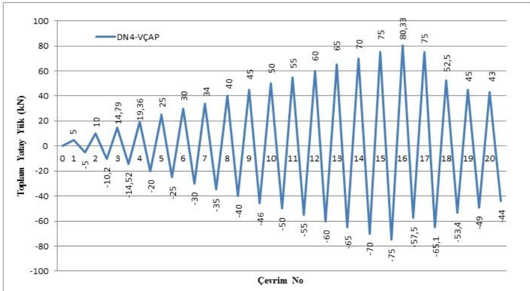
Şekil 4.29. Merkezi V çelik çapraz çerçeve numunesinin (DN4-VÇAP) yatay yük geçmişi.
