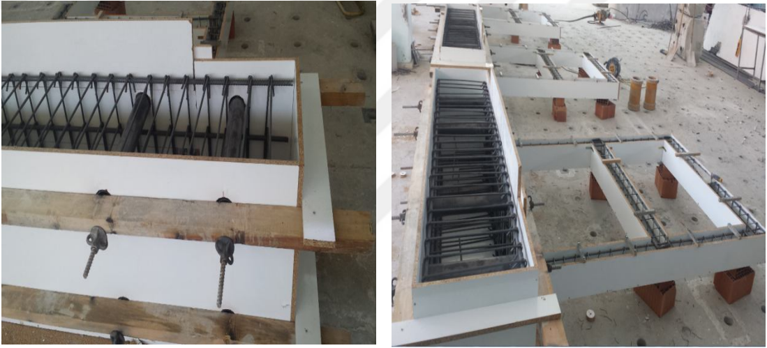
Şekil 3.8. Donatıların hazırlanması ve kalıplara yerleştirilmesi.
