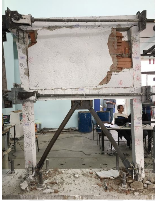
Şekil 4.32. Merkezi v çelik çapraz çerçeve numunesinin (DN4-VÇAP) deneyden sonraki görünüşü.
