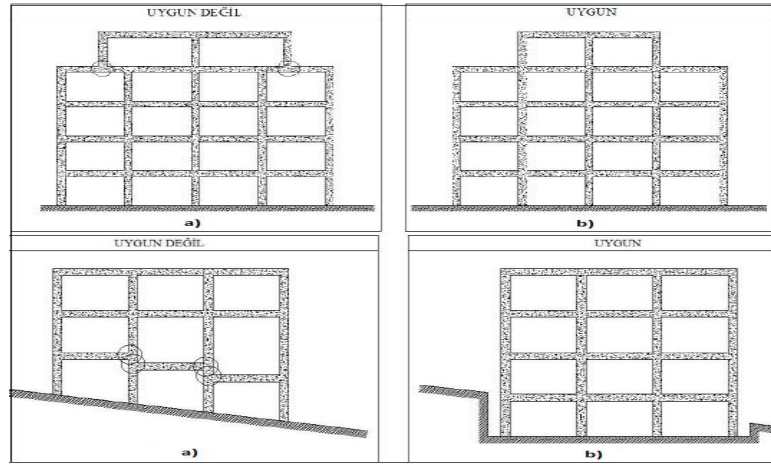
Şekil 1.4. Depreme dayanıklı yapı tasarımında uygun ve uygun olmayan taşıyıcı sistem sürekliliği düzeni (Celep ve Kumbasar, 2004).
