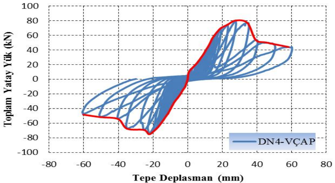
Şekil 4.36. Merkezi ters V çelik çaprazlı çerçeve numunesine (DN4-VÇAP) ait yatay yük-tepe deplasmanı çevrimsel histeresis eğrisi ve dayanım zarfı.
