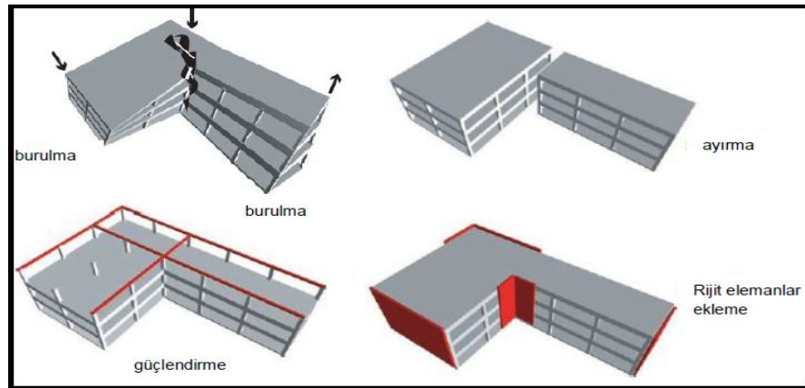
Şekil 1.5. Depreme dayanıklı yapı tasarımında yapı rijitliğinin arttırılması (Arnold, 1982)
