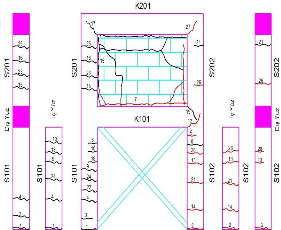
Şekil 4.23. Merkezi X çelik çapraz çerçeve numunesinin (DN3-XÇAP) deneyden sonraki görünüşü.
