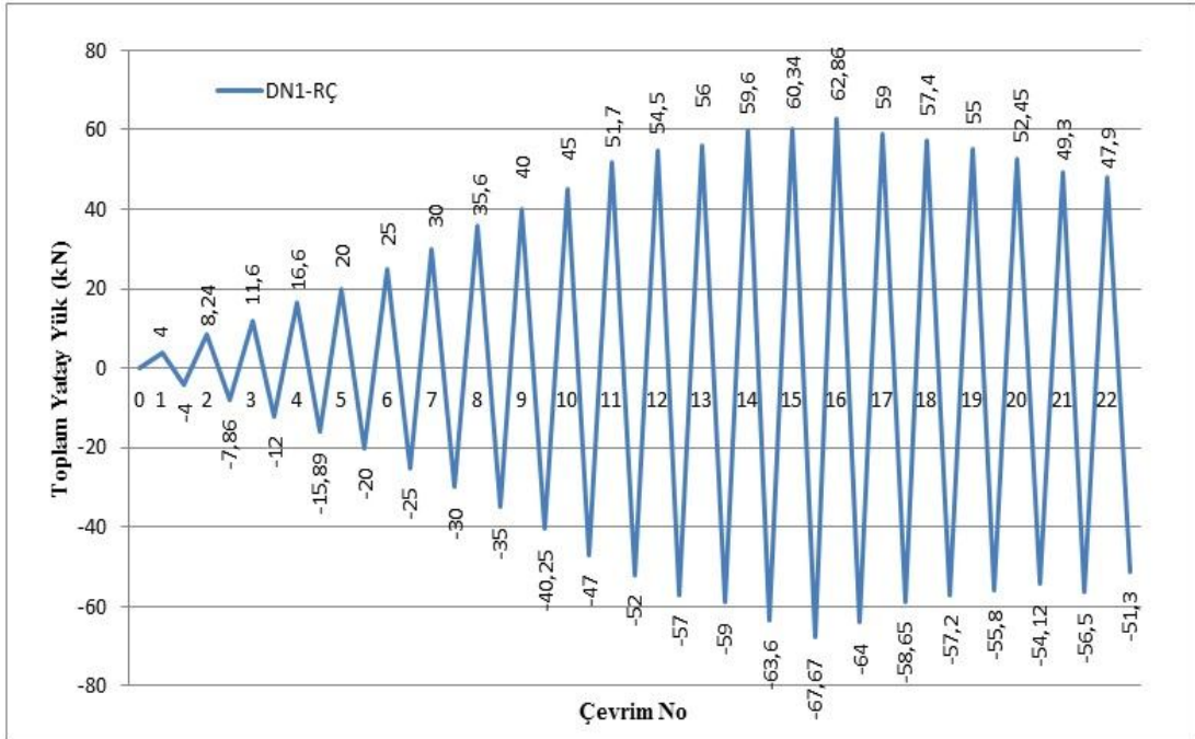
Şekil 4.2. Referans numunesinin (DN1-RÇ) yatay yük geçmişi.
