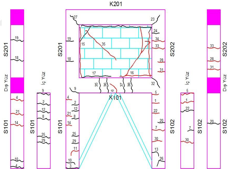
Şekil 4.33. Merkezi V çelik çapraz çerçeve numunesinde (DN4-VÇAP) meydana gelen çatlaklar ve numaraları.
