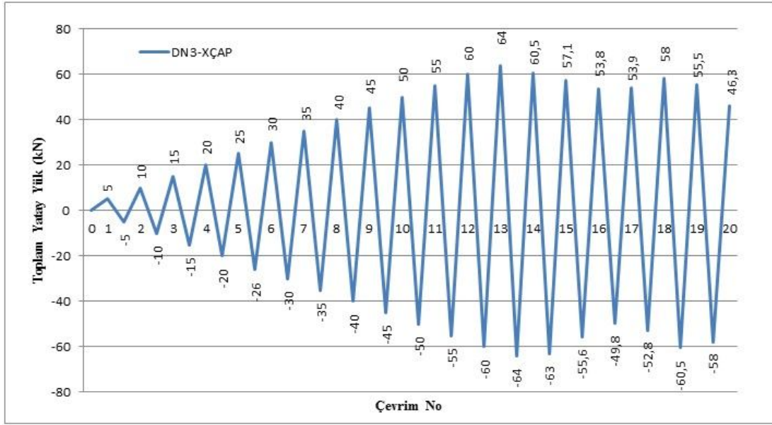
Şekil 4.20. Merkezi X çelik çapraz çerçeve numunesinin (DN3-XÇAP) yatay yük geçmişi.
