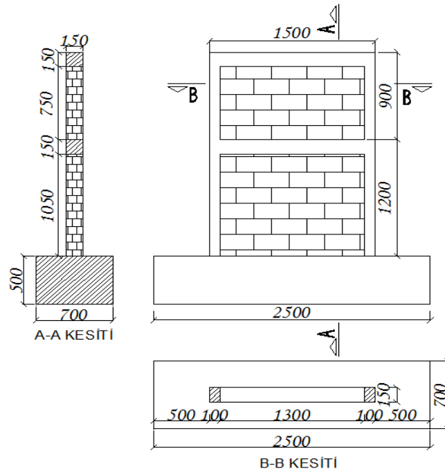
Şekil 3.1. Referans deney elemanının görünümü ve boyutları (ölçüler mm'dir)
