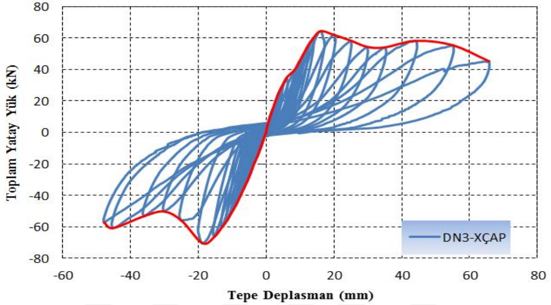
Şekil 4.26. Merkezi X çelik çaprazlı numuneye (DN3-XÇAP) ait yatay yük-tepe deplasmanı çevrimsel histerezis eğrisi ve dayanım zarfı.
