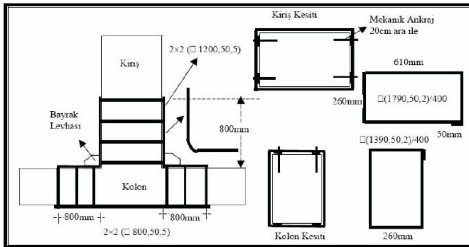
Şekil 1.14. Çelik lamalarla güçlendirilmiş bir birleşim bölgesi (Tonyalı, 2006).
