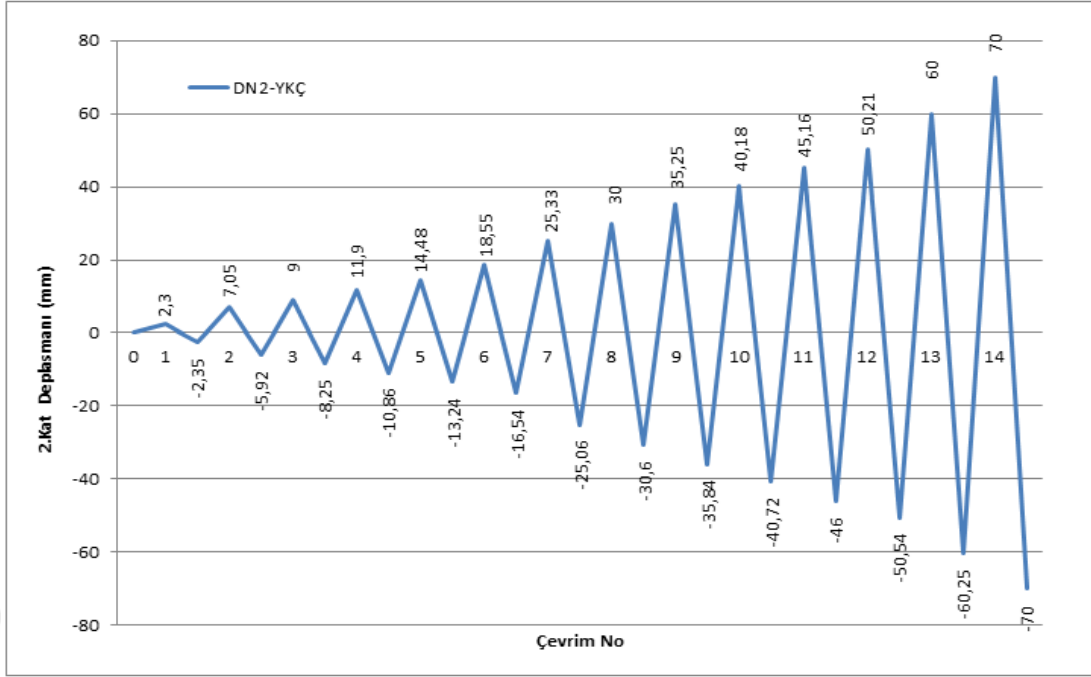
Şekil 4.12. Yumuşak katlı çerçevenin (DN2-YKÇ) tepe deplasman geçmişi.
