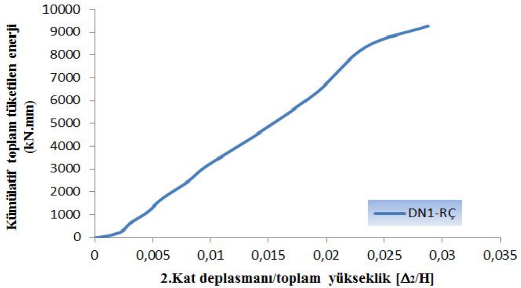
Şekil 4.9. Referans numunesine (DN1-RÇ) ait kümülatif toplam tüketilen enerji – 2. kat ötelenme oranı grafiği.
