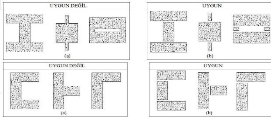
Şekil 1.3. Depreme dayanıklı yapı tasarımında bina geometrisinin uygun ve uygun olmayan yapı planı (Celep ve Kumbasar, 2004).
