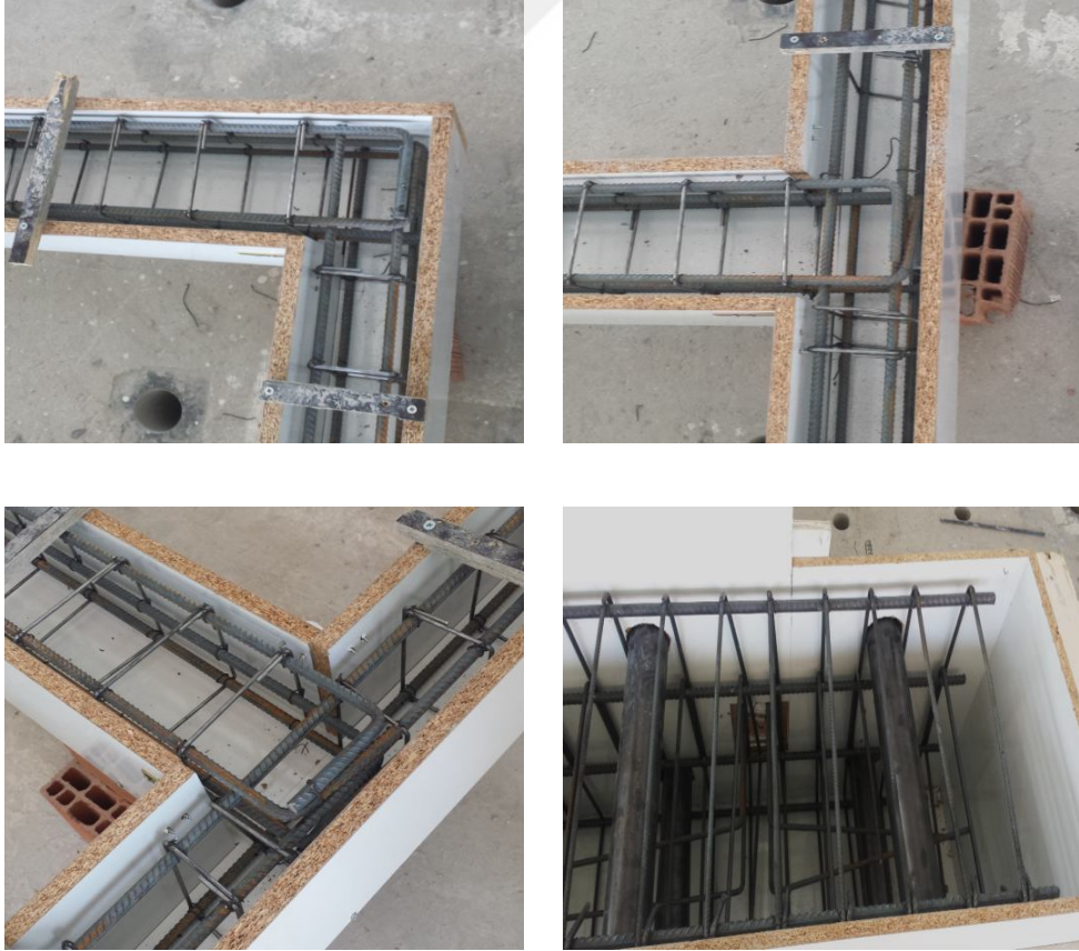
Şekil 3.4. Çerçeve numuneleri birleşim bölgelerine ait donatı detayı.
