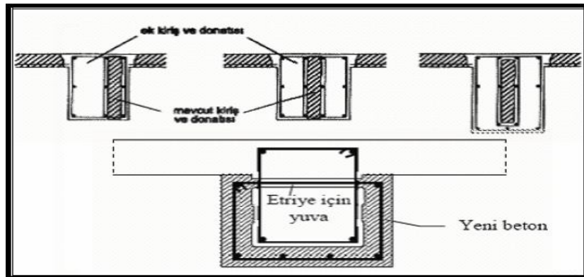
Şekil 1.12. Kiriş mantolaması (Tonyalı, 2006)
