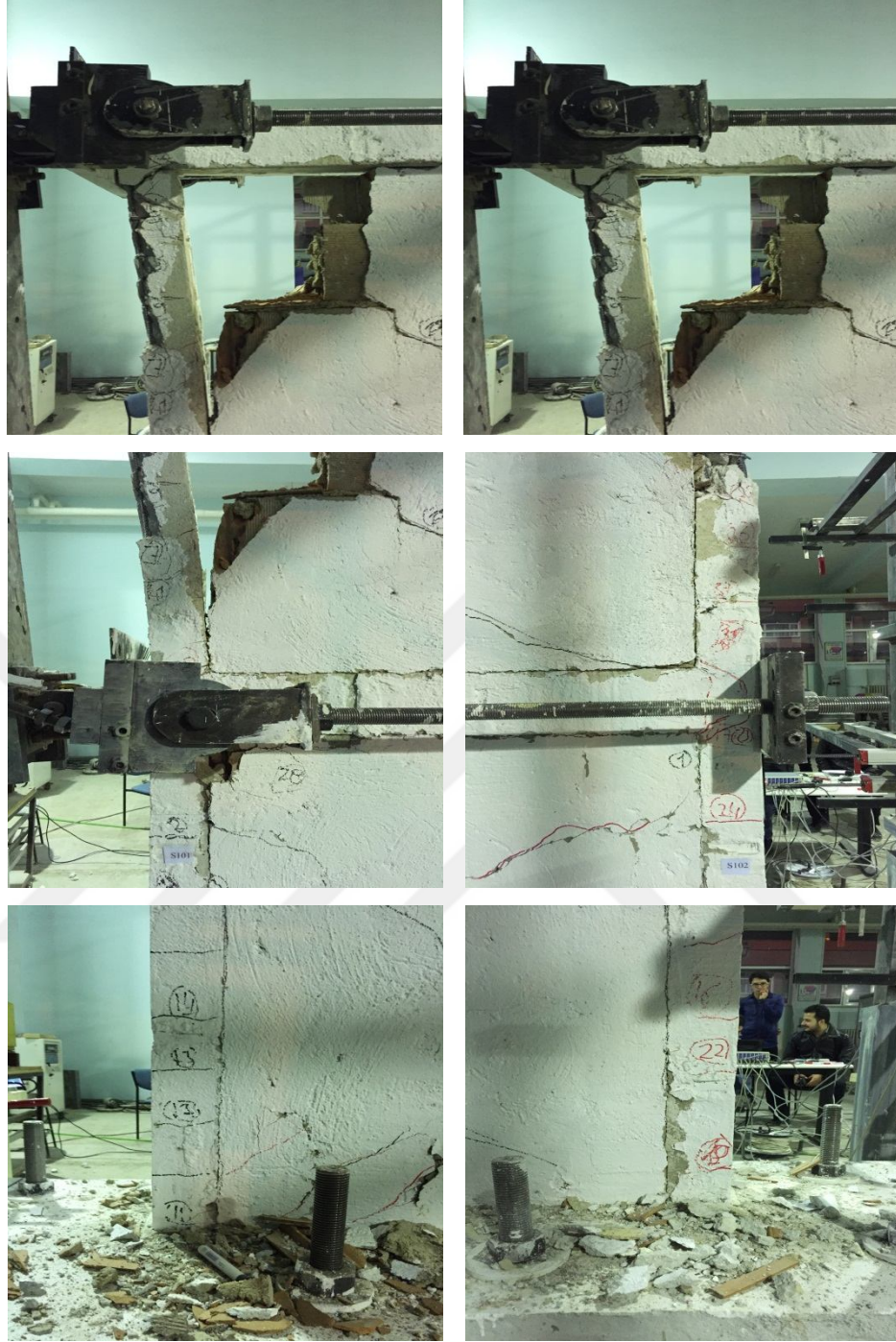
Şekil 4.5. Deney sonunda referans çerçeve numunesi (DN1-RÇ) düğüm noktaları hasarları.
