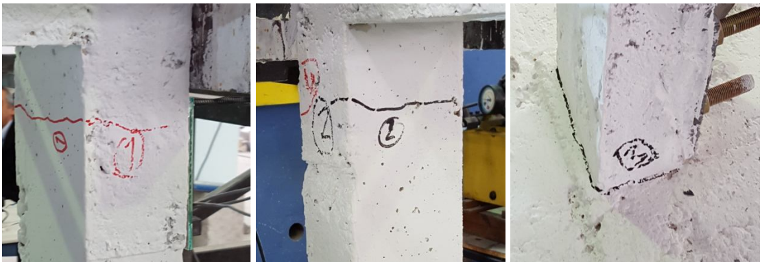
Şekil 4.31. Merkezi V çelik çapraz çerçeve numunesine (DN4-VÇAP) ait ilk çatlaklar.
