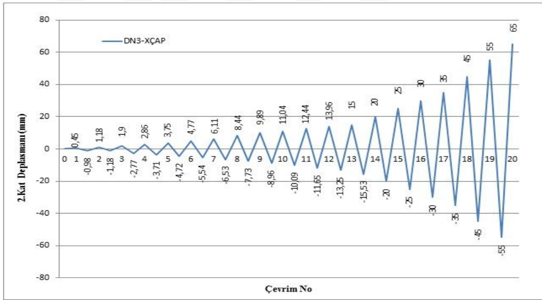
Şekil 4.21. Merkezi X çelik çapraz çerçeve numunesinin (DN3-XÇAP) tepe deplasman geçmişi.
