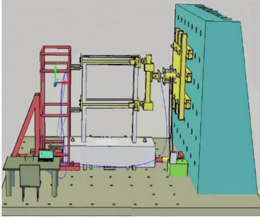
Şekil 3.20. Yükleme düzeneğinin görünümü (Ünal ve ark., 2013)
