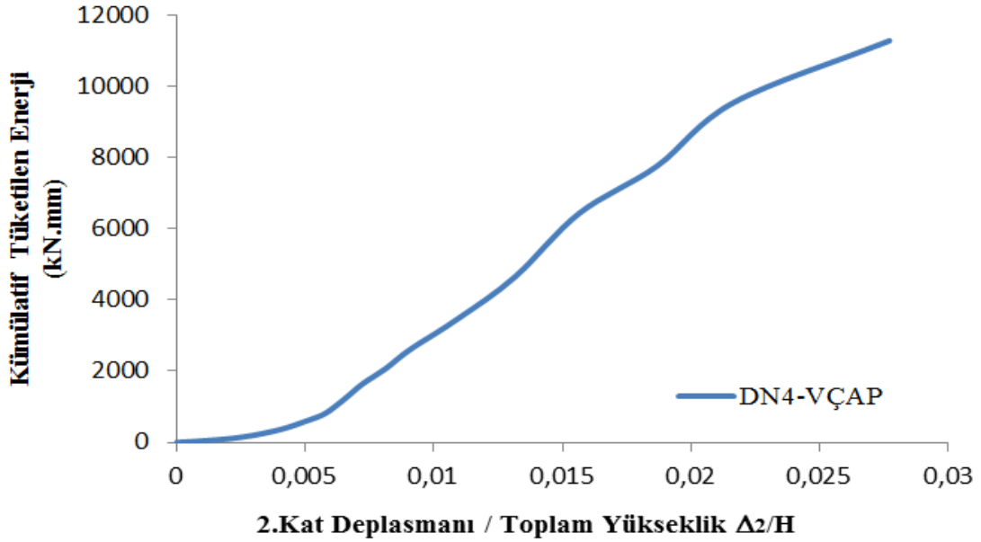
Şekil 4.37. Merkezi ters V çelik çaprazlı çerçeve numunesine (DN4-VÇAP) ait kümülatif toplam tüketilen enerji – 2. kat ötelenme oranı grafiği.
