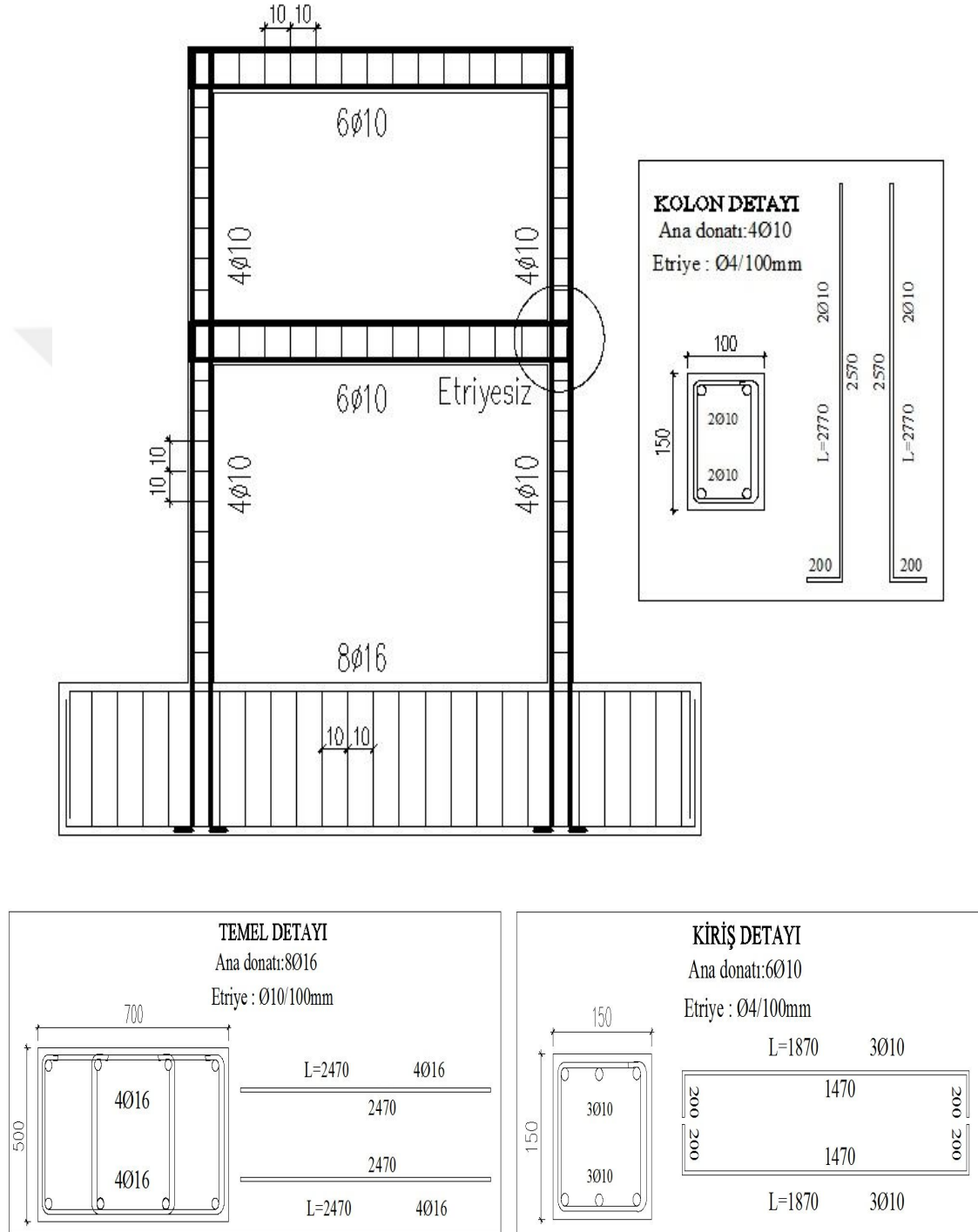
Şekil 3.2. Betonarme çerçevelerin donatı detayları.
