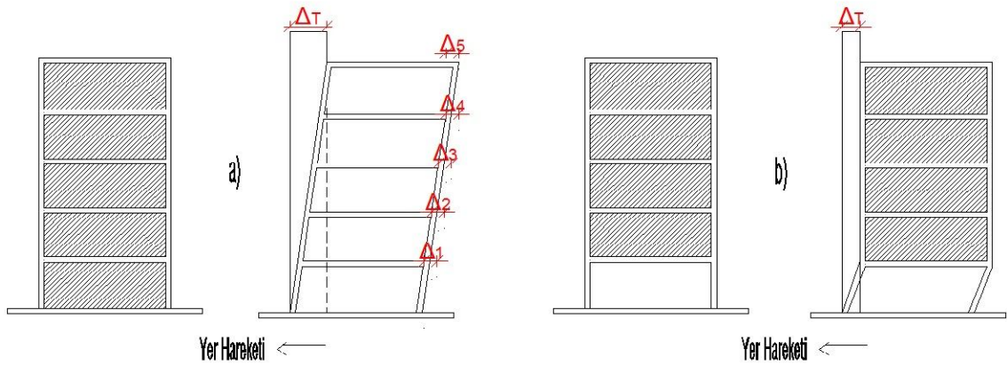
Şekil 1.8. a) Düzenli bina deplasman durumu b) Yumuşak kat düzensizliği bulunan bina deplasman durumu.
