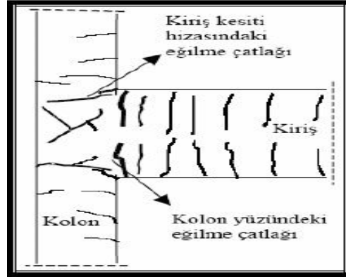
Şekil 1.13. Birleşim bölgesi çatlakları (Tonyalı, 2006)
