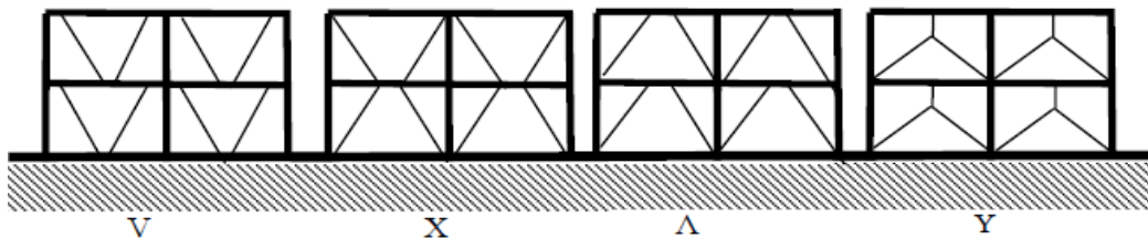
Şekil 1.15. Literatürde Mevcut Güçlendirme İçin Kullanılan Çelik Çaprazlar (Güneysisi ve Altay, 2004)
