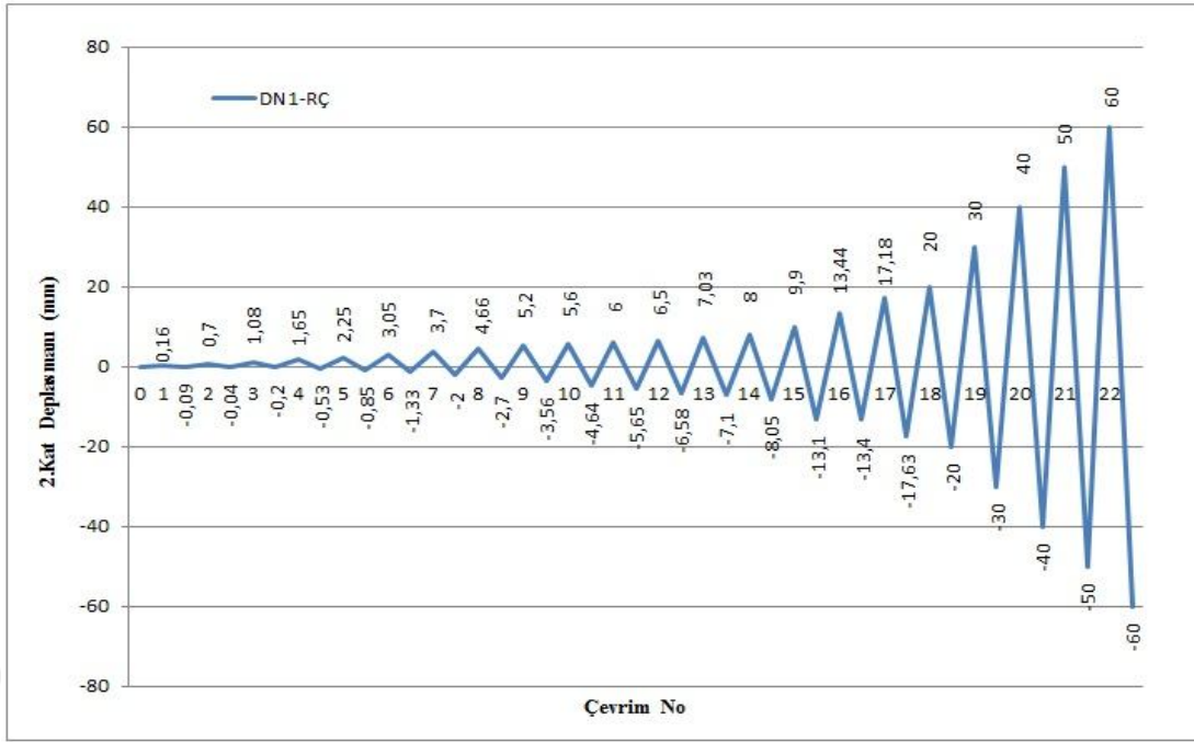
Şekil 4.3. Referans numunesinin (DN1-RÇ) tepe deplasman geçmişi.
