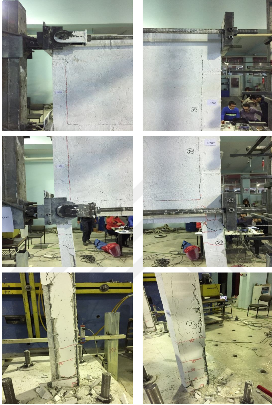
Şekil 4.15. Deney sonunda yumuşak katlı çerçeve numunesi (DN2-YKÇ) düğüm noktaları hasarları.
