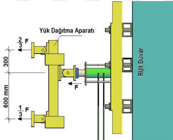
Şekil 3.21. Yükleme düzeneğinin görünümü (Ünal ve ark., 2013)
