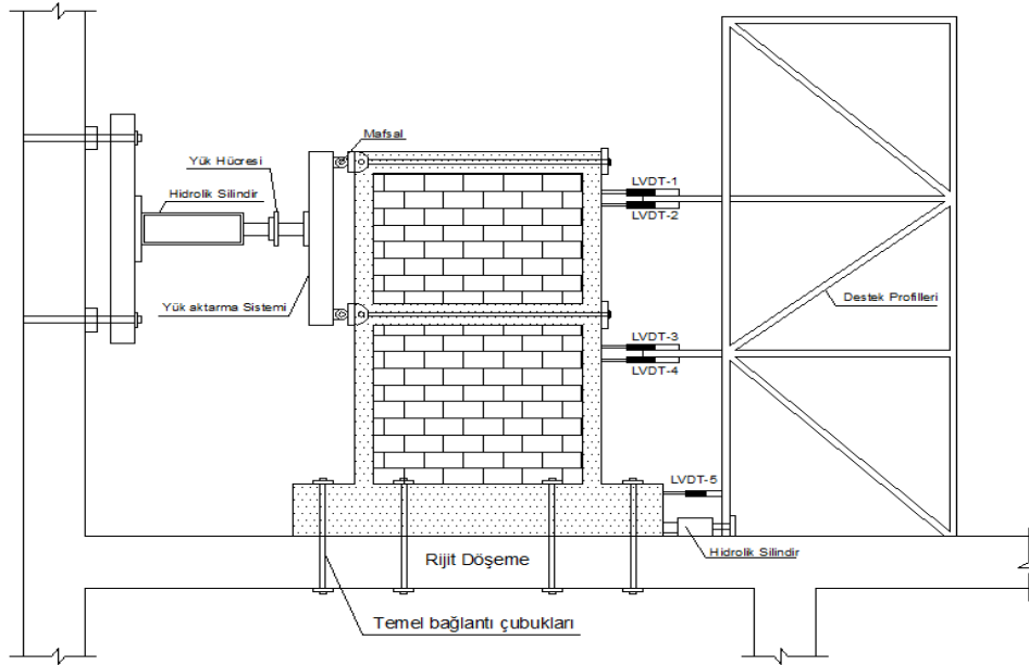
Şekil 3.25. Deneye tabi tutulan referans betonarme çerçeve.
