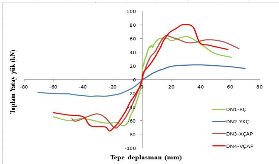
Şekil 4.38. Deney numunelerinin yatay yük – 2. kat yer değiştirmesi dayanım zarfları.
