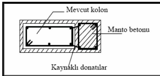
Şekil 1.11. Kolon mantolaması (Tonyalı, 2006).
