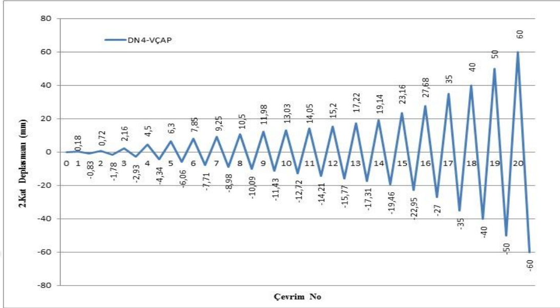
Şekil 4.30. Merkezi V çelik çapraz çerçeve numunesinin (DN4-VÇAP) tepe deplasman geçmişi.
