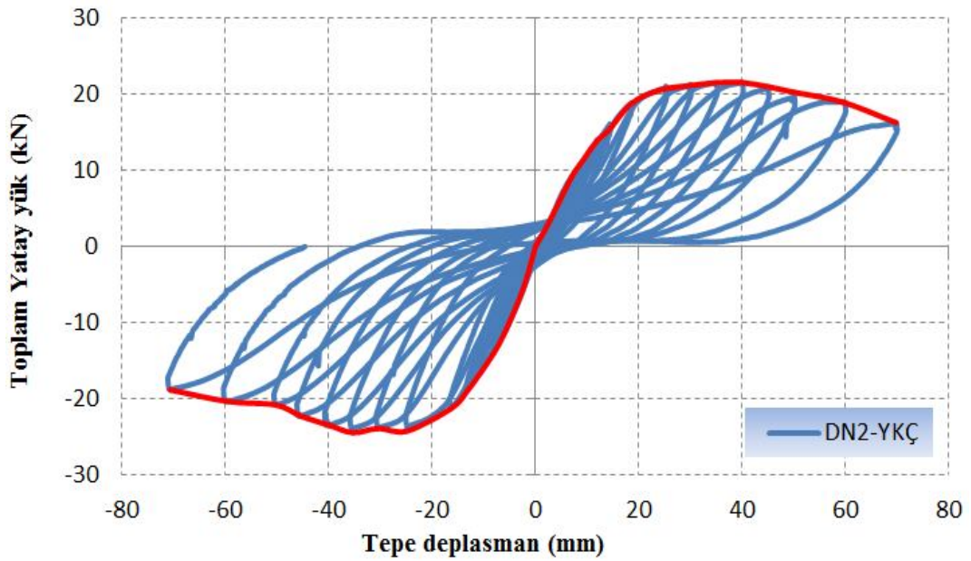
Şekil 4.17. Yumuşak katlı çerçeve numunesine (DN2-YKÇ) ait yatay yük-tepe deplasmanı çevrimsel histeresis eğrisi ve dayanım zarfı.
