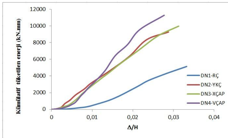
Şekil 4.39. Deney numunelerinin kümülatif toplam enerji grafikleri.
