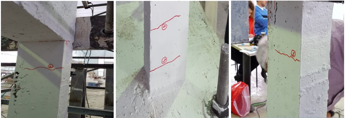
Şekil 4.13. Yumuşak katlı çerçeve numunesine (DN2-YKÇ) ait ilk çatlaklar.
