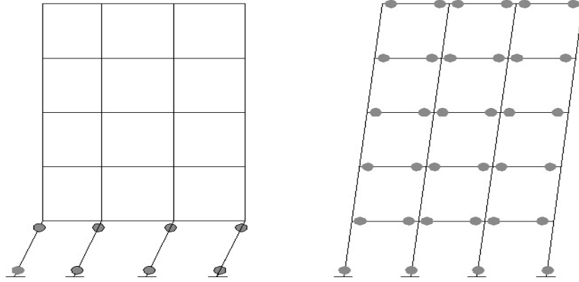
Şekil 1.9. Yumuşak kat ve ideal göçme mekanizması.
