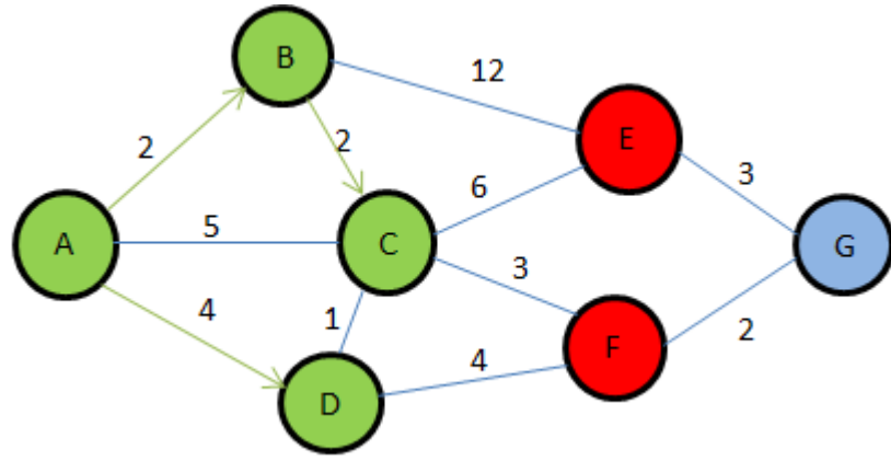
Şekil 3.8: Dijkstra algoritması görseli - 7
