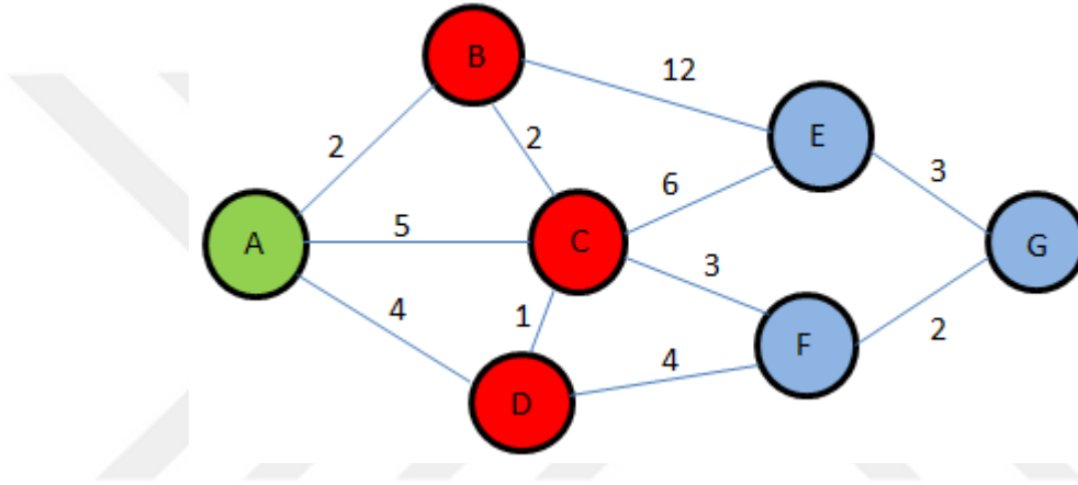
Şekil 3.2: Dijkstra algoritması görseli - 1
