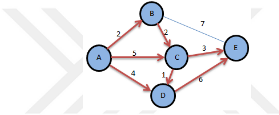
Şekil 3.19: Bellman - Ford algoritması serim gösterimi - 8
