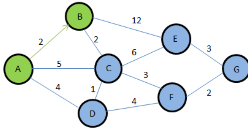
Şekil 3.3: Dijkstra algoritması görseli - 2
