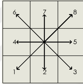
Şekil 2.5: Sekiz komşuluk
