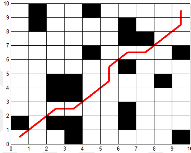
Şekil 5.4: 10x10'luk çevrede TARYPP için Bellman-Ford Algoritması sonucu
