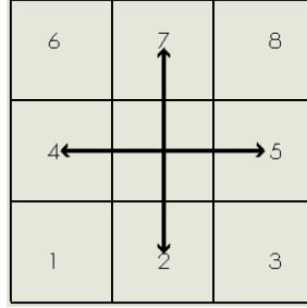
Şekil 2.4: Dört komşuluk
