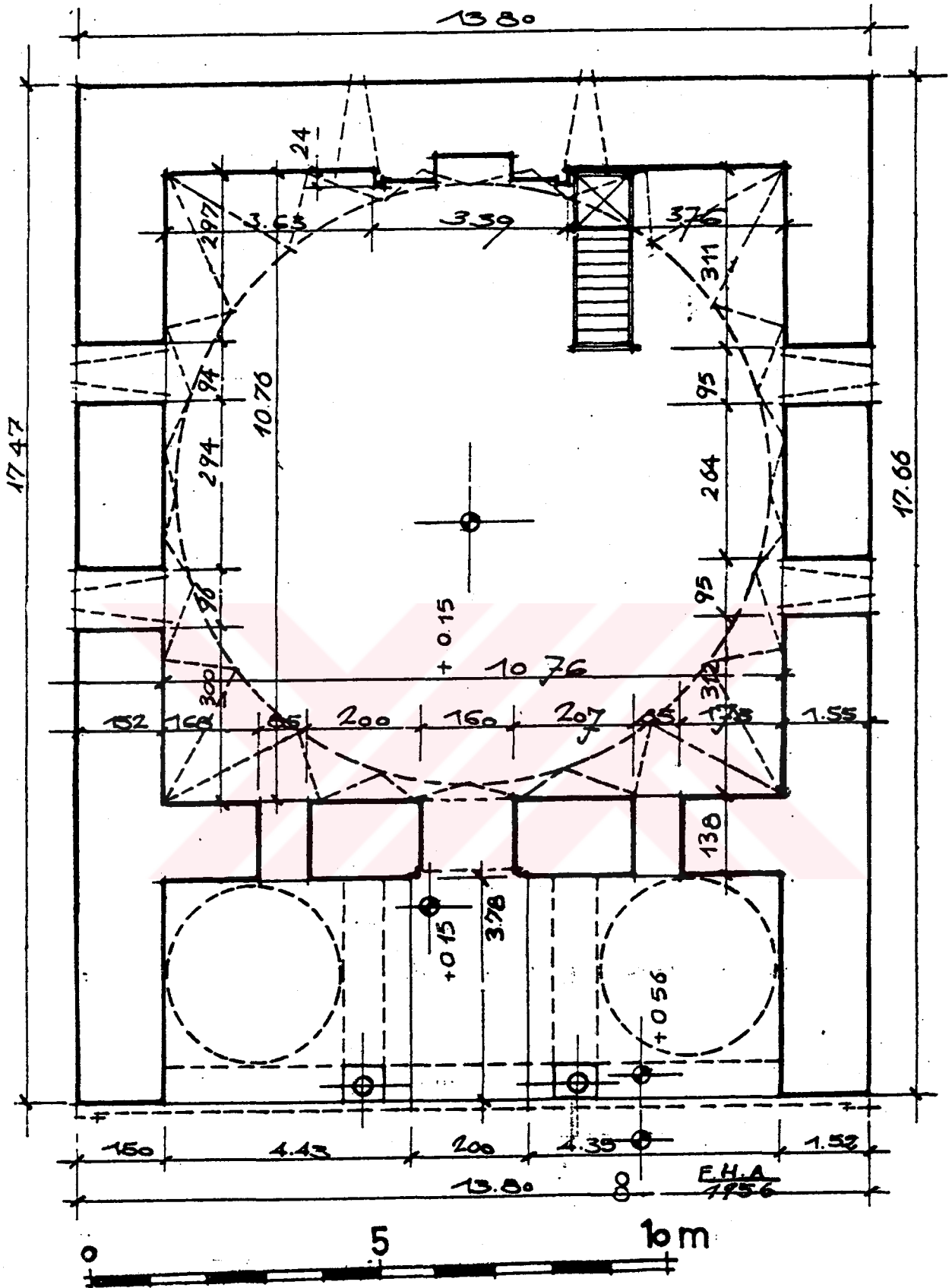
Behramkale, Hüdavendigâr Camisi Planı (1966, E.H. AYVERDİ)
