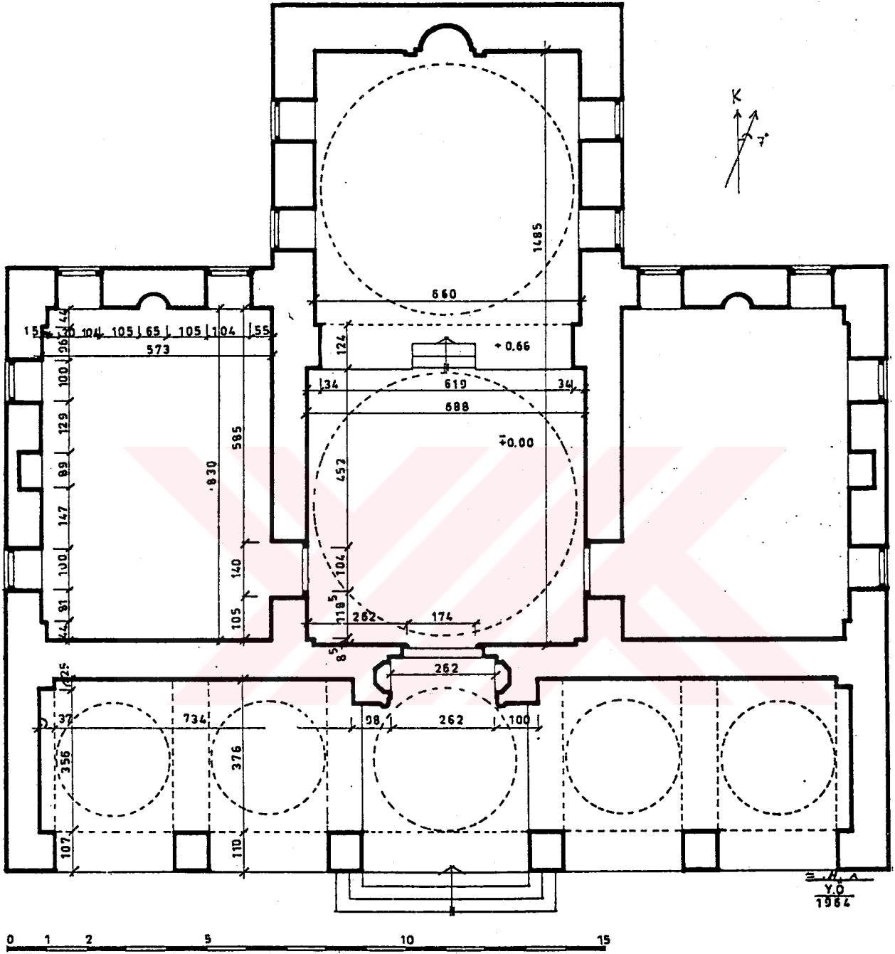
Bursa Ali Paşa Camisi Planı (1966, E.H. AYVERDİ)
