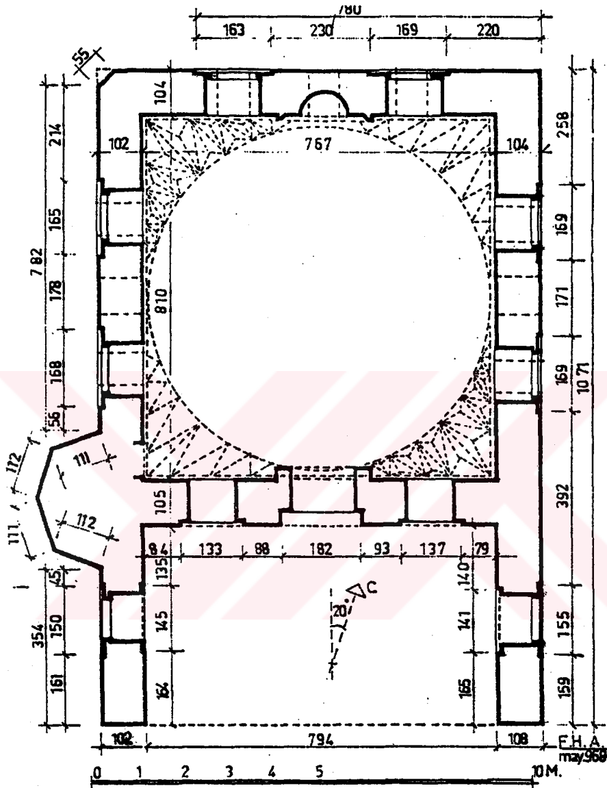
Bursa İbrahim Paşa Camisi Planı (1966, H.E. AYVERDİ)
