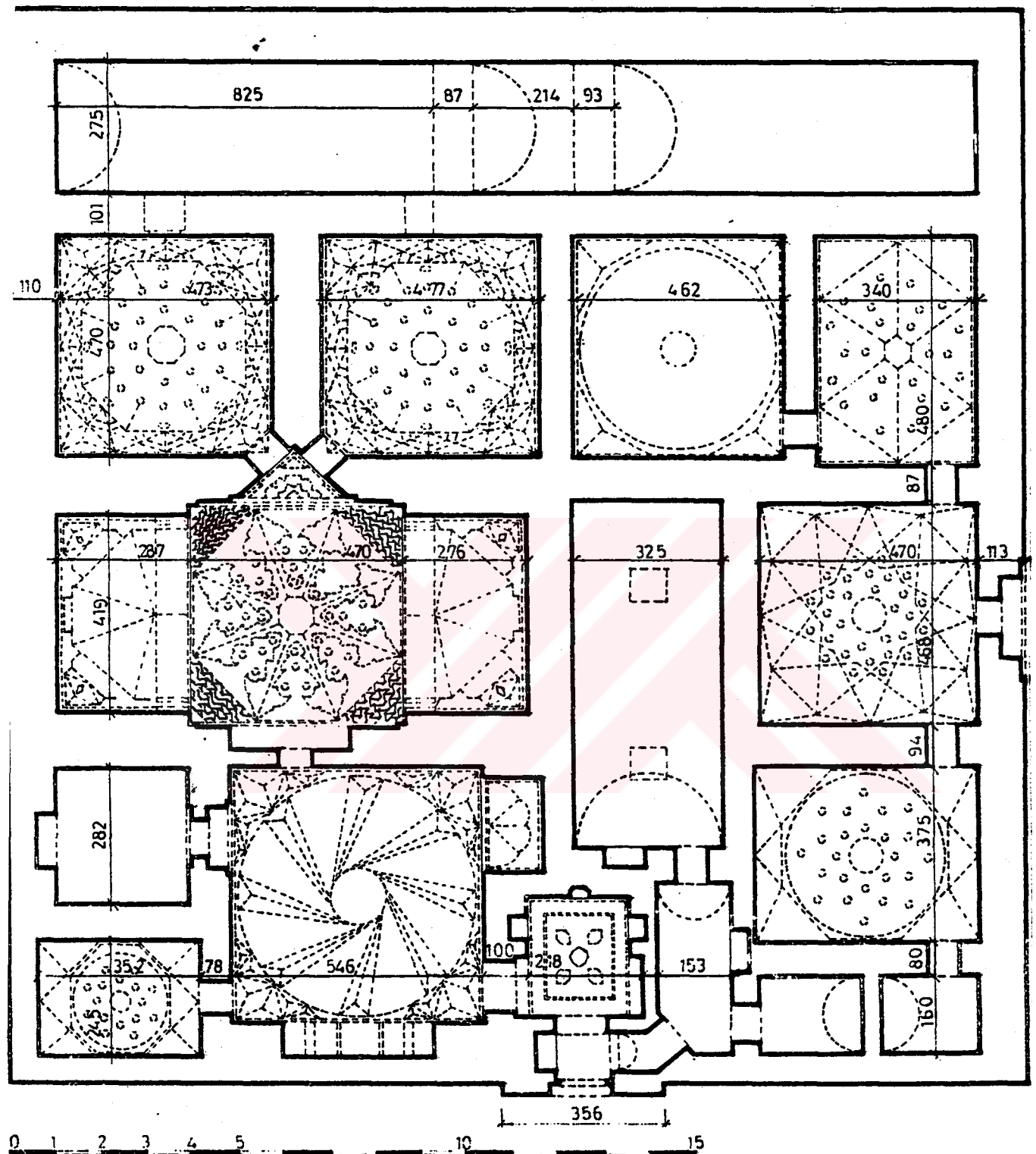
Edirne, Gazi Mihal Bey Hamamı Planı (1972, E.H. AYVERDİ).
