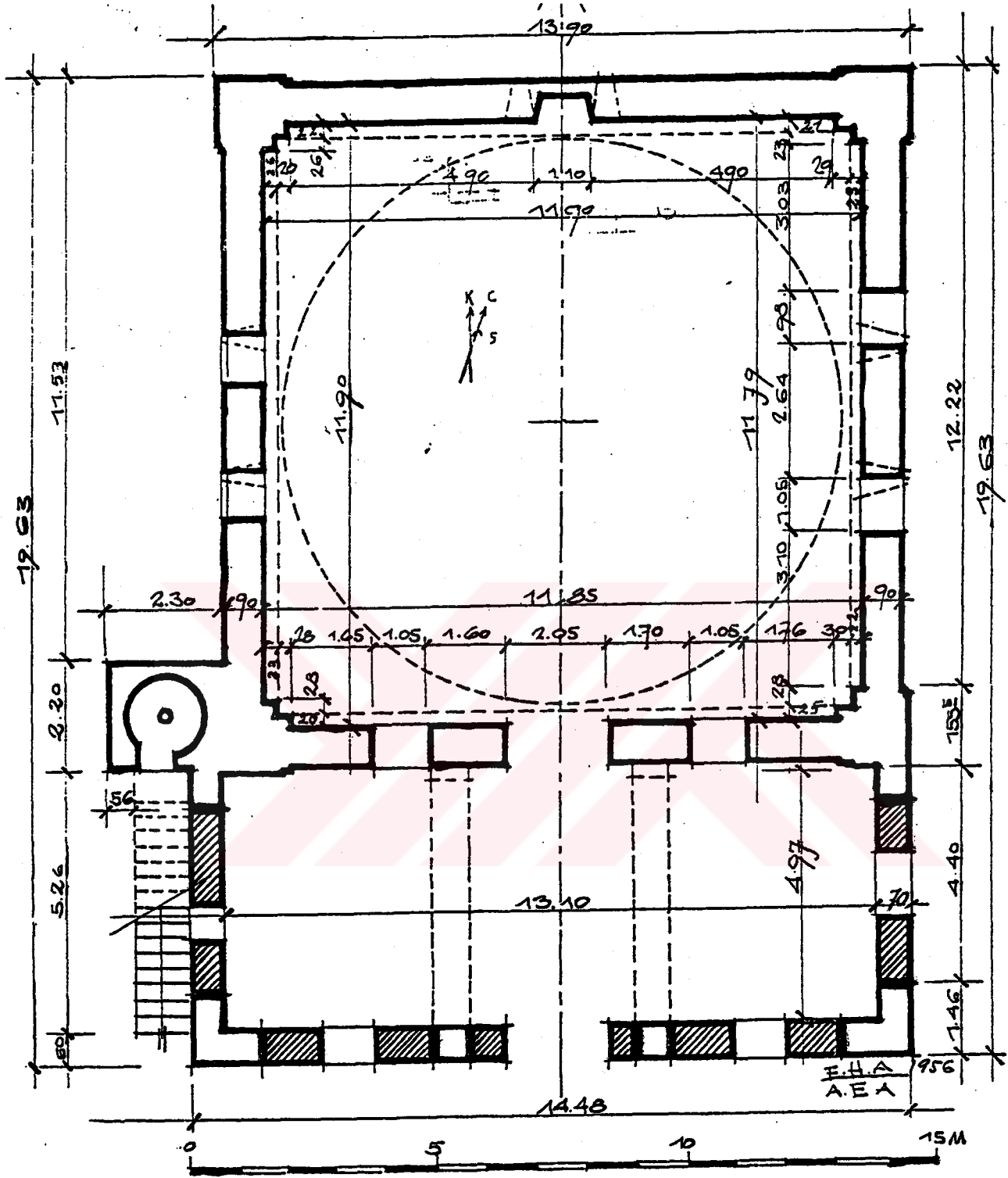
Tuzla, Hüdavendigâr Camisi Planı (1966, E.H. AYVERDİ)
