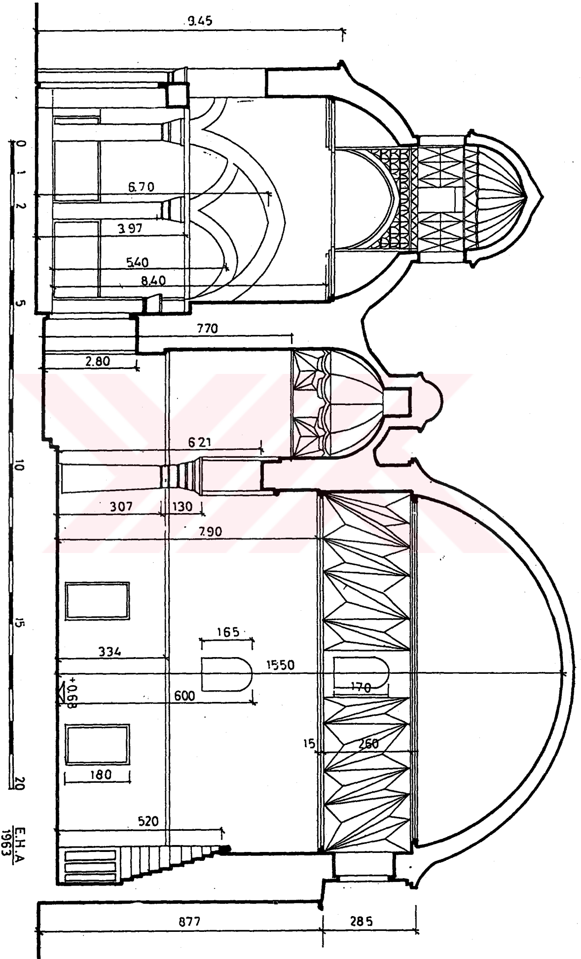
İznik Yeşil Camisi Boylamasına Kesit (1966, E.H. AYVERDİ).
