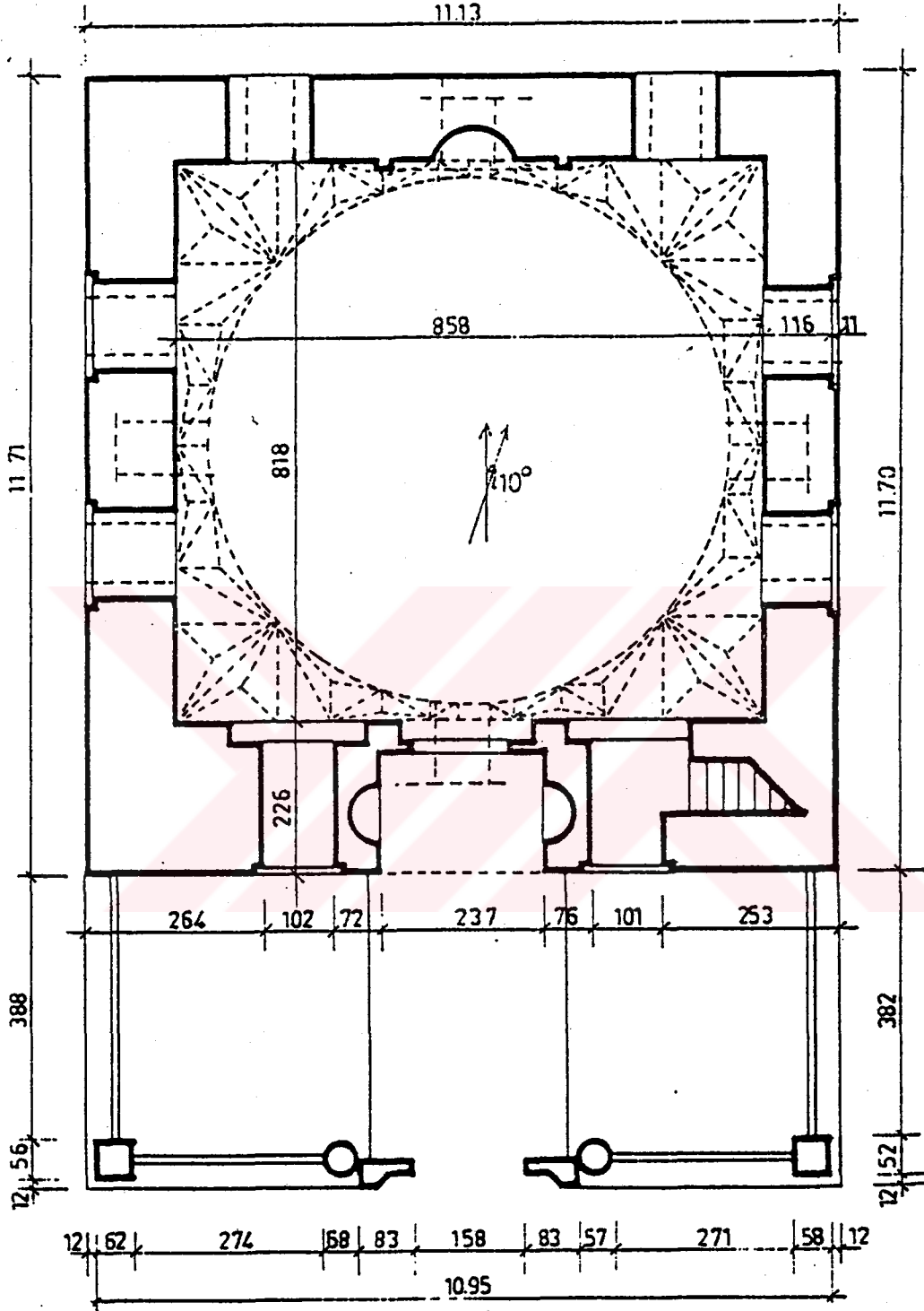
İznik Mahmut Çelebi Camisi planı (1972 E.H. AYVERDİ)
