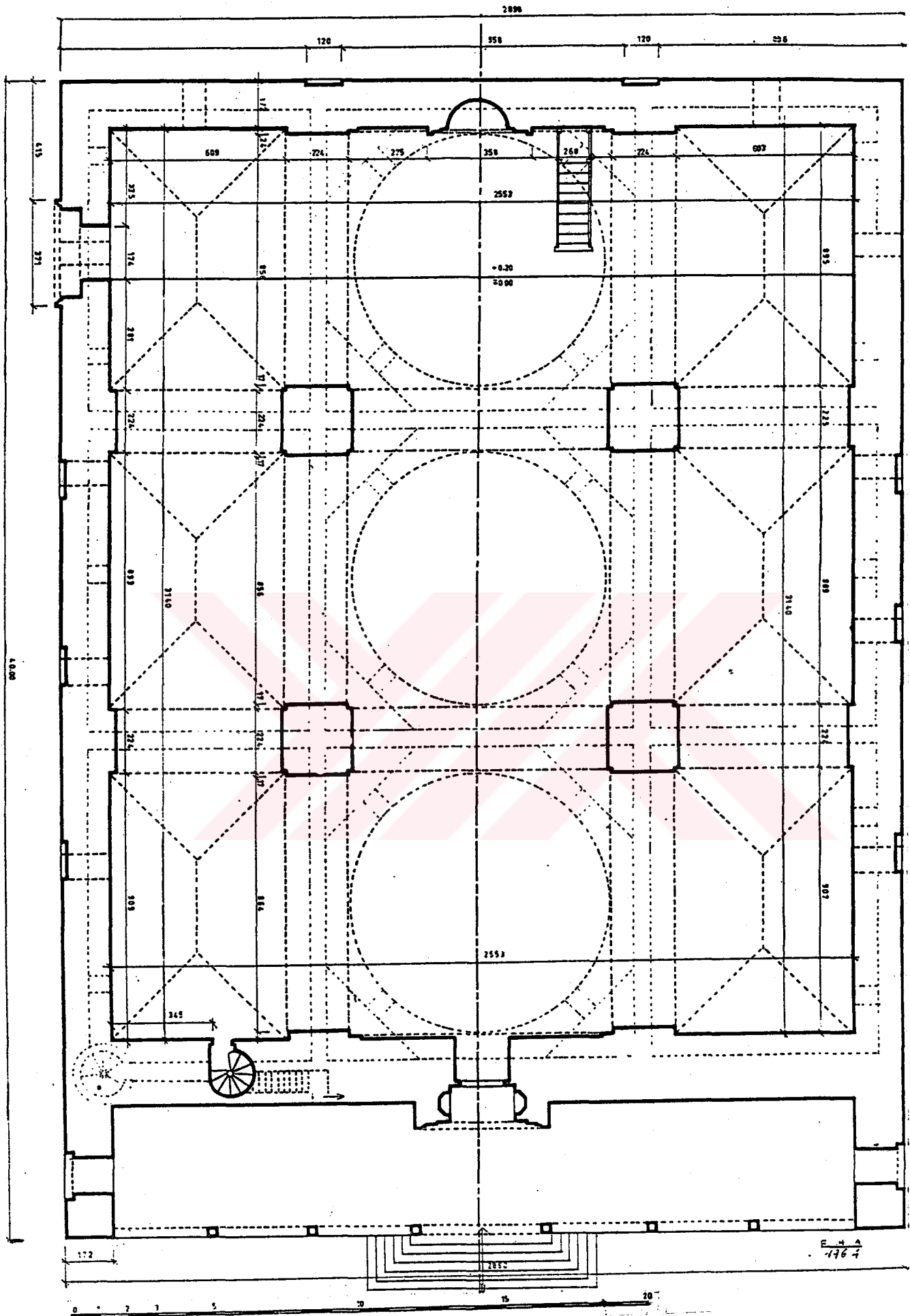
Filibe, Hüdavendigâr Camisi Planı (1966, E.H. AYVERDİ)
