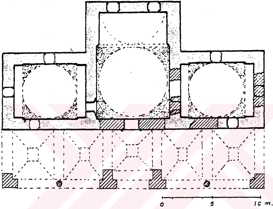
Gümülcine Gazi Evrenos Bey İmaretî Planı (1990 b, M.KİEL).
