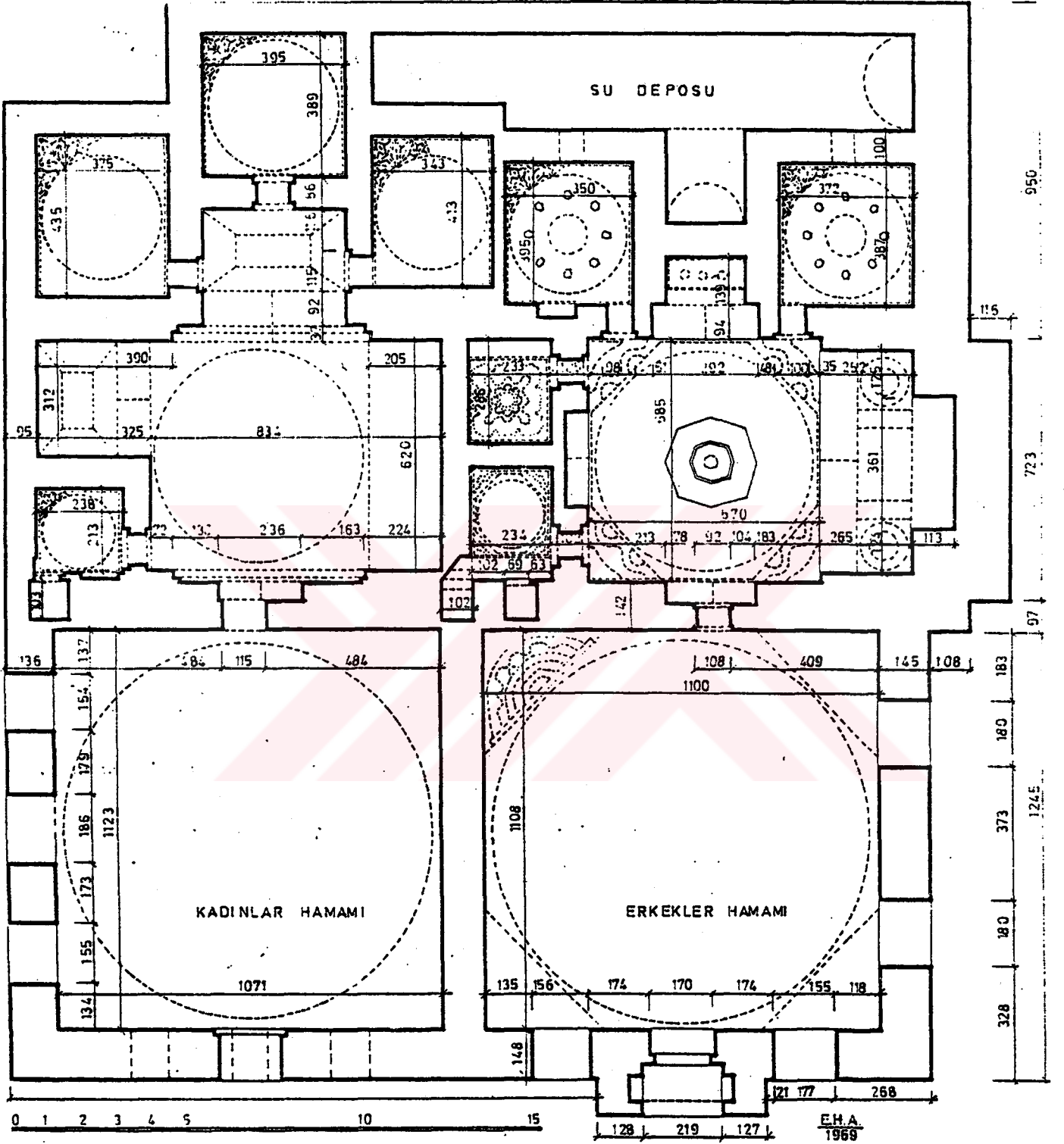
Bursa İbrahim Paşa Hamamı Planı (1966, E.H. AYVERDİ)
