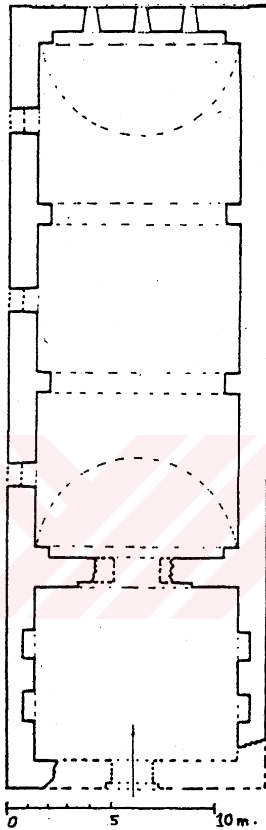
Loutra (Ilıca), Evrenos Bey Hanı Planı. (1990b, M. KİEL)
