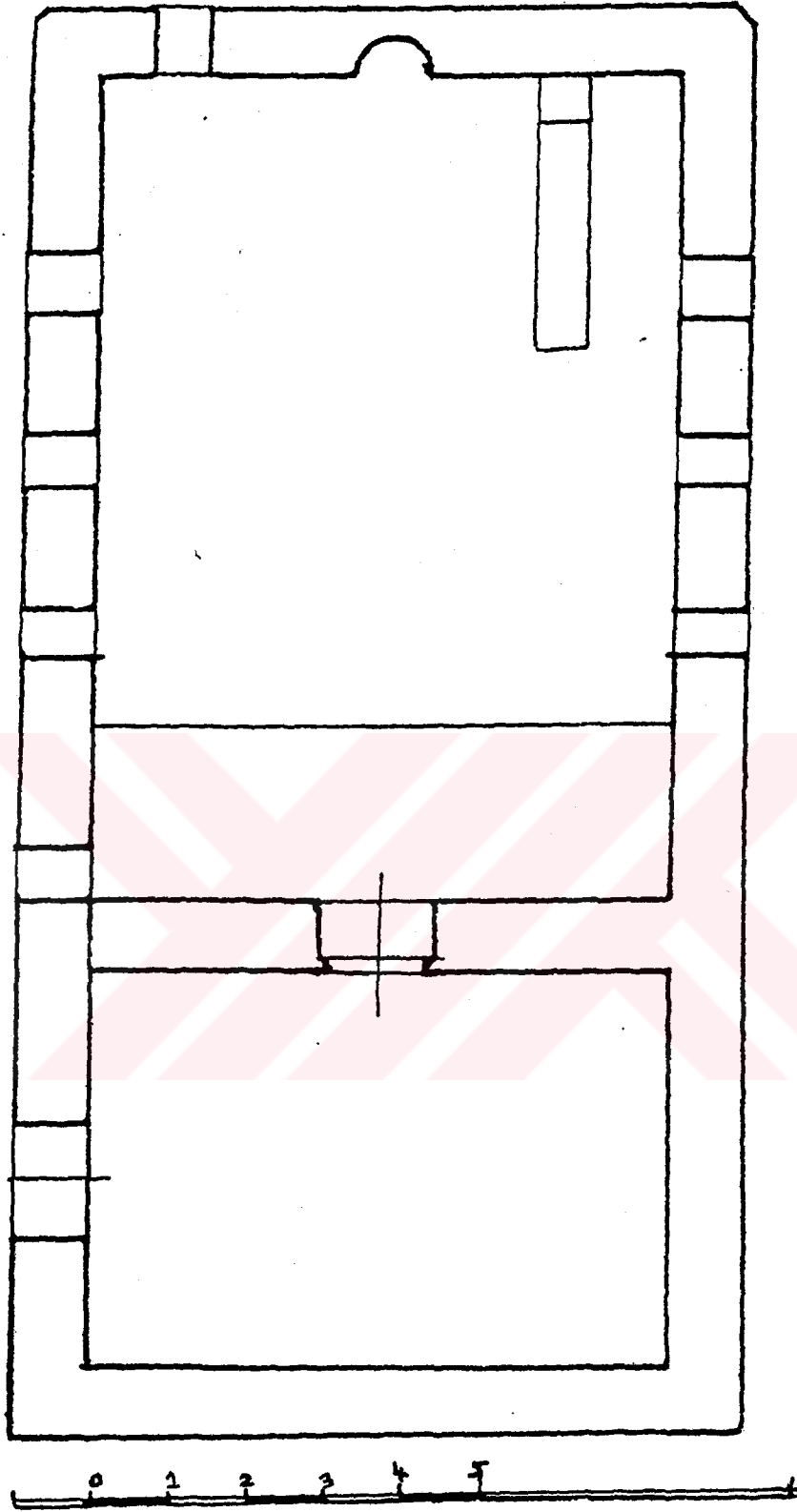
Bilecik-Gölpazarı Mihâl Bey Camisi, Planı (1977, S. ERKEN)
