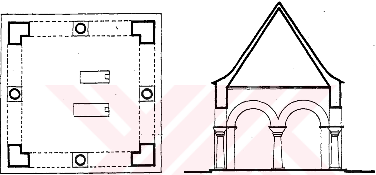
Gebze, Malkoçoğlu Mehmed Bey Türbesi Plan ve Kesiti (1966, E.H. AYVERDİ).
