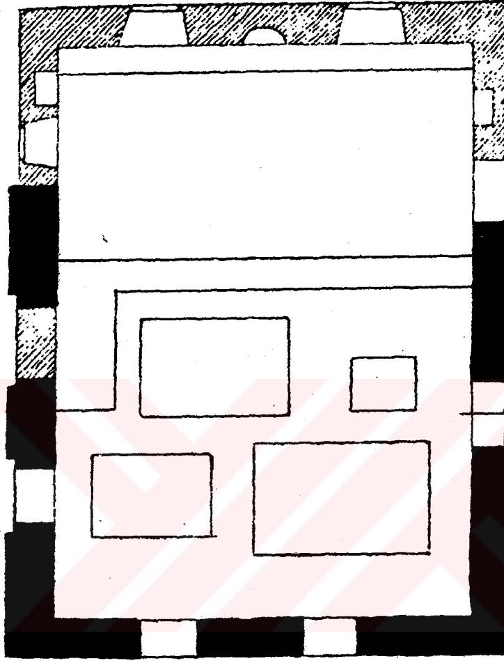
İznic Çandarlı Halil Paşa Türbesi Planı (1941, K. OTTODORN)
