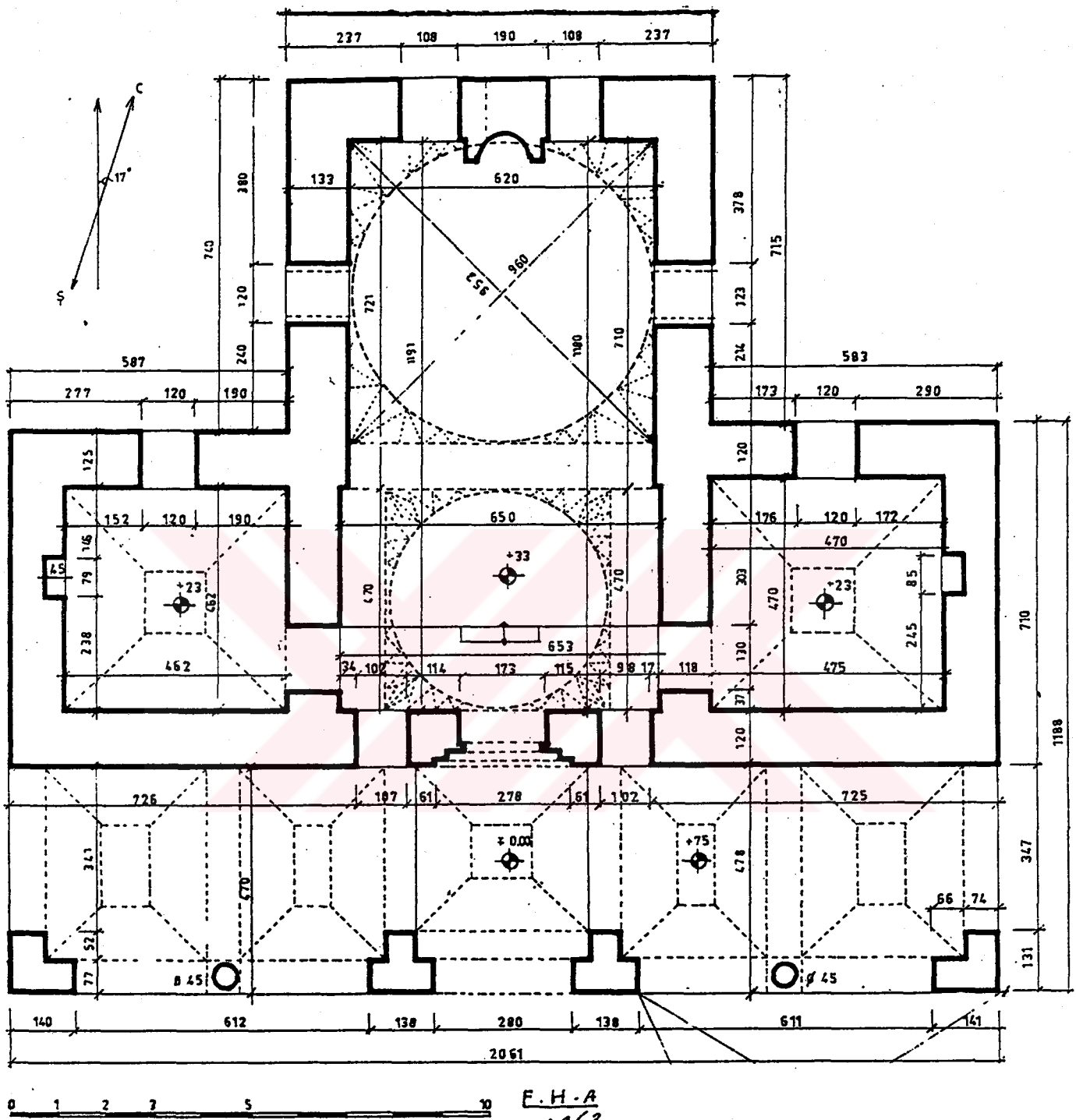
İzmir Yakup Çelebi İmaretî Planı (1972, E. H. AYVERDİ)
