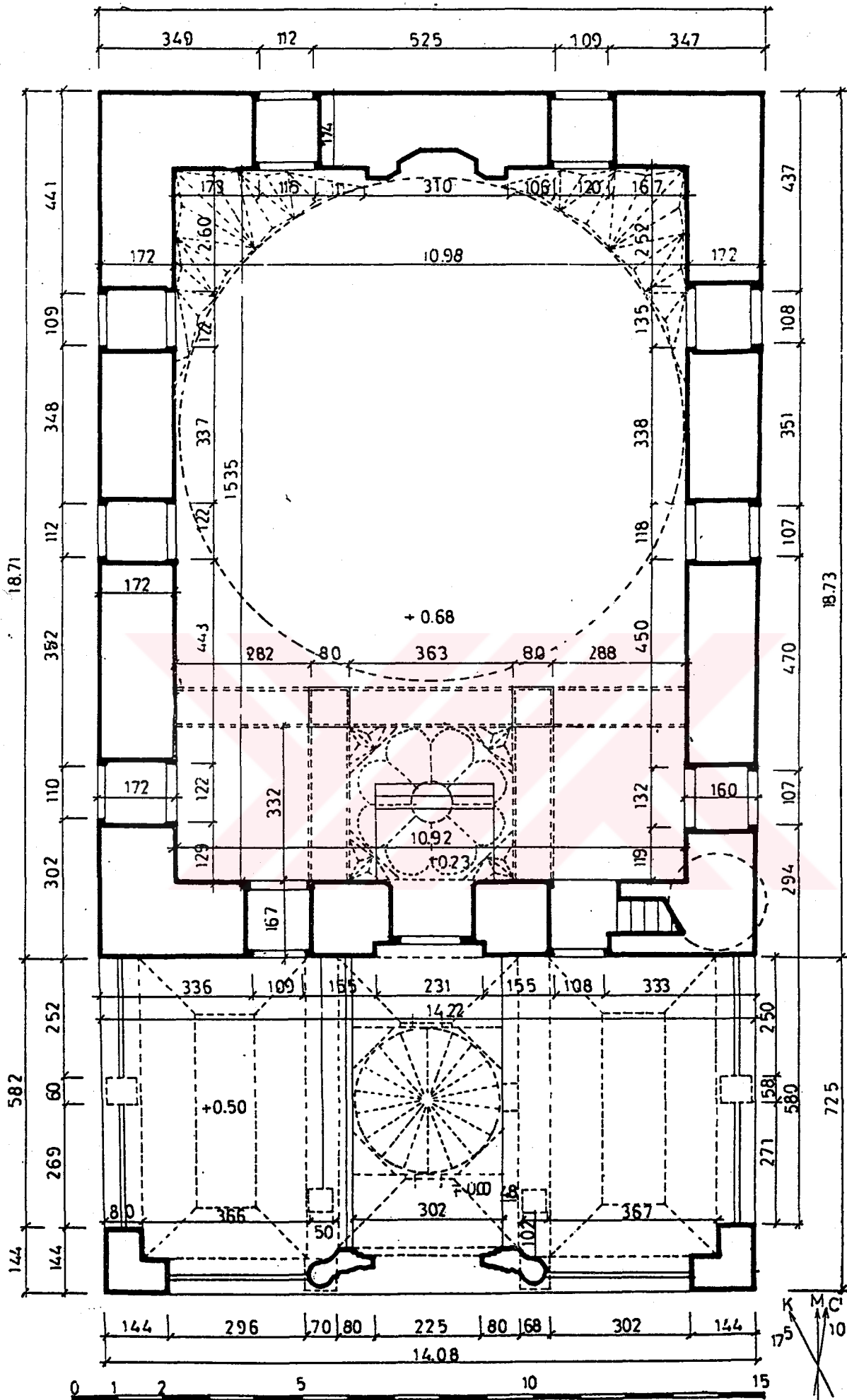
İznik Yeşil Camisi Planı (1966, E.H.AYVERDİ).
