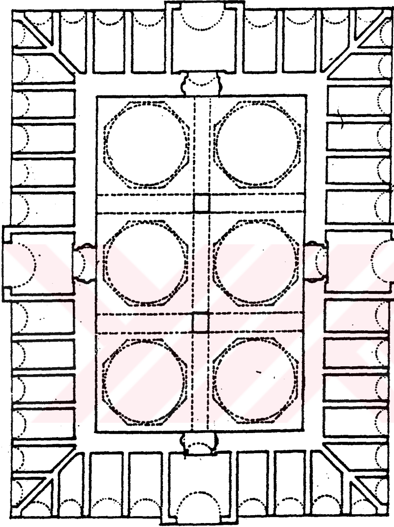
Serez Bedesteni Plan (1985, M.CEZAR)
