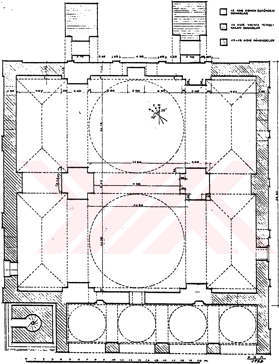
Bursa Şehadet Camisi Planı (1966, E. H. AYVERDİ)
