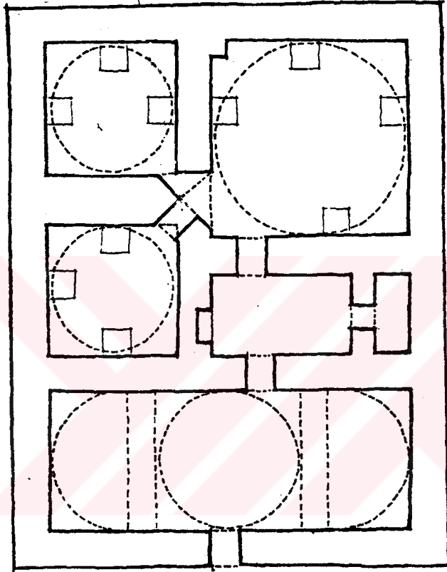
Bilecik-Gölpazarı Mihal Bey Hamamı Krokisi (1966, E.H. AYVERDİ)
