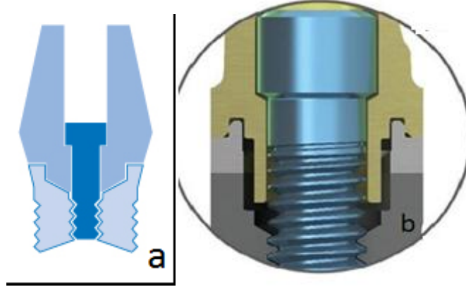
Şekil 2 a,b: İnternal altıgen bağlantı tipi (51, 53).
