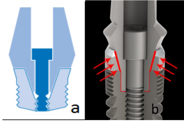
Şekil 3 a,b: Morse taper bağlantı tipi (51, 58).
