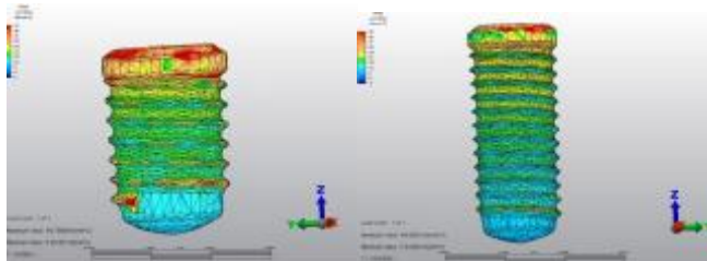
Şekil 8: 6mm ve 10 mm'lik implantlara dik kuvvet uygulanması ile görülen gerilim bölgeleri (122).
