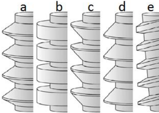
Şekil 9: Mevcut yiv şekilleri; a) V şekilli, b) kare şekilli, c) payanda şekilli, d) tersine payanda şekilli, e) spiral şekilli (136).
