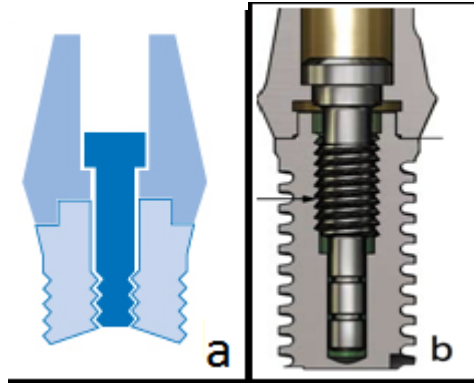
Şekil 1 a,b: Eksternal altıgen bağlantı (51, 52).
