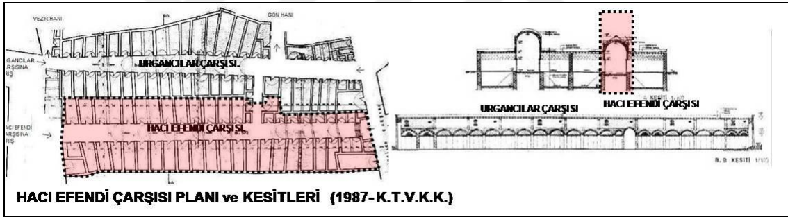
Şekil 3.50 Hacı Efendi Çarşısı plan ve kesitleri
