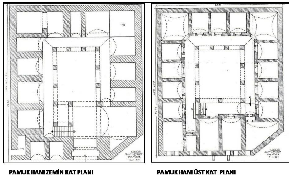
Şekil 3.25 Pamuk Hanı Zemin Kat ve Üst Kat Planı (Kayseri Vakıflar Müdürlüğü)
