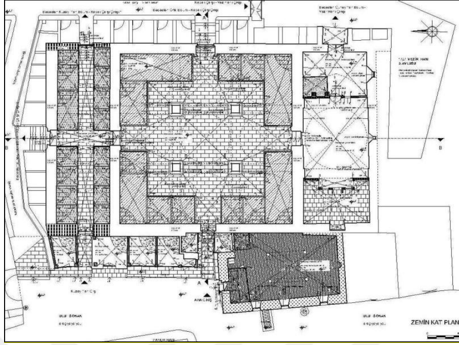
Şekil 3.29 Bedesten planı (Fernaz Öncel)
