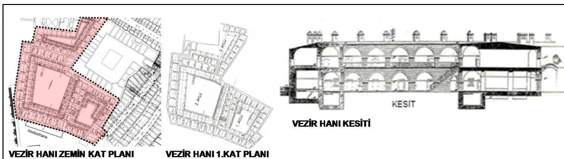
Şekil 3.47 Vezir Hanı zemin kat planı, 1. kat planı ve kesiti (K.T.V.K.K.)
