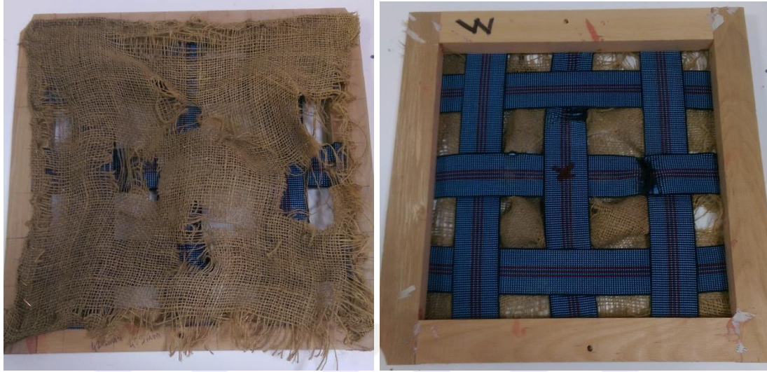
Resim 1.5. 50 mm aralıkla bağlanan astarlı elastik kolanlı döşemede deney sonu
