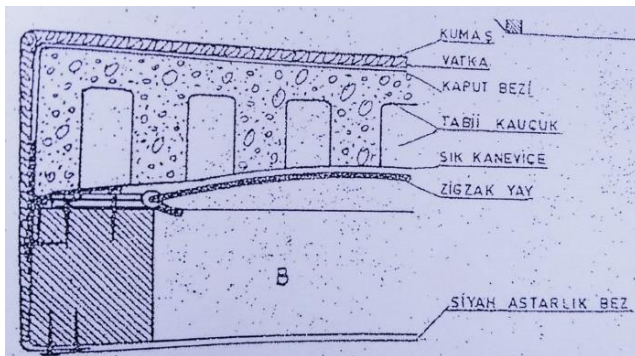
Şekil 2.22. Yay üzerine duvarlı kauçuk döşeme kesiti
