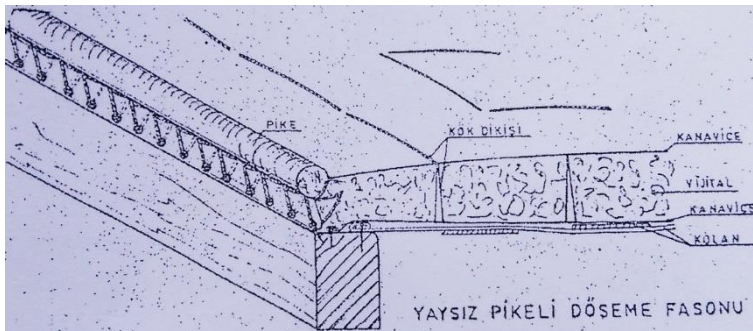
Şekil 2.24. Yaysız pikeli döşeme kesiti
