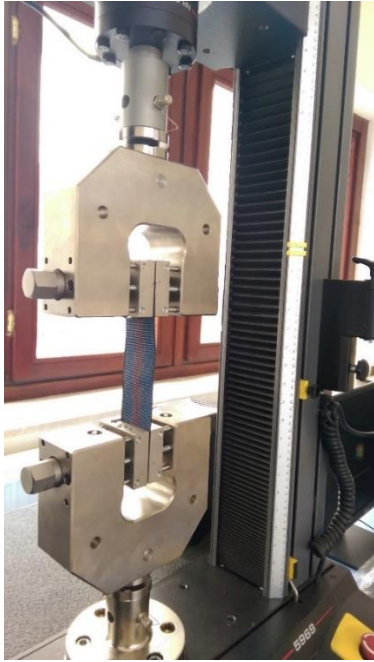
Resim 1.10. Universal test cihazında elastik kolan performans deneyi düzeneği
