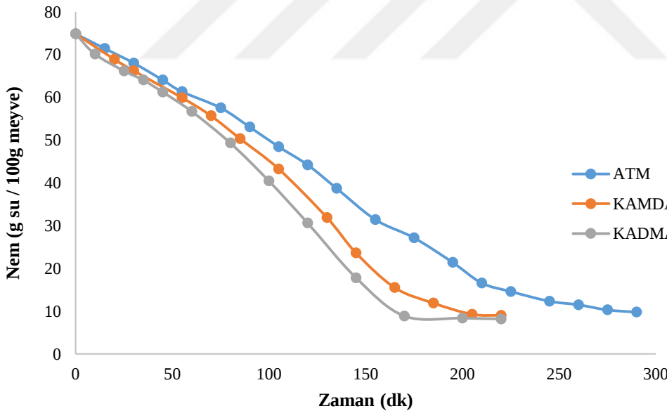
Şekil 4.12. Muzların kurutma işlemine ait kuruma eğrileri
