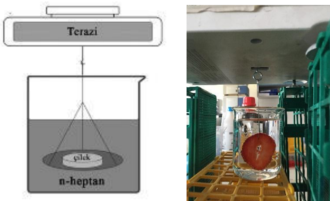
Şekil 3.10. Hacim analizi düzeneği
