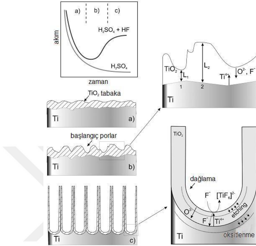
Şekil 4.2 Anotlama ile nanotüp/nanopor oluşum mekanizması Sol üst köşede: Flor katkılı ve katkısız elektrolit içinde titanyumun oksitlenmesi ile oluşan akım-zaman eğrisi a) Bariyer tabakasının oluşumu b) nanotüp oluşum başlangıcı c) anotla sonucu oluşan \text{TiO}_2 nanotüplerin nihai hali (Bavykin ve Walsh, 2010).
