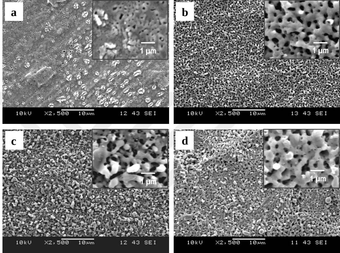
Şekil 6.19 \text{H}_2\text{SO}_4 içerikli elektrolit içinde anotlanan mikro poroz \text{TiO}_2 kaplamalarının SEM görüntüleri (a) HS-100 (b) HS-150 (c) HS-200 (d) HS-250
