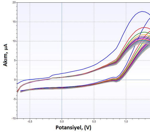
Şekil 4.1. DTP(aril)anilin'in elektropolimerizasyonu [(1:1 ACN/DCM ortamında 15 döngülü voltamogram (-0,7V-1,4 V, 0,1 V/s)]
