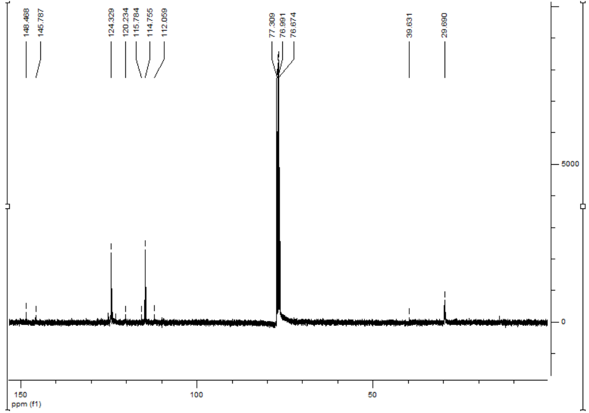
EK 1- 4-(4H-ditiyol [3,2-b:2',3'-d]pirol-4-il)anilin (N-Ph-NH 2 monomerinin) 100 MHz 13 C-NMR spektrumu 110-150ppm arası açılmış spektrum (CDCl 3 )
