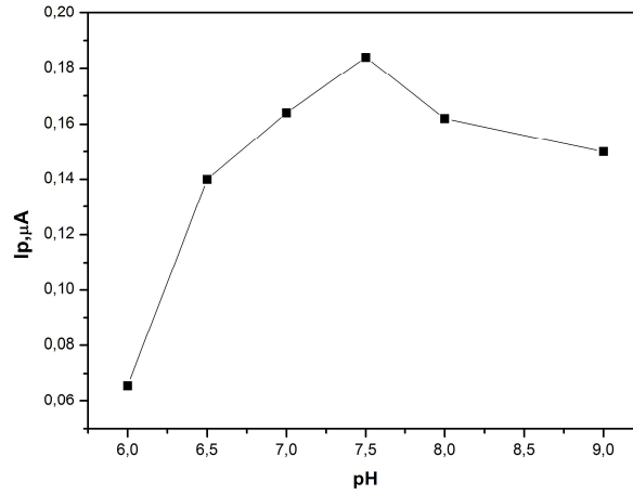
Şekil 4.5. DTP(aril)anilin modifiye elektrot cevabına pH’nın etkisi (0,1M PBS, Kolesterol derişimi; 19,8µM, -0,7V, 0,1V/s, oda sıcaklığı)
