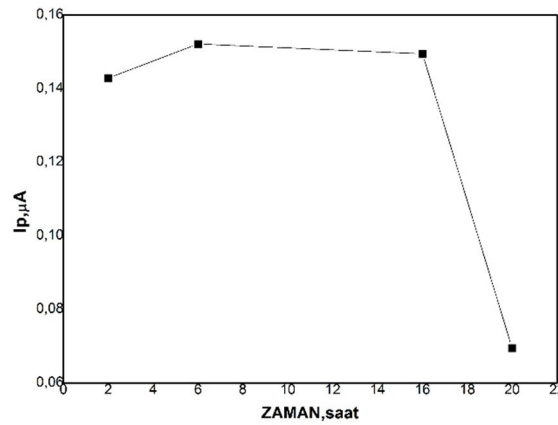
Şekil 4.4. DTP(aril)anilin modifiye elektrot cevabına immobilizasyon süresinin etkisi (0,1M PBS pH 7,5, -0,7V, 0,1V/s, oda sıcaklığı)
