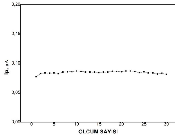
Şekil 4.9. DTP(aril)anilin modifiye COx enzim elektrodunun tekrarlanabilirlik ve operasyonel stabilite çalışması (0,1M PBS pH 7,5, -0,7V, 0,1V/s, oda sıcaklığı, kolesterol derişimi, 19,8 µM)
