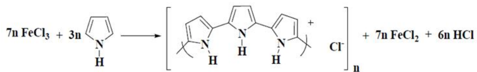
Şekil 1.6. Pirolün demir (III) klorür ile kimyasal polimerizasyonu
