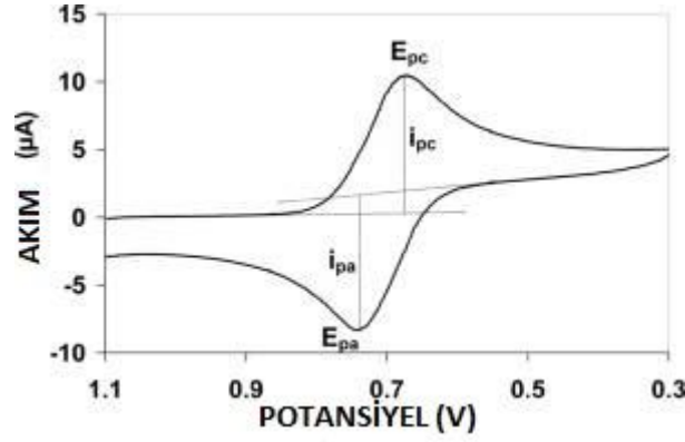
Şekil 1.15. Şekil CV Akım/Potansiyel eğrisi
