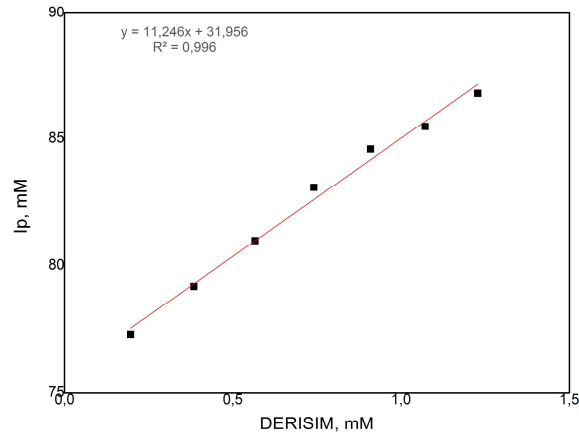
Şekil 4.3. DTP(aril) anilin ile modifiye edilmiş elektrodun H_2O_2 cevabı (0,1M PBS pH 7,5, -0,7V, 250s, 0,1V/s, oda sıcaklığı)
