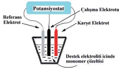
Şekil 1.7. Elektroliz hücresi
