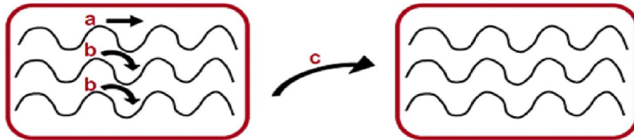
Şekil 1.5. a-Zincir üzerinde yükün taşınması, b-Zincirlerin arasında yükün taşınması, c-Partiküller arasında yükün taşınması
