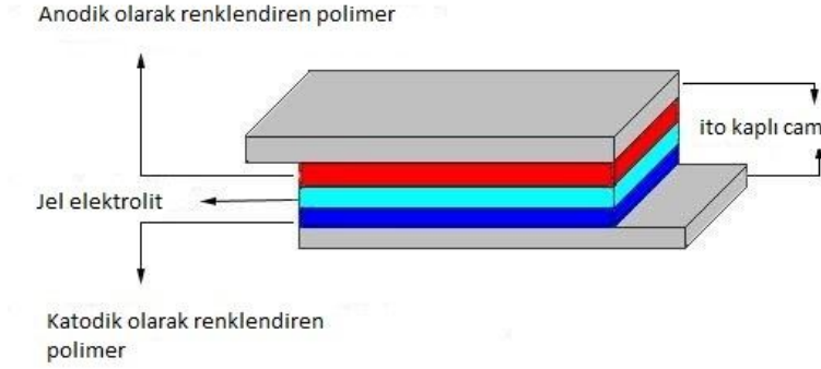
Şekil 1.10. Elektrokromik materyal çalışma prensibi
