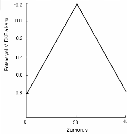
Şekil 1.14. CV için potansiyel – zaman eğrisi
