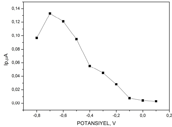
Şekil 4.6. DTP(aril)anilin modifiye elektrot cevabına çalışma potansiyelinin etkisi (0,1M PBS, Kolesterol derişimi; 19,8µM, pH 7,5, 0,1V/s, oda sıcaklığı)
