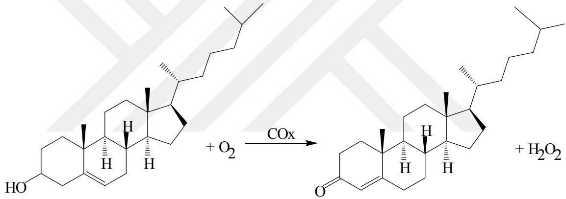
Şekil 1.24. COx enzimi çalışma mekanizması
