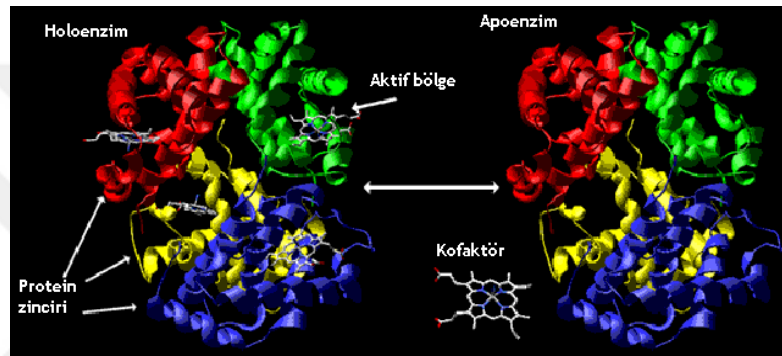
Şekil 1.20. Enzim yapısı
