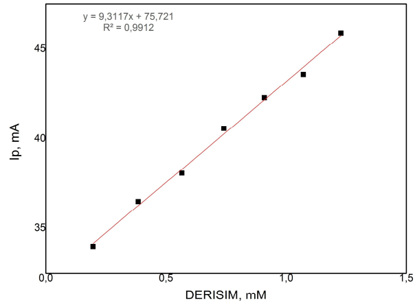
Şekil 4.2. Modifiye edilmemiş çıplak elektrodun H_2O_2 cevabı (0,1M PBS pH 7,5, -0,7V, 250s, 0,1V/s, oda sıcaklığı)
