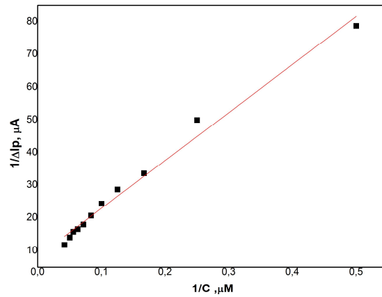
Şekil 4.10. DTP(aril)anilin modifiye kolesterol oksidaz enzim elektrodunun aktivitesinin belirlenmesi için çizilen Lineweaver Burk eğrisi (0,1M PBS pH 7,5, oda sıcaklığı, -0,7V, Kolesterol derişimi 19,8 \mu M )
