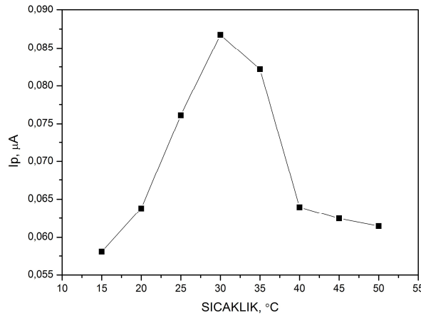
Şekil 4.7. DTP(aril)anilin modifiye elektrot cevabına sıcaklığın etkisi (0,1M PBS, pH 7,5, Kolesterol derişimi; 19,8 \mu M, -0,7V, 0,1V/s)
