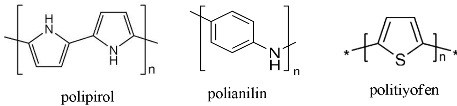
Şekil 1.2. Bazı iletken polimerler
