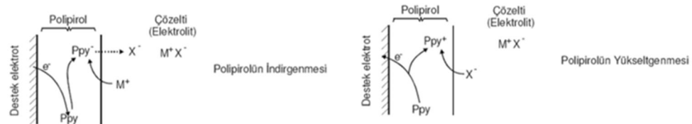
Şekil 1.9. Polipirol'ün indirgenmesi ve yükseltgenmesi
