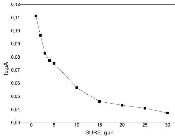
Şekil 4.11. DTP(aril)anilin modifiye kolesterol oksidaz enzim elektrodunun raf ömrü (0,1M PBS pH 7,5, oda sıcaklığı, -0,7V, Kolesterol derişimi 19,8 \mu M )
