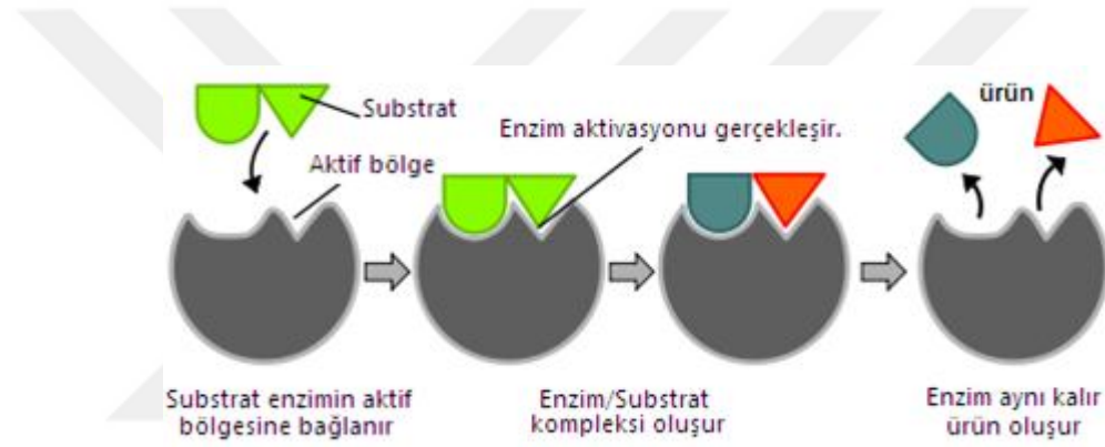
Şekil 1.21. Enzim-substrat kompleksinin oluşması
