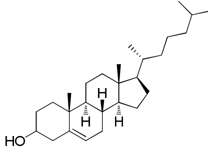
Şekil 1.1. Kolesterolün yapısı
