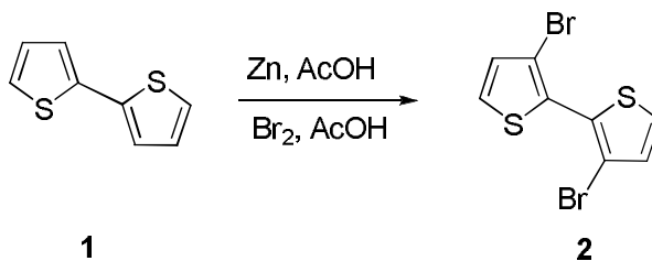
Şekil 3.1. 3,3'-dibrom-2,2'-bitiyofen (2) sentezi
