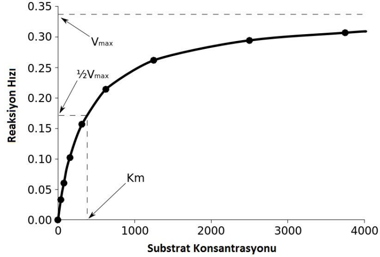
Şekil 1.22. Reaksiyon hızı-substrat derişimi grafiği
