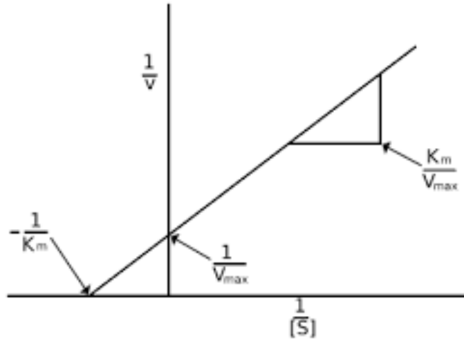
Şekil 1.23. Lineweaver-Burk eğrisi
