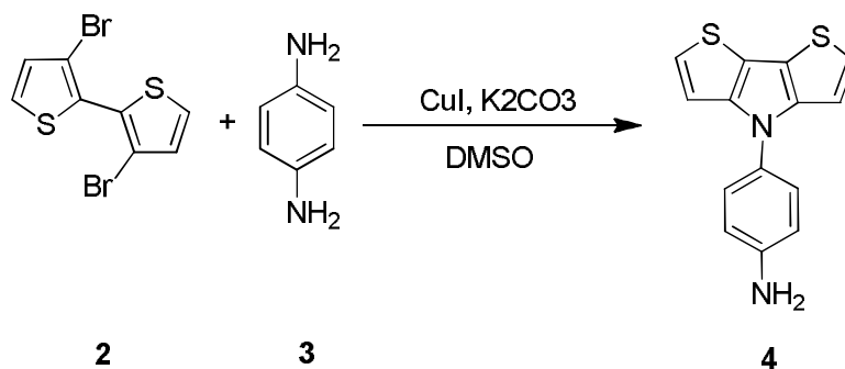
Şekil 3.2. 4-(4H-ditiyol[3,2-b:2',3'-d]pirol-4-il)anilin sentezi
