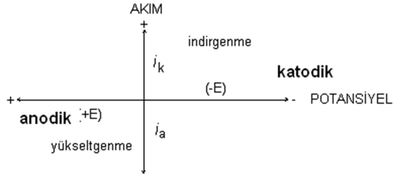
Şekil 1.13. Voltamogram çizim prensibi
