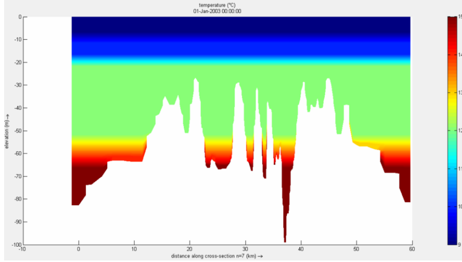
Şekil 4.8 : İstanbul Boğazı'nın başlangıç sıcaklık değerlerini gösteren boykesit.
