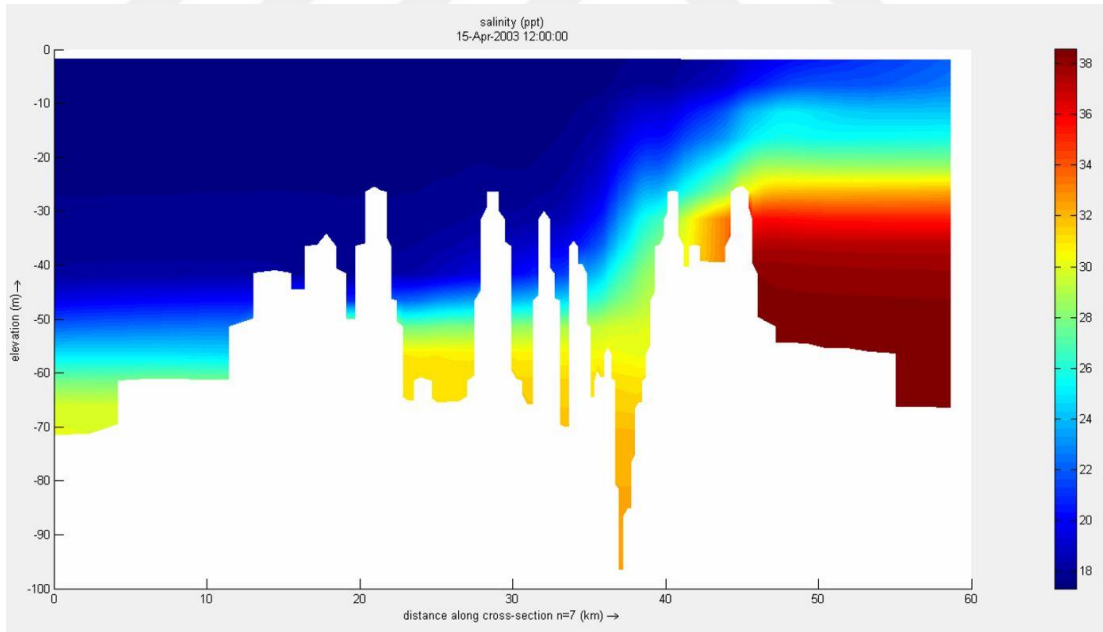
Şekil 5.17 : 15 Nisan 2003 tarihine ait İstanbul Boğazı boykesiti tuzluluk profili.
