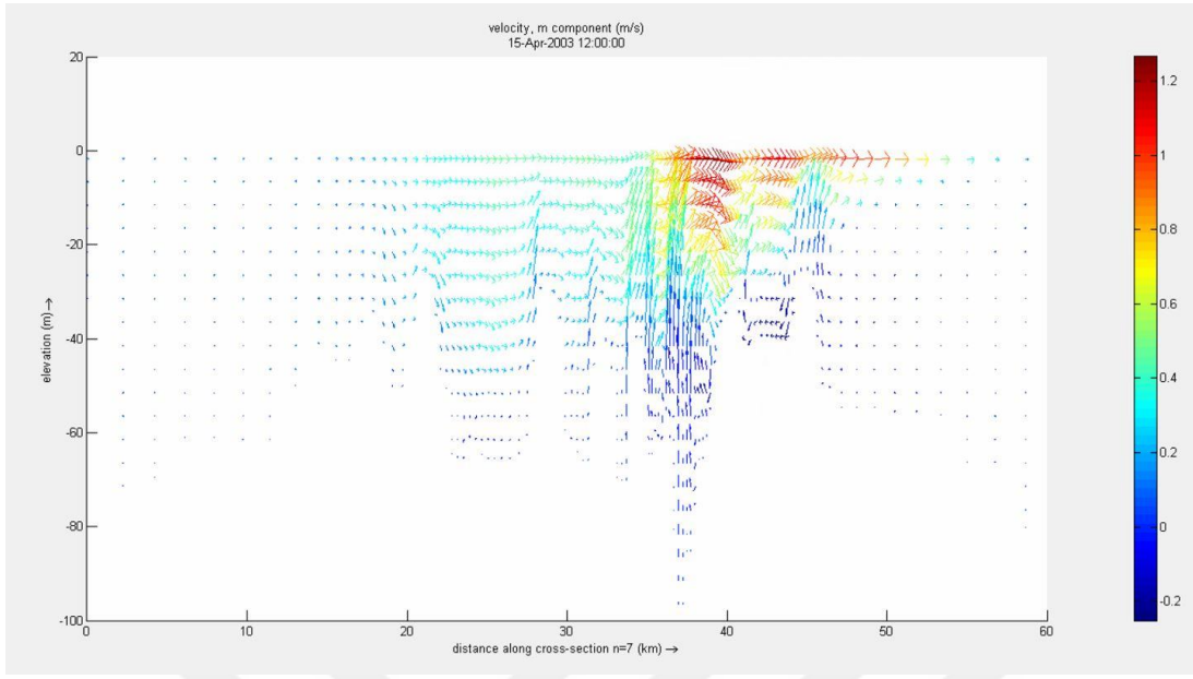
Şekil 5.25 : 15 Nisan 2003 tarihine ait İstanbul Boğazı boykesiti hız profili.
