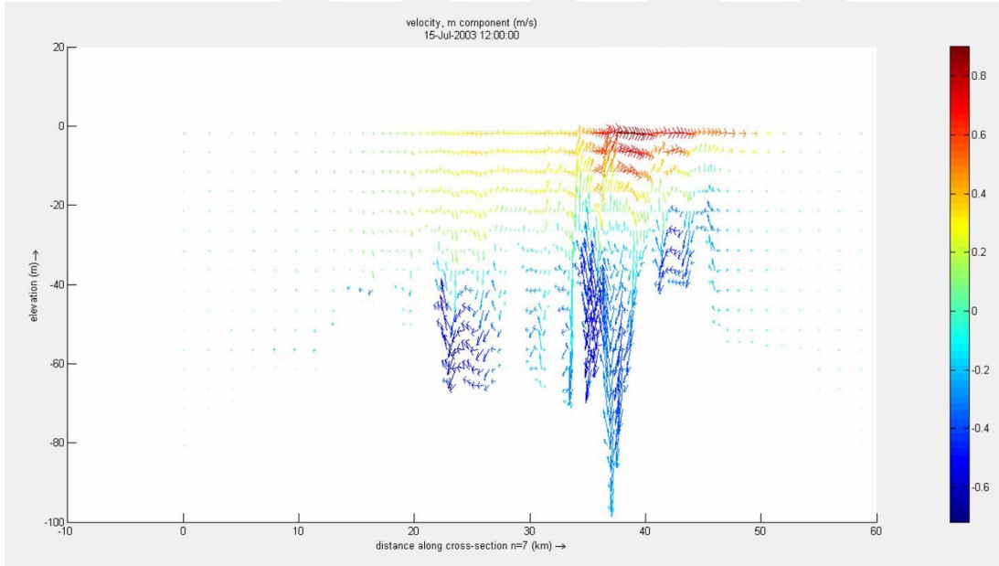
Şekil 5.26 : 15 Temmuz 2003 tarihine ait İstanbul Boğazı boykesiti hız profili.
