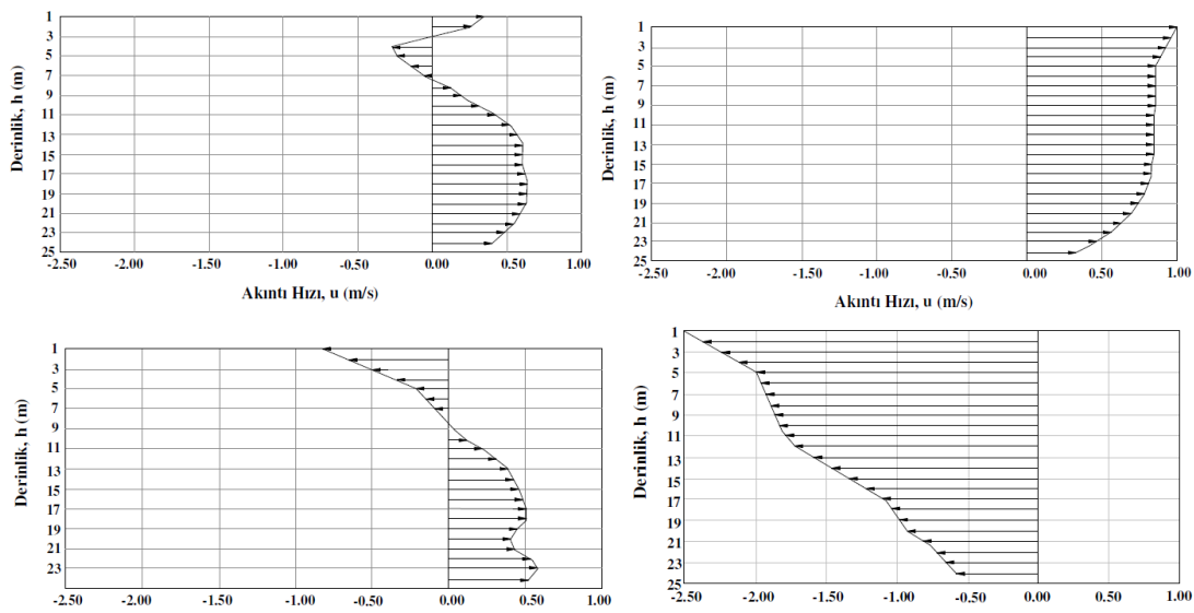
Şekil 2.4 : İstanbul Boğazı’nın güney eşiği üzerinde 4 farklı tipte oluşan hız profili (Yüksel vd., 2008).
