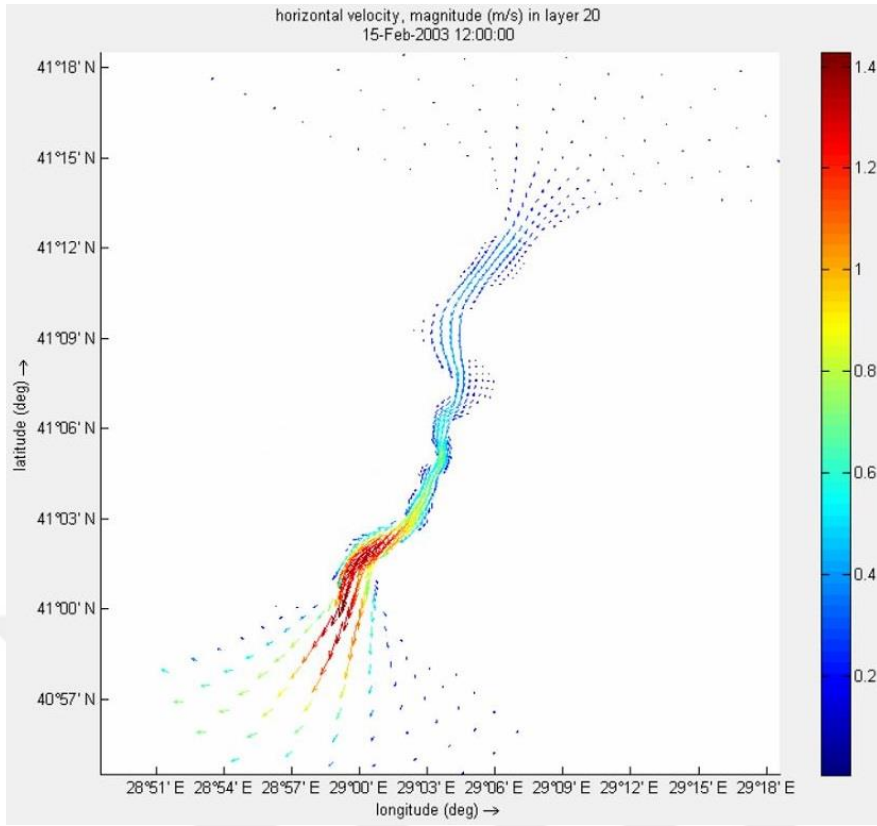
Şekil 5.28 : 15 Şubat 2003 tarihinde İstanbul Boğazı'nda 5 m derinlikte hız vektörleri.
