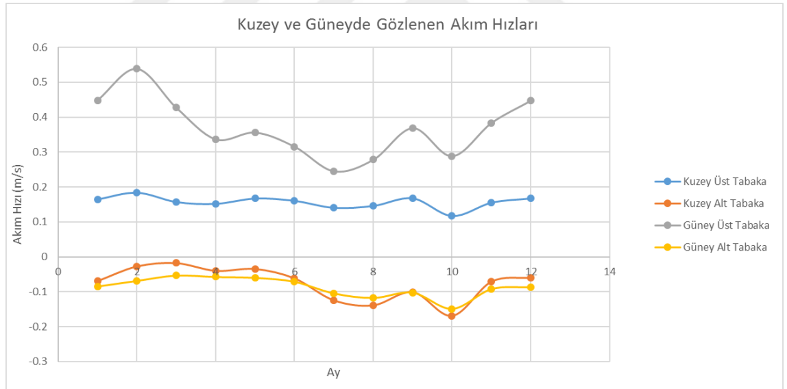
Şekil 5.36 : İstanbul Boğazı'nda gözlenen aylık ortalama akım hızları.
