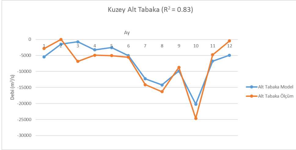
Şekil 5.41 : İstanbul Boğazı'nın kuzeyinde ölçüm ve modelin alt tabaka debileri.
