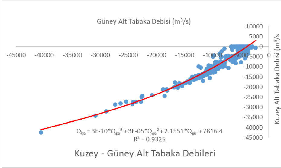
Şekil 5.48 : Kuzey ile güney alt tabaka debileri arasındaki regresyon eğrisi.
