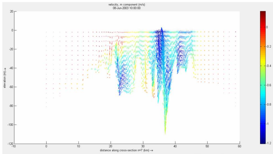
Şekil 5.8 : Marmara'nın baskın olması halinde 08.06.2003 tarihinde İstanbul Boğazı boykesiti hız vektörleri.
