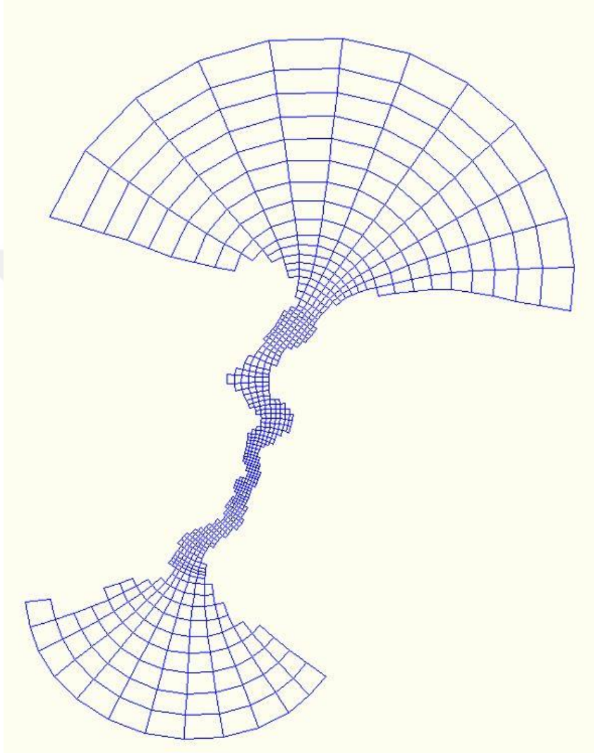
Şekil 4.2 : İstanbul Boğazı'nın yatay hesap ağı.
