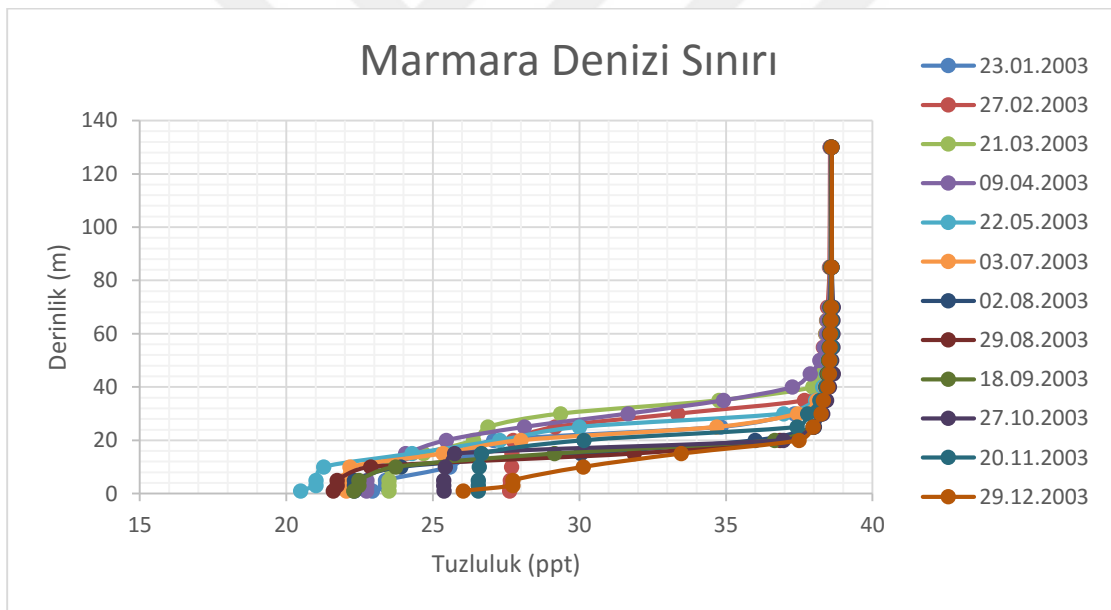
Şekil 3.4 : İstanbul Boğazı'nın Marmara Denizi sınırı için tuzluluk ölçüm tablosu.
