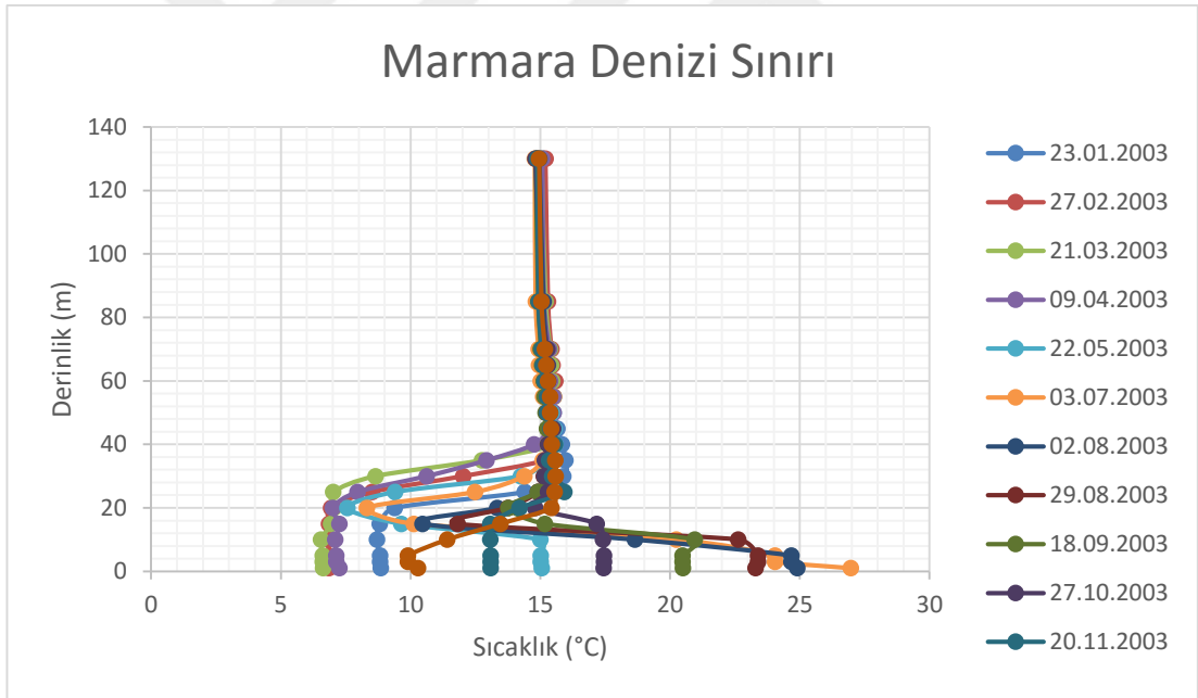
Şekil 3.6 : İstanbul Boğazı'nın Marmara Denizi sınırı için sıcaklık ölçüm tablosu.
