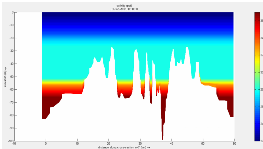
Şekil 4.7 : İstanbul Boğazı'nın başlangıç tuzluluk değerlerini gösteren boykesit.
