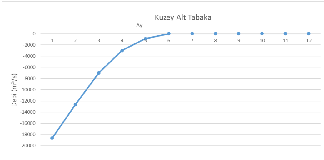
Şekil 5.2 : Karadeniz’in baskın olduğu duruma ait Boğaz’ın kuzey kesimindeki alt tabaka debi-zaman grafiği.
