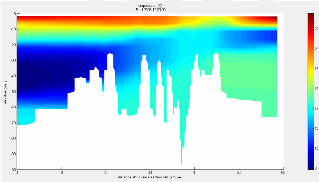
Şekil 5.13 : 15 Temmuz 2003 tarihine ait İstanbul Boğazı boykesiti sıcaklık profili.
