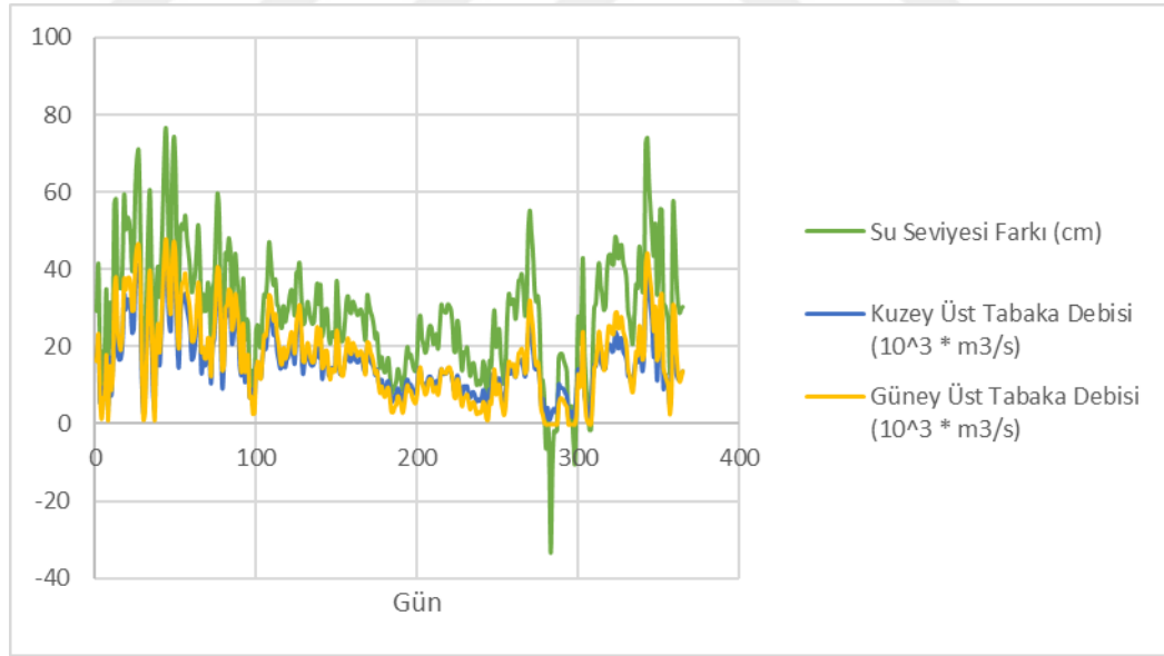
Şekil 5.44 : Günlük su seviyesi farkı ve kuzey ve güneydeki üst tabaka akımı debisi.
