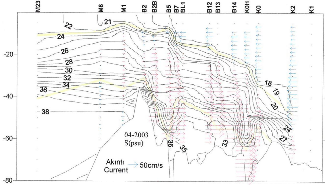
Şekil 5.21 : İstanbul Boğazı'nda Nisan ayına ait boykesit tuzluluk değerleri (İSKİ, 2004).
