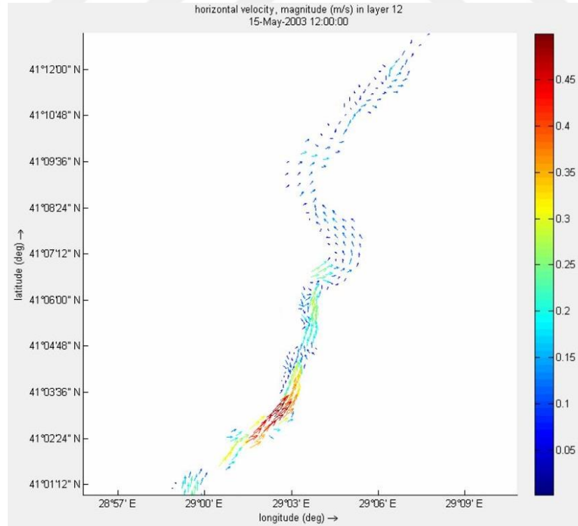
Şekil 5.33 : 15 Mayıs 2003 tarihinde İstanbul Boğazı'nda 45 m derinlikte hız vektörleri.
