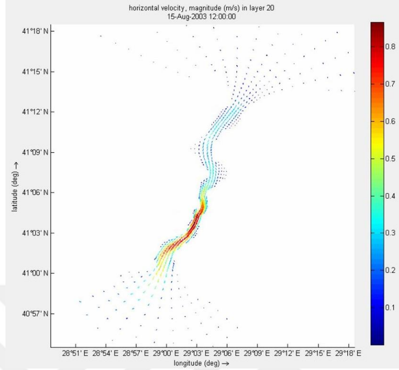
Şekil 5.30 : 15 Ağustos 2003 tarihinde İstanbul Boğazı'nda 5 m derinlikte hız vektörleri.
