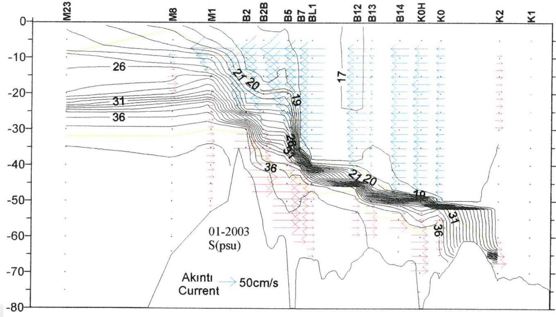
Şekil 5.20 : İstanbul Boğazı'nda Ocak ayına ait boykesit tuzluluk değerleri (İSKİ, 2004).
