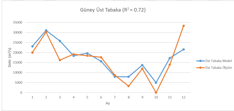
Şekil 5.42 : İstanbul Boğazı'nın güneyinde ölçüm ve modelin üst tabaka debileri.
