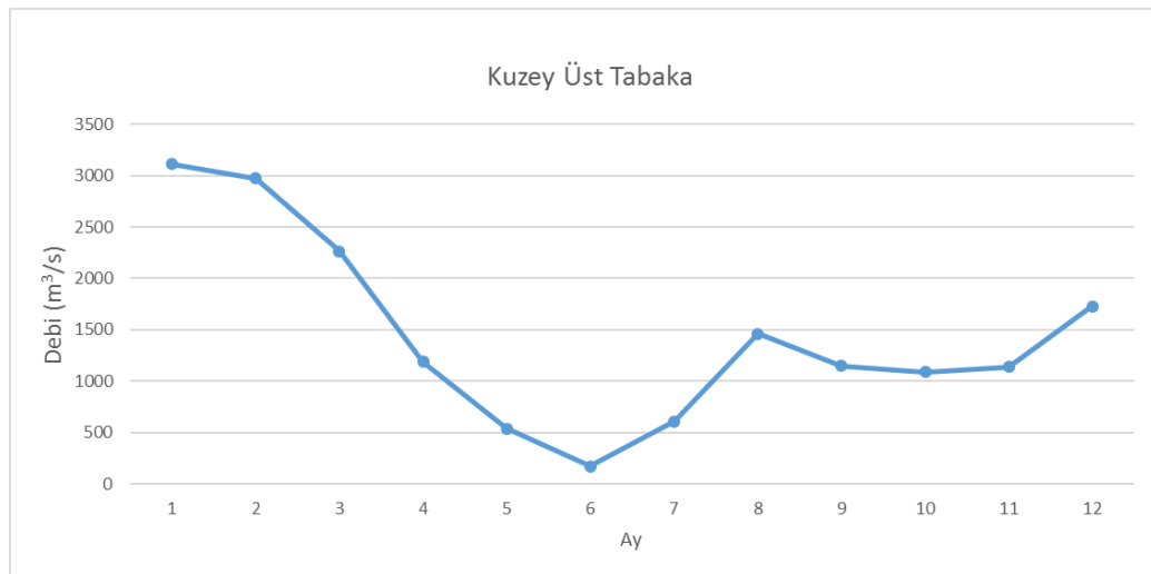
Şekil 5.6 : Marmara'nın baskın olduğu duruma ait Boğaz'ın kuzey kesimindeki üst tabaka debi-zaman grafiği.
