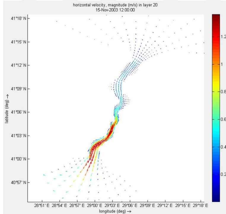
Şekil 5.31 : 15 Kasım 2003 tarihinde İstanbul Boğazı'nda 5 m derinlikte hız vektörleri.
