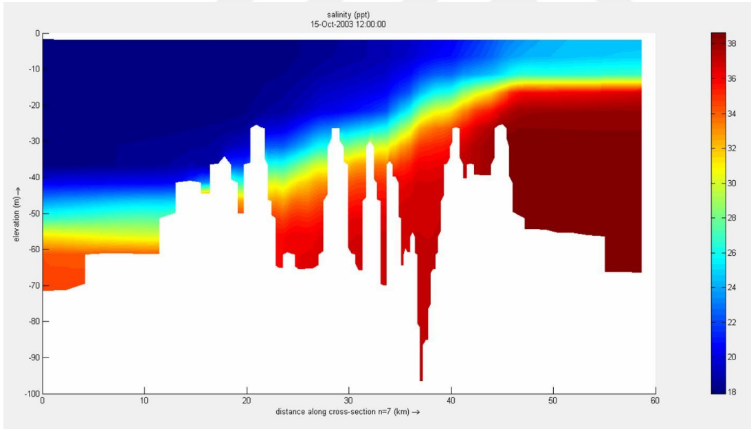
Şekil 5.19 : 15 Ekim 2003 tarihine ait İstanbul Boğazı boykesiti tuzluluk profili.
