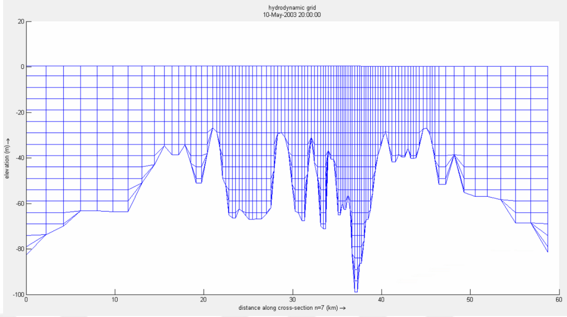
Şekil 4.3 : İstanbul Boğazı'nın boykesiti ve dikey hesap ağı.
