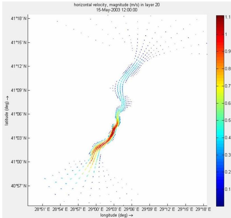
Şekil 5.29 : 15 Mayıs 2003 tarihinde İstanbul Boğazı'nda 5 m derinlikte hız vektörleri.
