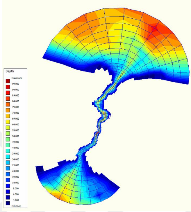
řekil 4.4 : İstanbul Bođazı'nın Delft3D ile hesap yapımı i in hazırlanmıř batimetrisi.
