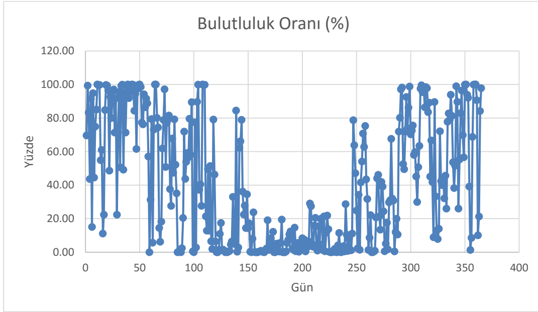
Şekil 3.11 : 2003 yılına ait İstanbul’daki bulutluluk oranı tahmin değerleri.
