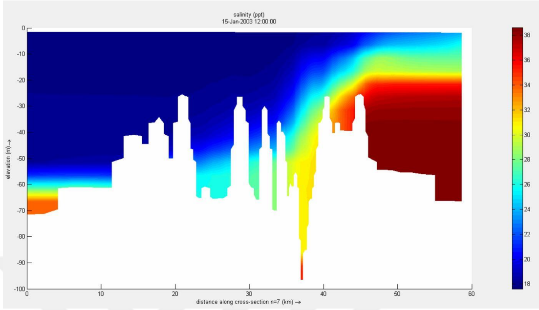
Şekil 5.16 : 15 Ocak 2003 tarihine ait İstanbul Boğazı boykesiti tuzluluk profili.
