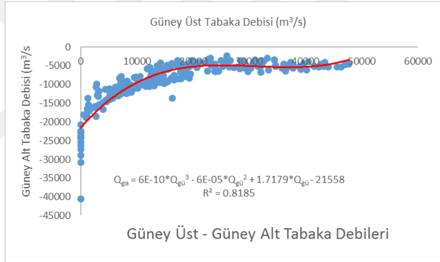
Şekil 5.50 : Güney üst ile alt tabaka debileri arasındaki regresyon eğrisi.
