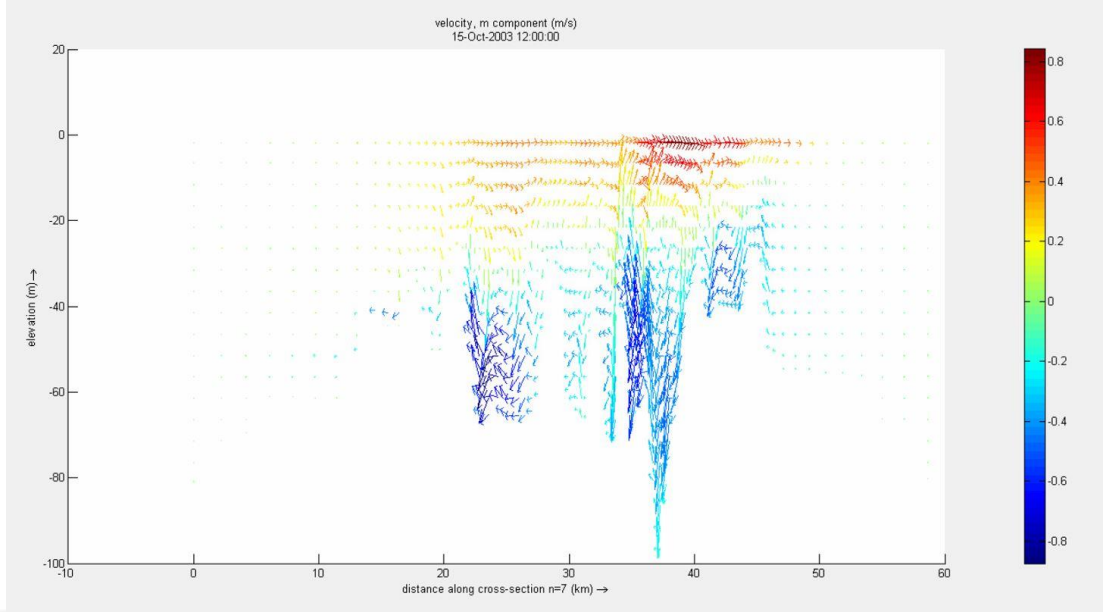
Şekil 5.27 : 15 Ekim 2003 tarihine ait İstanbul Boğazı boykesiti hız profili.
