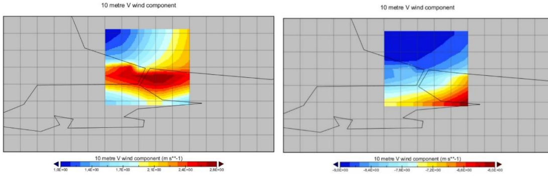
Şekil 3.14 : İstanbul’da 15.01.2003 ve 15.04.2003 tarihlerinde V yönündeki rüzgar hızı dağılımı.
