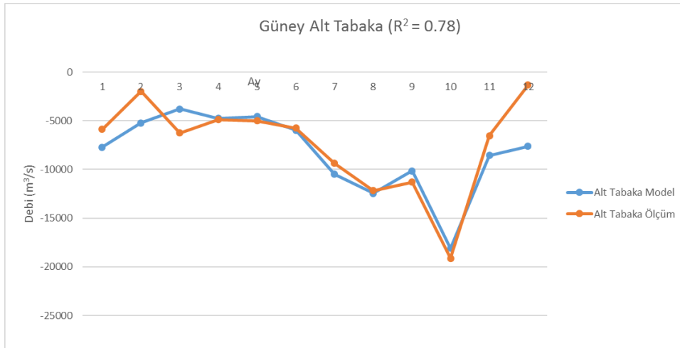
Şekil 5.43 : İstanbul Boğazı'nın güneyinde ölçüm ve modelin alt tabaka debileri.
