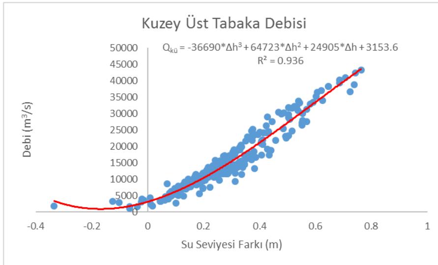
Şekil 5.45 : Kuzey üst tabaka debisi ile su seviyesi arasındaki regresyon eğrisi.
