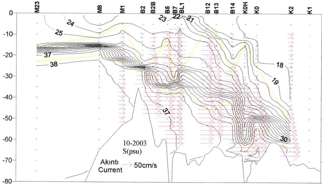
Şekil 5.23 : İstanbul Boğazı'nda Ekim ayına ait boykesit tuzluluk değerleri (İSKİ, 2004).
