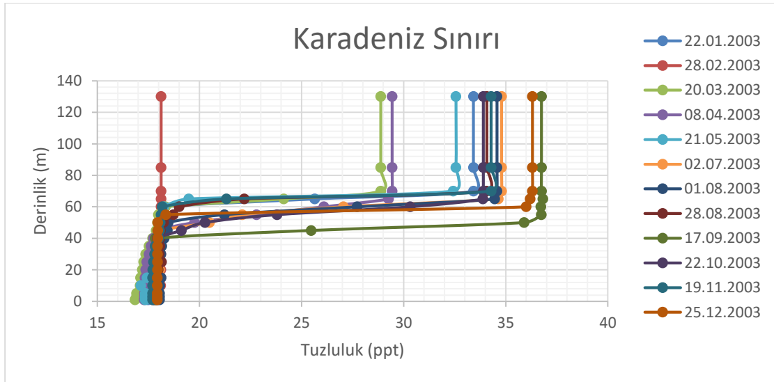
Şekil 3.3 : İstanbul Boğazı'nın Karadeniz sınırı için tuzluluk ölçüm tablosu.
