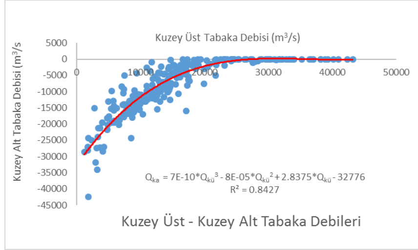
Şekil 5.49 : Kuzey üst ile alt tabaka debileri arasındaki regresyon eğrisi.
