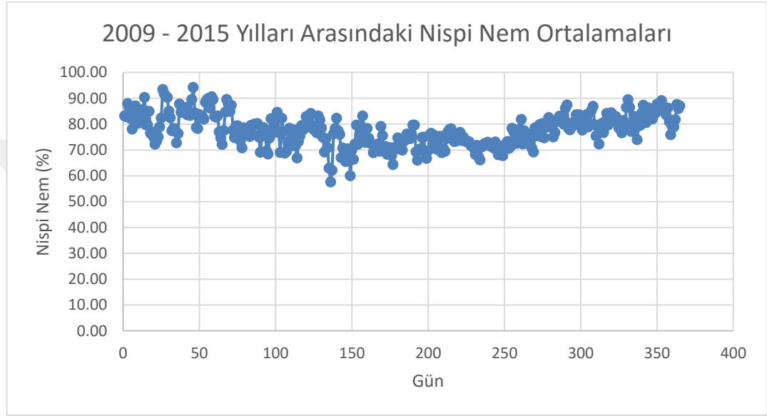
Şekil 3.10 : AKOM tarafından 2009-2015 yılları arasında yapılan nispi nem ölçümlerinin günlük bazda ortalamaları.
