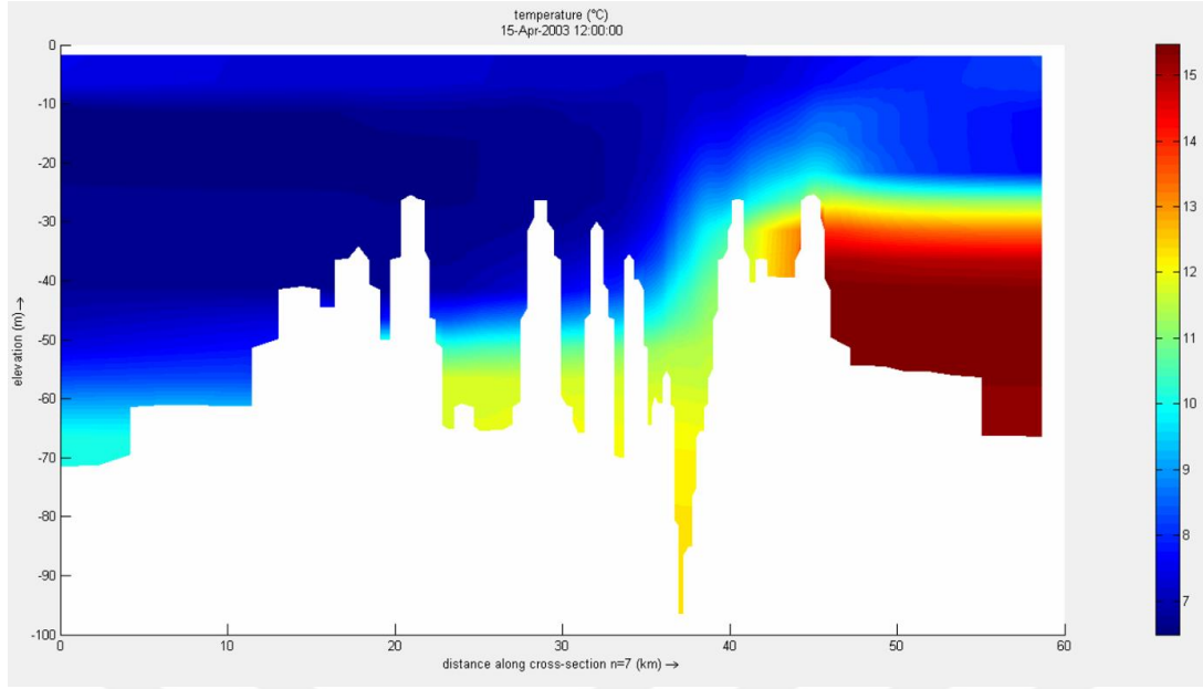
Şekil 5.12 : 15 Nisan 2003 tarihine ait İstanbul Boğazı boykesiti sıcaklık profili.
