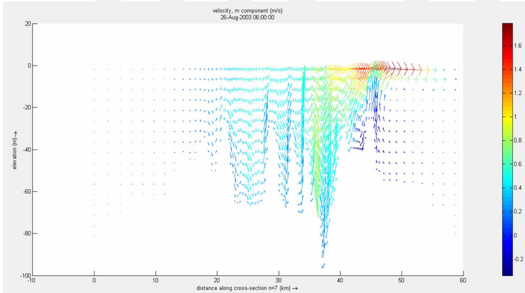
Şekil 5.5 : Karadeniz'in baskın olması halinde 26.08.2003 tarihinde İstanbul Boğazı boykesiti hız vektörleri.
