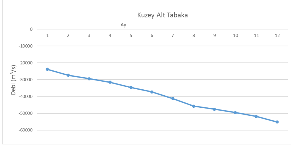
Şekil 5.7 : Marmara'nın baskın olduğu duruma ait Boğaz'ın kuzey kesimindeki alt tabaka debi-zaman grafiği.
