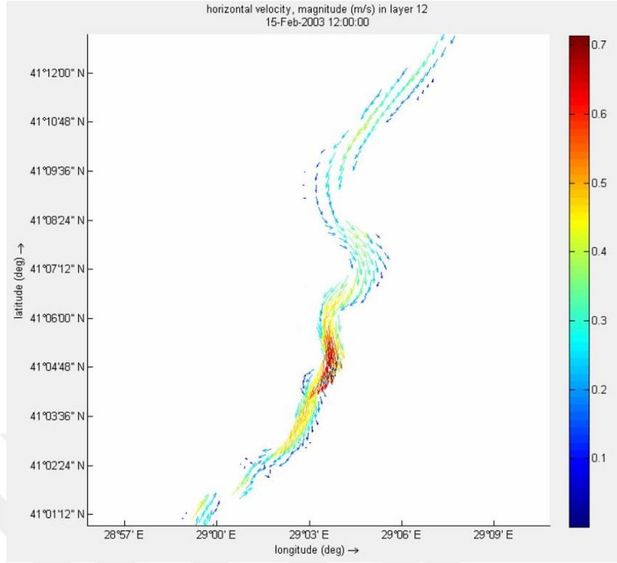
Şekil 5.32 : 15 Şubat 2003 tarihinde İstanbul Boğazı'nda 45 m derinlikte hız vektörleri.
