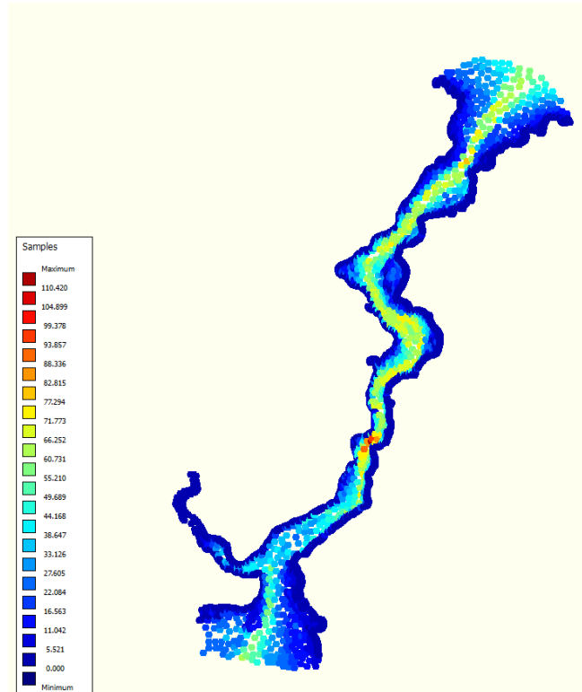
Şekil 3.1 : İstanbul Boğazı'na ait batimetri haritası.
