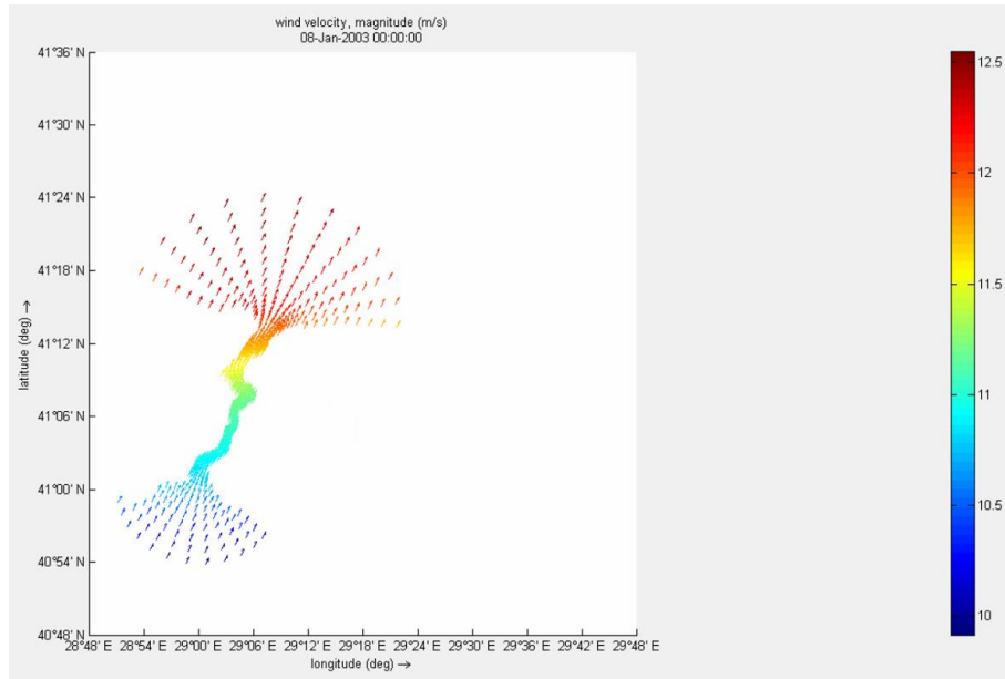
Şekil 4.6 : Lodos’un hakim olduğu bir zaman dilimine ait rüzgar hız vektörleri.
