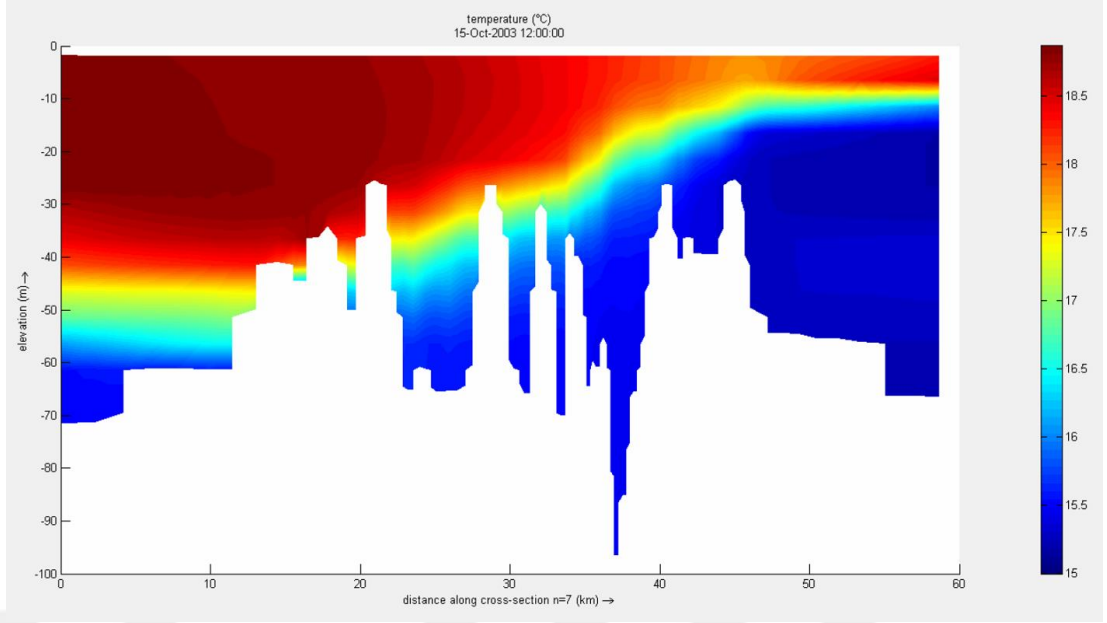
Şekil 5.14 : 15 Ekim 2003 tarihine ait İstanbul Boğazı boykesiti sıcaklık profili.
