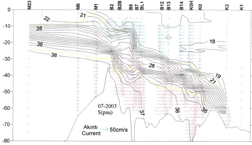
Şekil 5.22 : İstanbul Boğazı'nda Temmuz ayına ait boykesit tuzluluk değerleri (İSKİ, 2004).
