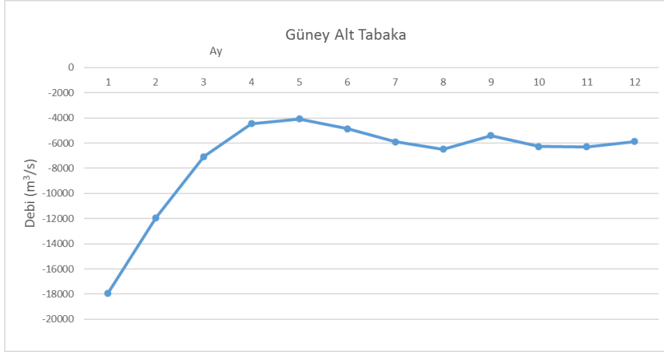
Şekil 5.4 : Karadeniz'in baskın olduğu duruma ait Boğaz'ın güney kesimindeki alt tabaka debi-zaman grafiği.
