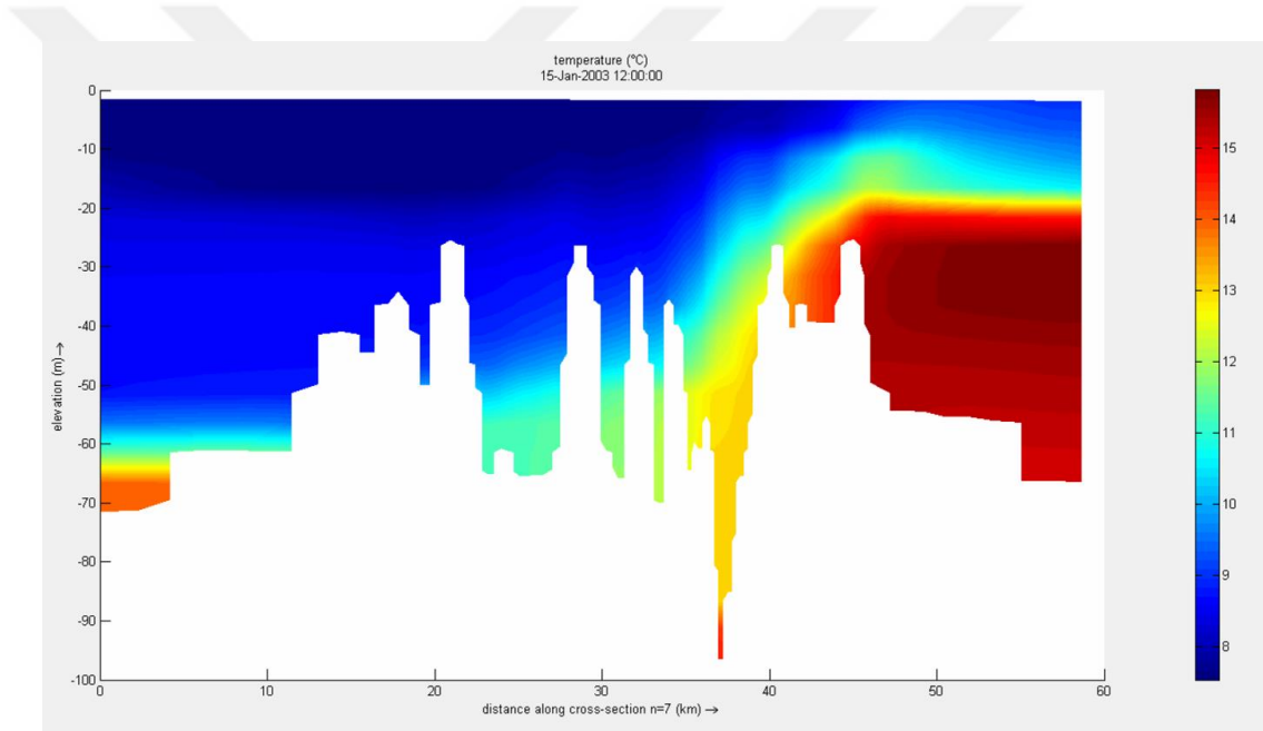
Şekil 5.11 : 15 Ocak 2003 tarihine ait İstanbul Boğazı boykesiti sıcaklık profili.
