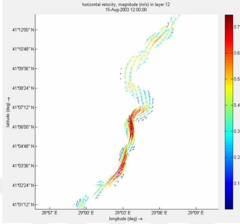
Şekil 5.34 : 15 Ağustos 2003 tarihinde İstanbul Boğazı'nda 45 m derinlikte hız vektörleri.
