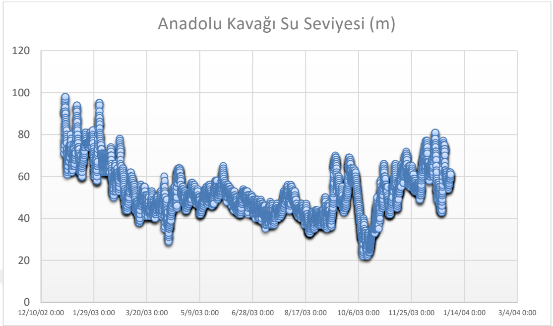
Şekil 3.8 : 2003 yılına ait Anadolu Kavağı'ndaki su seviyesi değerleri.
