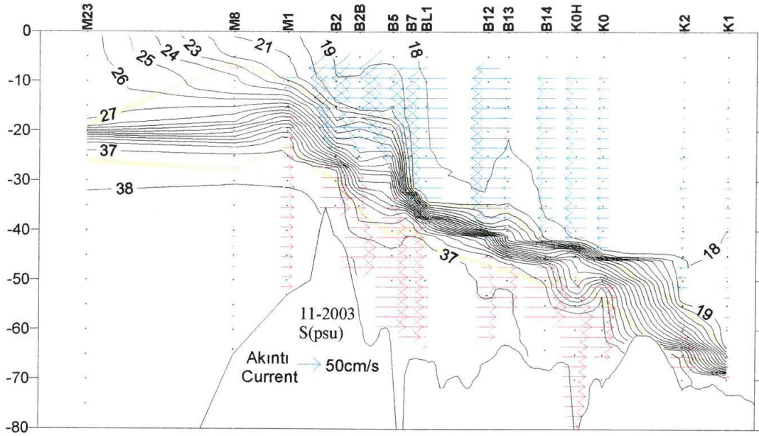
Şekil 2.6 : İstanbul Boğazı'nın 2003 Kasım ayına ait boykesit profili (İSKİ, 2004).
