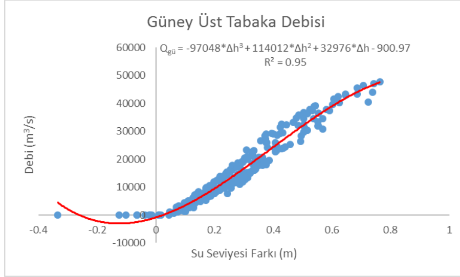
Şekil 5.46 : Güney üst tabaka debisi ile su seviyesi arasındaki regresyon eğrisi.
