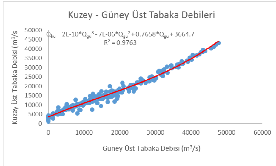
Şekil 5.47 : Kuzey ile güney üst tabaka debileri arasındaki regresyon eğrisi.
