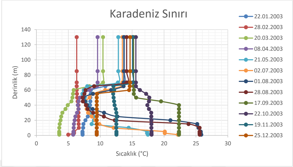
Şekil 3.5 : İstanbul Boğazı'nın Karadeniz sınırı için sıcaklık ölçüm tablosu.
