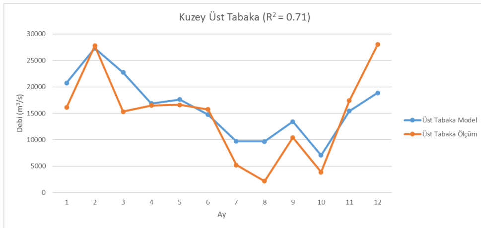
Şekil 5.40 : İstanbul Boğazı'nın kuzeyinde ölçüm ve modelin üst tabaka debileri.
