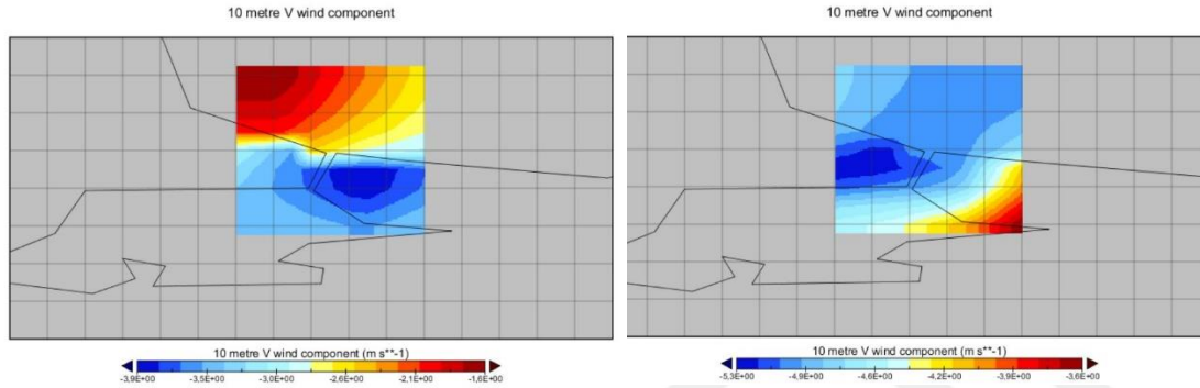
Şekil 3.15 : İstanbul’da 15.07.2003 ve 15.10.2003 tarihlerinde V yönündeki rüzgar hızı dağılımı.
