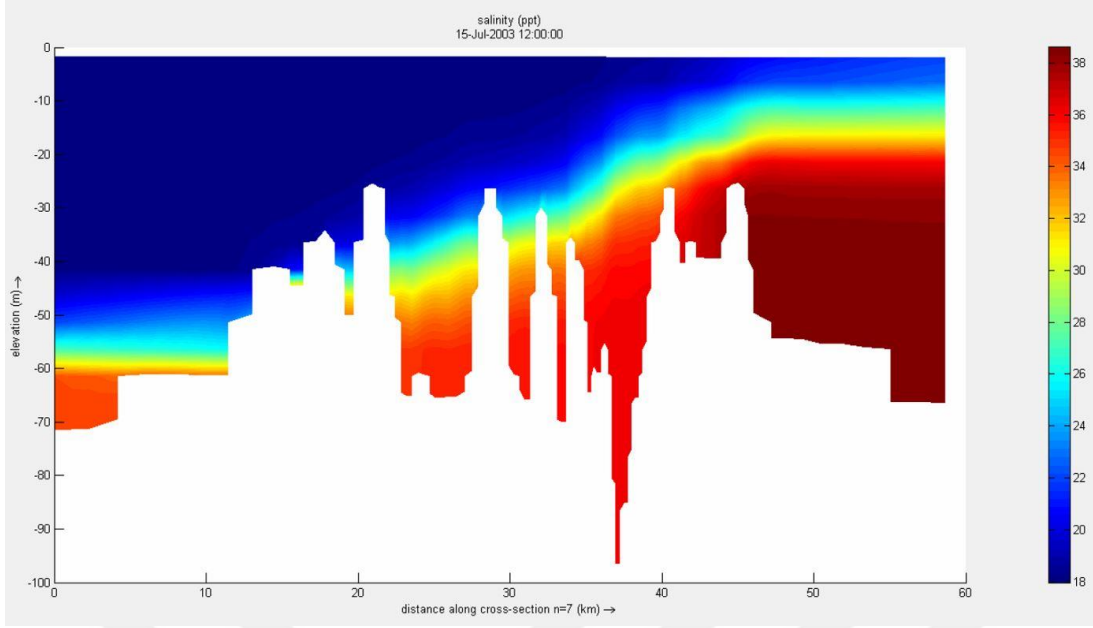
Şekil 5.18 : 15 Temmuz 2003 tarihine ait İstanbul Boğazı boykesiti tuzluluk profili.
