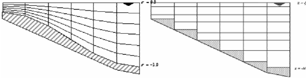
Şekil 4.1 : σ koordinat sistemi (solda) ve Z koordinat sistemi (sağda).
