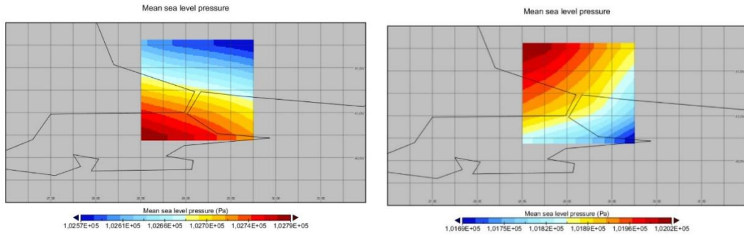
Şekil 3.16 : İstanbul'da 15.01.2003 ve 15.04.2003 tarihlerinde atmosfer basıncı dağılımı.
