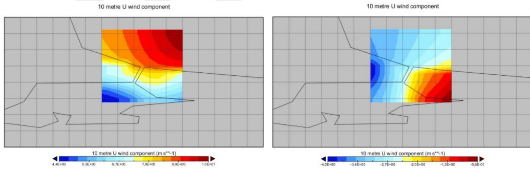
Şekil 3.12 : İstanbul'da 15.01.2003 ve 15.04.2003 tarihlerinde U yönündeki rüzgar hızı dağılımı.
