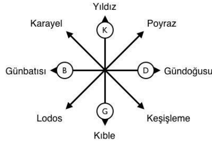
Şekil 2.3 : Yönlerine göre rüzgar isimleri.
