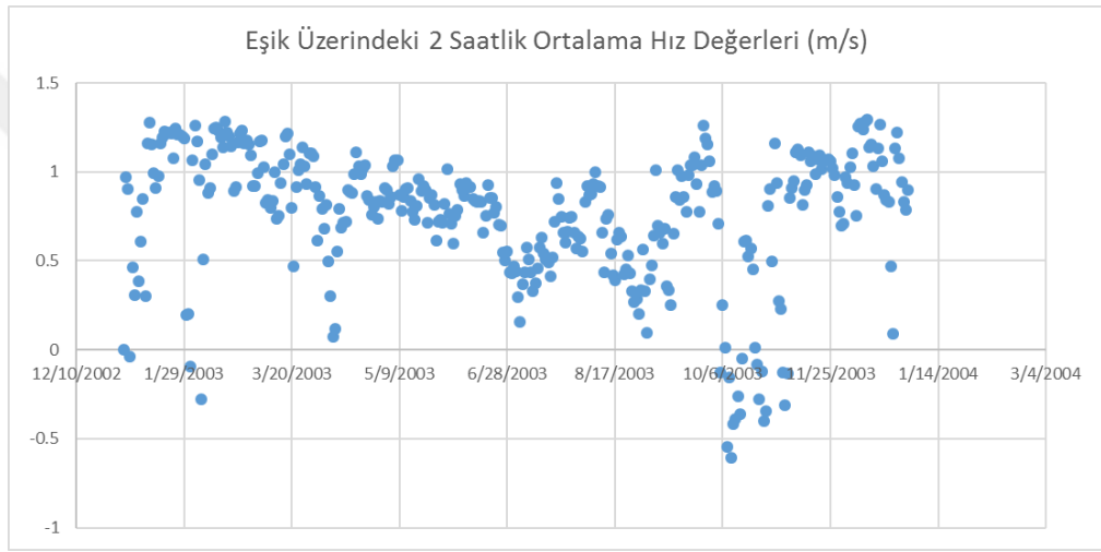
Şekil 5.38 : Güney eşiği üzerindeki 2 saatlik ortalama hız değerleri.
