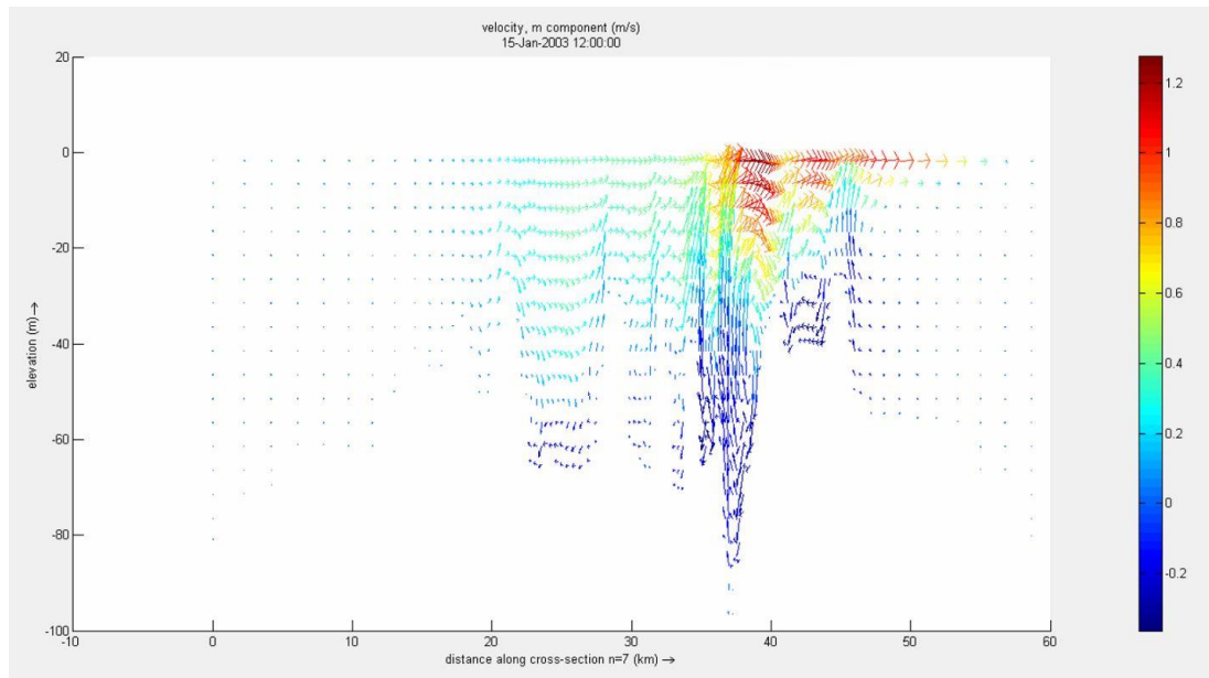
Şekil 5.24 : 15 Ocak 2003 tarihine ait İstanbul Boğazı boykesiti hız profili.
