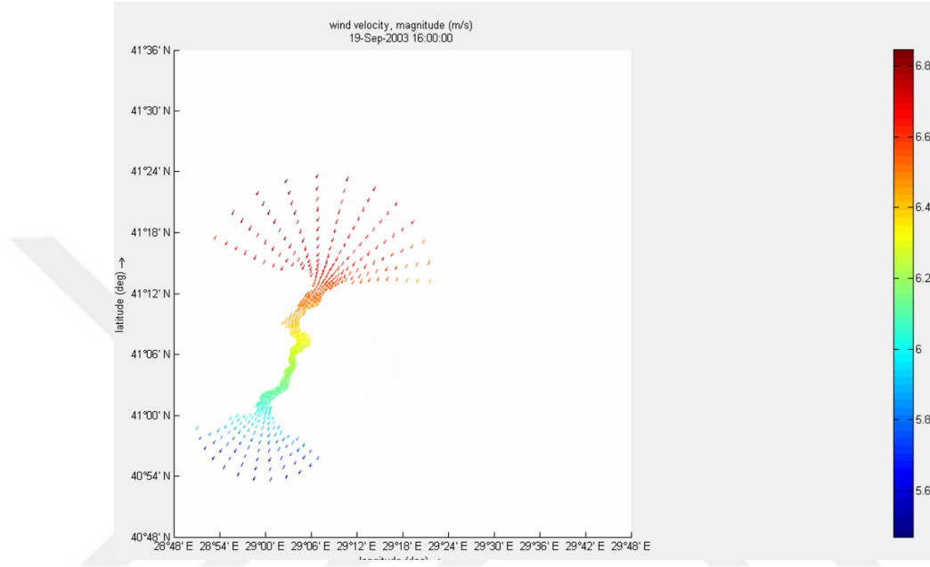
Şekil 4.5 : Poyraz’ın hakim olduğu bir zaman dilimine ait rüzgar hız vektörleri.
