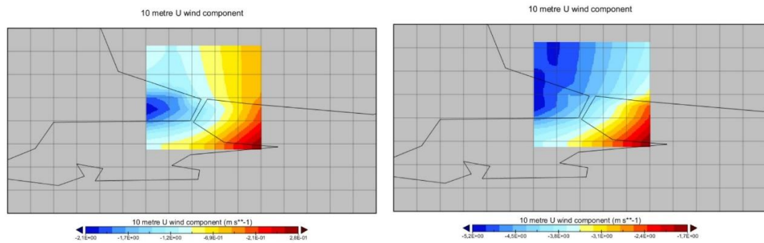
Şekil 3.13 : İstanbul'da 15.07.2003 ve 15.10.2003 tarihlerinde U yönündeki rüzgar hızı dağılımı.
