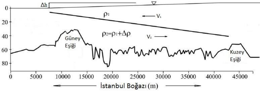
Şekil 1.2 : Tipik bir tabakalı akım yapısına sahip olan İstanbul Boğazı'nın boykesiti (Öztürk, 2010).
