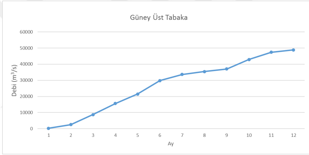
Şekil 5.3 : Karadeniz'in baskın olduğu duruma ait Boğaz'ın güney kesimindeki üst tabaka debi-zaman grafiği.
