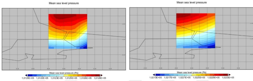
Şekil 3.17 : İstanbul'da 15.07.2003 ve 15.10.2003 tarihlerinde atmosfer basıncı dağılımı.
