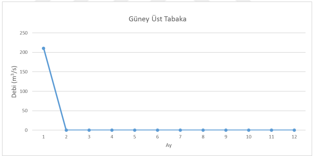
Şekil 5.9 : Marmara’nın baskın olduğu duruma ait Boğaz’ın güney kesimindeki üst tabaka debi-zaman grafiği.
