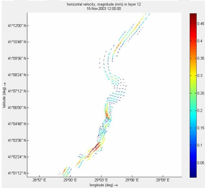
Şekil 5.35 : 15 Kasım 2003 tarihinde İstanbul Boğazı'nda 45 m derinlikte hız vektörleri.
