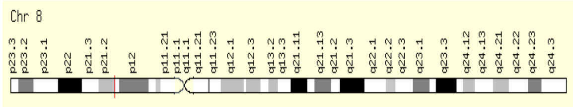
Şekil 7: Kromozom 8 ve CLU geninin lokasyonu
