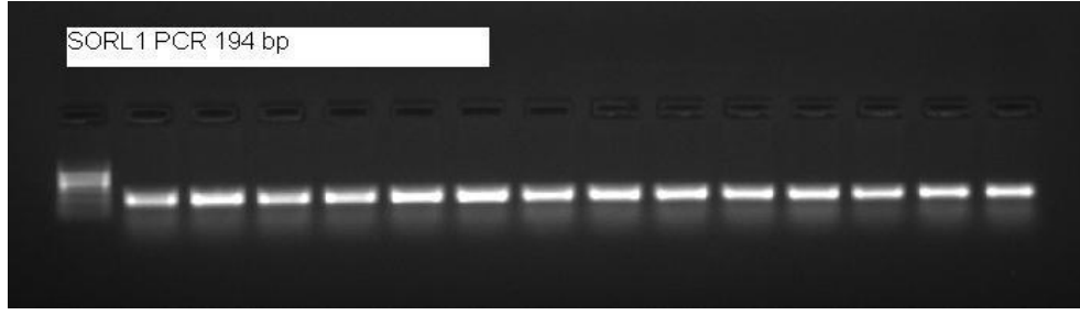
Şekil 11 : Uygun primerlerle çoğaltılan 194bp'lik (SORL1) PZR ürünlerinin %3'lük agaroz jeldeki görüntüsü. (Marker: 50 bp DNA marker)
