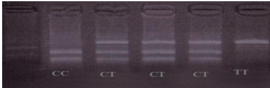
Şekil 14: SORL1 geni MsII enzimi kesimi sonucu ürünlerin%3'lük agaroz jeldeki bant görüntüsü
