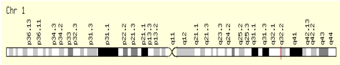
Şekil 9 : Kromozom 1 ve CR1 geninin lokasyonu
