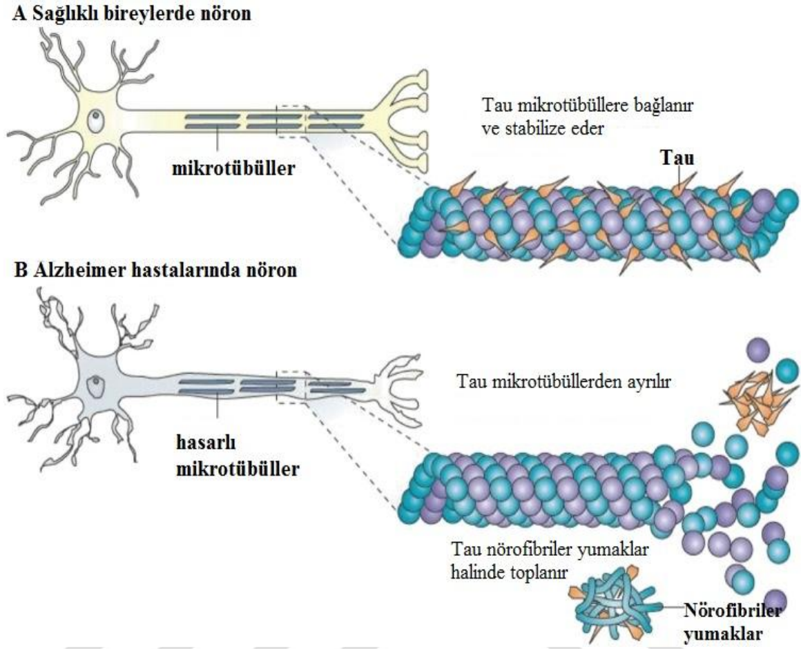
Şekil 3 : Alzheimer hastalarında görülen mikrotübül yapısı (42).
