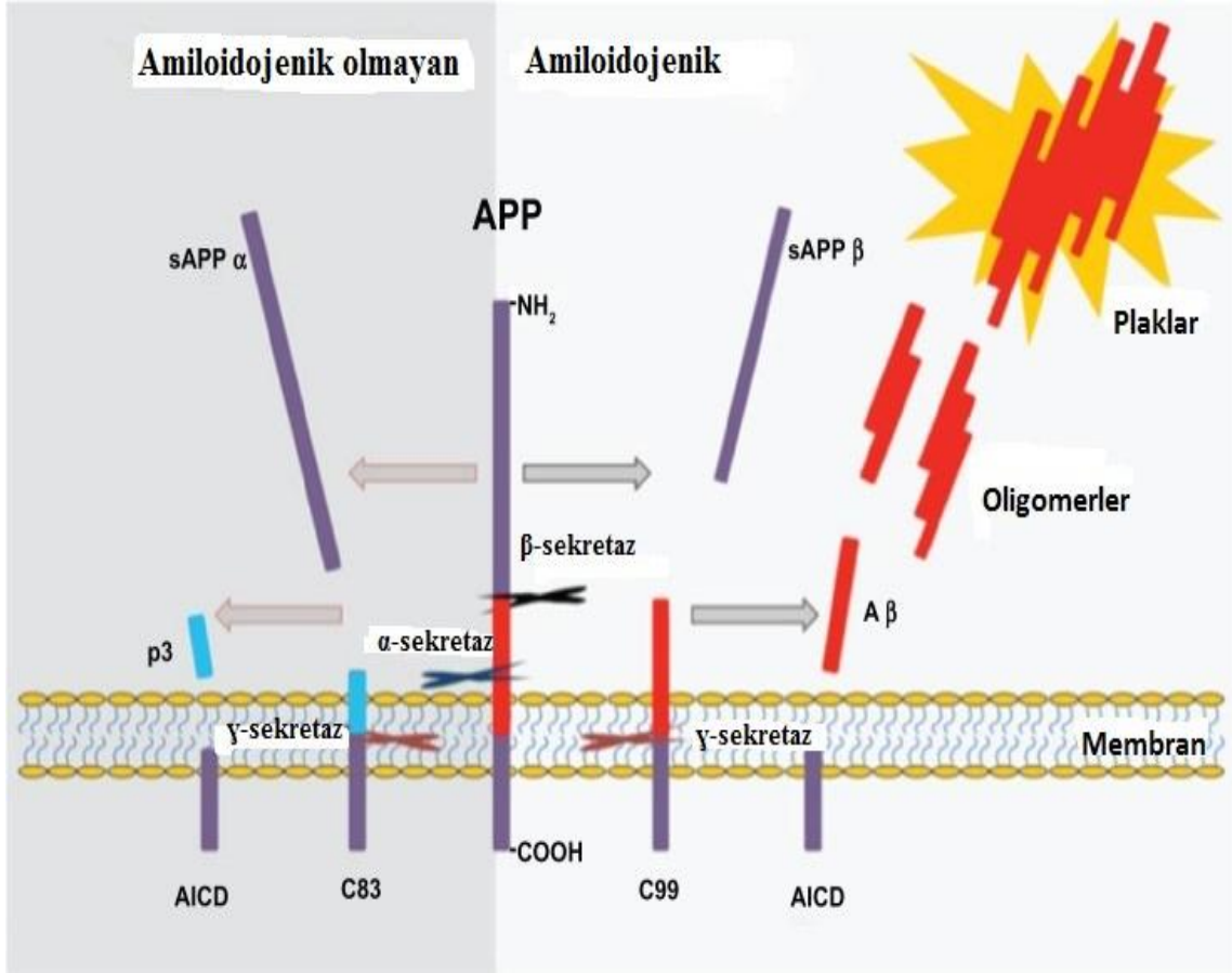
Şekil 4 : Amiloid Prekürsör protein (APP)'nin proteolitik kesimi (58).
