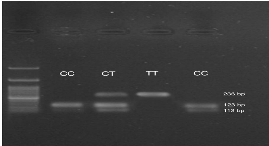
Şekil 12: CLU geni Hyp99i enzim kesimi sonucunda ürünlerin %3'lük agaroz jeldeki bant görüntüsü.
