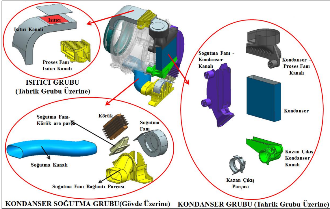
Şekil 4. 41 Kurutma sistemi parçaları
