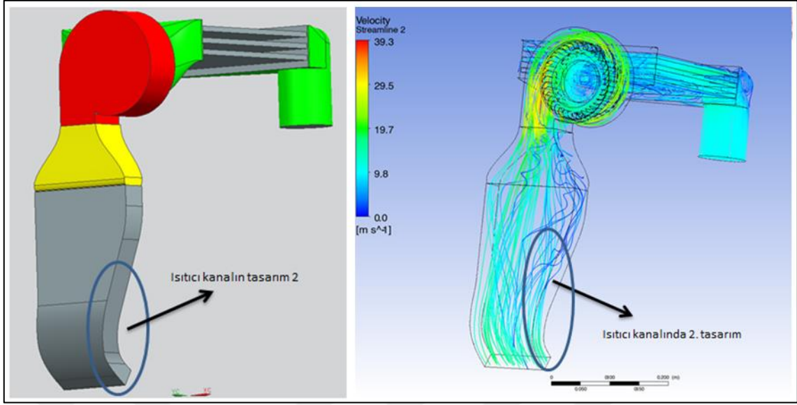
Şekil 4. 76 Isıtıcı kanalı konsept 2 akış hacmi ve CFD analizi
