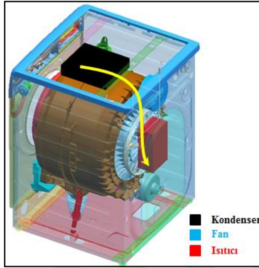
Şekil 3. 25 Yerleşim Konsepti 3
