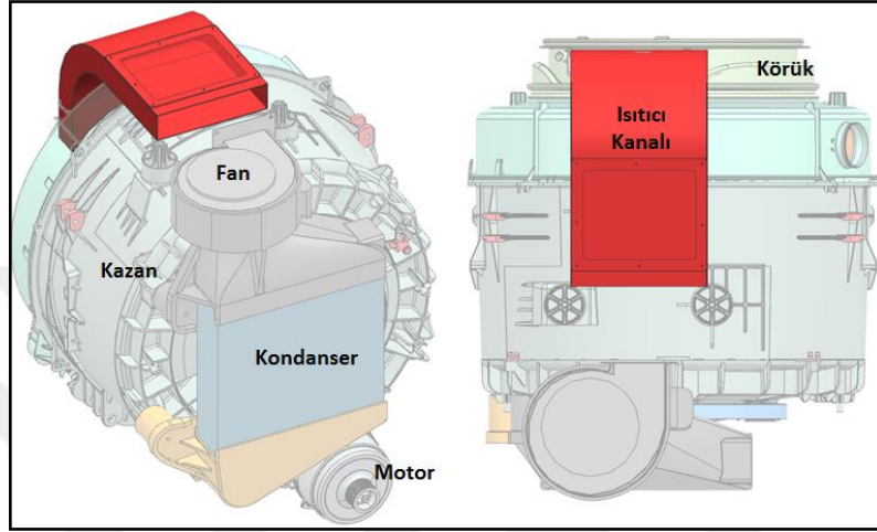
Şekil 4. 34 Isıtıcı kanalı
