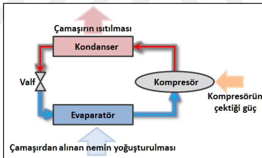
Isı pompası sistemi, ısının aktarılması prensibi ile çalışmaktadır. Elektrik enerjisi girişinden ve ortamdan çekilen ısı, ısı pompası sistemine girerek atılan ısıyı oluşturmaktadır. Kısaca proses havasından çekilen ısı ve elektrik enerjisi birleşerek bir ısı oluşturmaktadır. Bu ısı kondanser üzerinde proses havasının ısıtılmasında kullanılmaktadır. Isı pompası sistemi şekil 2.4' te gösterilmiştir.
