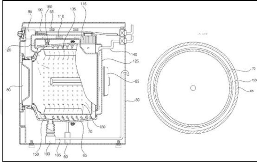
Şekil 1. 8 KR20070015294 (A) numaralı patente ait bir görünüş [5]
