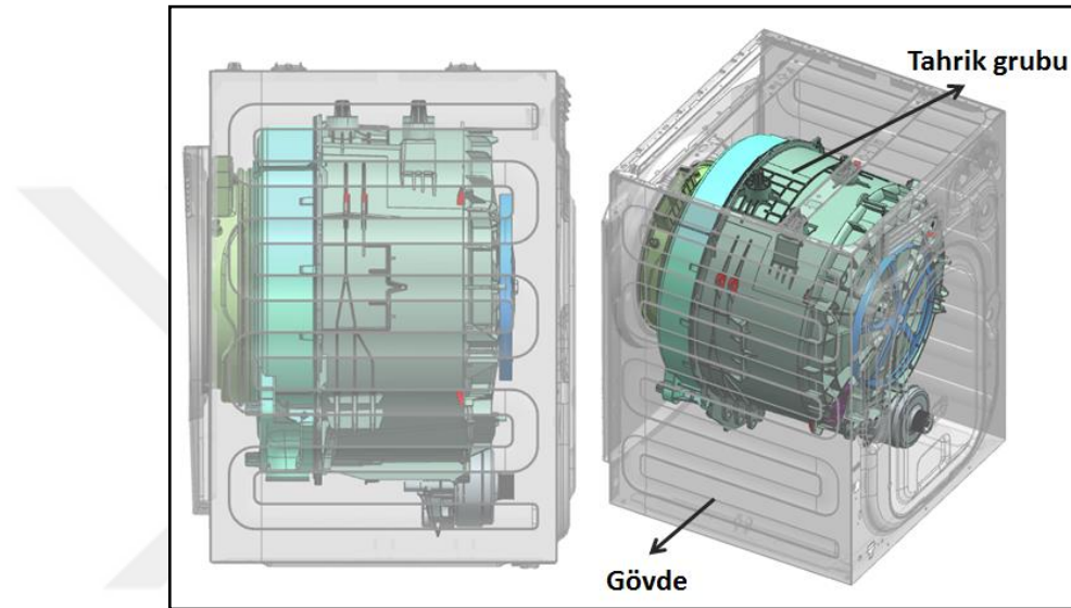
Şekil 4. 27 Tahrik grubunun gövde içerisine yerleşimi
