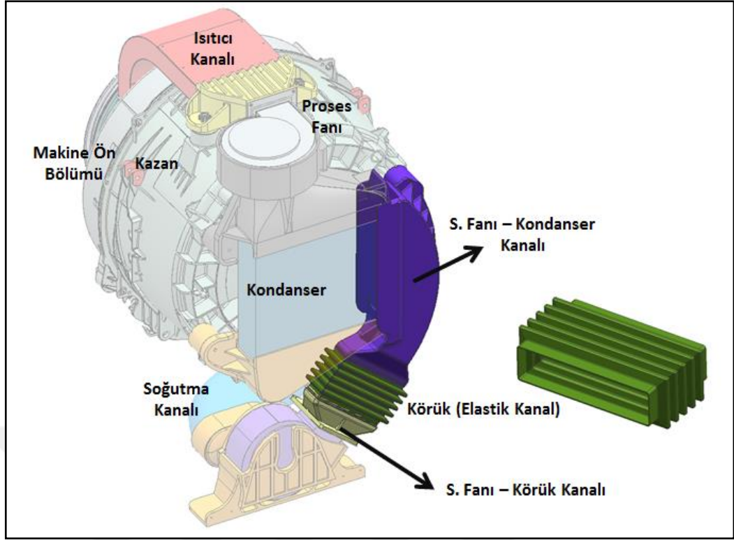
Şekil 4. 38 Soğutma fanı – kondanseri bağlantısı
