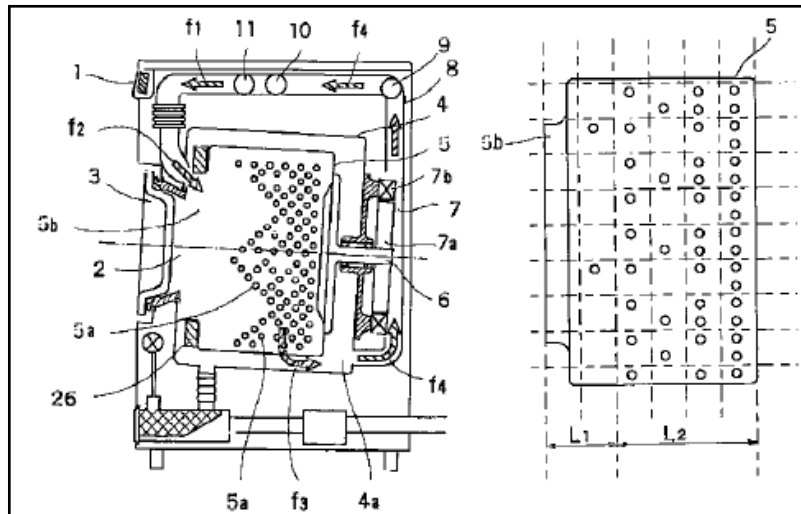
Şekil 1. 9 JP2000325688 (A) numaralı patente ait bir görünüş [6]
