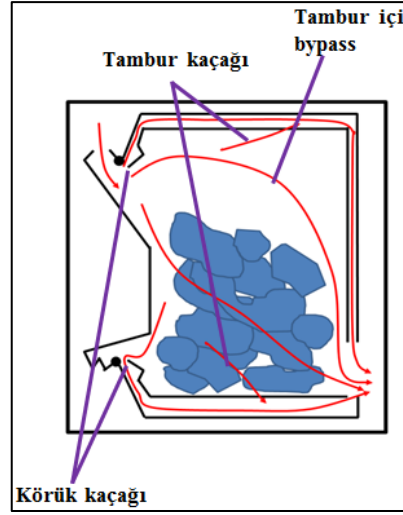
Şekil 4. 85 By-pass çeşitleri
