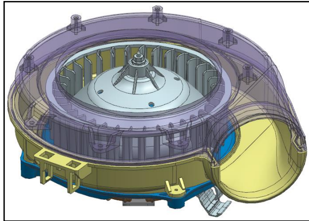
Şekil 2. 12 Fan
