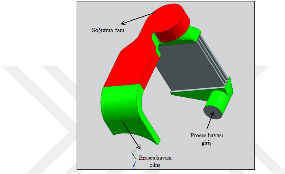
Şekil 4. 48 Proses kanalları akış hacmi
