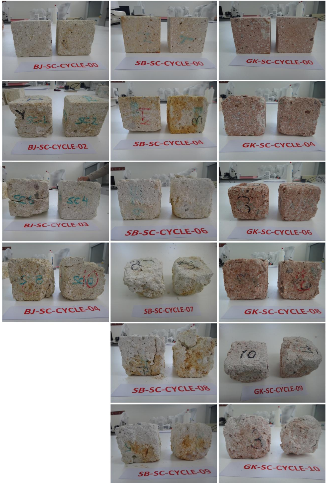
Resim 4.4. Tuz kristallenmesi deneyinde farklı çevrimler sonucundaki örneklerin genel görünümü
