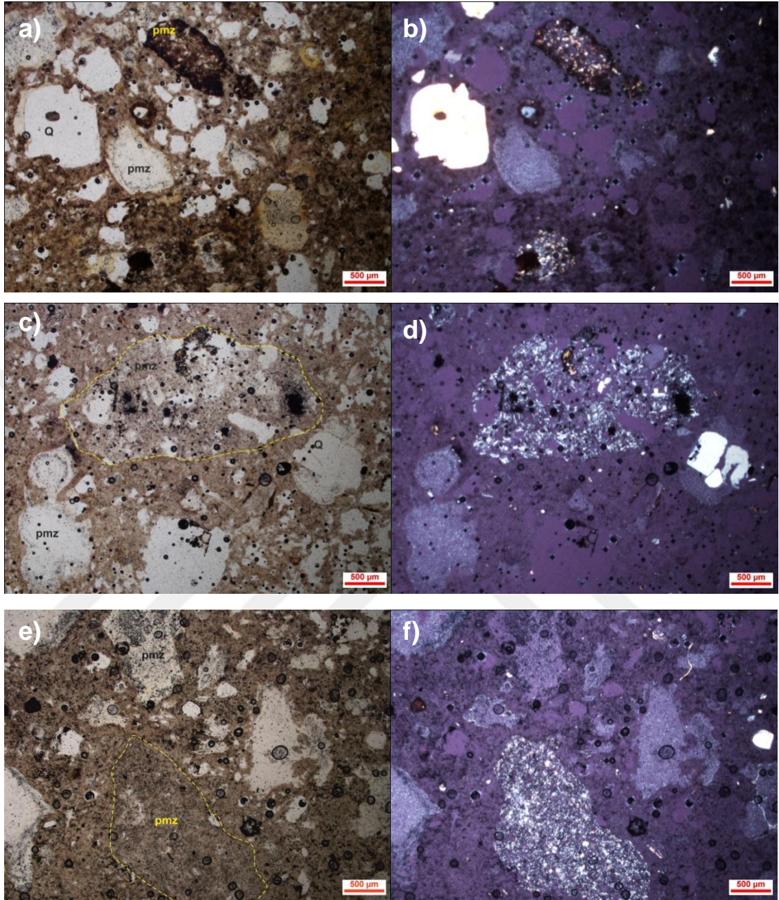
Resim 4.2. İğnimbiritlerin; alt seviyeye ait SB kodlu örneğin (a, b), orta seviyeye ait GK kodlu örneğin (c, d), üst seviyeye ait BJ kodlu örneğin (e, f) tek ve çift nikol mikroskop görüntüleri [42]
