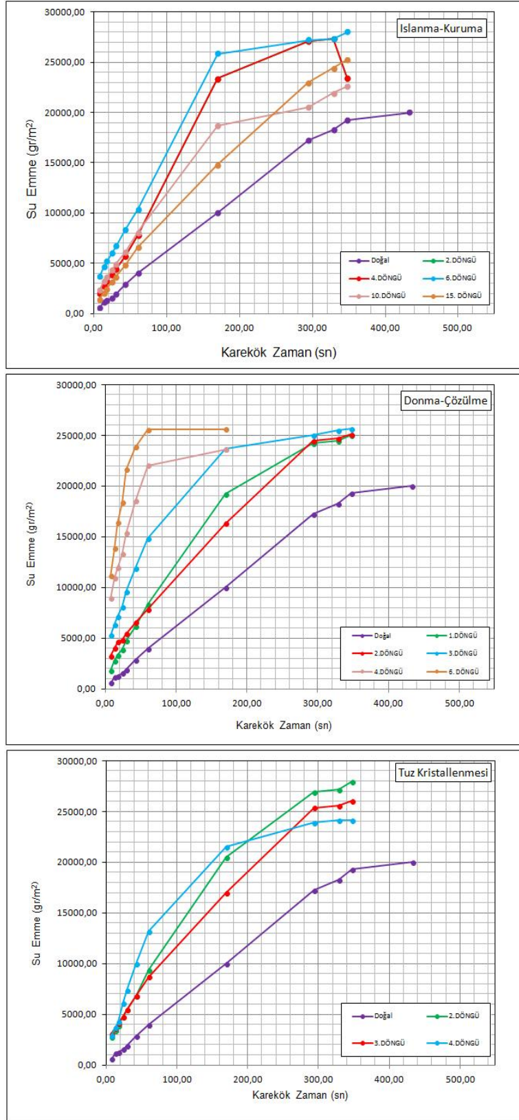
Şekil 4.13 Yapay bozunma deneyleri sonucunda ıgimbiritlerin (BJ) zamana göre kılcal su emme miktarı
