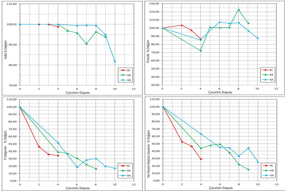
Şekil 4.12. Tuz kristallenmesi deneyi sonucunda ignimbiritlerin fiziksel ve mekanik özelliklerindeki değişim oranları
