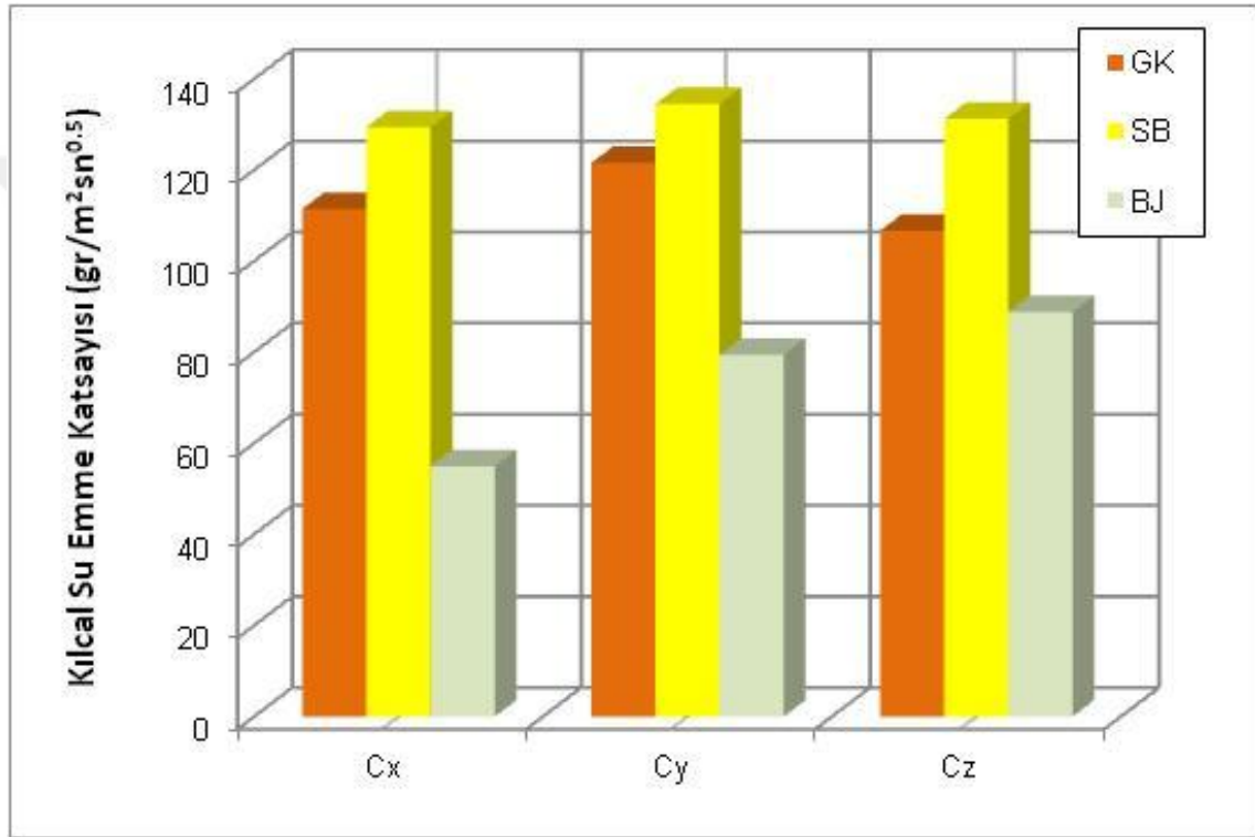
Şekil 4.7. Kılcal su emme katsayısının yönlere göre değişimi
