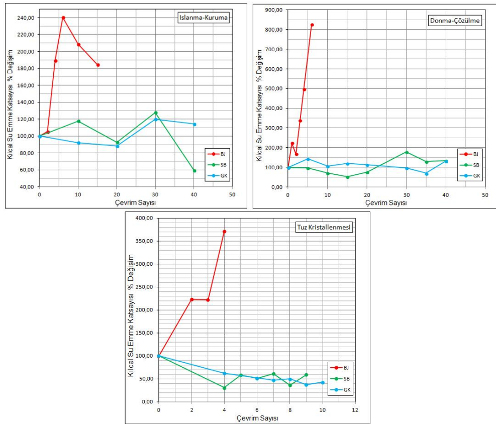
Şekil 4.16. Yapay bozunma deneyleri sonucunda ignimbritlerin kılcal su emme davranışlarında değişim grafikleri
