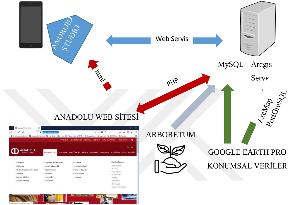
Şekil 3.1. Anadolu Mobil sistem mimarisi
