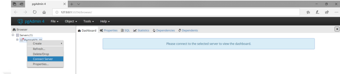
Şekil 2.16. PostgreSQL arayüzü
