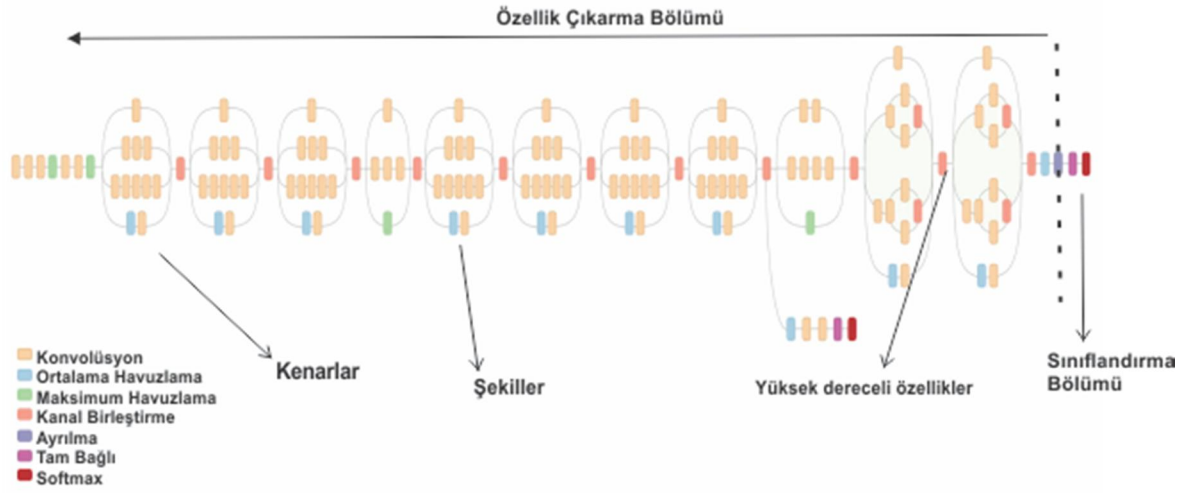
Şekil 4.4 Inception v3 modelinin özellik çıkarma ve sınıflandırma bölümleri [43]
