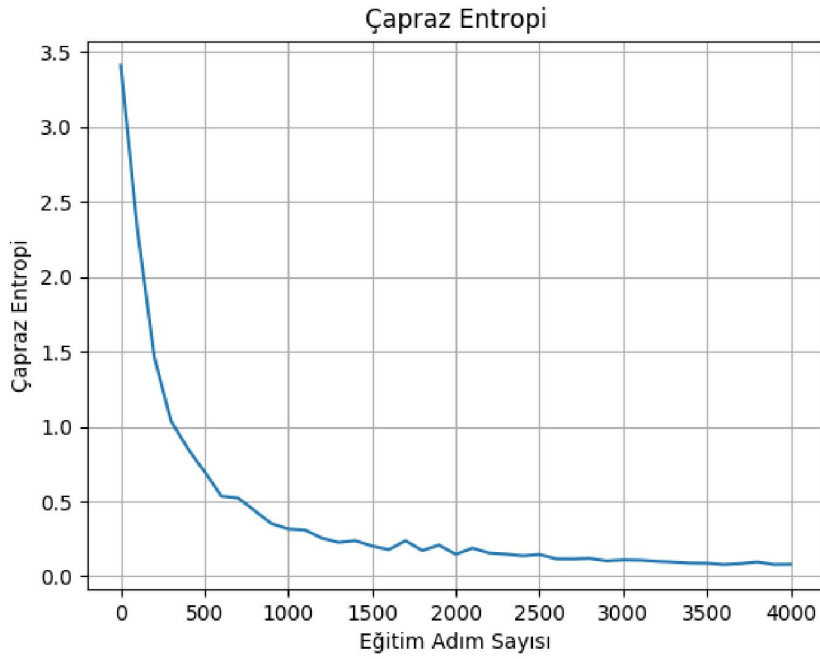
Şekil 5.2 İlk eğitimde çapraz entropi grafiği
