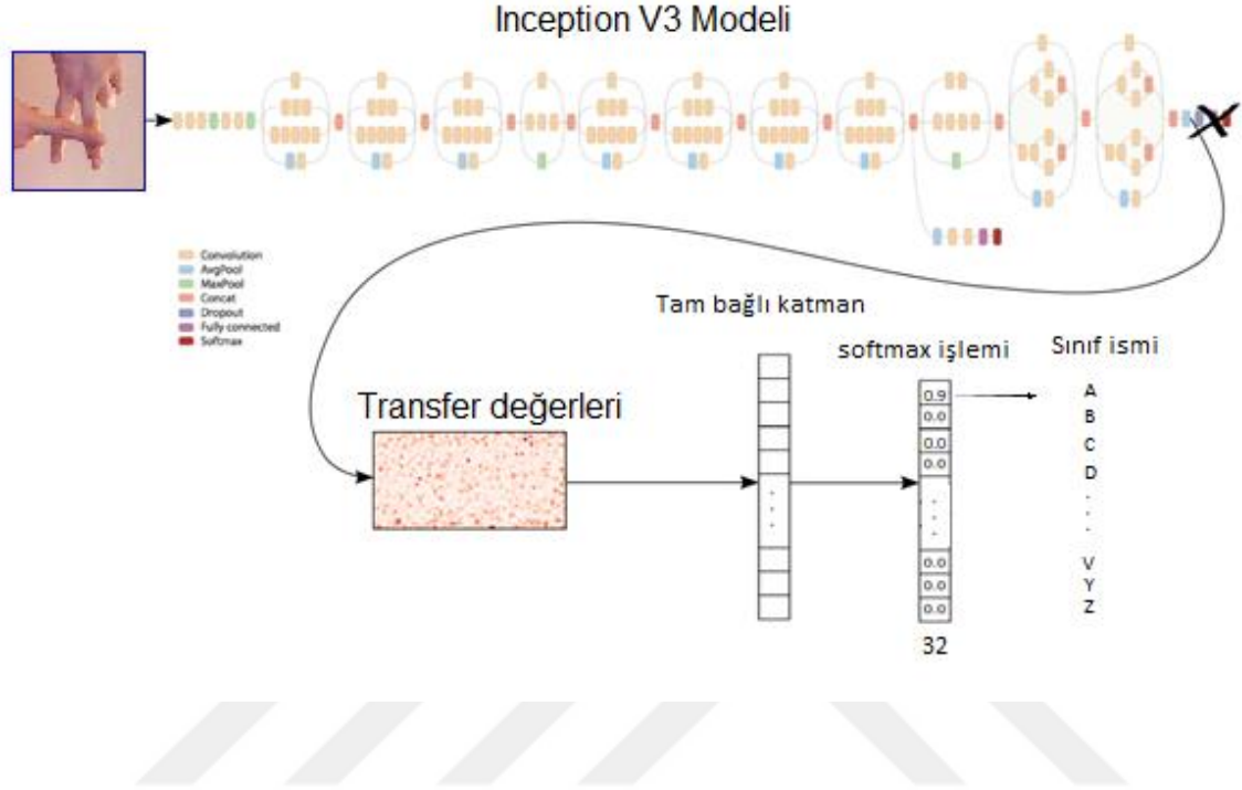
Şekil 4.20 Inception v3 ile öğrenmeyi transfer ederek sınıflandırma
