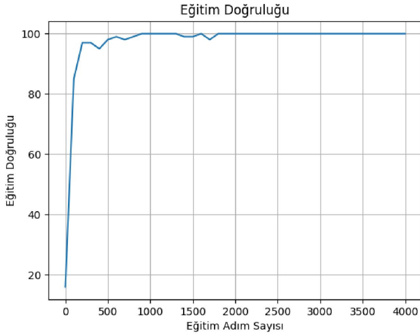
Şekil 5.1 İlk eğitimde eğitim doğruluğu grafiği (Veri setinin %80'lik kısmı)
