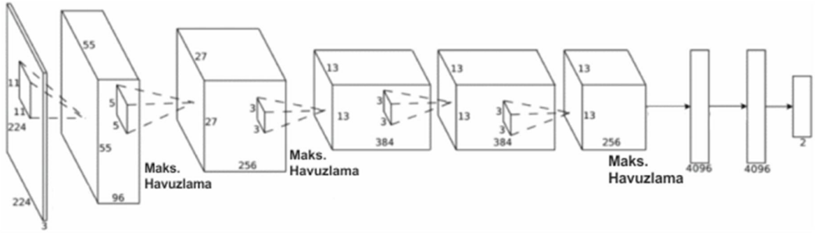
Şekil 3.20 AlexNet Yapısı [61]
