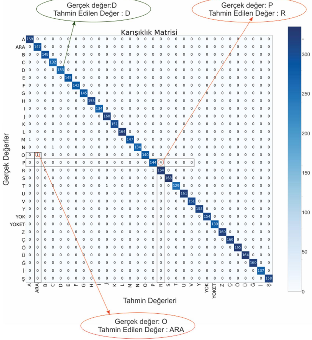
Şekil 5.4 Karışıklık matrisi
