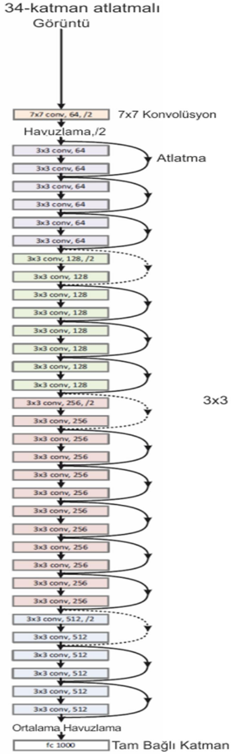
Şekil 3.24 ResNet Yapısı [65]
