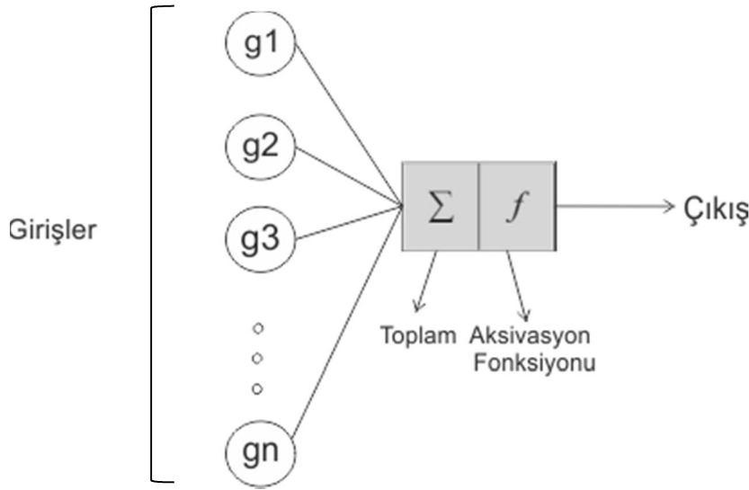
Şekil 3.3 Persepton yapısı
