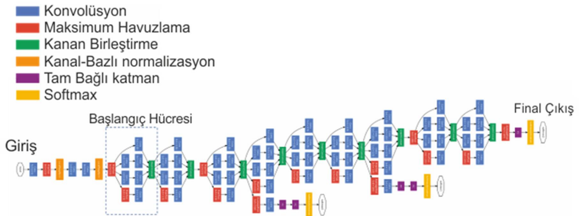
Şekil 3.22 Inception V1 yapısı [63]
