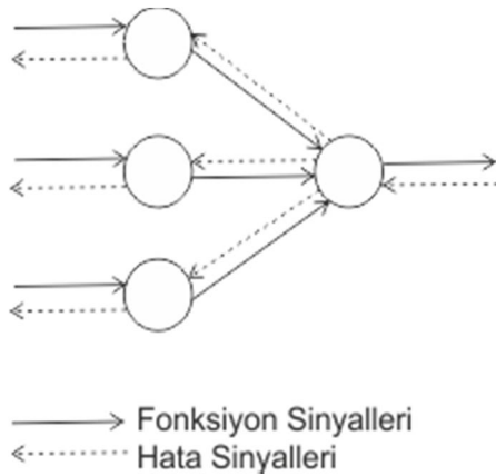
Şekil 3.5 Hata sinyalinin geri yayılımı
