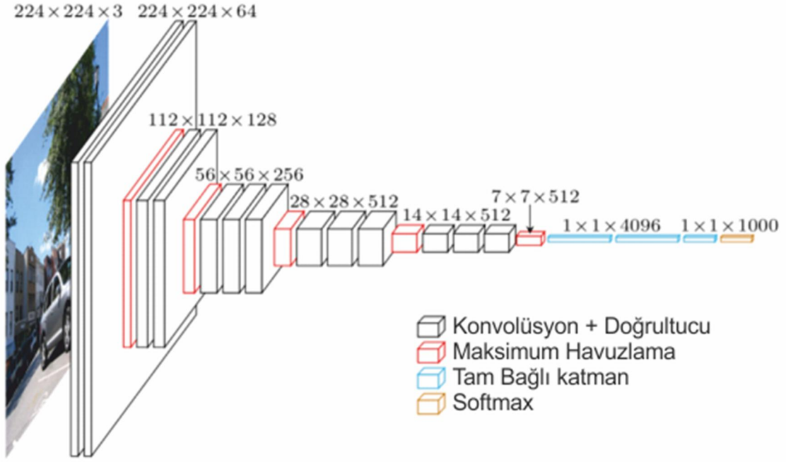
Şekil 3.21 VGGNet Yapısı [62]
