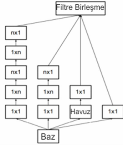
Şekil 4.2 Inception modeli-2 [43]
