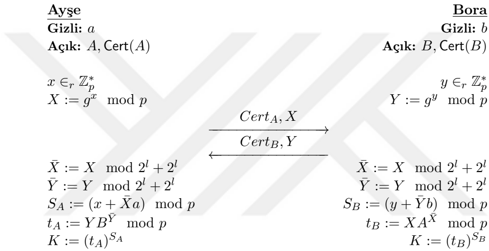
ŞEKİL 3.6: MQV Anahtar Anlaşma Protokolü ( l = |p/2| )
