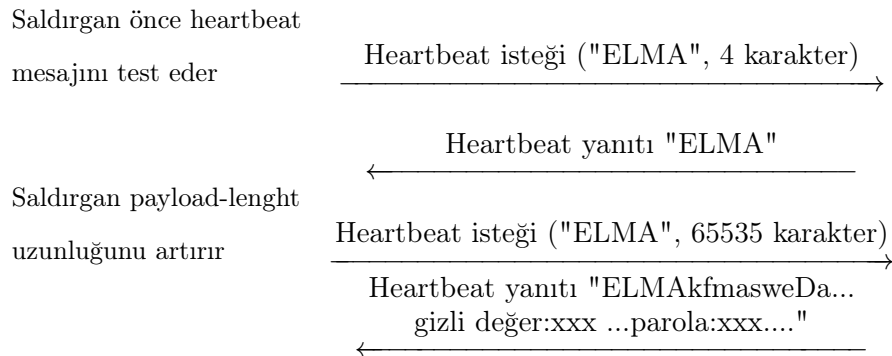
ŞEKİL 6.16: Heartbleed Saldırı Senaryosu
