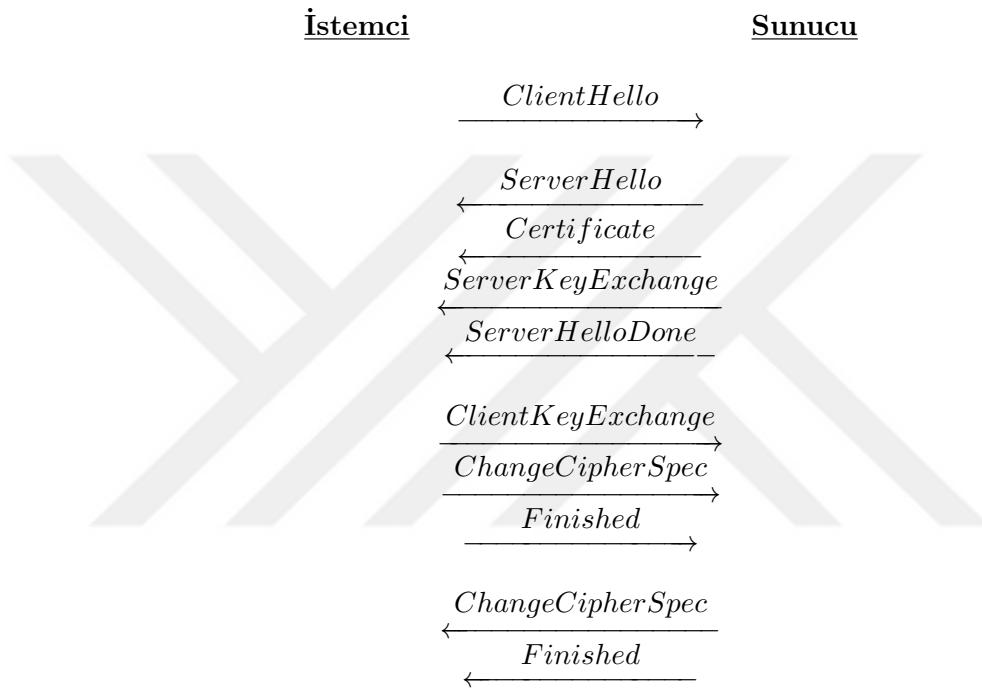
ŞEKİL 4.1: El Sıkışma Senaryosu
