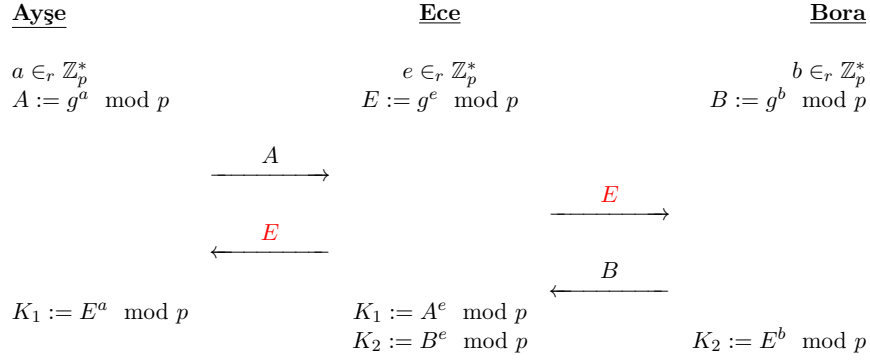
ŞEKİL 3.2: Temel Diffie-Hellman Anahtar Anlaşma Protokolüne Ortadaki Adam Saldırısı
