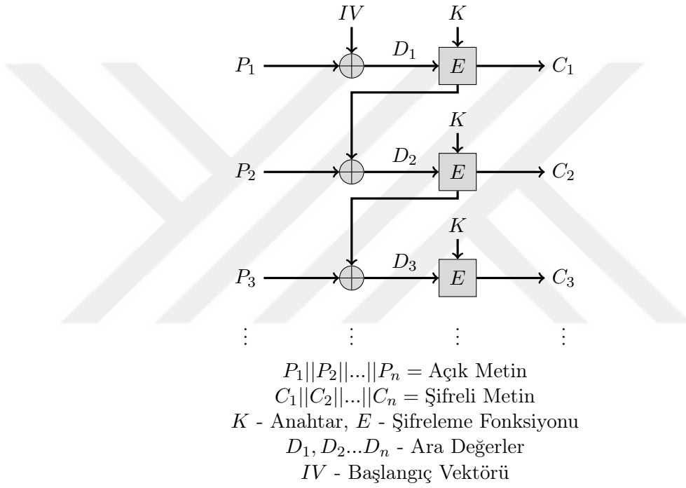
ŞEKİL 6.12: CBC Kipi ile Şifreleme
