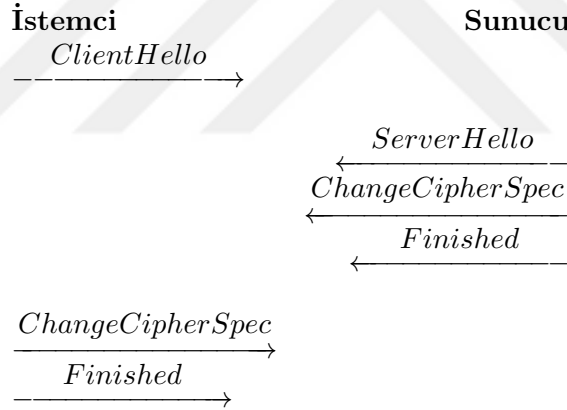
ŞEKİL 4.2: Oturum Yenileme
