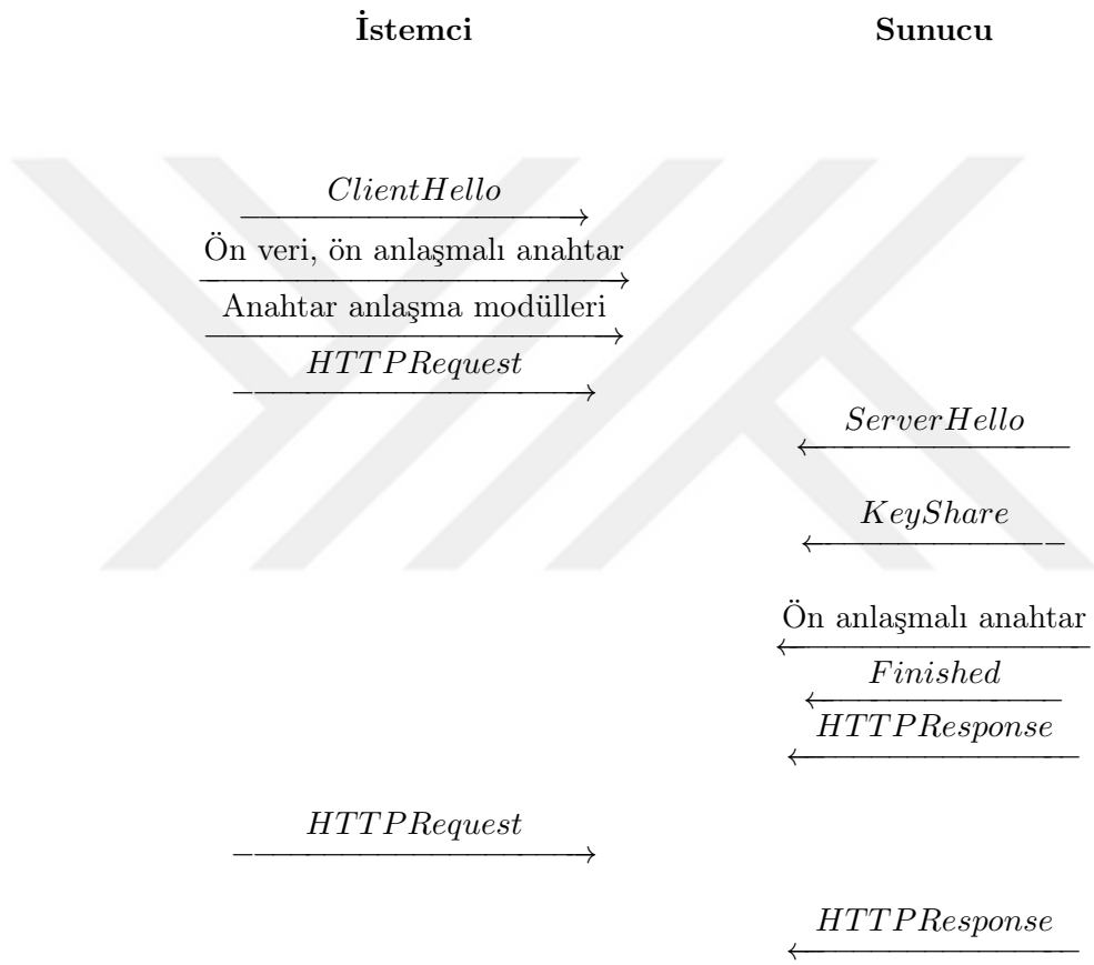
ŞEKİL 4.4: TLSv1.3 0-RTT
