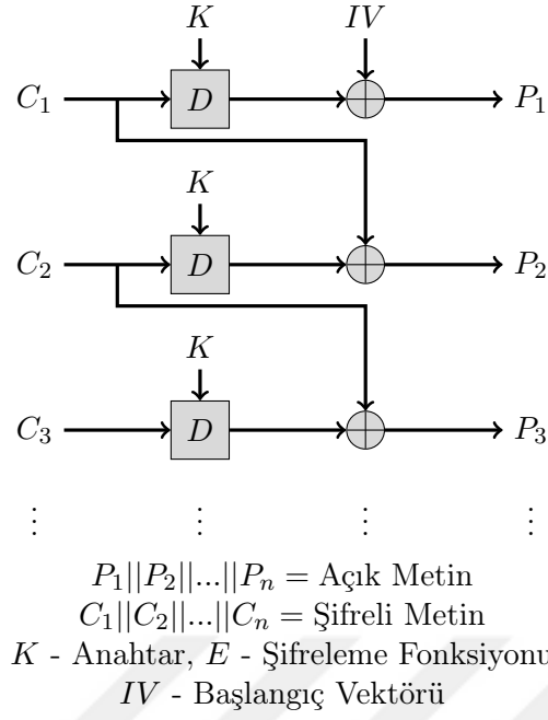
ŞEKİL 6.5: CBC Kipi ile Şifre Çözme
