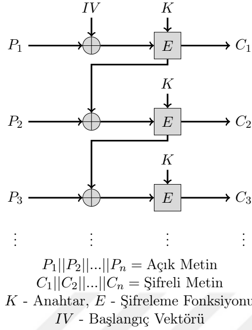
ŞEKİL 6.4: CBC Kipi ile Şifreleme
