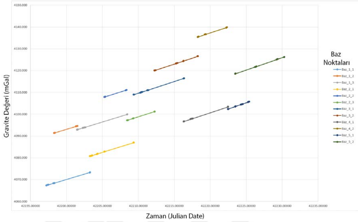
Şekil 4.2: Kayma (Drift) düzeltilmesi için baz noktalarında alınmış ölçümlerin zamana göre grafiği
