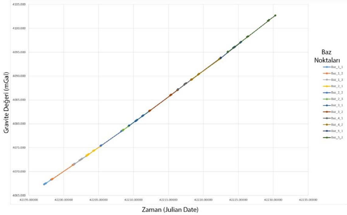
Şekil 4.3: Kayma (Drift) düzeltilmesi için baz noktalarında alınmış ölçümlerin zaman göre düzenlenip doğru haline getirilmiş grafiği
