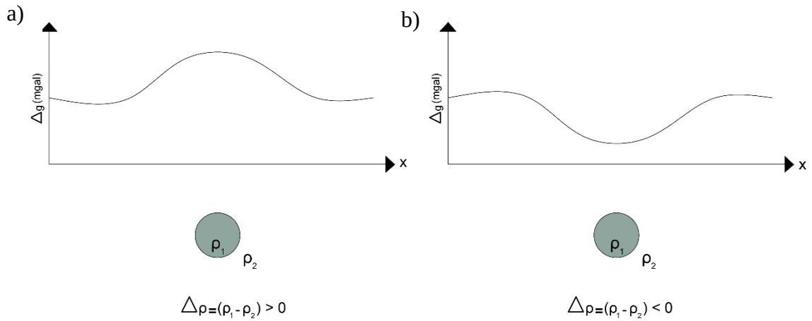
Şekil 2.1: a) Çevresine göre yüksek yoğunluğa sahip bir yer altı yapısının gravite yöntemi sonucu vereceği gravite anomalisi b) çevresinde göre alçak yoğunluğa sahip bir yeraltı yapısının gravite yöntemi sonucu vereceği gravite anomalisi verilmiştir
