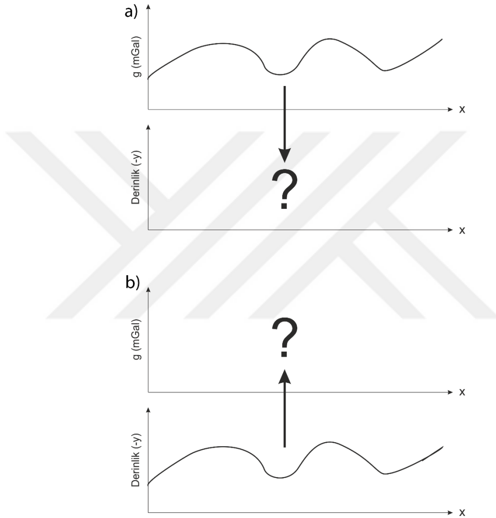
Şekil 2.16: Düz çözüm yöntemi a), arazide toplanan gerçek verilerden yeraltı yapısı kestirimi, ters çözüm yöntemi b), yeraltı yapısı modelinden kuramsal olarak jeofizik tepkinin hesaplanarak yinelemeler ile araziden elde edilen verilere uyarlanması
