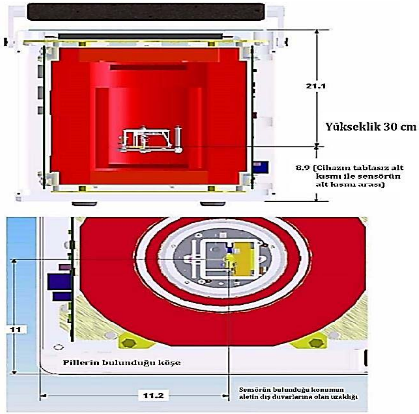
Şekil 2.20: Scintrex CG-5 cihazının içerisindeki sensörün yeri ve içyapısı (Scintrex, 2006)
