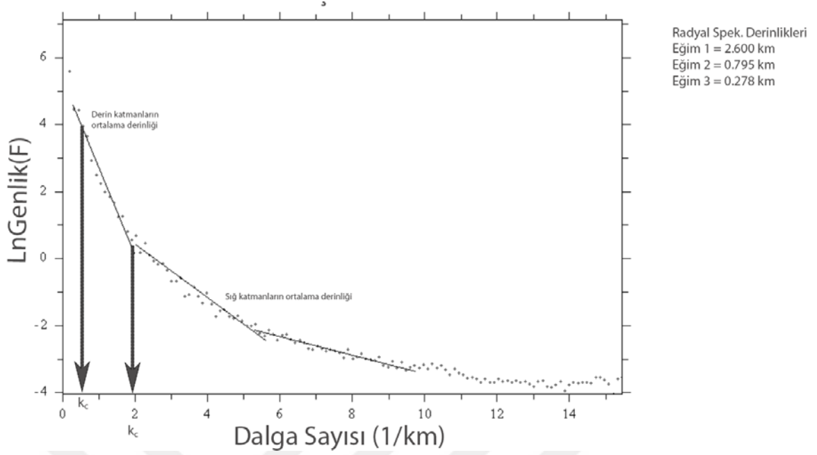
Şekil 4.6: Bouguer anomalilerinin radyal ortalama logaritmik genlik spektrumu ve kritik dalga sayıları ile kaynak arayüzey ortalama derinliklerinin kestirimi
