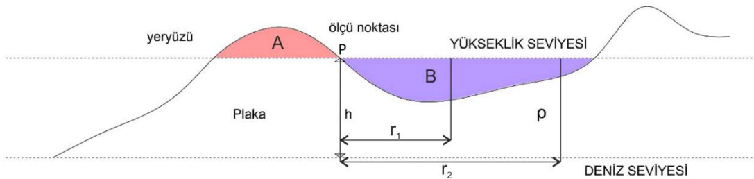
Şekil 2.10: Yükseklik düzeltmesi yapılırken mavi ile gösterilen B kısmı (çukur) malzeme dolu olarak, kırmızı renk ile gösterilen A kısmı (tepe) ise boşluk olarak hesaplanmıştır, şekilde r_1 ve r_2 topoğrafya düzeltmesi el/abak ile yapılırken kullanılan eş merkezli silindirlerin yarıçapları ve h ise indirgeme yüksekliğidir, bu etkileri düzeltmek amacı ile Topoğrafya düzeltmesi yapılır
