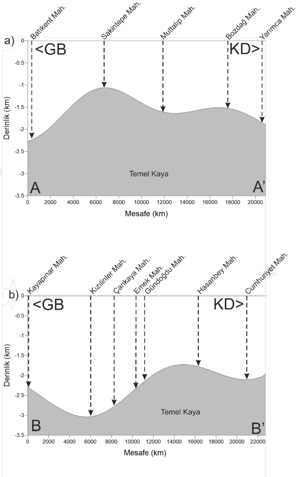
Şekil 4.12: Şekil 4.11'de gösterilen AA' a) ve BB' b) profillerinin derinlik haritası üzerinden alınmış kesitleri. En derin kısım güney olmak üzere güneyden kuzeye doğru bir artış görülmektedir
