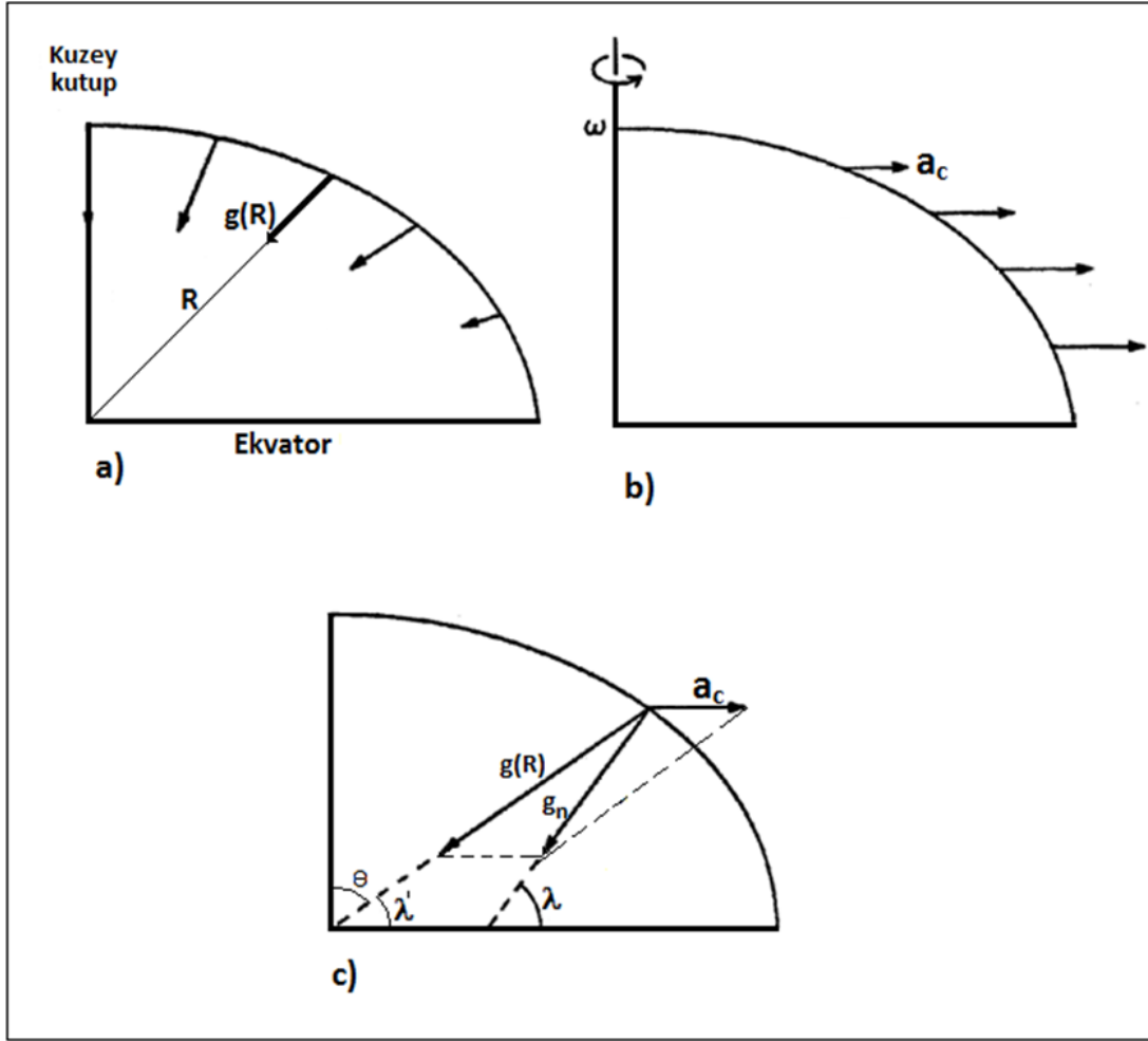
Şekil 2.7: Dönme elipsoidine dik (normal) olan gravite ivmesi ( g_n ), merkez kaç ivmesi ve yerin çekirdeğine yönelen gravite ivmesinin şematik gösterim, burada R: Elipsoid yarıçapı, \theta : Boylam açısı, \lambda' : Geosantrik enlem açısı, \lambda : Coğrafi enlem açısı, g(R) : Yerin çekirdeğine yönelen radyal doğrultuda gravite ivmesi veya mutlak gravite şeklindedir (Oruç, 2013)
