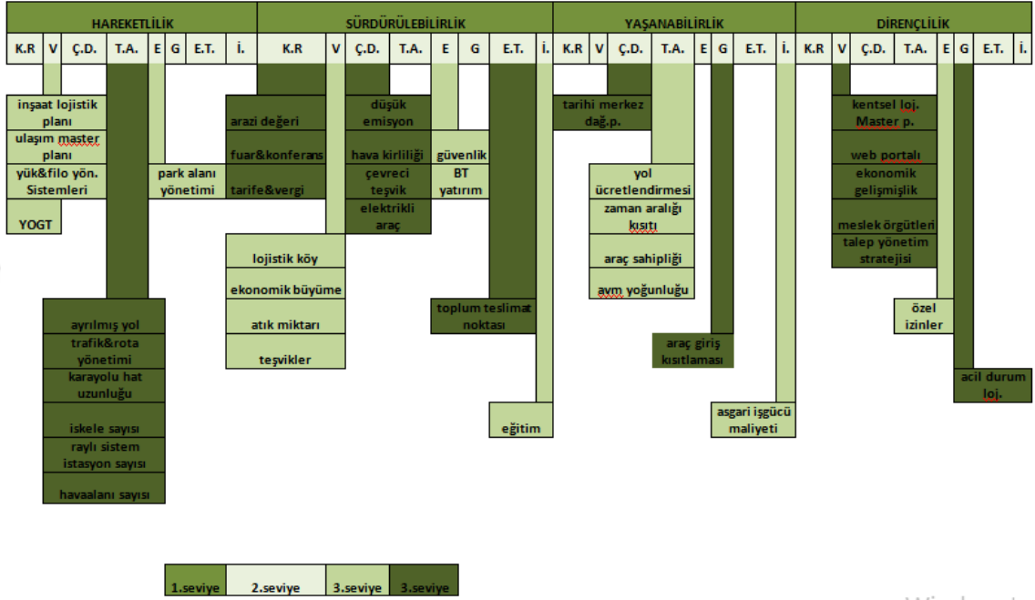
Şekil 3.4 - AHS Hiyerarşisi
