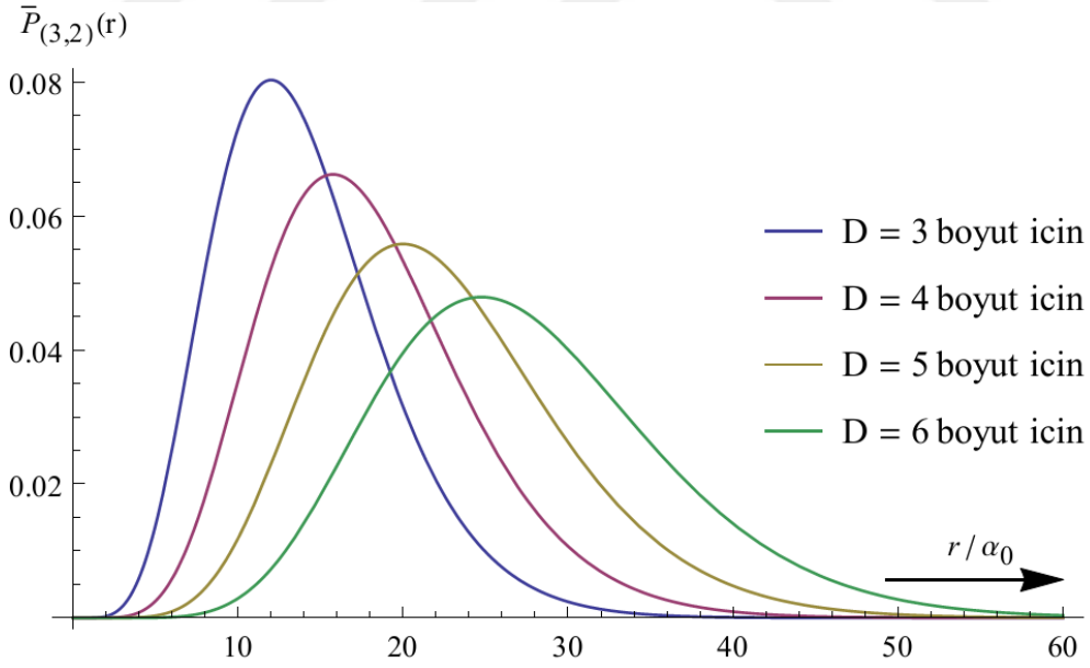
Şekil 2.20. n=3, k=2 kuantum sayıları için \bar{P}_{(3,2)} olasılık yoğunluk fonksiyonlarının grafikleri
