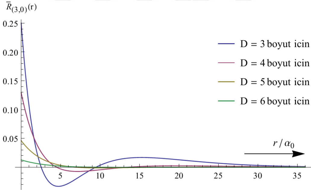
Şekil 2.8. n=3 , k=0 için \bar{R}_{(3,0)} radyal dalga fonksiyonlarının grafikleri
