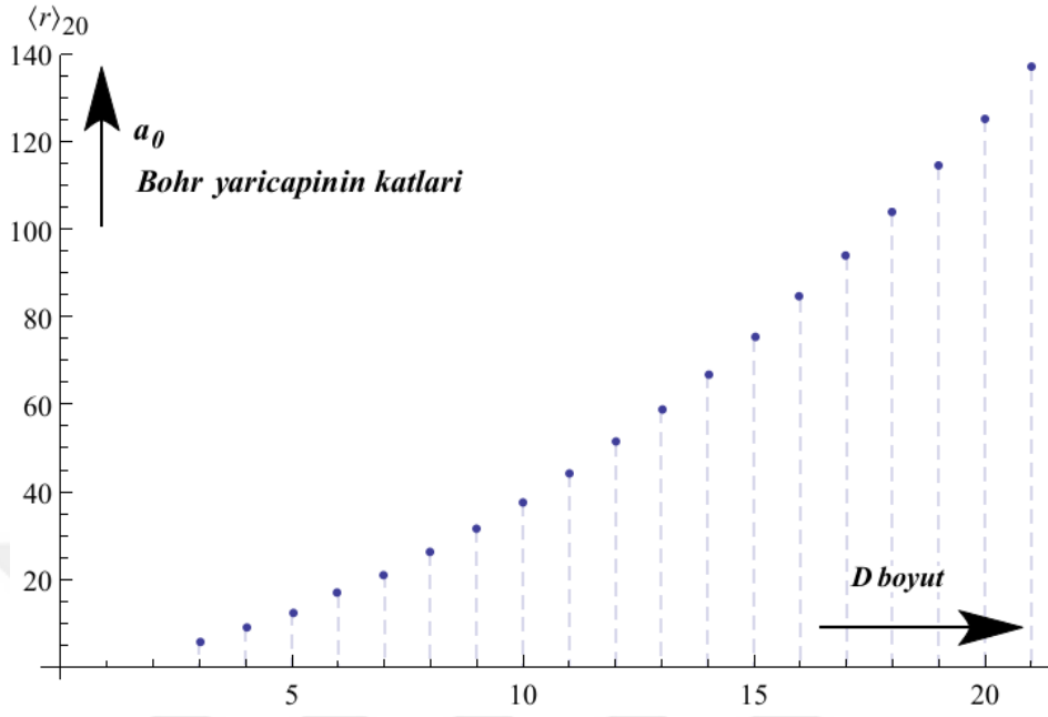
Şekil 2.3. \langle r \rangle_{(2,0)} yarıçap beklenen değerinin D boyutuna göre değişim grafiği
