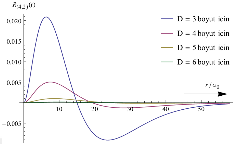
Şekil 2.13. n=4 , k=2 kuantum sayıları için \bar{R}_{(4,2)} radyal dalga fonksiyonlarının grafikleri
