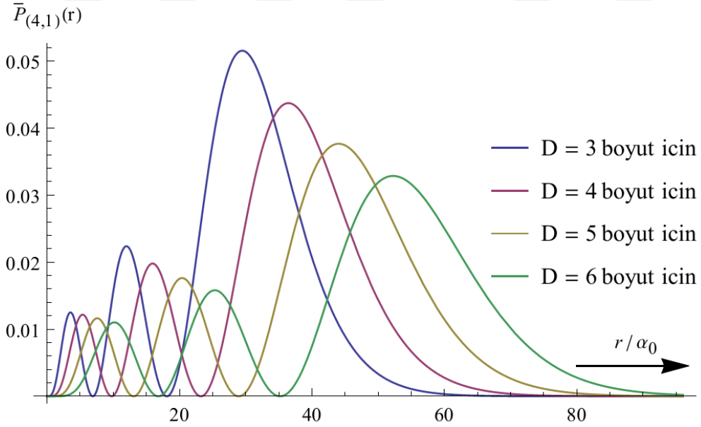
Şekil 2.22. n=4, k=1 kuantum sayıları için \bar{P}_{(4,1)} olasılık yoğunluk fonksiyonlarının grafikleri
