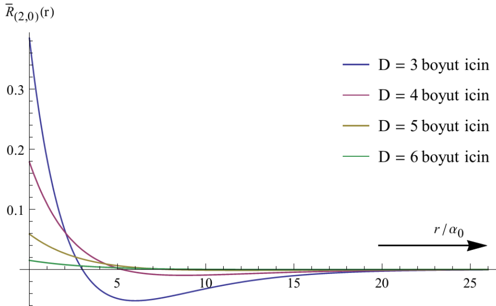
Şekil 2.6. n=2, k=0 için \bar{R}_{(2,0)} radyal dalga fonksiyonlarının grafikleri
