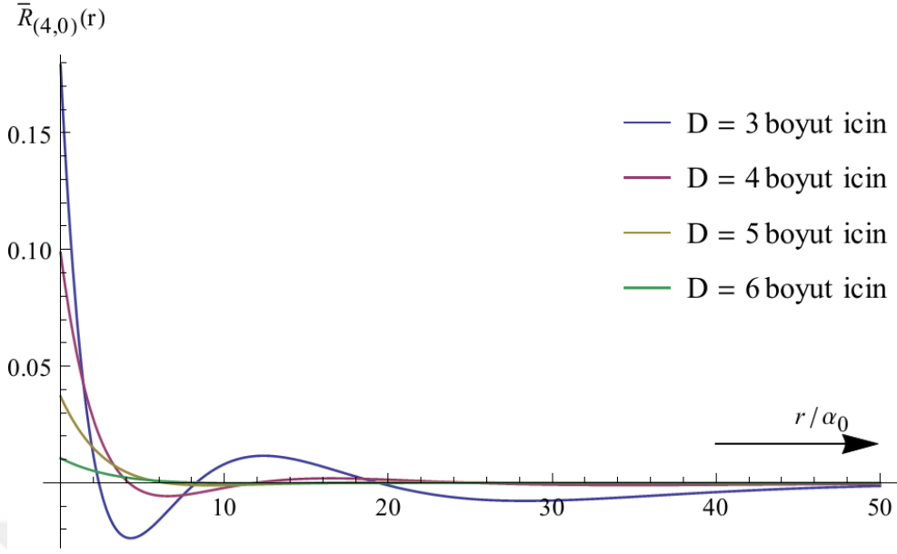
Şekil 2.11. n=4, k=0 kuantum sayıları için \bar{R}_{(4,0)} radyal dalga fonksiyonlarının grafikleri
