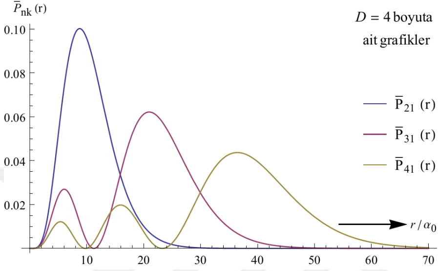
Şekil 2.29. D=4 boyutta \bar{P}_{21}(r) , \bar{P}_{31}(r) , \bar{P}_{41}(r) boyutsuz olasılık yoğunluk fonksiyonlarının karşılaştırmalı grafikleri
