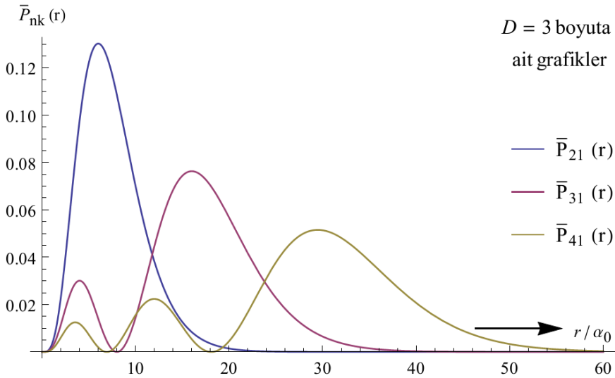
Şekil 2.26. D=3 boyutta \bar{P}_{21}(r) , \bar{P}_{31}(r) , \bar{P}_{41}(r) radyal olasılık yoğunluk fonksiyonlarının karşılaştırmalı grafikleri
