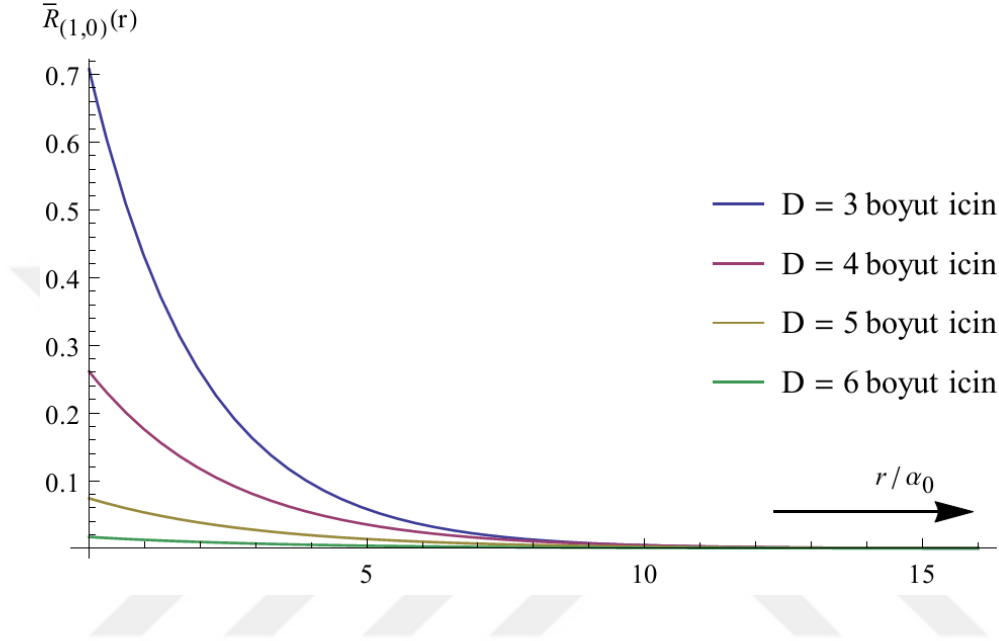
Şekil 2.5. n=1, k=0 için \bar{R}_{(1,0)} radyal dalga fonksiyonlarının grafikleri
