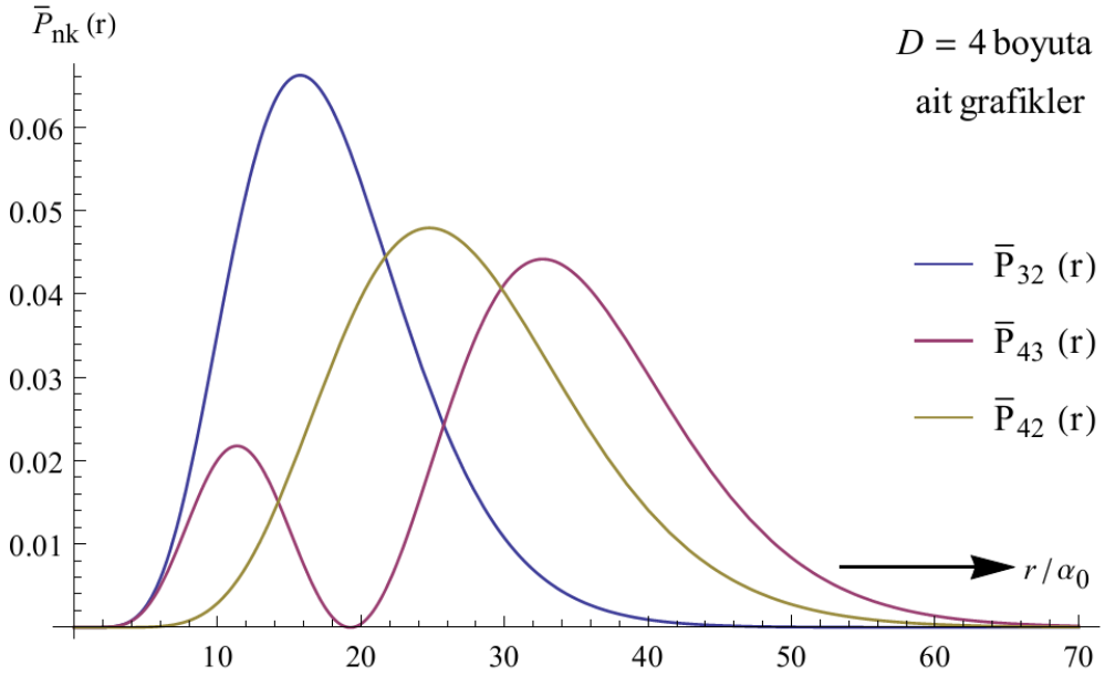
Şekil 2.30. D=4 boyutta \bar{P}_{32}(r) , \bar{P}_{42}(r) , \bar{P}_{43}(r) radyal olasılık yoğunluk fonksiyonlarının karşılaştırmalı grafikleri
