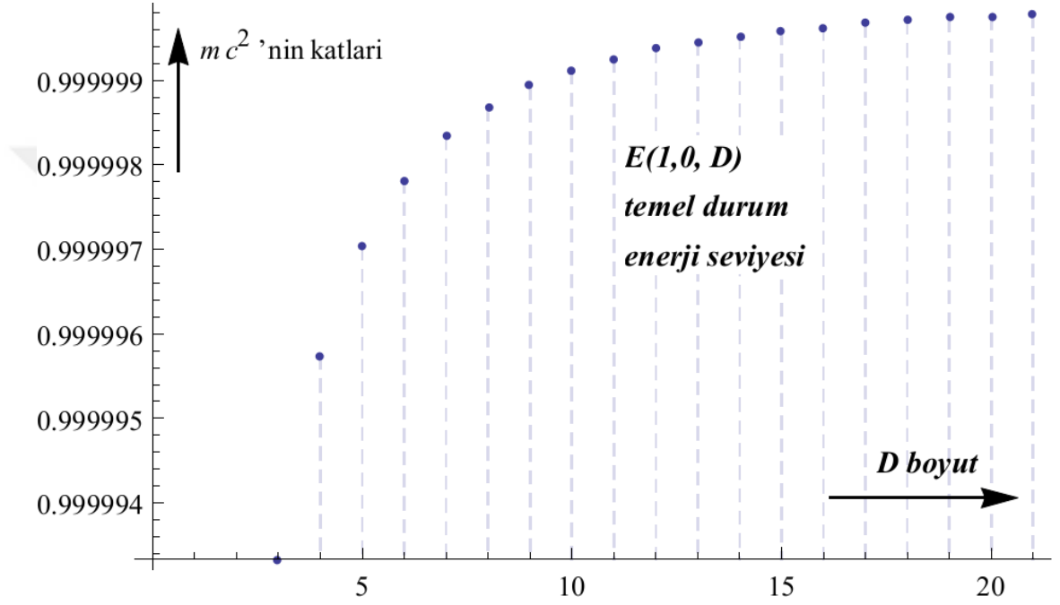
Şekil 2.1. Hidrojen benzeri atom için E(1,0,D) şeklindeki enerji öz değerlerinin D boyutuna göre değişim grafiği
