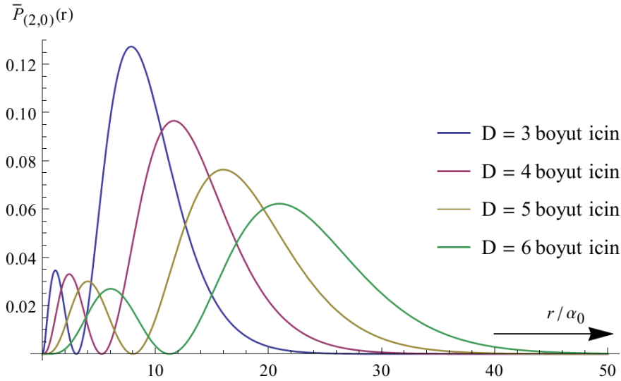
Şekil 2.16. n=2, k=0 kuantum sayıları için olasılık \bar{P}_{(2,0)} yoğunluk fonksiyonlarının grafikleri
