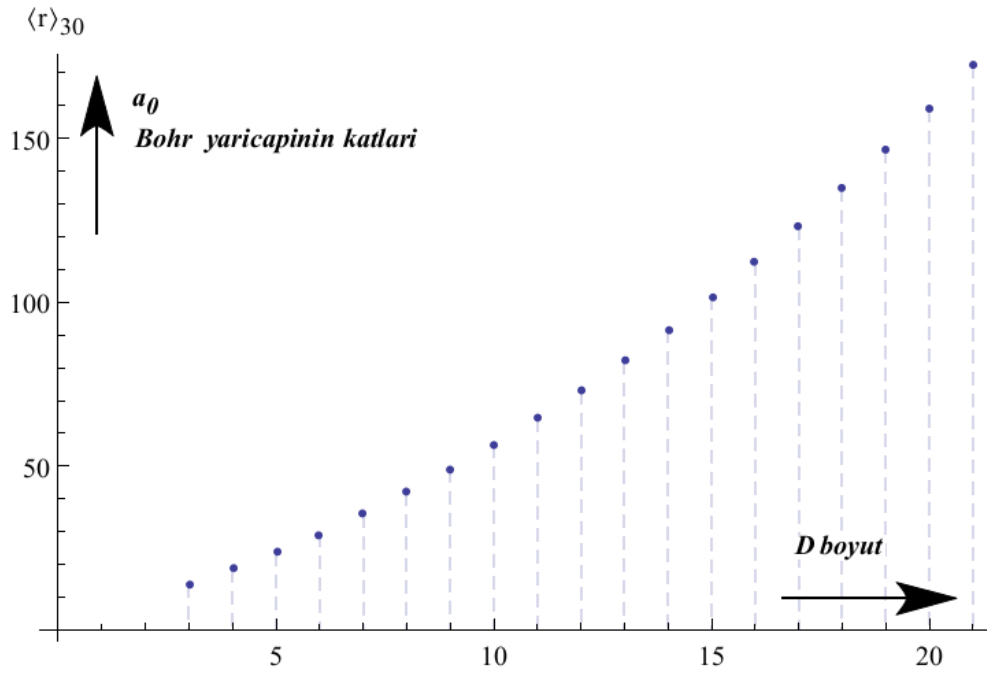
Şekil 2.4. \langle r \rangle_{(3,0)} yarıçap beklenen değerinin D boyutuna göre değişim grafiği
