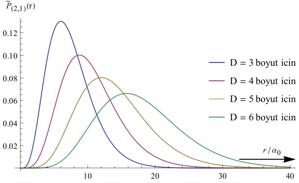
Şekil 2.17. n=2, k=1 kuantum sayıları için \bar{P}_{(2,1)} olasılık yoğunluk fonksiyonlarının grafikleri
