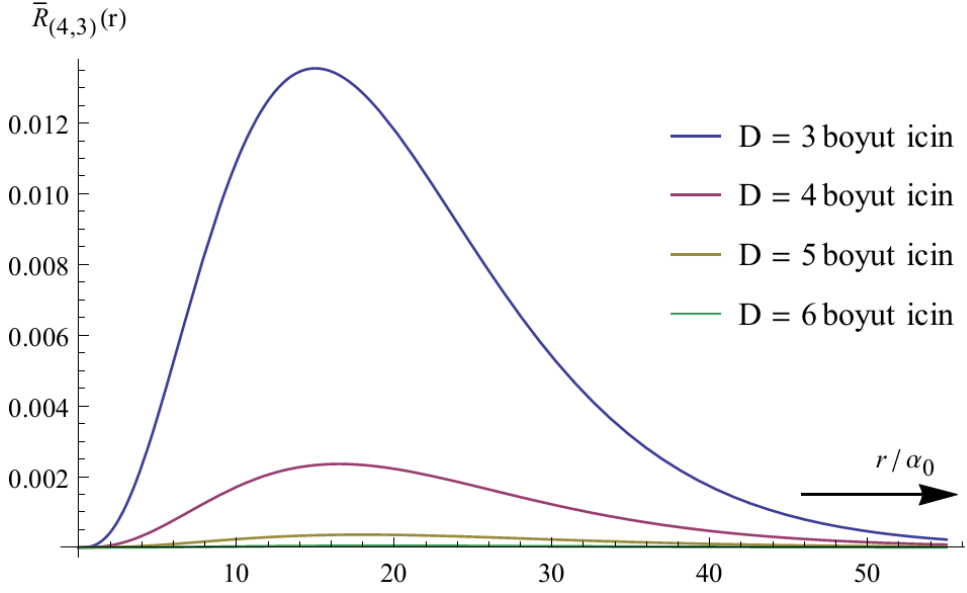
Şekil 2.14. n=4 , k=3 kuantum sayıları için boyutsuz şekilde çizilmiş \bar{R}_{(4,3)} radyal dalga fonksiyonlarının grafikleri
