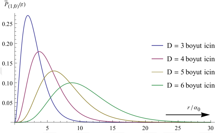
Şekil 2.15. n=1, k=0 kuantum sayıları için \bar{P}_{(1,0)} olasılık yoğunluk fonksiyonlarının grafikleri
