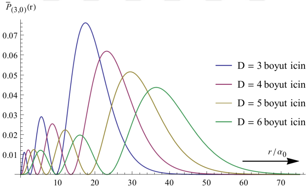
Şekil 2.18. n=3, k=0 kuantum sayıları için \bar{P}_{(3,0)} olasılık yoğunluk fonksiyonlarının grafikleri
