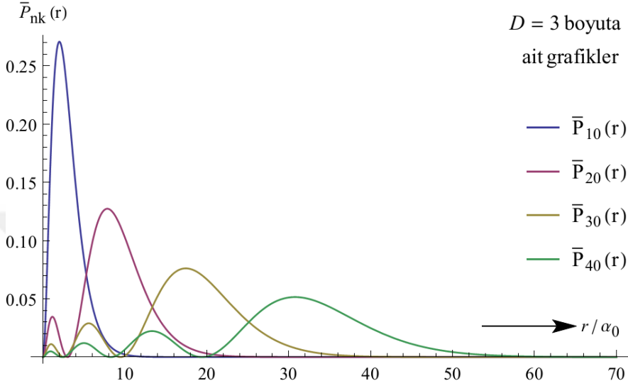
Şekil 2.25. D=3 boyutta \bar{P}_{10}(r) , \bar{P}_{20}(r) , \bar{P}_{30}(r) , \bar{P}_{40}(r) radyal olasılık yoğunluk fonksiyonlarının karşılaştırmalı grafikleri
