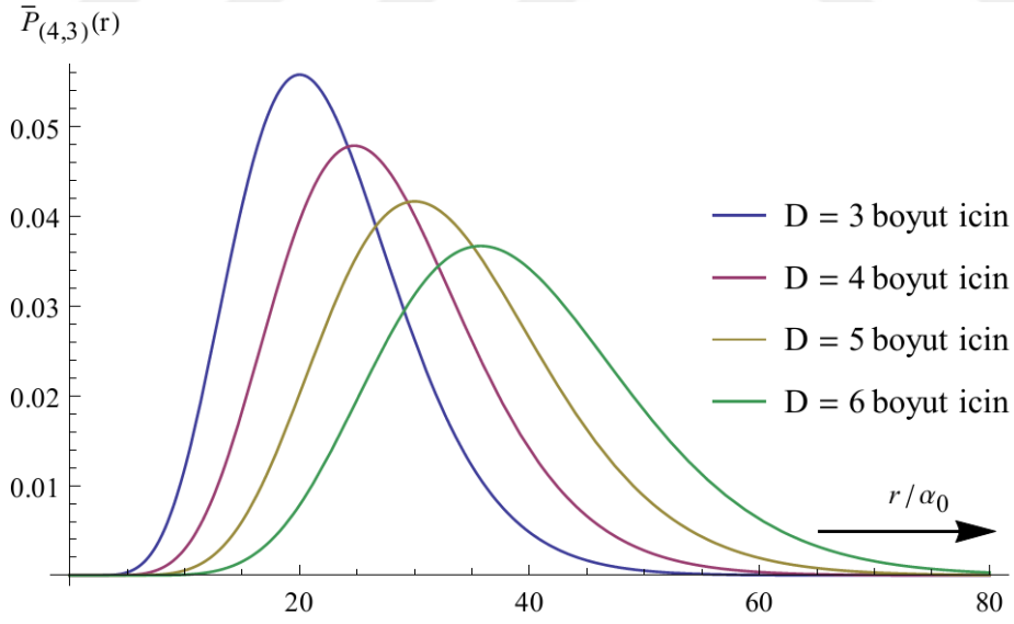
Şekil 2.24. n=4, k=3 kuantum sayıları için \bar{P}_{(4,3)} olasılık yoğunluk fonksiyonlarının grafikleri
