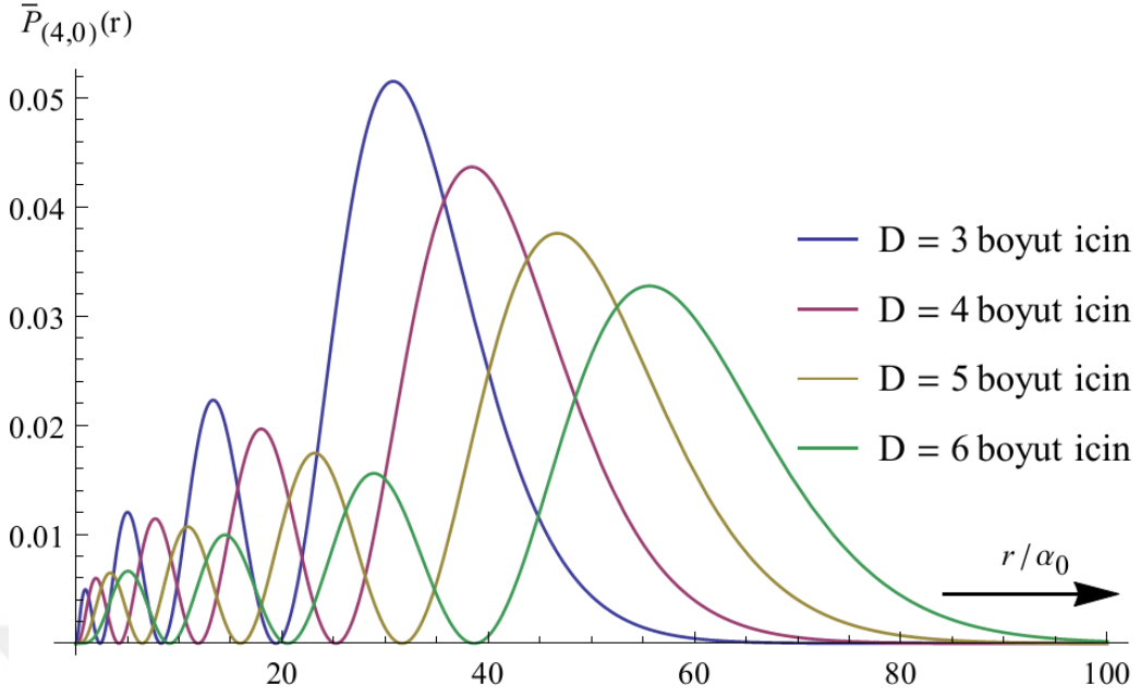
Şekil 2.21. n=4, k=0 kuantum sayıları için \bar{P}_{(4,0)} olasılık yoğunluk fonksiyonlarının grafikleri
