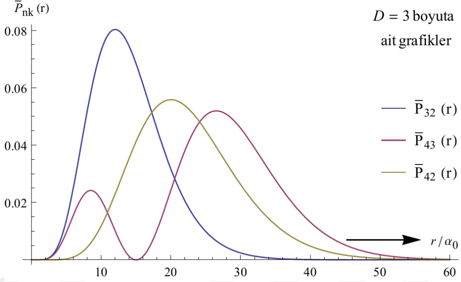
Şekil 2.27. D=3 boyutta \bar{P}_{32}(r) , \bar{P}_{42}(r) , \bar{P}_{43}(r) radyal olasılık yoğunluk fonksiyonlarının karşılaştırmalı grafikleri
