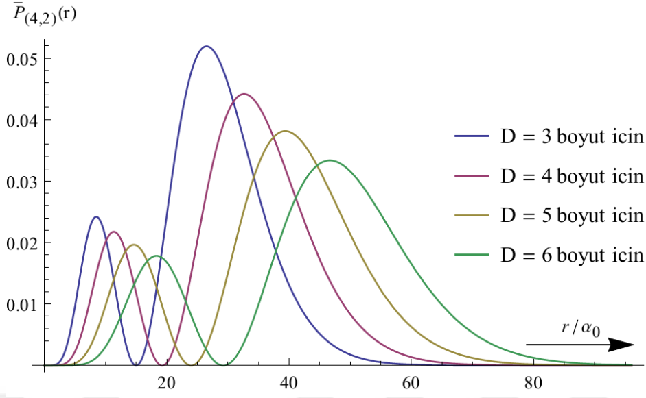
Şekil 2.23. n=4, k=2 kuantum sayıları için \bar{P}_{(4,2)} olasılık yoğunluk fonksiyonlarının grafikleri
