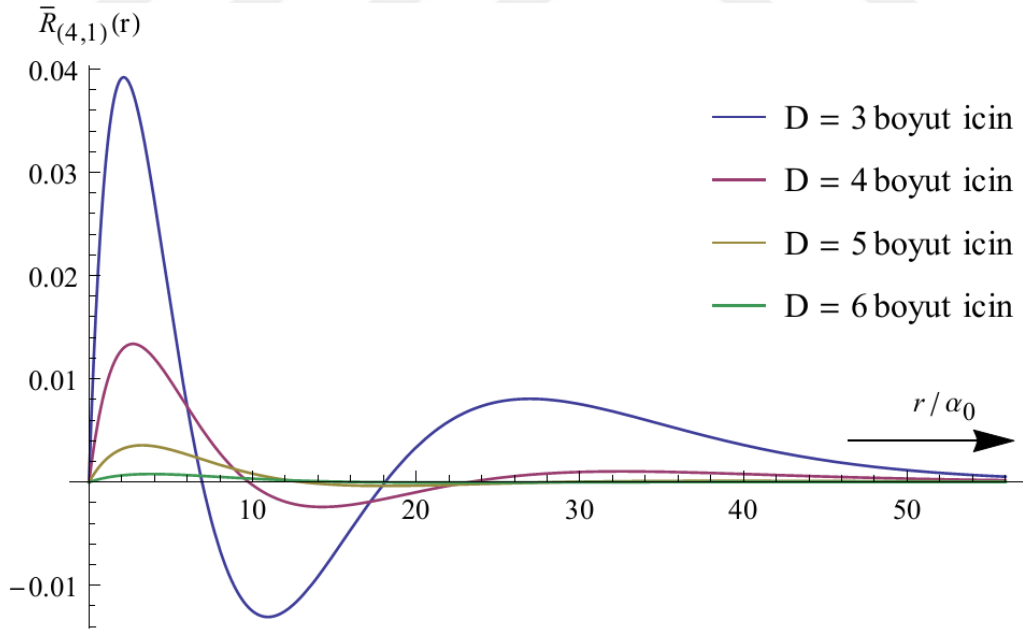
Şekil 2.12. n=4, k=1 kuantum sayıları için \bar{R}_{(4,1)} radyal dalga fonksiyonlarının grafikleri
