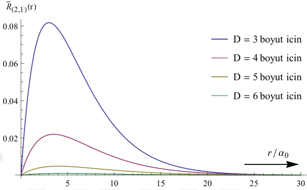
Şekil 2.7. n=2 , k=1 için \bar{R}_{(2,1)} radyal dalga fonksiyonlarının grafikleri
