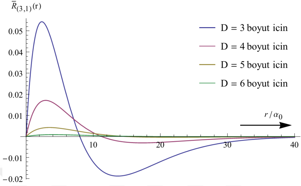
Şekil 2.9. n=3, k=1 için \bar{R}_{(3,1)} radyal dalga fonksiyonlarının grafikleri
