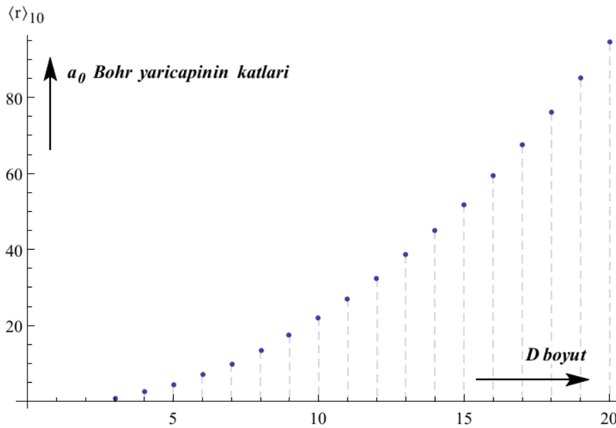
Şekil 2.2. \langle r \rangle_{(1,0)} yarıçap beklenen değerinin D boyutuna göre değişim grafiği
