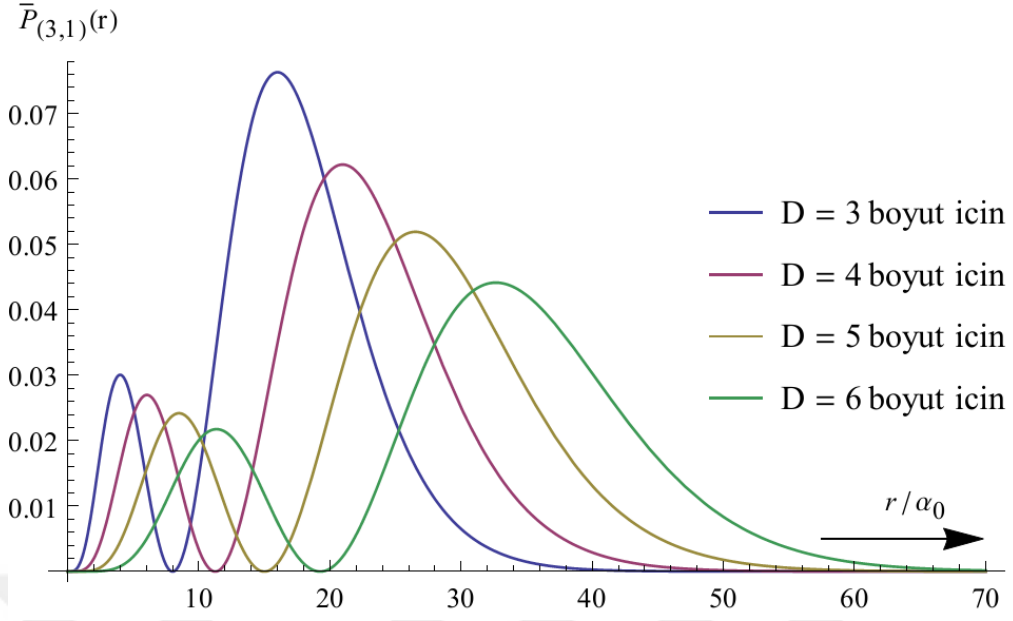
Şekil 2.19. n=3, k=1 kuantum sayıları için \bar{P}_{(3,1)} olasılık yoğunluk fonksiyonlarının grafikleri
