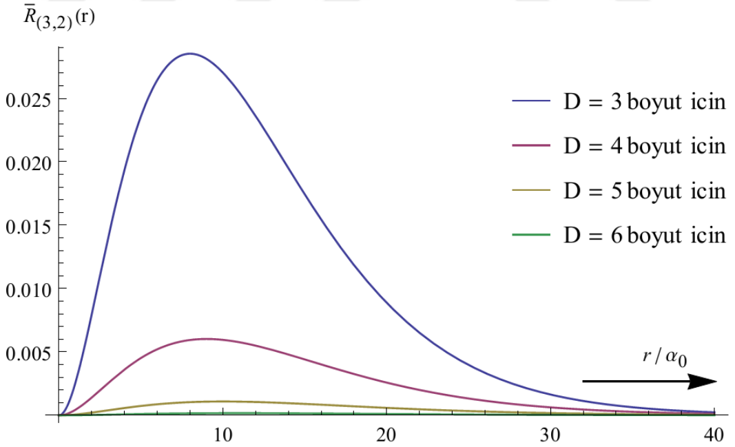
Şekil 2.10. n=3, k=2 kuantum sayıları için \bar{R}_{(3,2)} radyal dalga fonksiyonlarının grafikleri
