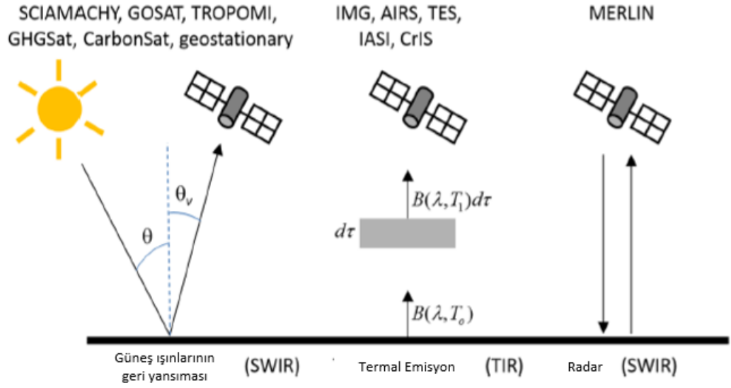
Şekil 2.3 : Metan ölçümünde kullanılan yöntemler, Jacob ve diğ. (2016)'dan uyarlanmıştır.
