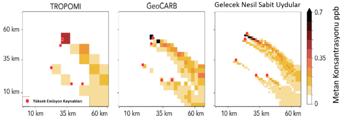
Şekil 2.2 : Fakrılı uydular için aynı kaynağa ait görüntüler, Cusworth ve diğ. (2018)'den uyarlanmıştır.
