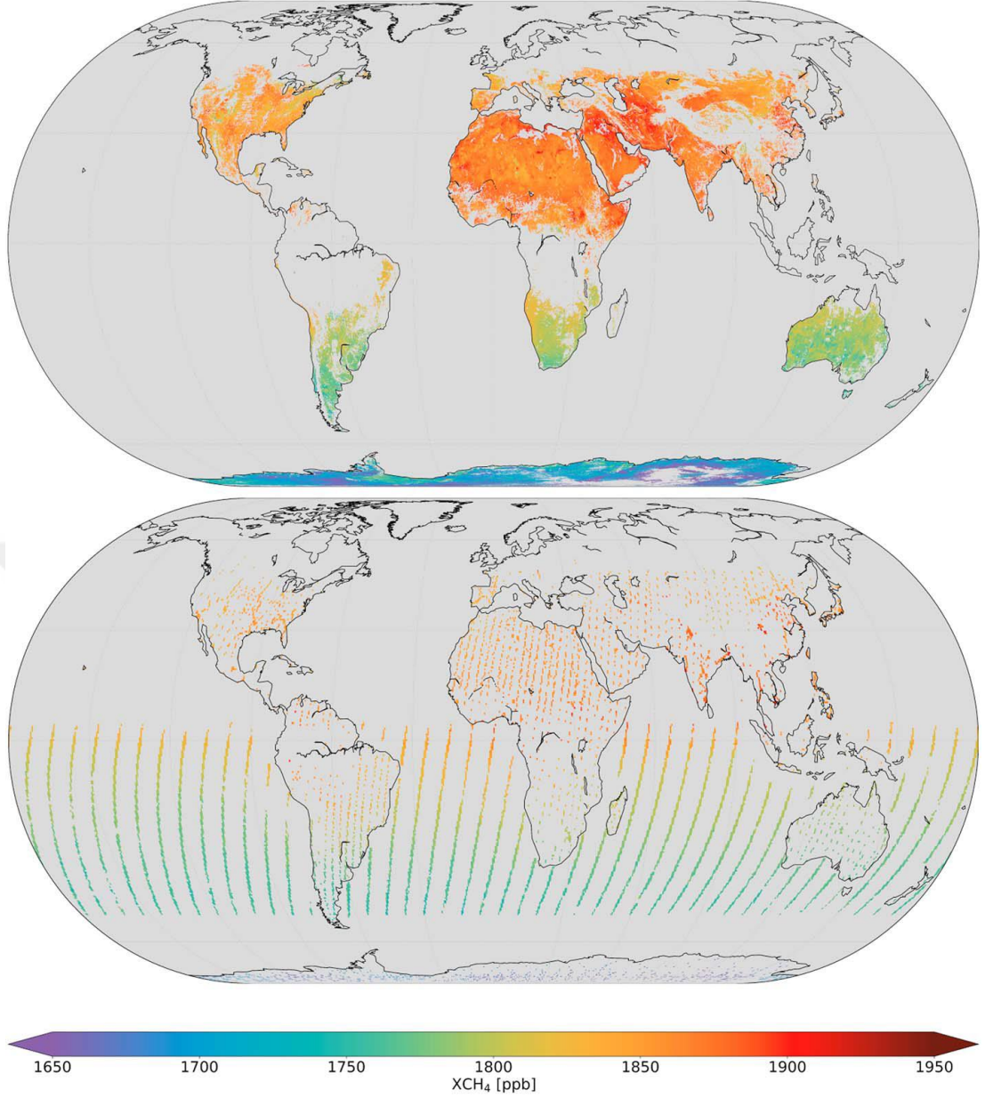
Şekil 2.1 : Küresel 12 Kasım – 30 Aralık 2017 döneminde CH 4 (ppb) TROPOMI (üst) ve GOSAT (alt) ortalama ölçümleriyle elde edilen dağılımı, Hu ve diğ. (2018)'den uyarlanmıştır.
