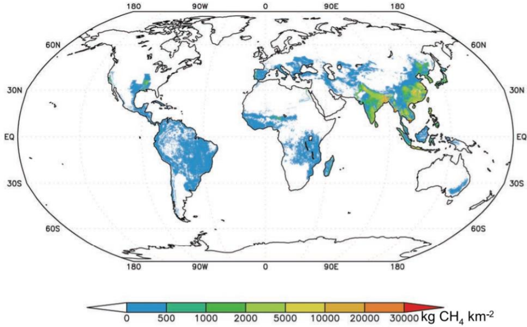
Şekil 3.6 : Pirinç tarlalarından kaynaklanan 5 dakika alansal çözünürlükte küresel yıllık metan emisyonları, Yan ve diğ. (2009)'dan uyarlanmıştır.
