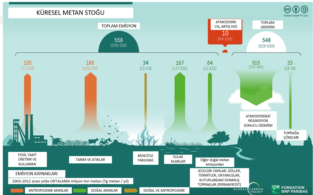
Şekil 1.6 : Küresel atmosferik metan kaynakları ve yutakları. Bousquet, Peregonand ve Canadell, (2013)'den uyarlanmıştır.
