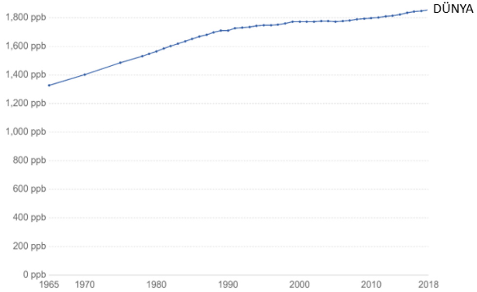
Şekil 1.10 : Küresel yıllık ortalama atmosferik metan konsantrasyonu EEA ve NOAA (2017)'den uyarlanmıştır.
