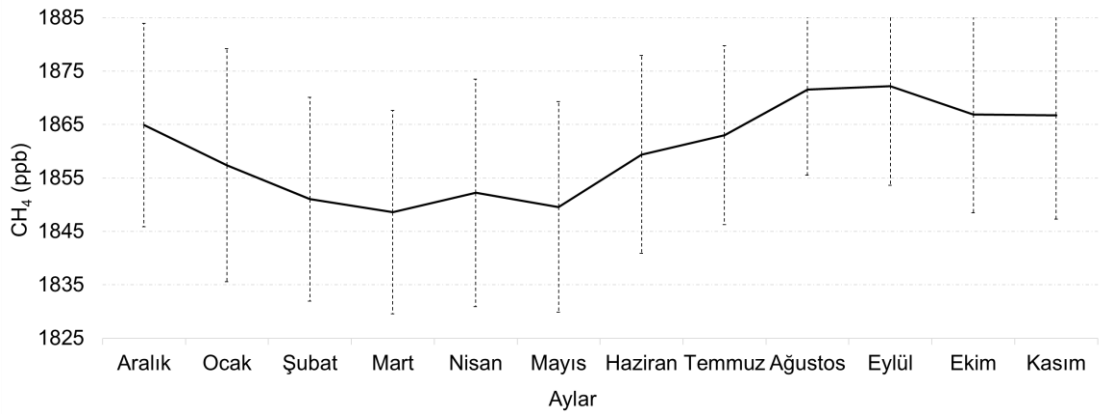
Şekil 4.9 : TROPOMI Türkiye aylık metan konsantrasyonu değişimi.
