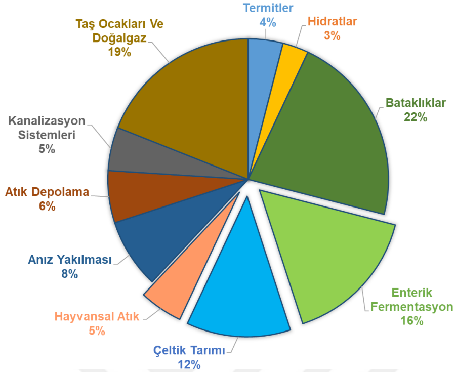
Şekil 1.7 : Küresel metan kaynakları ve yüzde olarak katkıları, NASA Methane Matters, ( t.y.) 'dan uyarlanmıştır.
