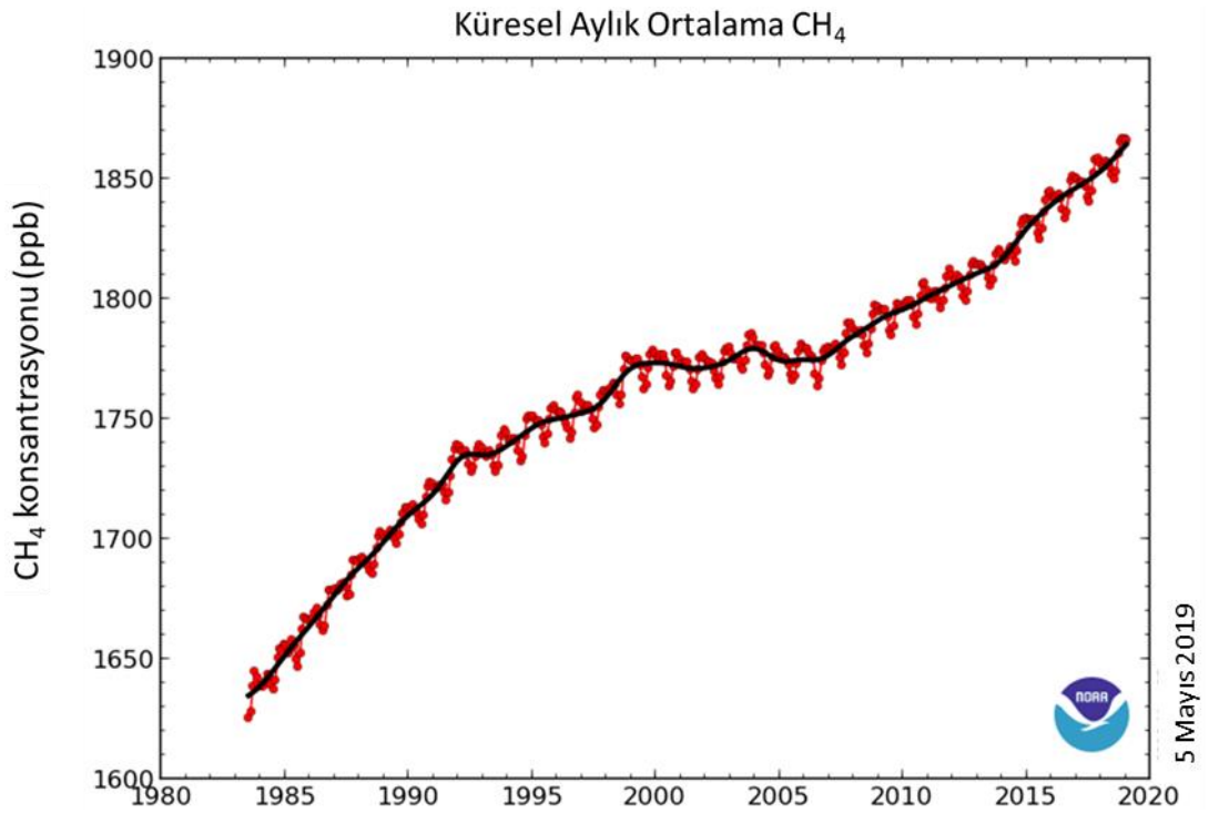
Şekil 1.11 : Küresel çapta aylık ortalama atmosferik metan konsantrasyonundaki eğilim, NOAA, (2019)'dan uyarlanmıştır.
