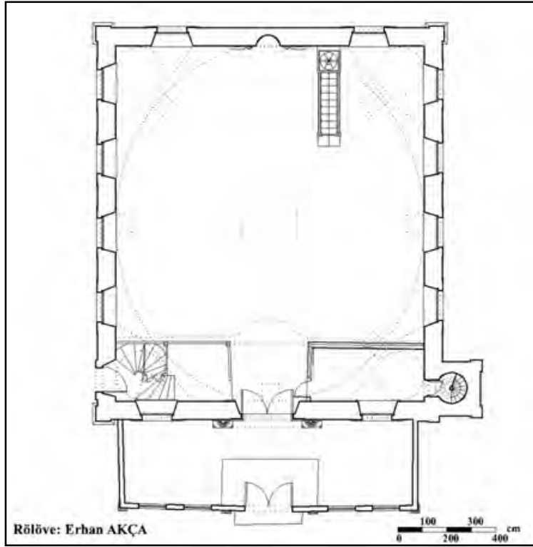
Resim 5.26. Abdülhamid döneminde yapılmış olan camilerinden Mahmudiye Hara cami planı (Aydın, 2009)
