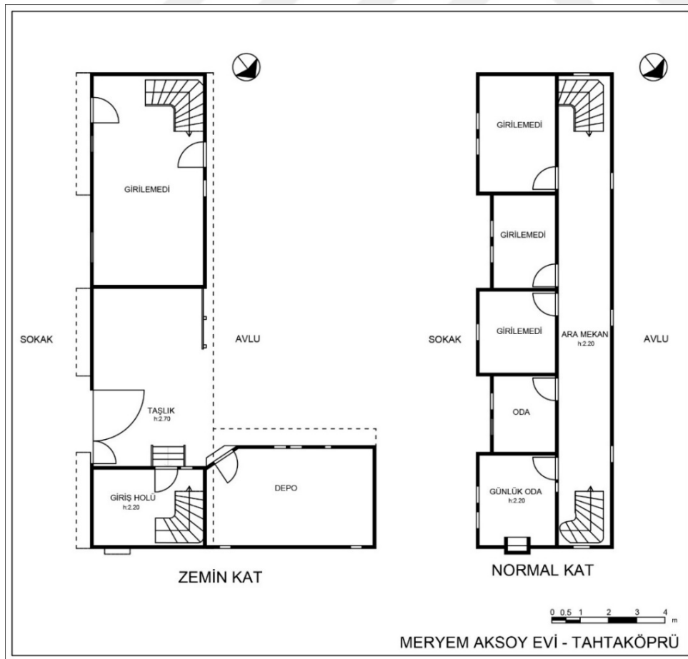
Resim 4.31. Meryem Aksoy evi kat planları
