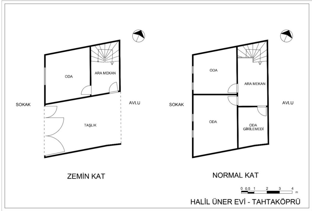
Resim 4.93. Halil Üner evi kat planları
