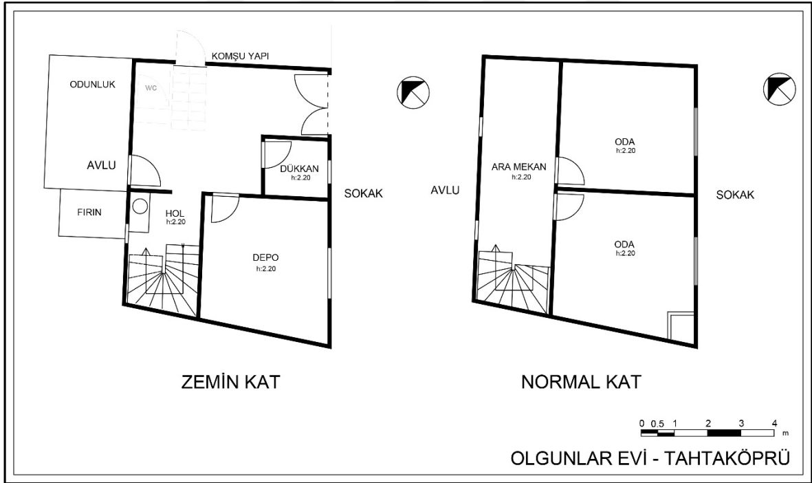
Resim 4.42. Olgunlar evi kat planları
