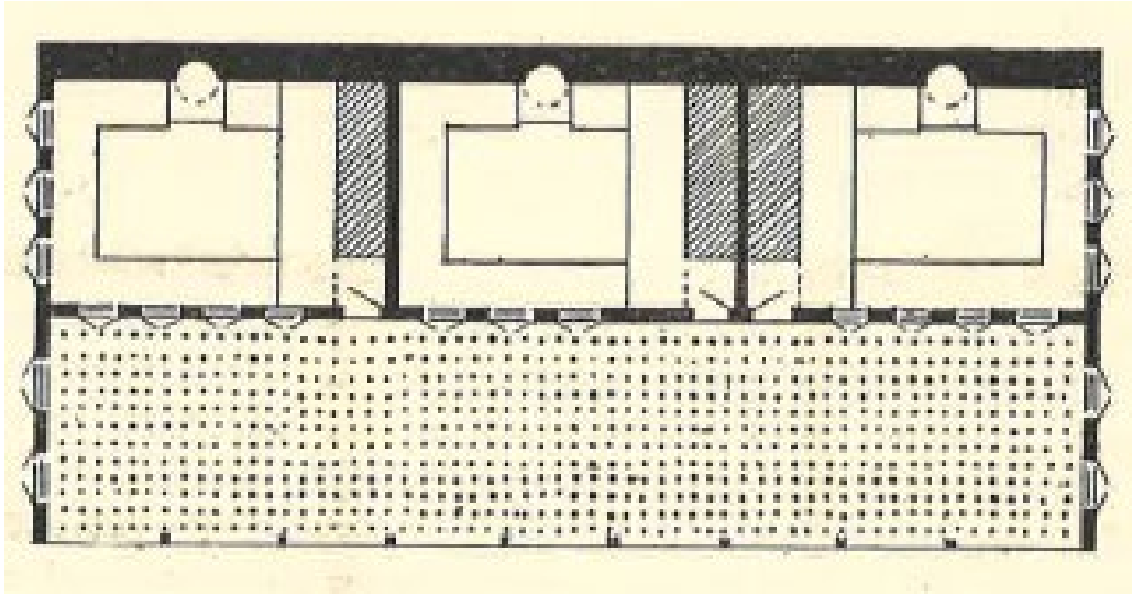
Resim 5.13. Dış sofalı tip (Eldem, 1954:34)
