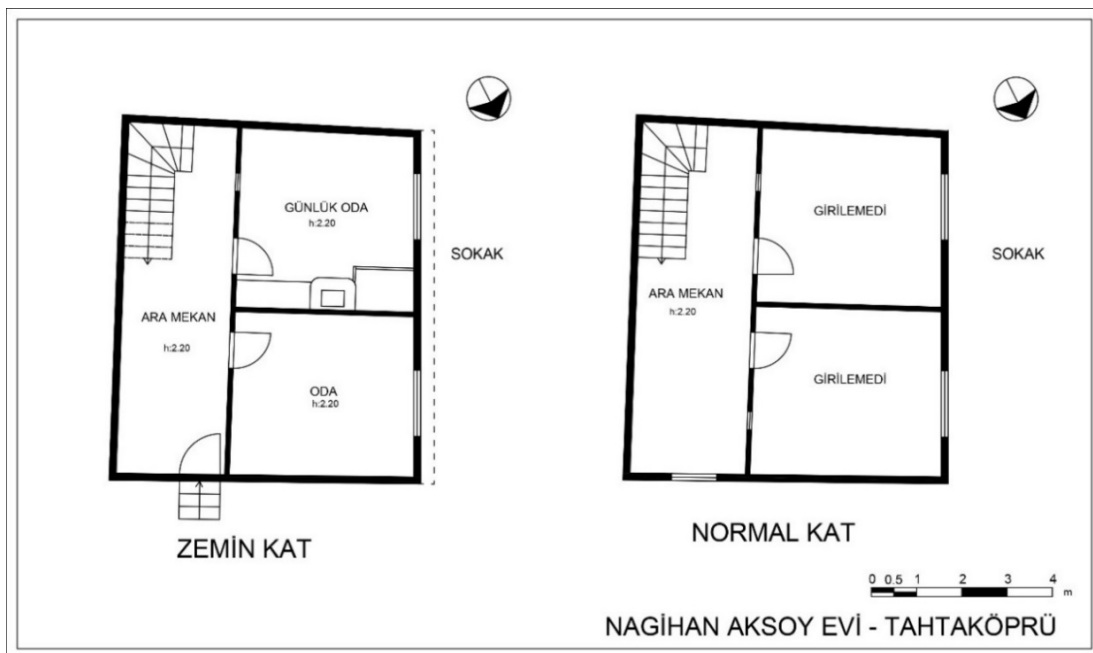
Resim 4.74. Nagihan Aksoy evi kat planları
