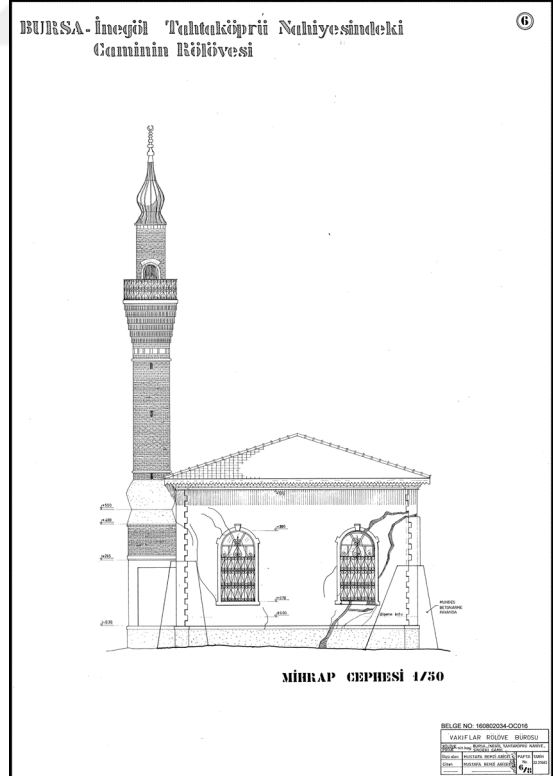
Resim 4.7. Tahtaköprü Hamidiye Camisi rölöve görüşleri(Tahtaköprü Belediyesi Arşivi)
