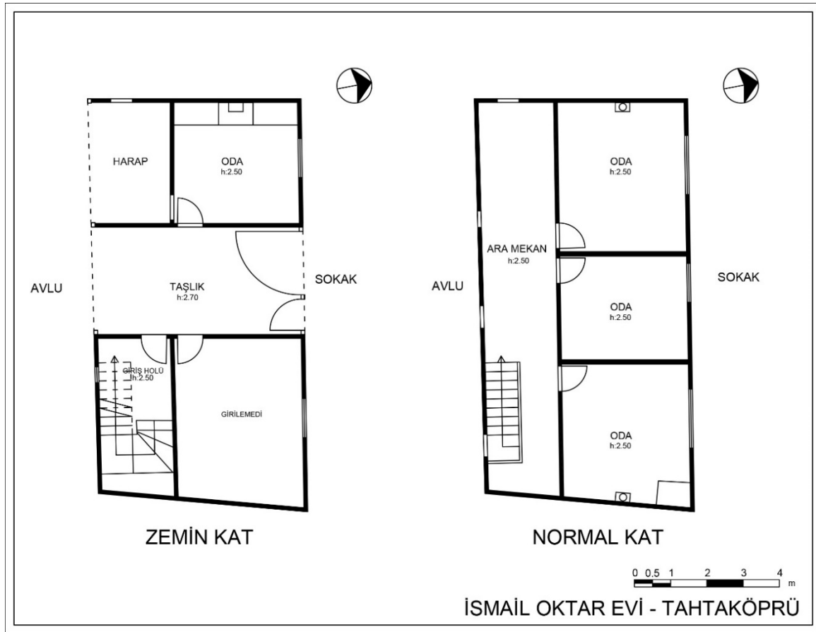
Resim 4.107. İsmail Oktar evi kat planları
