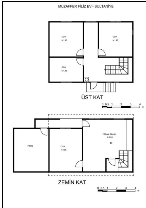
Resim 3.38. Muzaffer Filiz evi planı
