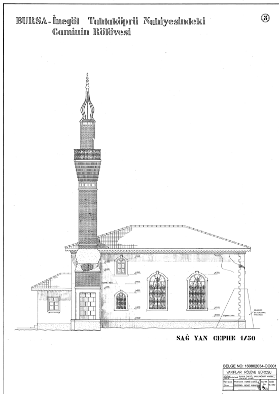
Resim 4.7. Tahtaköprü Hamidiye Camisi rölöve görüşleri(Tahtaköprü Belediyesi Arşivi)
