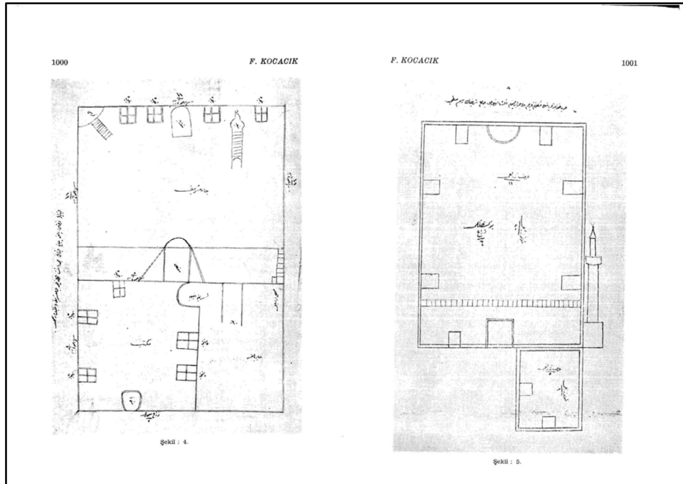
Resim 5.27. Muhacir köyleri için çizilmiş iki cami ve mektep planı (Kocacık, 1979)
