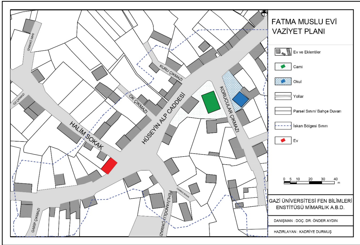
Resim 4.63. Fatma Muslu evi vaziyet planı
