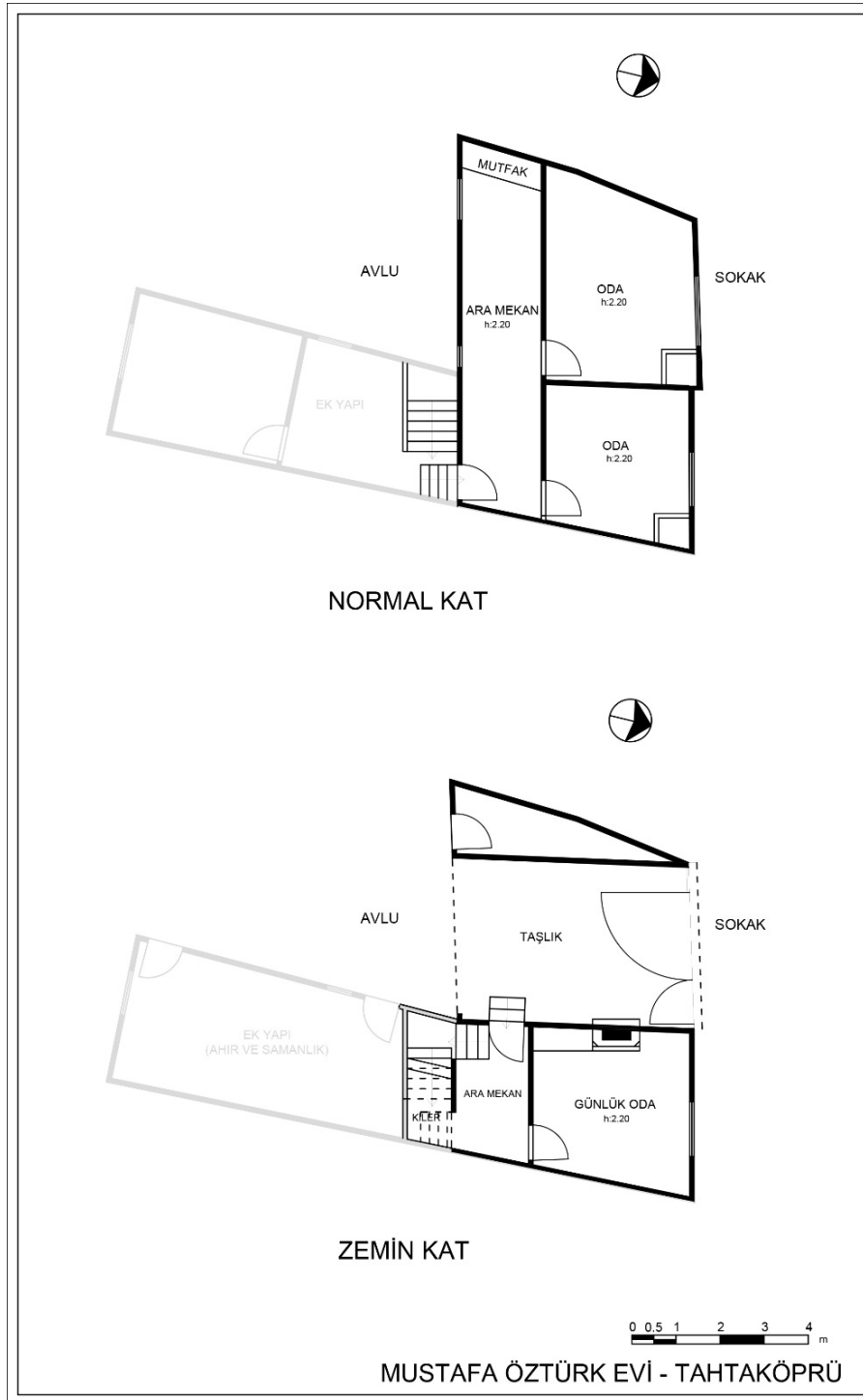
Şekil 4.13 Mustafa Öztürk evi kat planları
