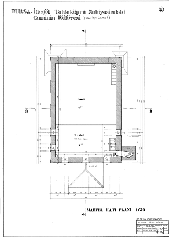
Resim 4.6. Tahtaköprü Hamidiye Camisi planları (Tahtaköprü Belediyesi Arşivi)
