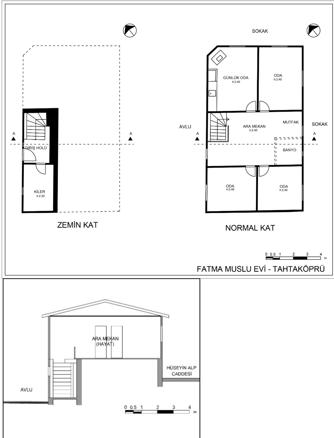
Resim 4.65. Fatma Muslu evi kat planları
