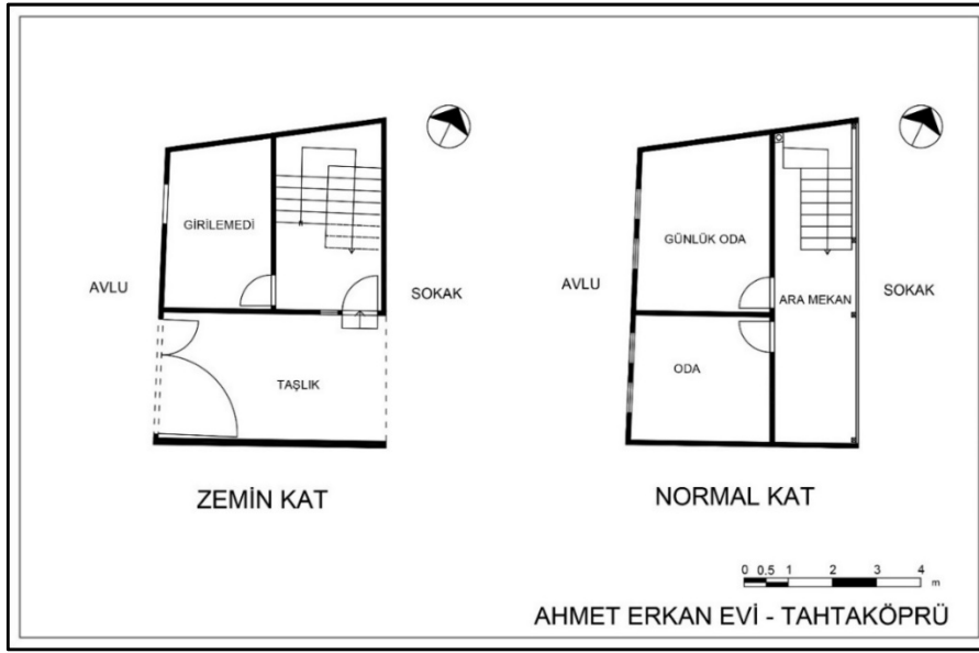
Resim 4.85. Ahmet Erkan evi kat planları
