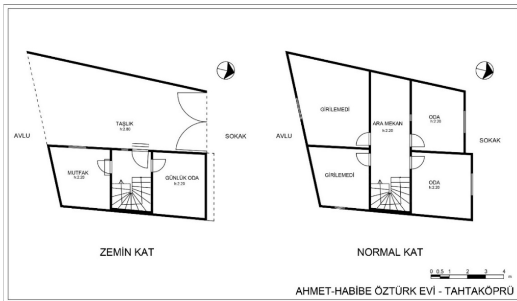
Resim 4.22. Ahmet –Habibe Öztürk evi kat planları
