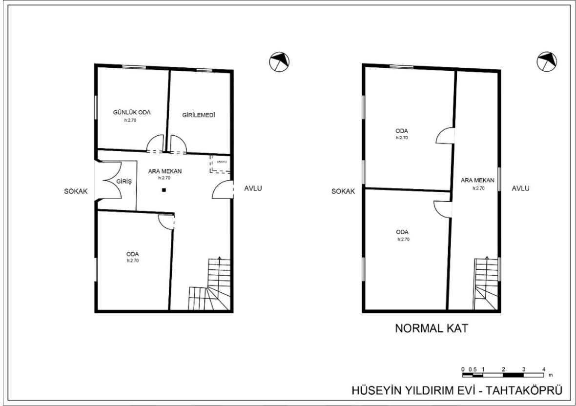
Resim 4.80. Hüseyin Yıldırım evi kat planları
