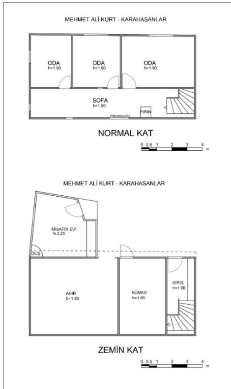
Resim 3.46. Mehmet Ali Kurt evi planları
