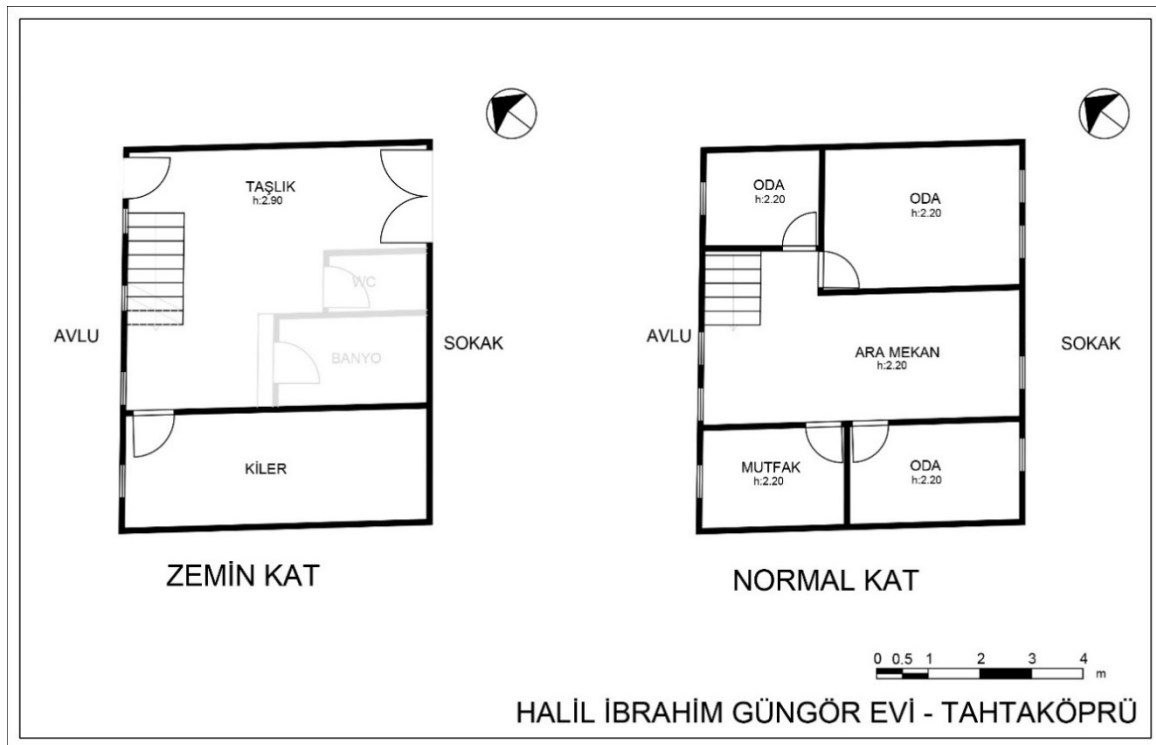
Resim 4.59. Halil İbrahim Güngör evi kat planları
