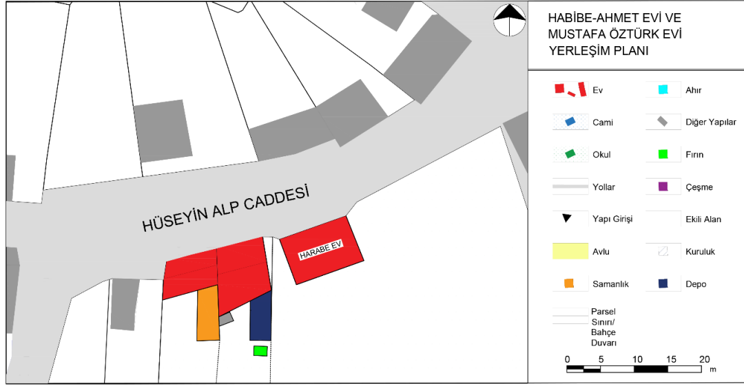
Resim 4.11. Ahmet-Habibe Öztürk ve Mustafa Öztürk evi yerleşim planı
