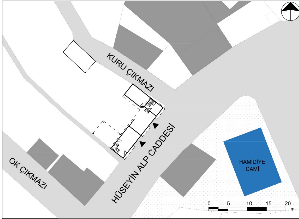
Resim 4.30. Meryem Aksoy evi yerleşim planı
