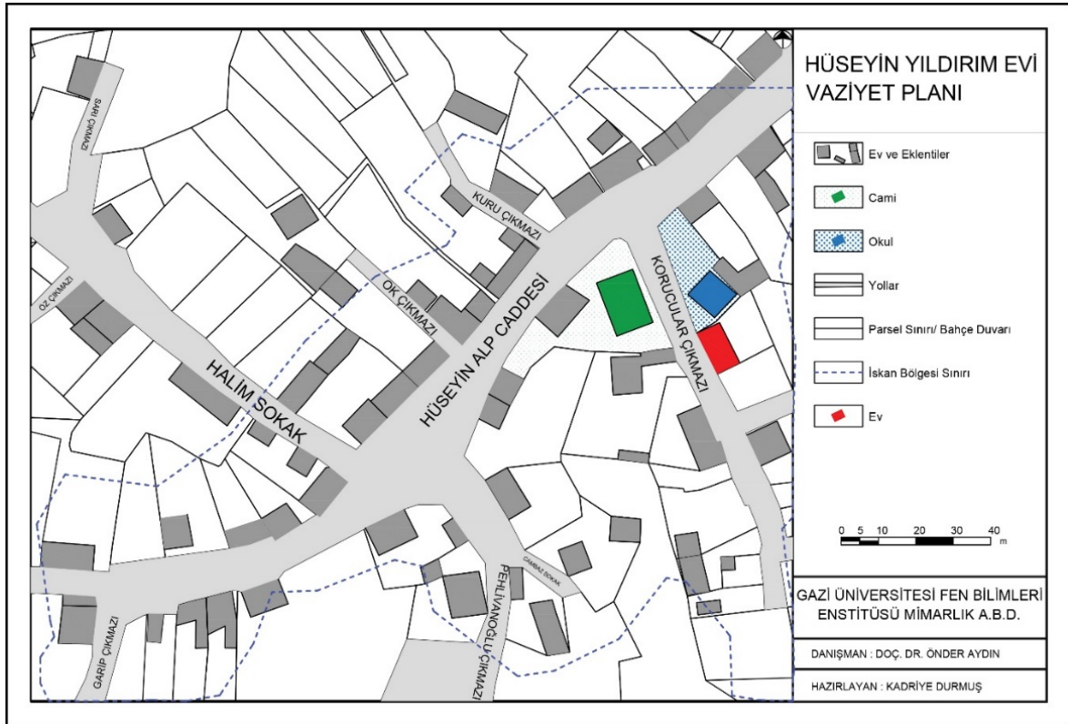
Resim 4.78. Hüseyin Yıldırım evi vaziyet planı
