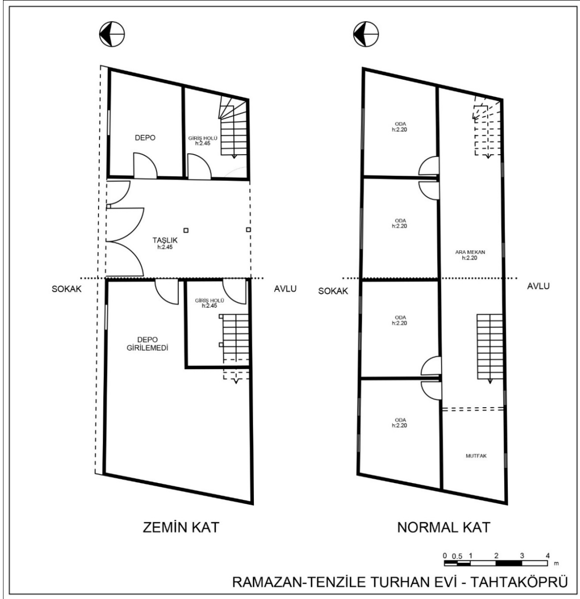
Resim 4.102. Ramazan-Tenzile Turhan evi kat planları
