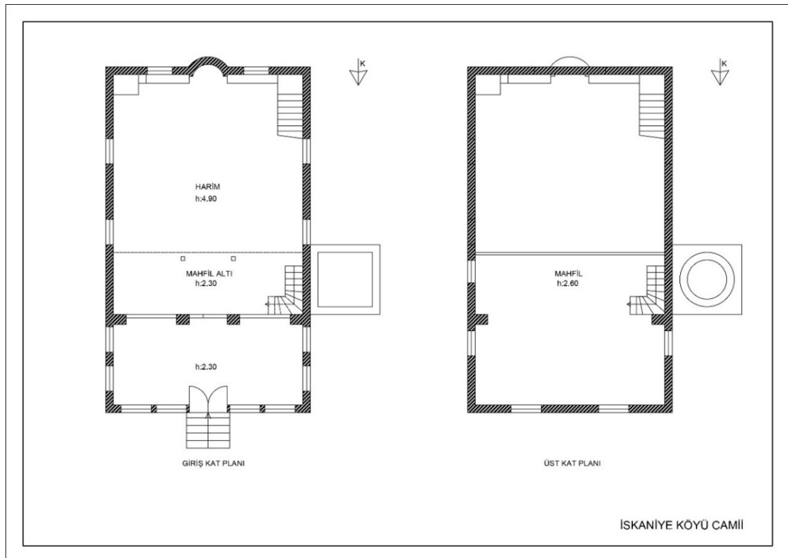
Resim 3.92. İskaniye Köyü Camisi planları
