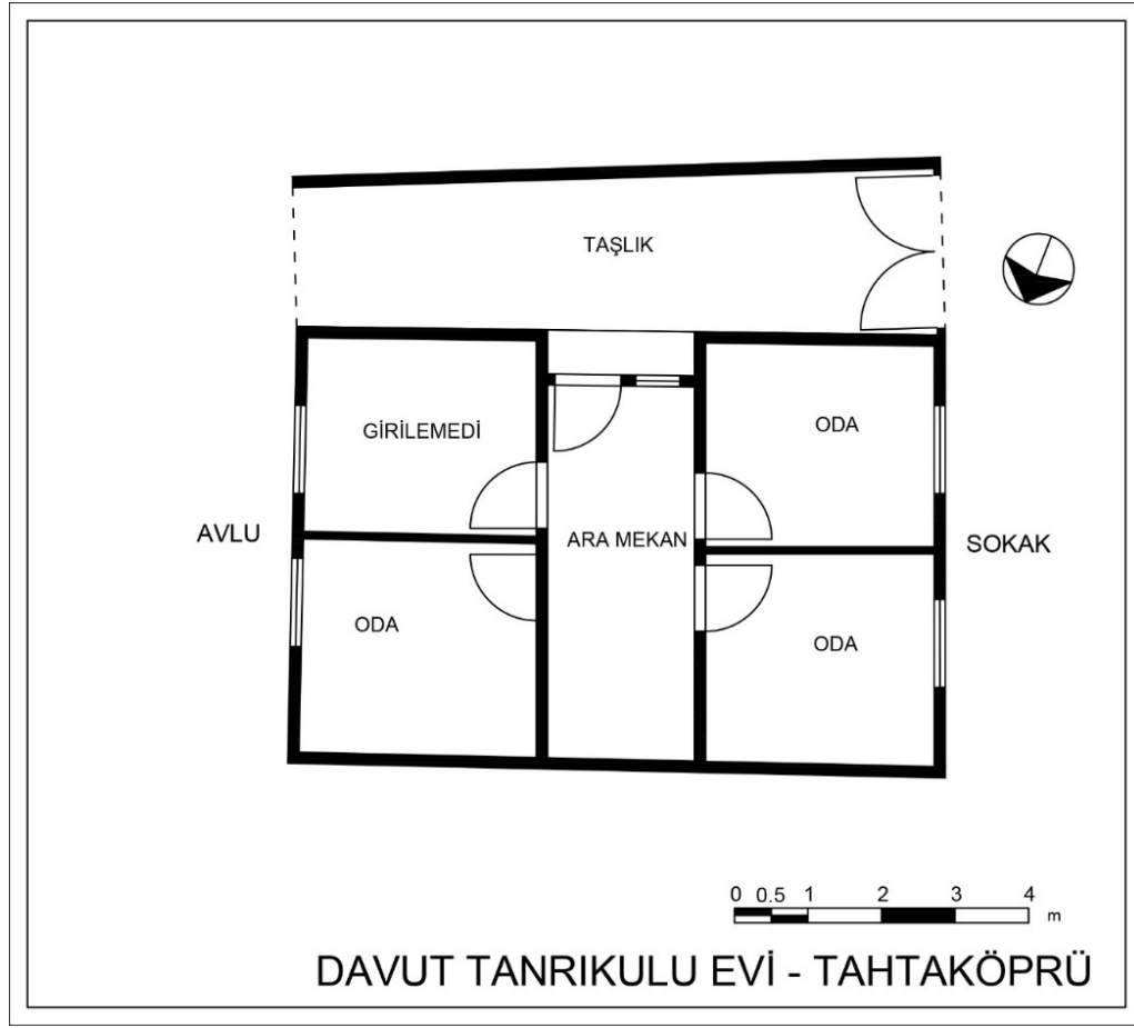
Resim 4.96. Davut Tanrikulu evi planı
