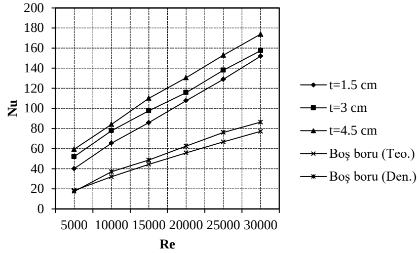
a) 3 adet türbülátör bulunması durumunda
