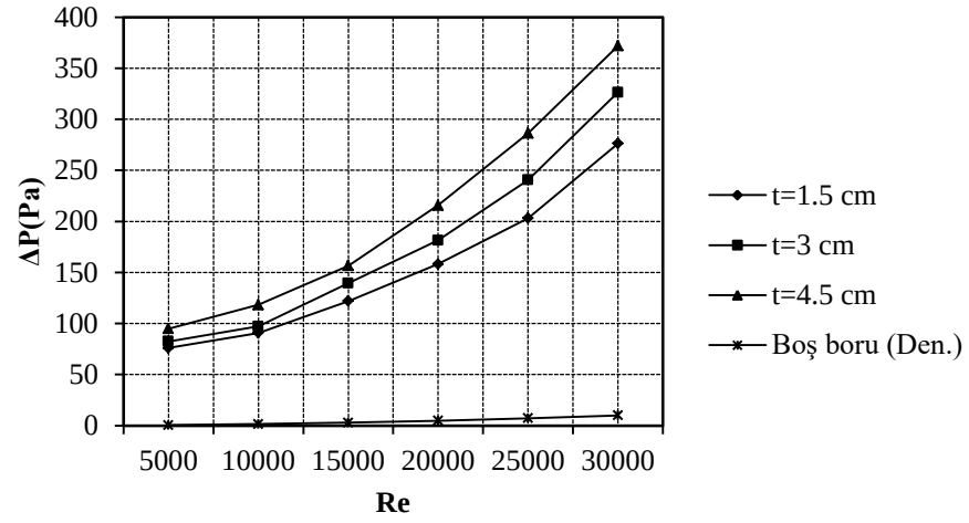
a) 3 adet türbülátör bulunması durumunda
