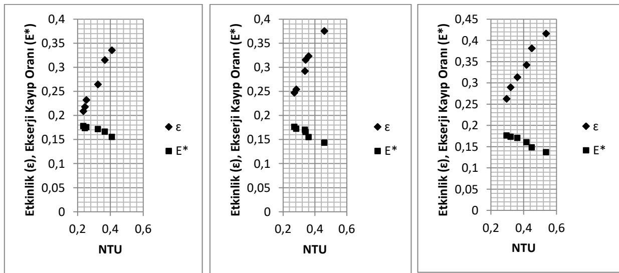
Şekil 4.12. Sonda 3 adet türbülötör bulunması durumunda Etkinlik, Ekserji Kayıp Oranı - NTU değişimi
