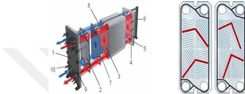
Şekil 1.8. Plakalı ısı değiştiricisinin şematik yapısı ve plaka üzerindeki balık sırtı yapısı (Karaali, 2009)
