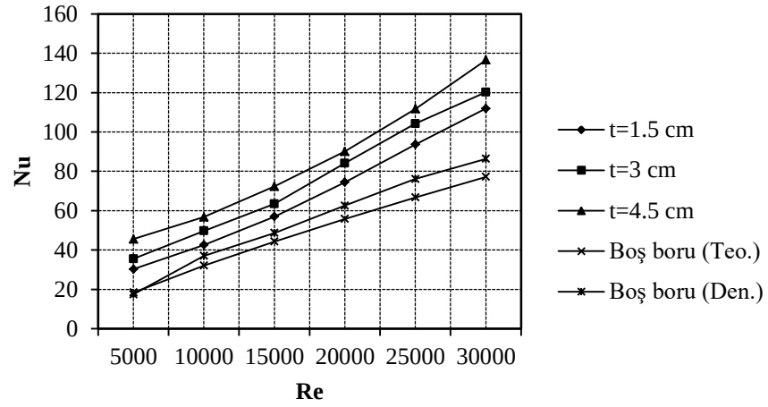
a) 3 adet türbülátör bulunması durumunda
