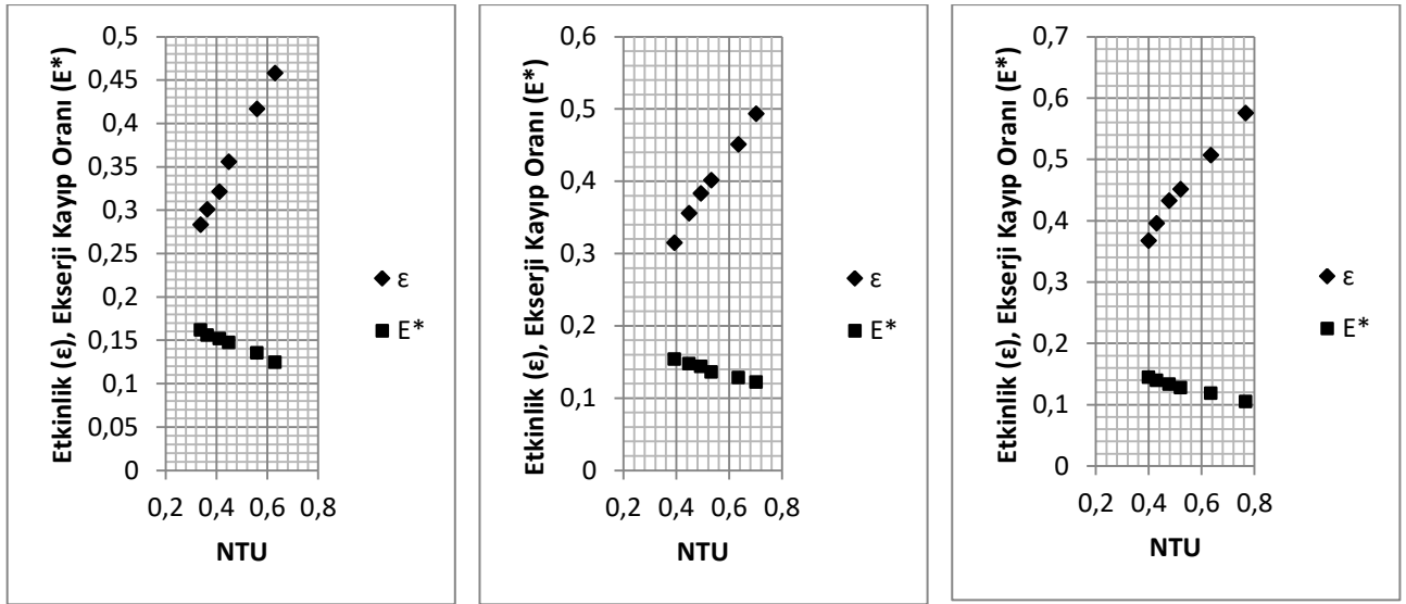
a) t = 1.5 cm aralıkta b) t = 3 cm aralıkta c) t = 4.5 cm aralıkta Şekil 4.16. Girişte 5 adet türbülötör bulunması durumunda Etkinlik, Ekserji Kayıp Oranı - NTU değişimi
