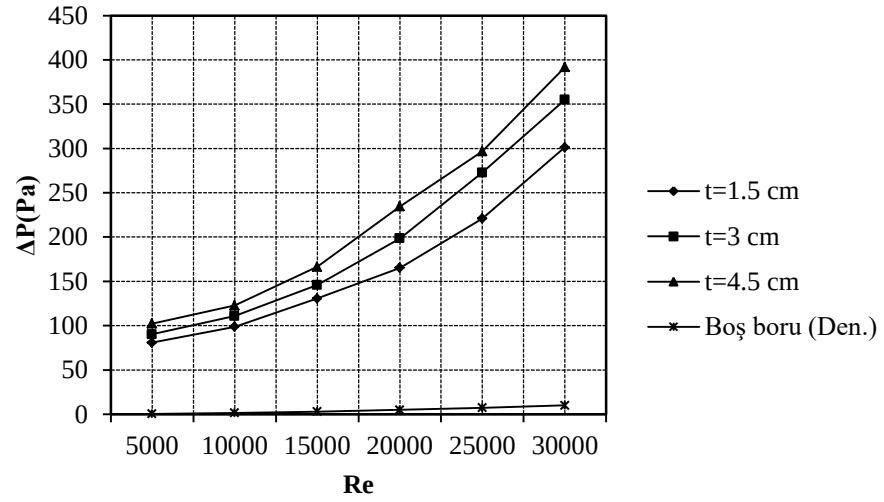
b) 4 adet türbülátör bulunması durumunda
