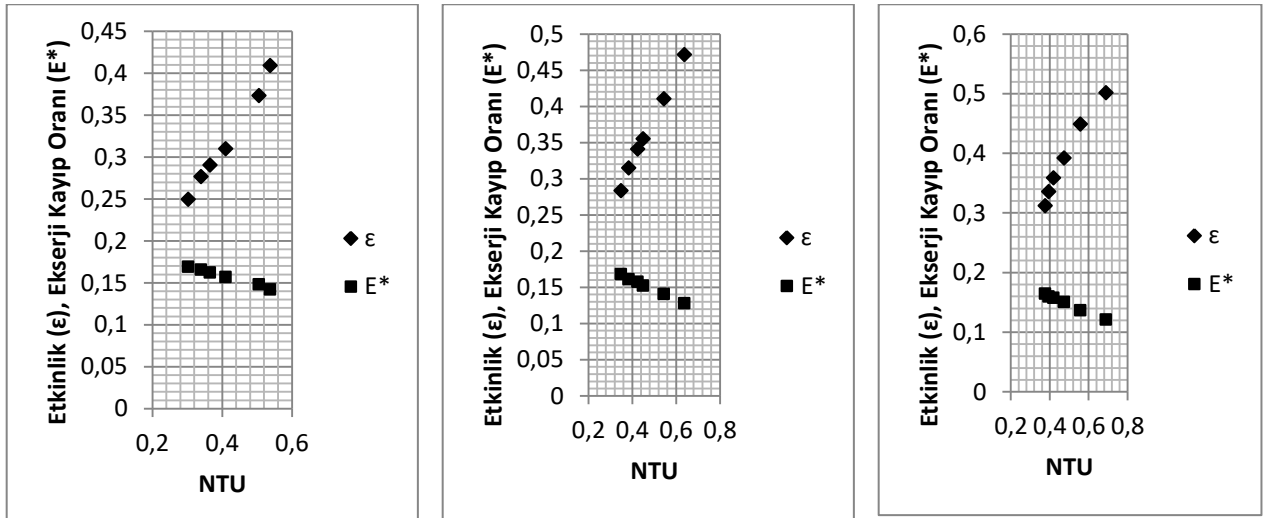
a) t = 1.5 cm aralıkta b) t = 3 cm aralıkta c) t = 4.5 cm aralıkta Şekil 4.18. Sonda 5 adet türbülötör bulunması durumunda Etkinlik, Ekserji Kayıp Oranı - NTU değişimi
