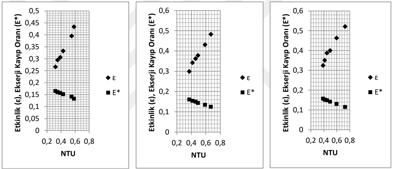
a) t = 1.5 cm aralıkta b) t = 3 cm aralıkta c) t = 4.5 cm aralıkta Şekil 4.17. Ortada 5 adet türbülötör bulunması durumunda Etkinlik, Ekserji Kayıp Oranı - NTU değişimi
