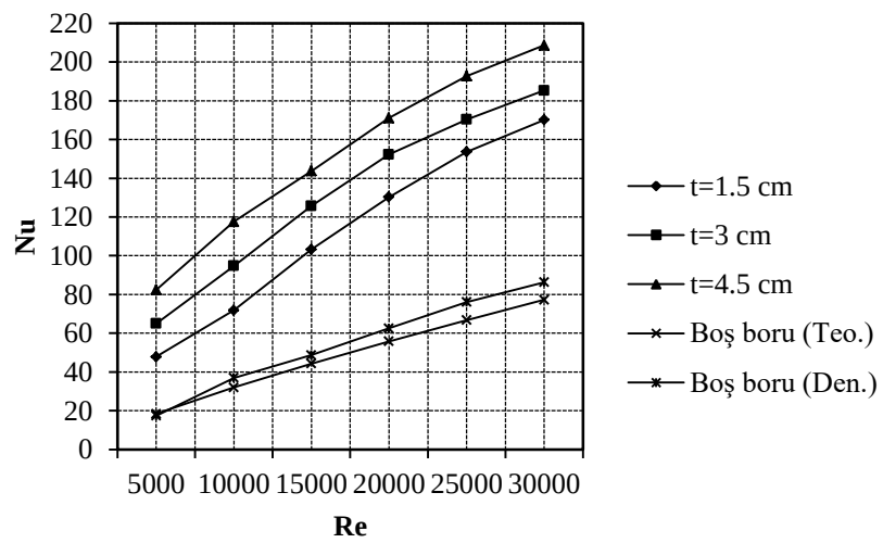
b) 4 adet türbülátör bulunması durumunda
