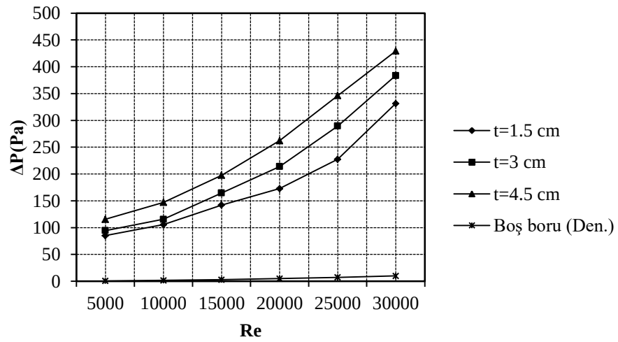
c) 5 adet türbülátör bulunması durumunda
