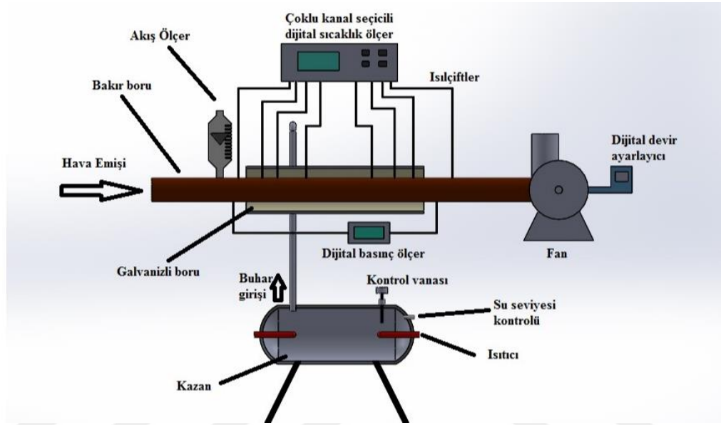
řekil 3.1. Deney düzeneđinin řematik grnř
