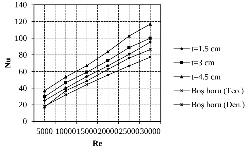
a) 3 adet türbülator bulunması durumunda
