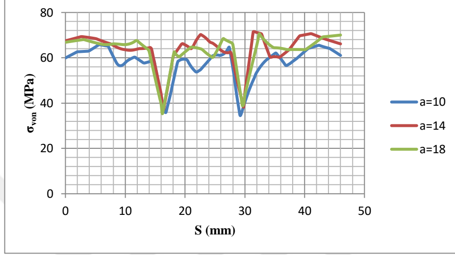
Şekil 5.54: Sekizgen dil tasarımlı tırnak genişliği b=2 mm için Yol 3 boyunca gerilme değerleri
