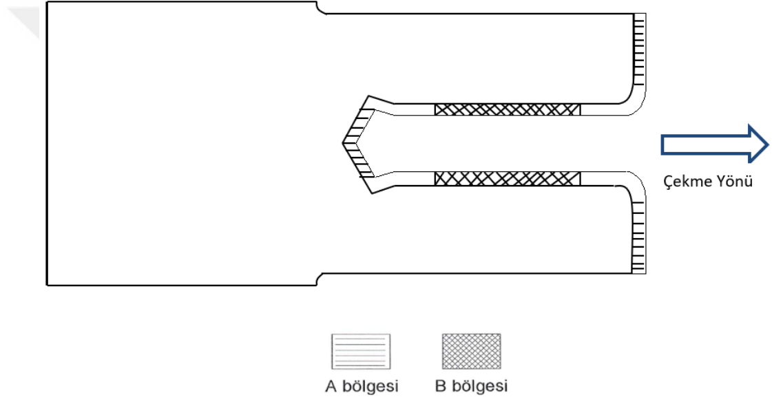
Şekil 4.14: Çekme gerilmesi sırasında oluşan deformasyon bölgeleri
