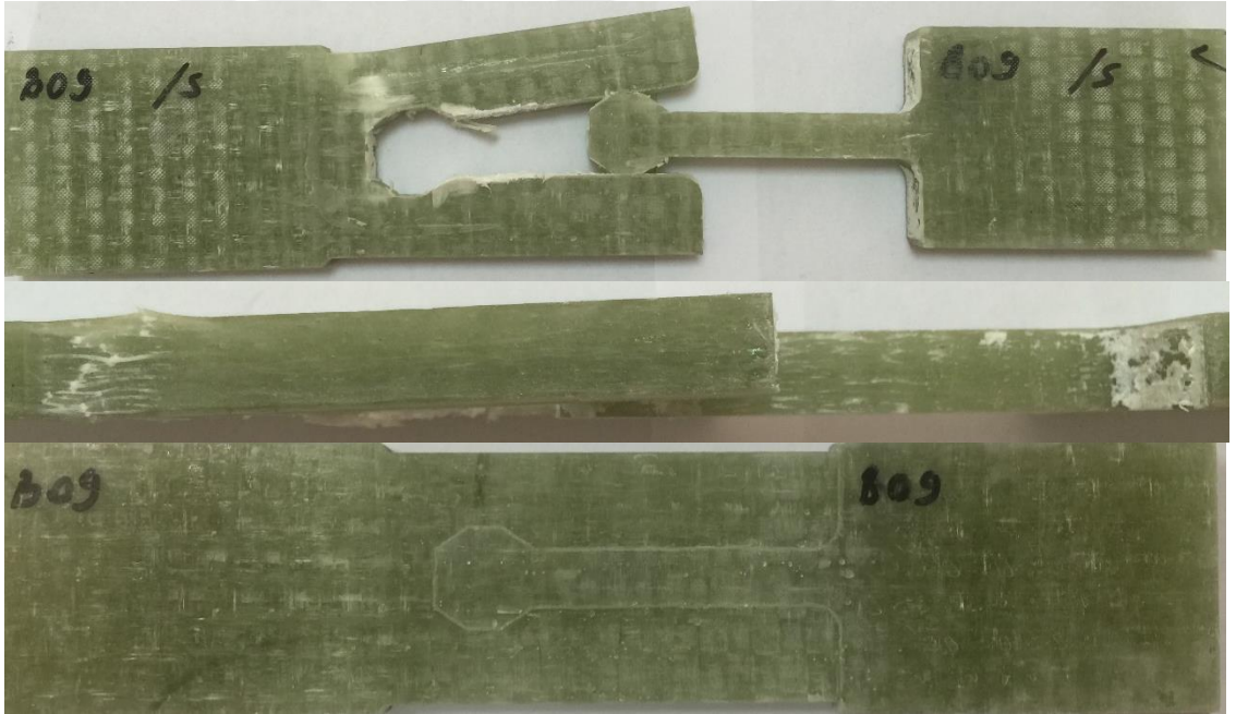
Şekil 4.43: Deney öncesi sekizgen dil tasarımı (B09 numunesi) ve deney sonrası oluşan deformasyonlar
