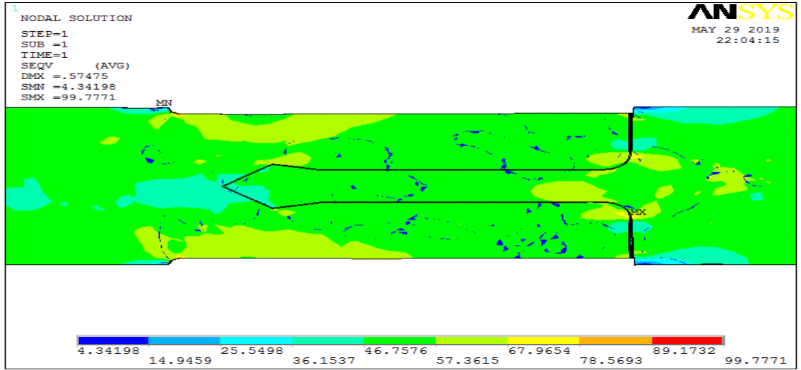
Şekil 5.23: Beşgen dil tasarımında tırnak uzunluğu 18 mm ve tırnak genişliği 2 mm (A08 numunesi) için von Mises gerilmesi
