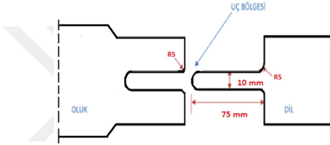
Şekil 4.1: Dil uç geometrisi oluşturulmayan tasarım
