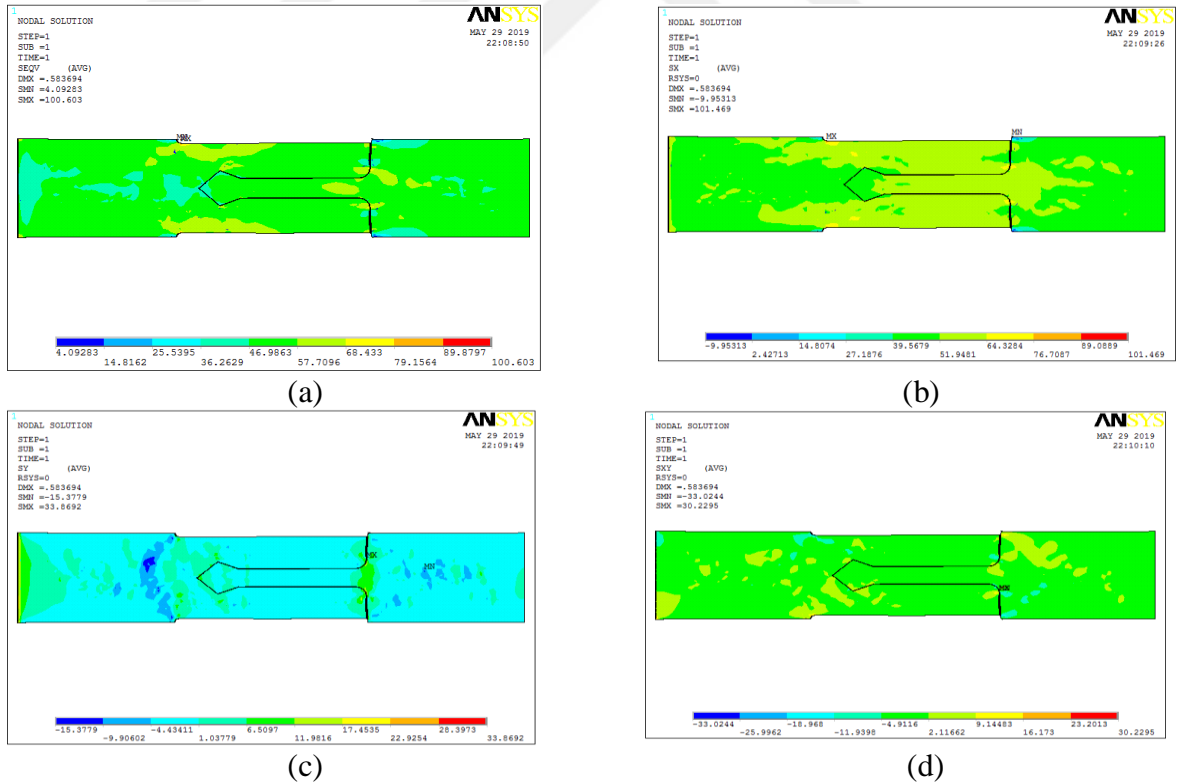
Şekil 5.26: Beşgen dil tasarımında a=18 mm ve b=4 mm için analiz sonuçları (a) von Mises ( \sigma_{von} ) (b) x eksenini boyunca ( \sigma_{xx} ) (c) y eksenini boyunca (açılma) ( \sigma_{yy} ) (d) kayma ( \tau_{xy} ) gerilmeleri
