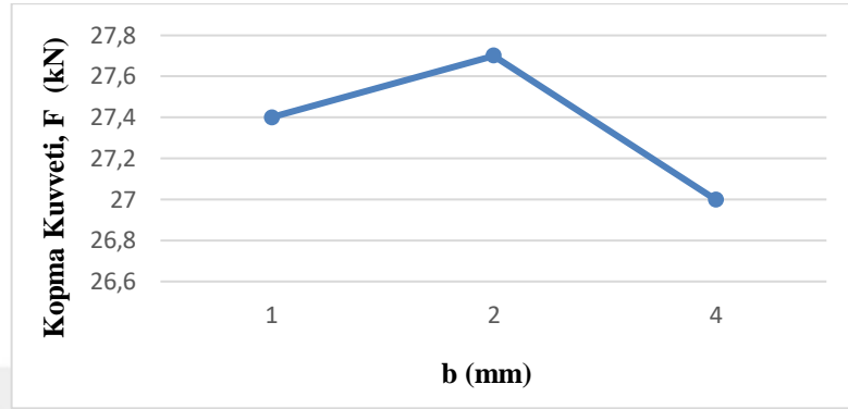
Şekil 4.36: Sekizgen dil tasarımında tırnak uzunluğu 10 mm için değişen tırnak genişliğinin kopma mukavemetine etkisi
