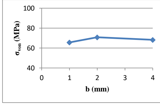
Şekil 5.63: Tırnak uzunluğu a=18 mm için von Mises sonuçları
