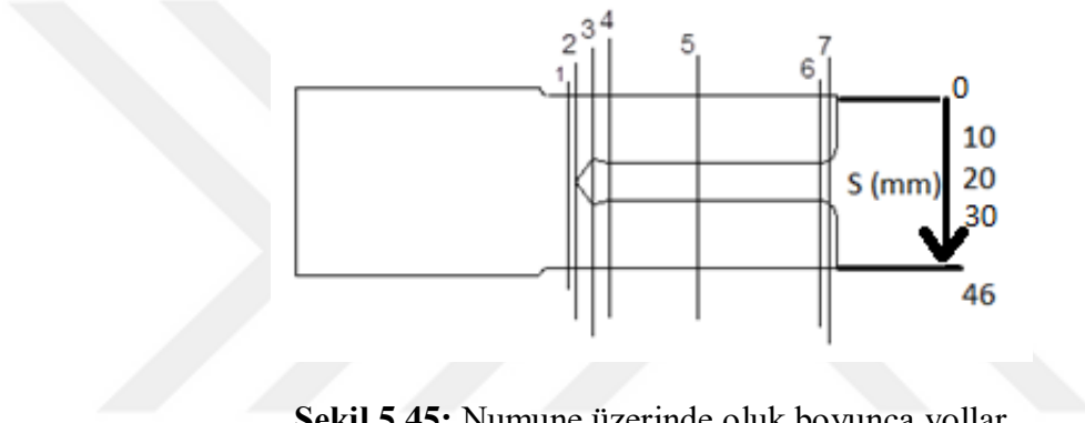
Şekil 5.45: Numune üzerinde oluk boyunca yollar
