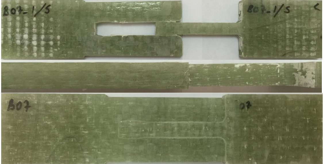
Şekil 4.41: Deney öncesi sekizgen dil tasarımı (B07 numunesi) ve deney sonrası oluşan deformasyonlar
