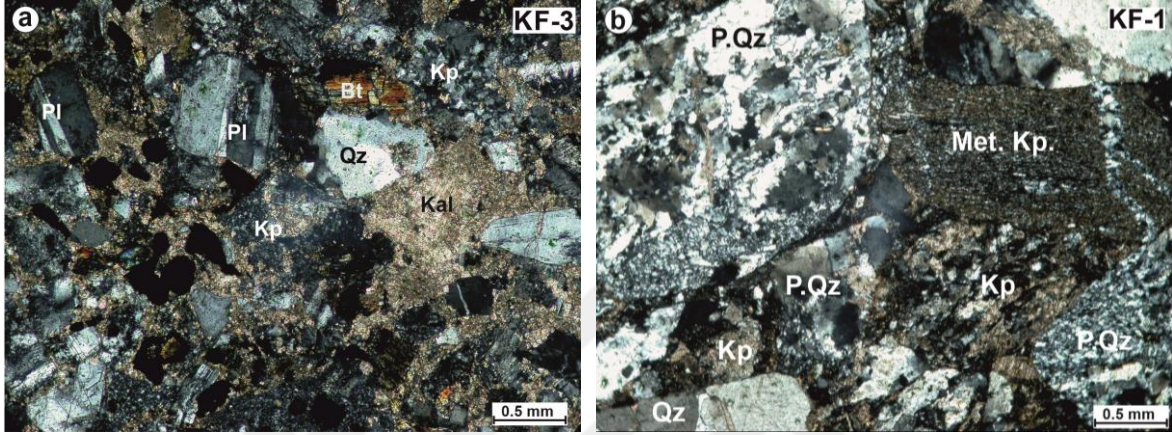
Şekil 3.10. Kelkit Formasyonu'ndan alınan ince taneli kumtaşı örneğinin mikroskobik görünümü. (a) Kuvars, polikristalin kuvars ve kayaç parçaları, (b) Polijen konglomerada bulunan metamorfik kayaç parçası ve polikristalin kuvarslar. Qz: kuvars, Pl: plajiyoklas, Bt biyotit, Kp: kayaç parçası, Kal: kalsit, P.Qz: polikristalin kuvars, Met.Kp.: metamorfik kayaç parçası.
