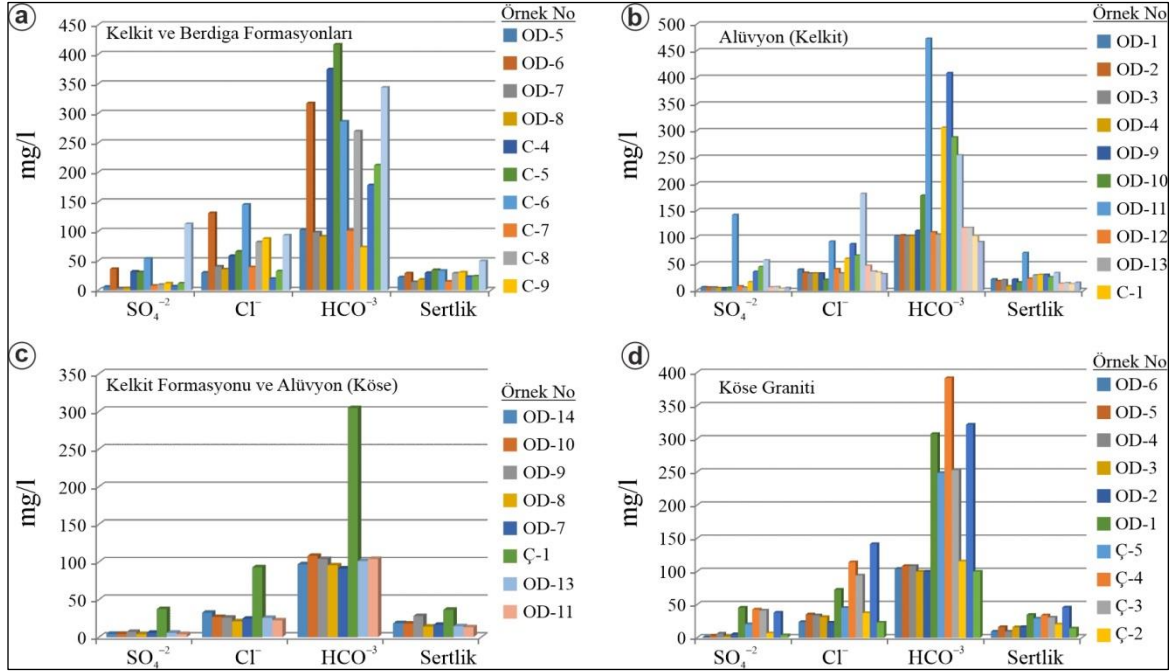
Şekil 4.1. Çalışma alanından lokasyon ve kayaç türlerine göre derlenen su numunelerinin \text{SO}_4^{2-} , \text{Cl}^- , \text{HCO}_3^- ve sertlik ( \text{Fr}^\circ ) parametrelerinin karşılaştırılmış dağılımı. (a) Kelkit ve Berdiga Formasyonlarından alınan örneklere ait parametreler. (b) Kelkit yerleşim merkezinde alüvyonlardan alınan örnekler. (c) Köse İlçe merkezinde Kelkit Formasyonu ve alüvyonlardan derlenen numuneler. (d) Köse yerleşim merkezinde Köse Granitinden derlenen numuneler.
