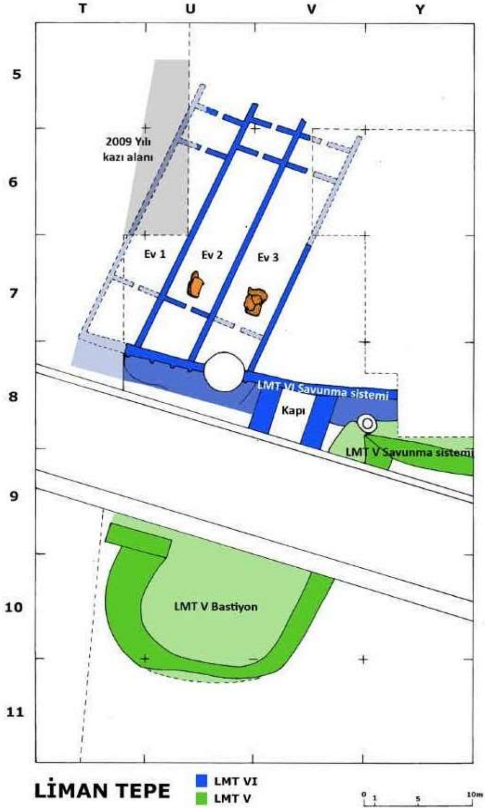
Resim 3. Limantepe V. ve VI. Tabakalara Ait Savunma Sistemi (Erkanal, Şahoğlu, Tuncel, Kouka, Keskin, Tuğcu 2008 yılı kara kazıları)
