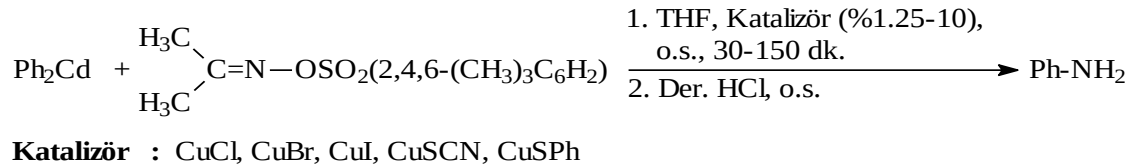
Şekil 1.2 Difenilkadmiyum reaktifinin Ia ile Cu(I) katalizli optimizasyon reaksiyonları
