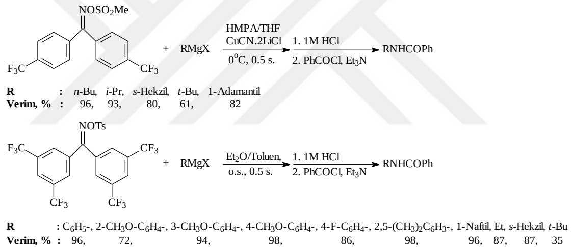
Şekil 2.3 4,4'-bis(triflormetil)benzofenon O -metilsülfoniloksim ve 3,3',5,5'-tetrakis(triflormetil)benzofenon O -tosiloksim reaktiflerinin Grignard reaktifleri ile aminasyon reaksiyonları
