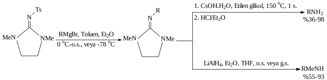
Şekil 2.6 2-imidazolidinonun O-sülfonil oksim ile Grignard reaktiflerinin aminasyonu
