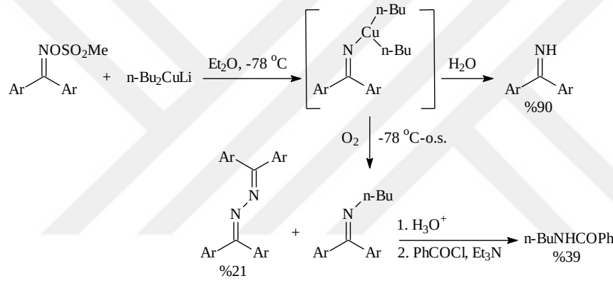
Şekil 2.10 Homokupratlarla ketoksimlerin elektrofilik aminasyonu
