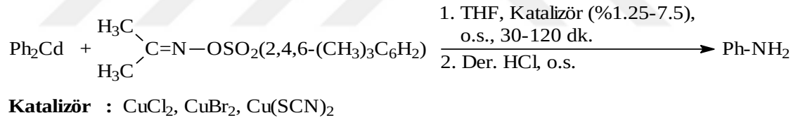
Şekil 1.4 Difenilkadmiyum reaktifinin Ia ile Cu(II) katalizli optimizasyon reaksiyonları
