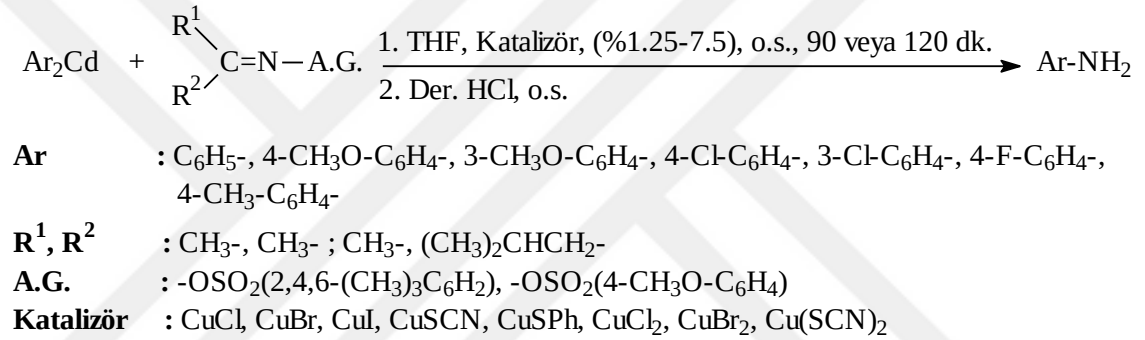
Şekil 5.5 Diarilkadmiyum reaktiflerinin ketoksimlerle Cu(I) ve Cu(II) katalizli elektrofilik aminasyonları
