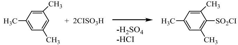
Şekil 3.6 Mesitilensülfonil klorürün hazırlanması
