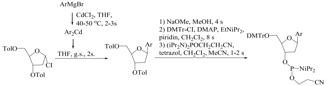
Şekil 2.18 DNA yapısındaki fosforamitlerin modifiye edilmesi
