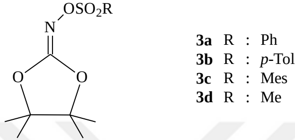
Şekil 2.7 1,3-dioksolan-2-on O -sülfonil oksim türevlerinin aminasyon reaktifleri
