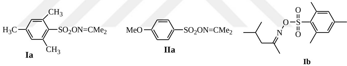
Şekil 5.3 Elektrofilik aminasyon reaksiyonunda, ketoksim yapısının aminasyon reaksiyonuna etkisinin incelenmesi amacıyla sentezlenen ketoksimler
