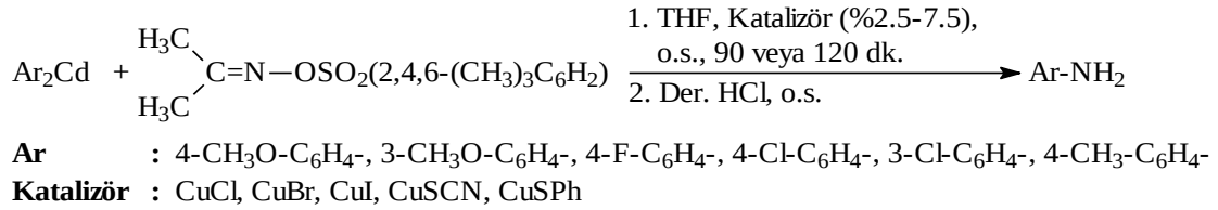
Şekil 1.3 Diarilkadmiyum reaktiflerinin Ia ile Cu(I) katalizli reaksiyonları
