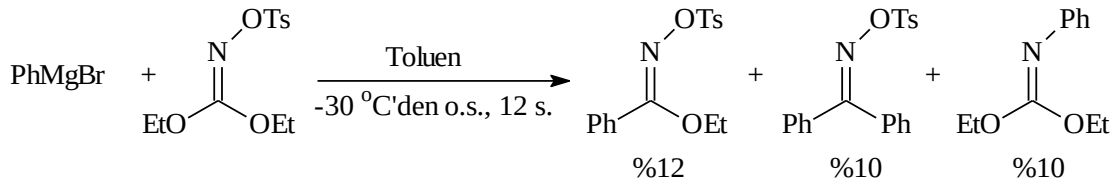
Şekil 2.4 Organomagnezyum reaktiflerinin, üre ve karbonatların O-sülfoniloksimleri ile elektrofilik aminasyonu
