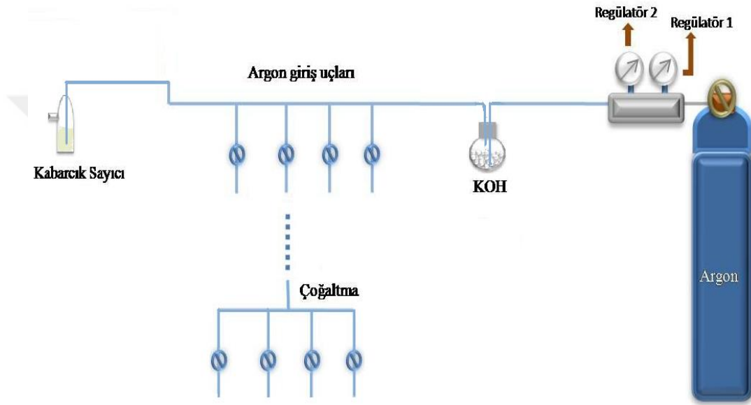
Şekil 3.1 İnert atmosfer düzeneği
