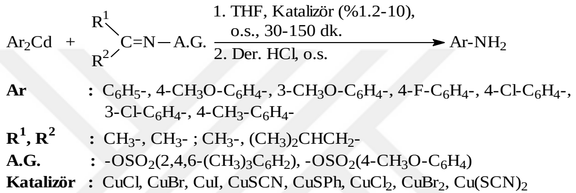
Şekil 1.1 Diarilkadmiyum reaktiflerinin ketoksimler ile Cu(I) ve Cu(II) katalizli elektrofilik aminasyon reaksiyonları
