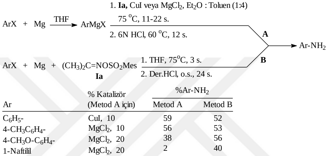
Şekil 2.1 Aseton O-(2,4,6-trimetilfenilsülfonil) oksim ile arilmagnezyumların aminasyon reaksiyonları
