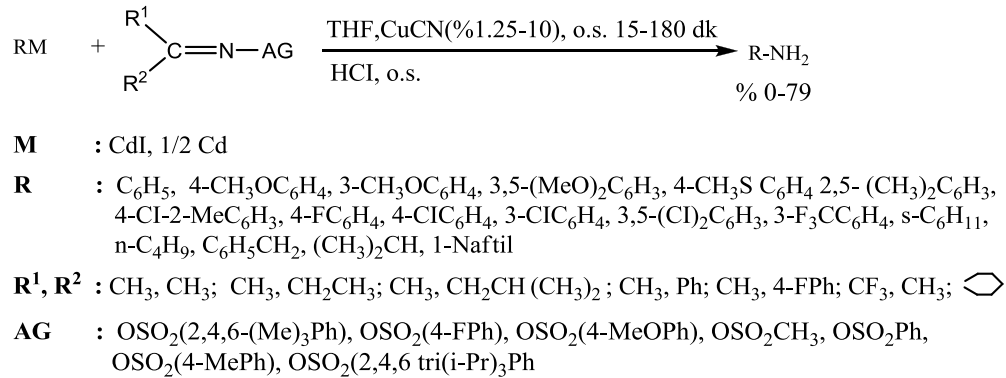
Şekil 2.19 Organokadmiyum reaktiflerinin ketoksimler ile elektrofilik aminasyon reaksiyonları
