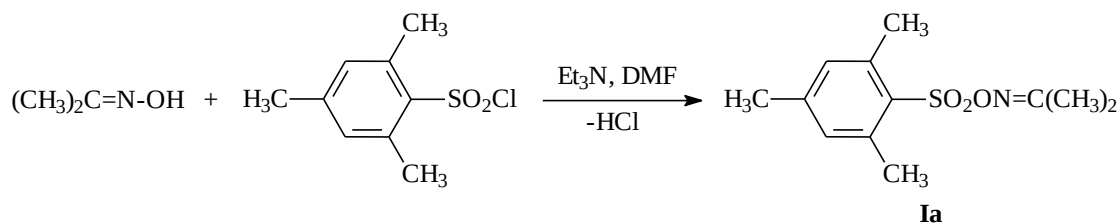
Şekil 3.7 Aseton O-(2,4,6-trimetilfenilsülfonil) oksim (Ia) sentezi
