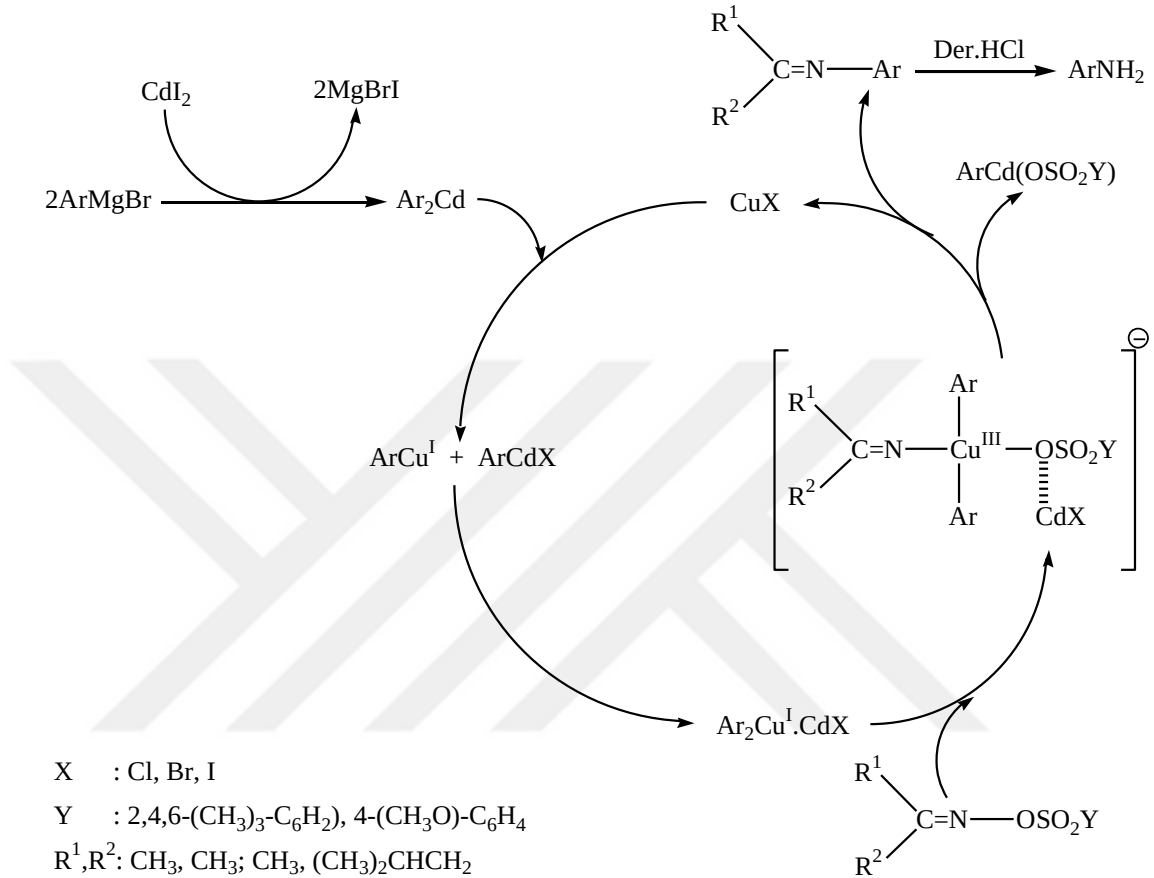
Şekil 5.1 Diarilkadmiyum bileşiklerinin ketoksinlerle Cu(I) ve Cu(II) katalizli homokuprat üzerinden gerçekleşen elektrofilik aminasyon reaksiyonu mekanizması
