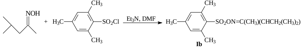
Şekil 3.10 4-metil-2-pentanon O-(2,4,6-trimetilfenilsülfonil) oksim (Ib) sentezi
