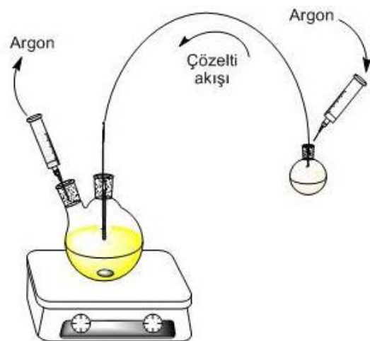
Şekil 3.3 İnert atmosferde çözelti aktarma düzeneği
