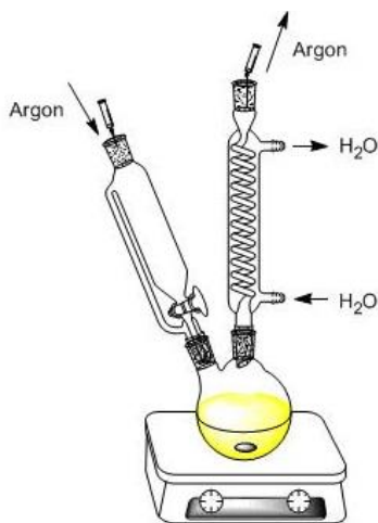
Şekil 3.2 İnert atmosferde reaksiyon düzeneği
