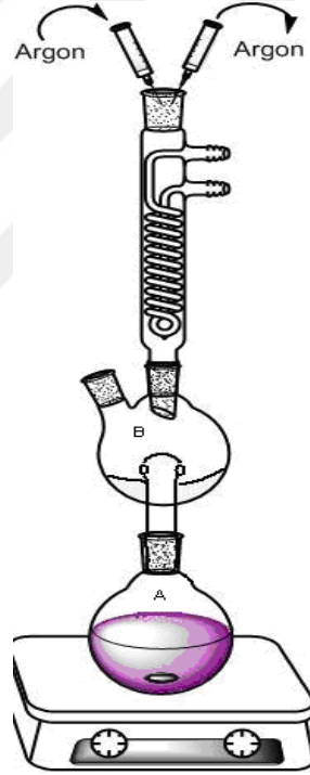
Şekil 3.4 Çözücü için inert atmosferde saflaştırma ve kurutma düzeneği
