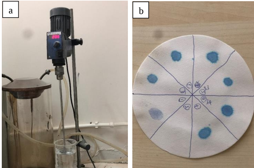
Şekil 3.7. Metilen mavisi deneyi; a) Metilen mavisi çözeltisi hazırlanması; b) Filtre kağıdında hale oluşumunun gözlenmesi
