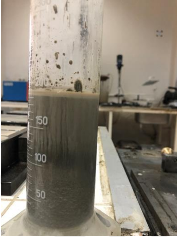
Şekil 3.15. Terleme yüzdesinin bulunması
