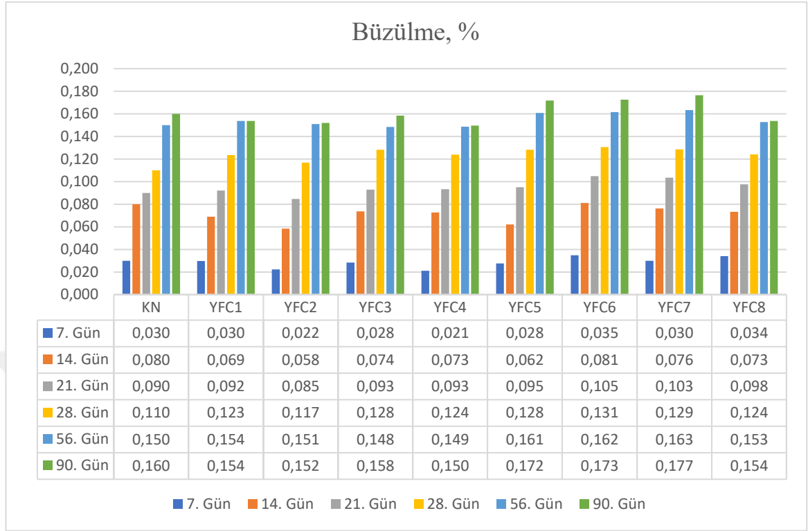
Şekil 4.4. YFC içerikli çimento harçlarının kuruma büzülmesi değerleri
