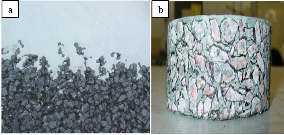
Şekil 1.1. a) Boşluklara nüfuz etme işlemi sırasında çimento harcı gözenekli asfalt iskelet b) yarı rijit kaplamasının karot numunesi
