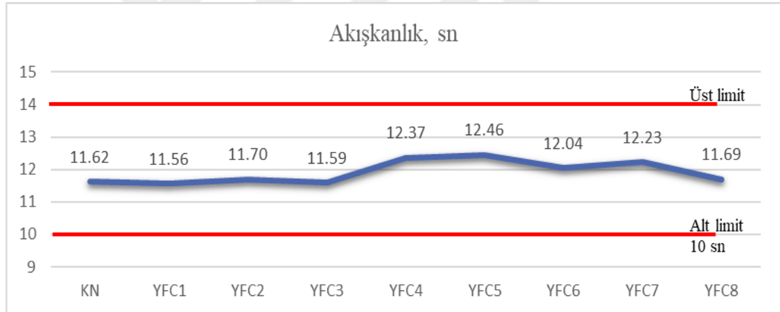
Şekil 4.1. YFC katkılı numunelerin akışkanlık sonuçları
