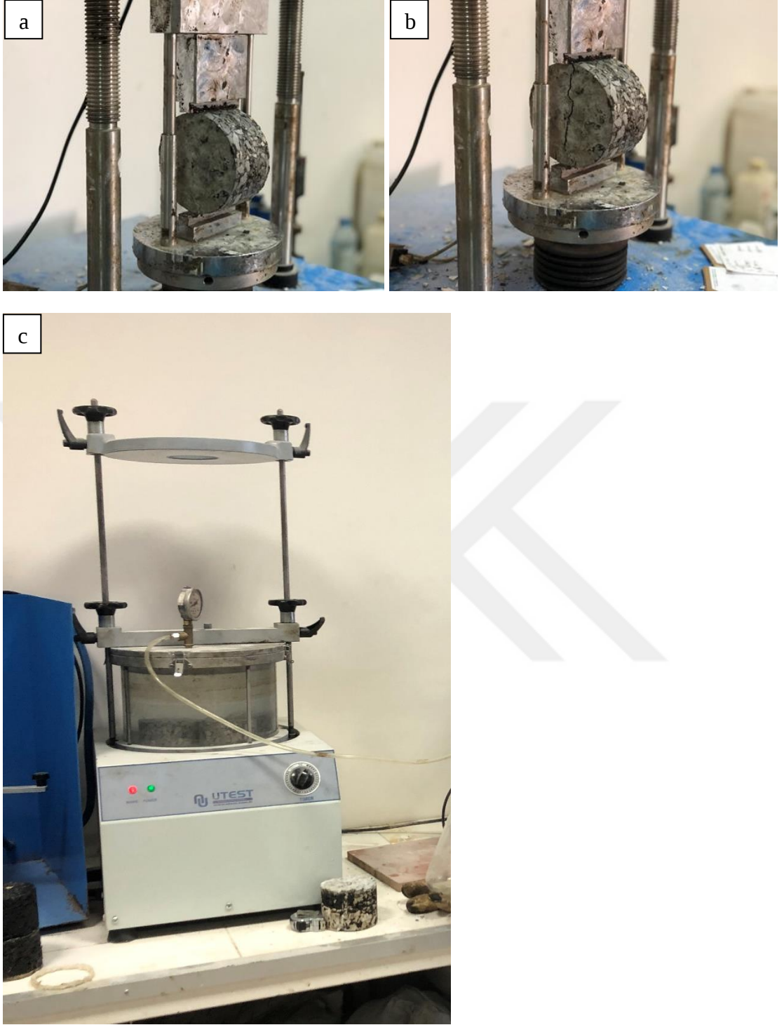
Şekil 3.23. Nem hasarına karşı direnç deneyi; a) Yük uygulanmadan önce; b) Yük uygulandıktan sonra; c) Vakumlu desikatörde numunenin su ile doyurulması
