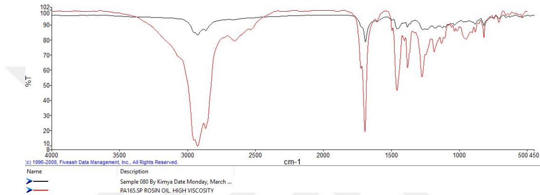
Fig. 27: KİSDA21/YB-235 envanter numaralı seramiğin FTIR sonucu 203 .
