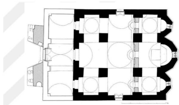
e. Pantanassa Athanasios Kilisesi (İ.S. 12. yy.)
