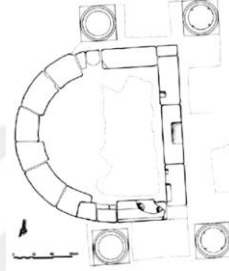
f. Banassara Güney Kilisesi Bema
