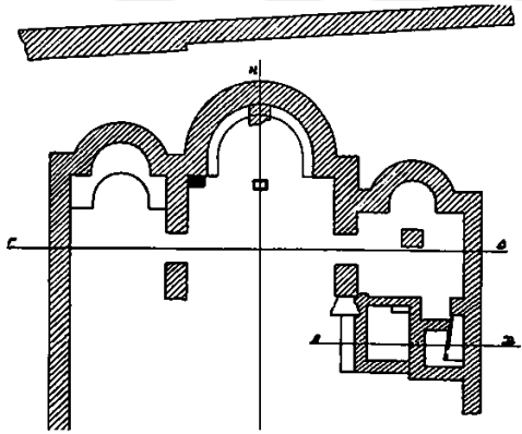
b. Selanik İkonaklast Kilisesi
