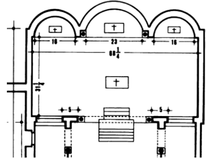
g. Montecassino San Benedetto Kilisesi (İ.S. 1066-1071)
