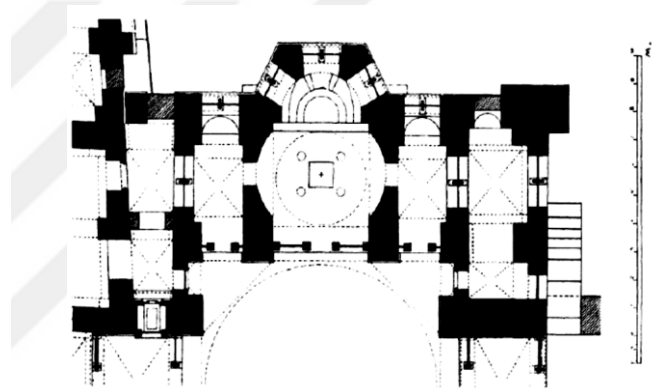
e. Hosios Loukas Kathedrali (İ.S. 956-970)
