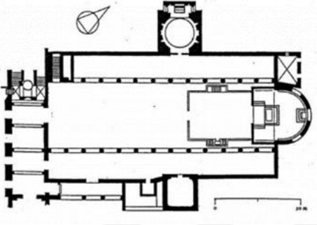
b. Roma Santa Sabina Bazilikası (İ.S. 422-432)
