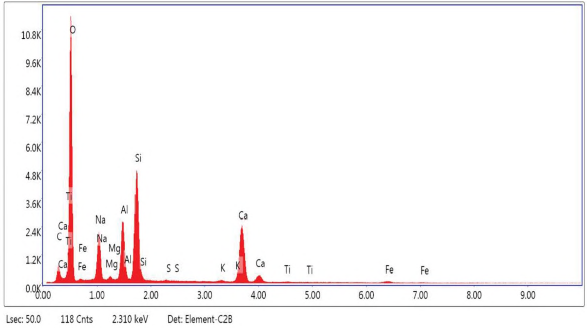
Şekil 4.15: %1,00 çelik lif içerikli numunenin EDS verileri
