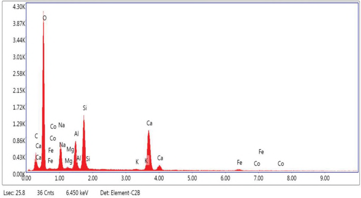
Şekil 4.17: %0,75 polipropilen lif içerikli numunenin EDS verileri
