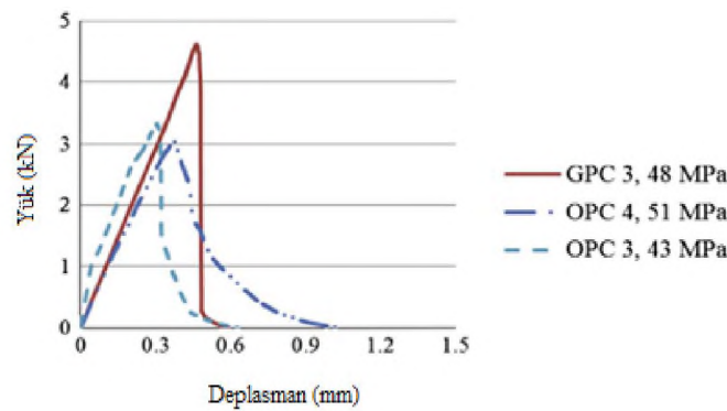
Şekil 2.11: Uçucu kül esaslı geopolimer beton (şekilde GPC) ve geleneksel Portland çimentolu betonun (şekilde OPC) yük-deplasman eğrisi altındaki davranış farkları [63].
