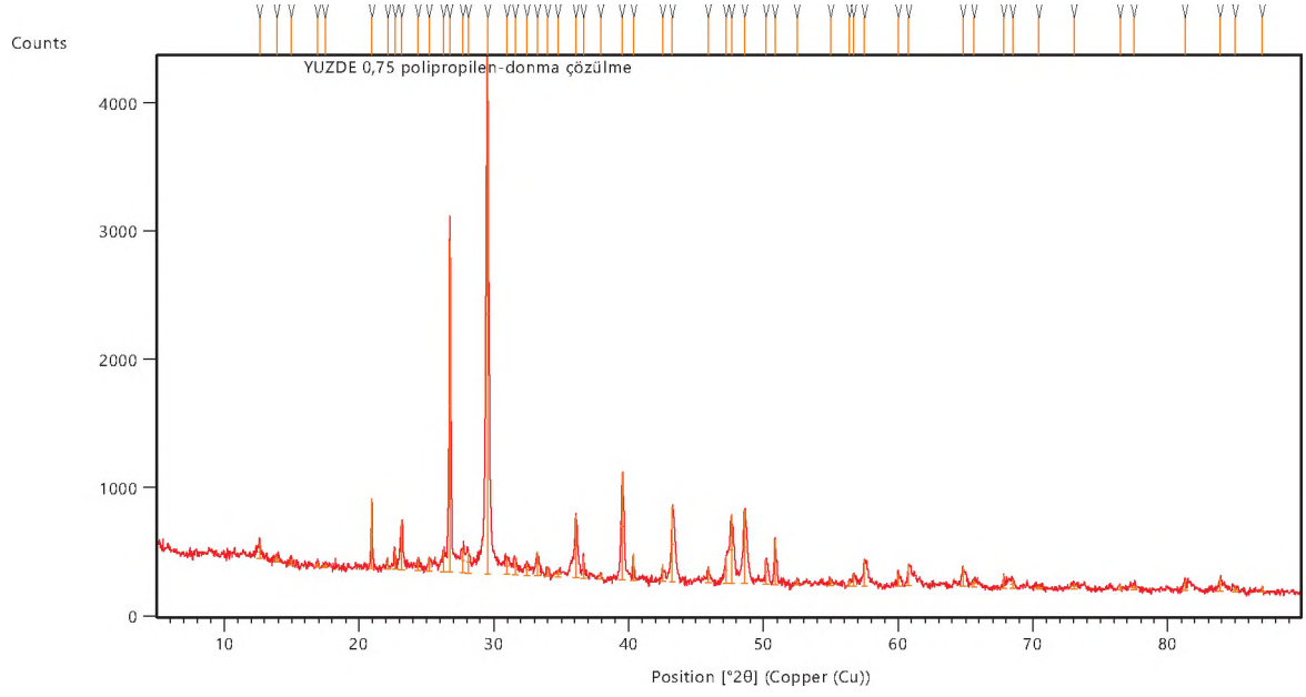
Şekil 4.28: Donma çözülme deneyi sonrası %0,75 polipropilen lif içerikli numunenin XRD grafiği
