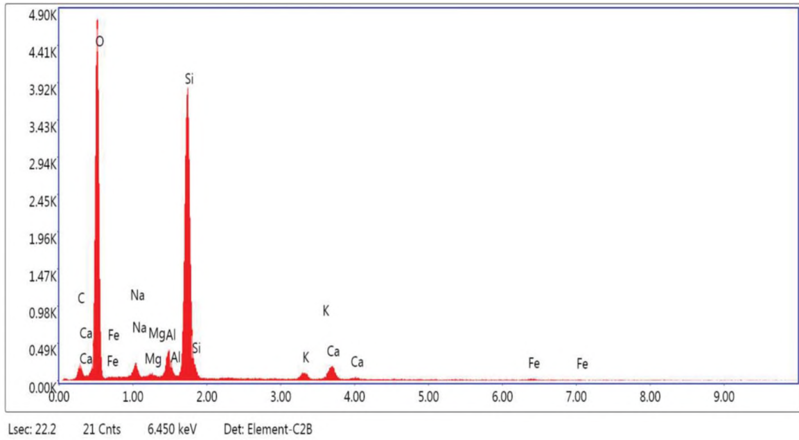
Şekil 4.16: %0,25 poliamid lif içerikli numunenin EDS verileri
