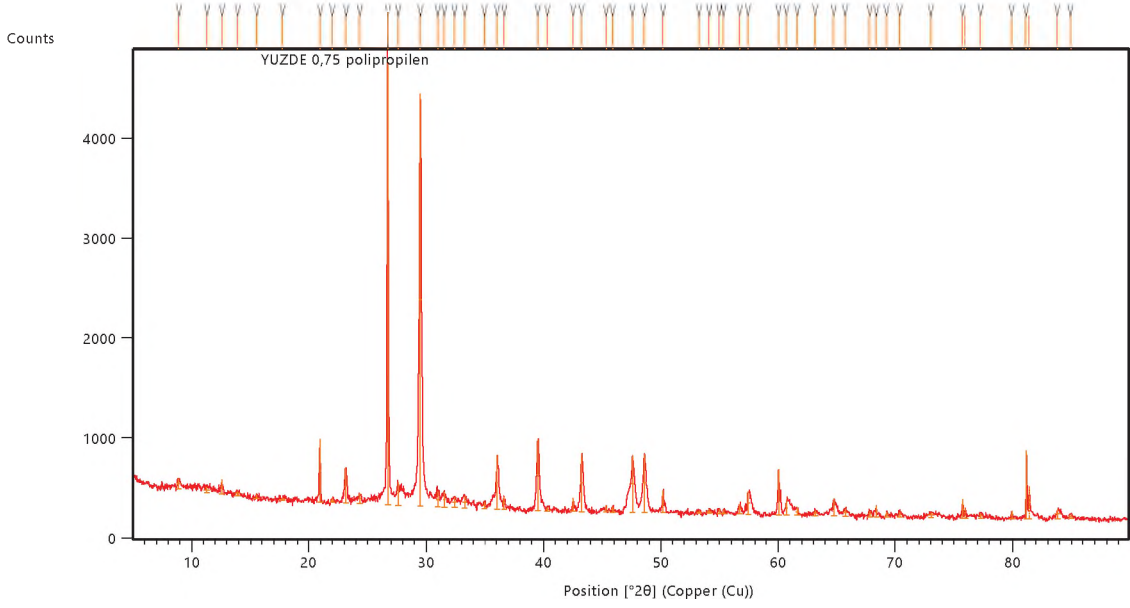
Şekil 4.11: %0,75 polipropilen lif içerikli numunenin XRD grafiği
