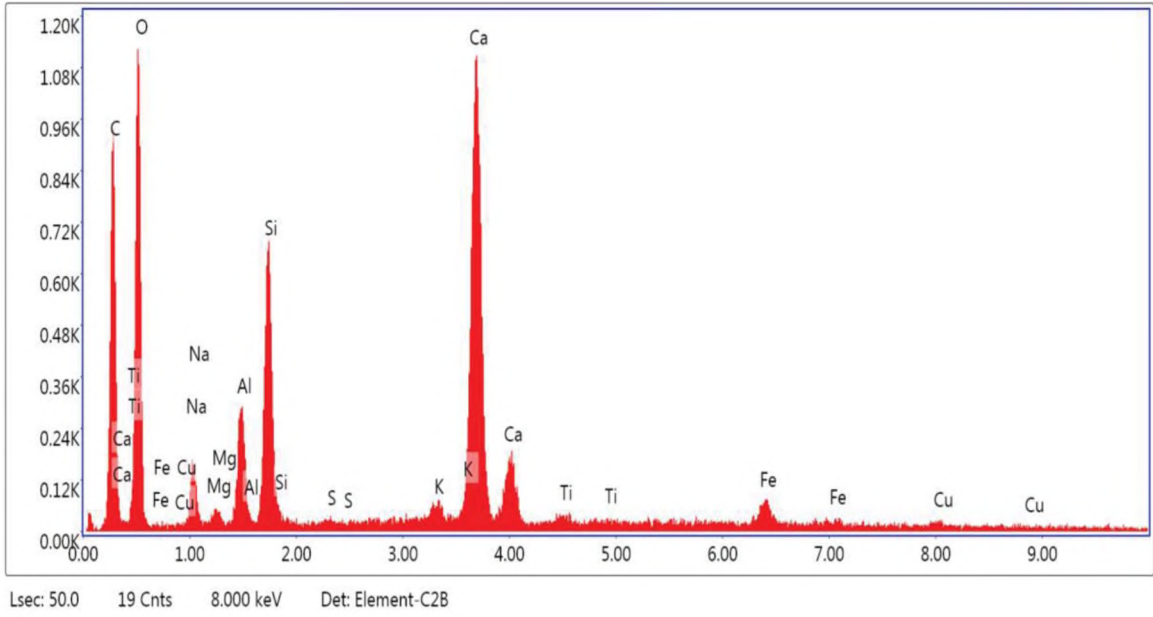
Şekil 4.34: Sodyum sülfat etkisi sonrası %1,00 polipropilen lif içerikli numunenin EDS verileri
