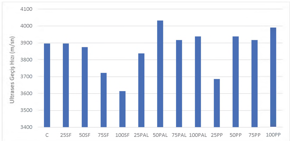
Şekil 4.6: Ultrases geiş hızları sonuçları
