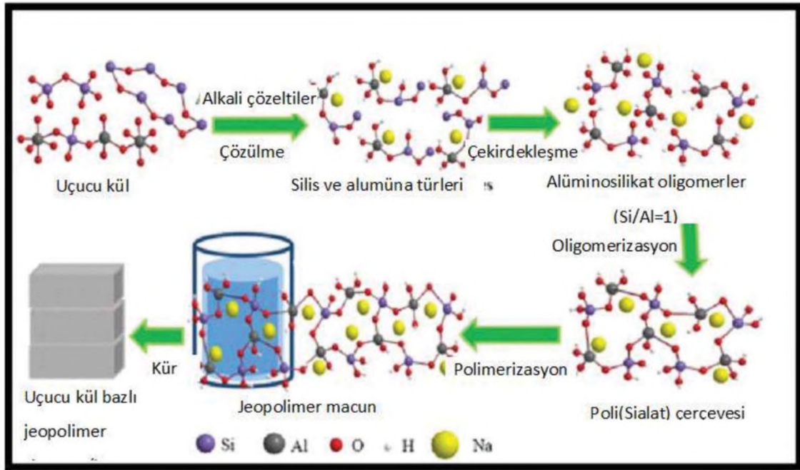
Şekil 2.2: Geopolimerizasyon süreci [15]
