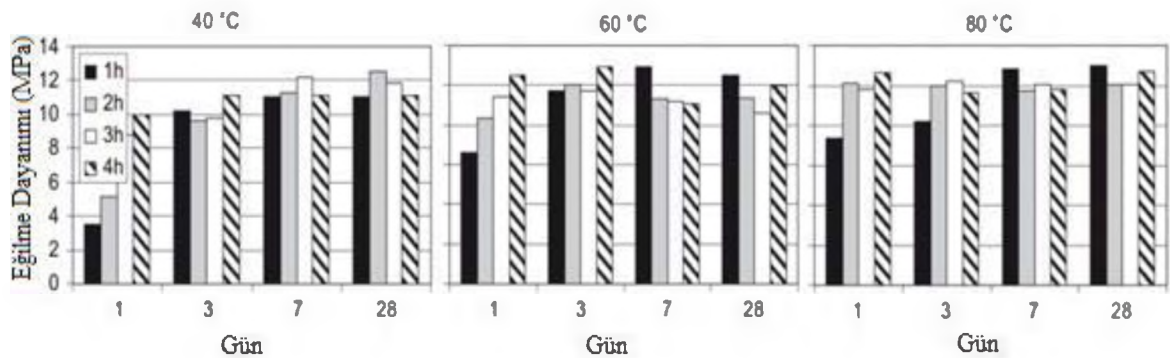
Şekil 2.12: Farklı kürlenme süreleri ve sıcaklıklarında kürlenmiş geopolimerlerin eğilme dayanımları [66]
