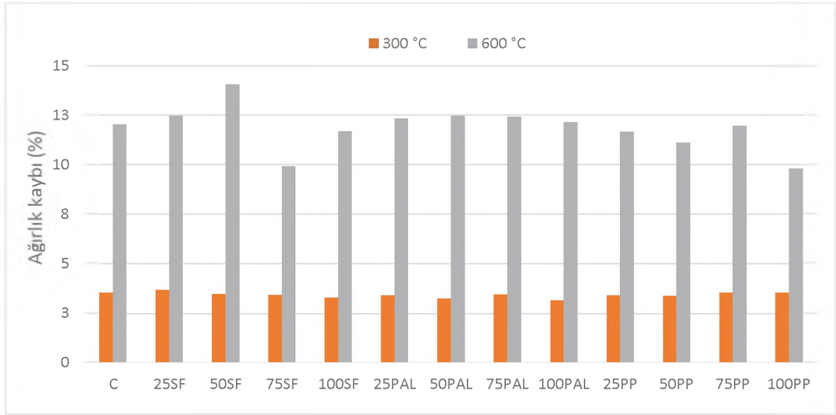
Şekil 4.21: Yüksek sıcaklık etkisindeki numunelerin ağırlık değişimi oranları
