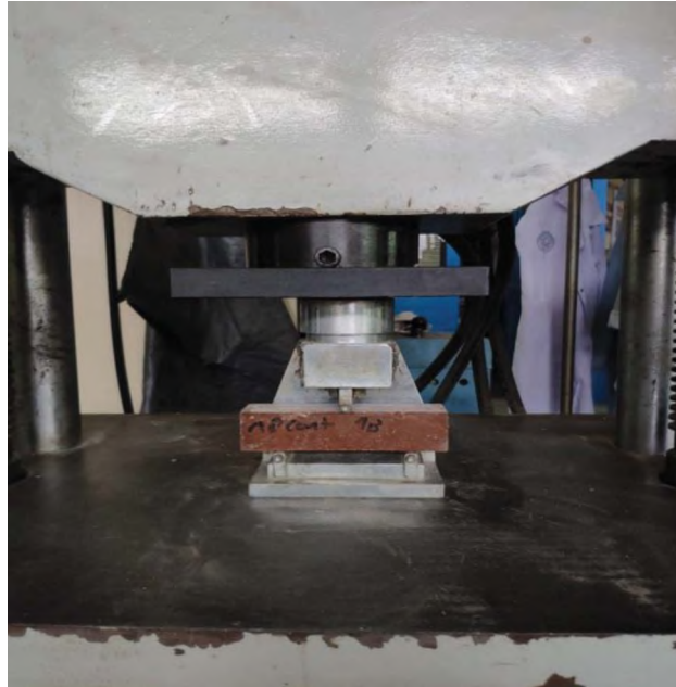
Şekil 3.5: Eğilme dayanımı deneyi
