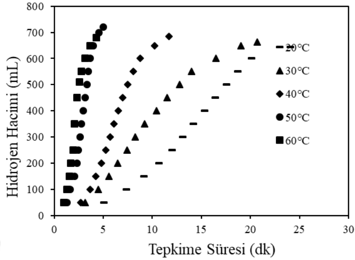
Şekil 6.17. CoO/MA katalizörü ile sodyum borhidrür hidrolizinde tepkime sıcaklığının hidrojen üretim hacmine etkisi (kalsinasyon sıcaklığı: 600°C, kalsinasyon süresi: 60 dk, sodyum hidroksit derişimi: %2,5, katalizör miktarı: 0,05 g, sodyum borhidrür derişimi: %2,5)
