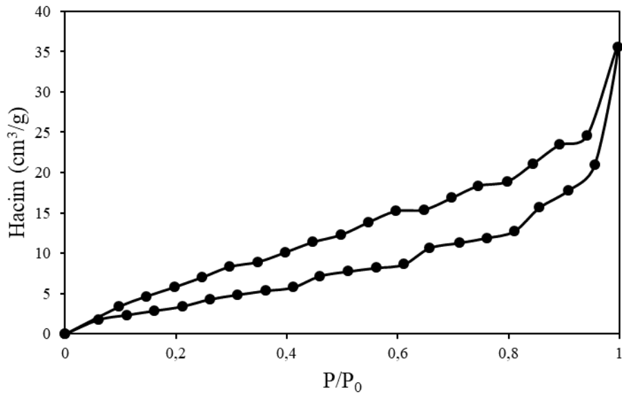
Şekil 6.32. %15 CoO/MA (500°C, 60 dk) katalizörünün azot adsorpsiyon-desorpsiyon izotermi
