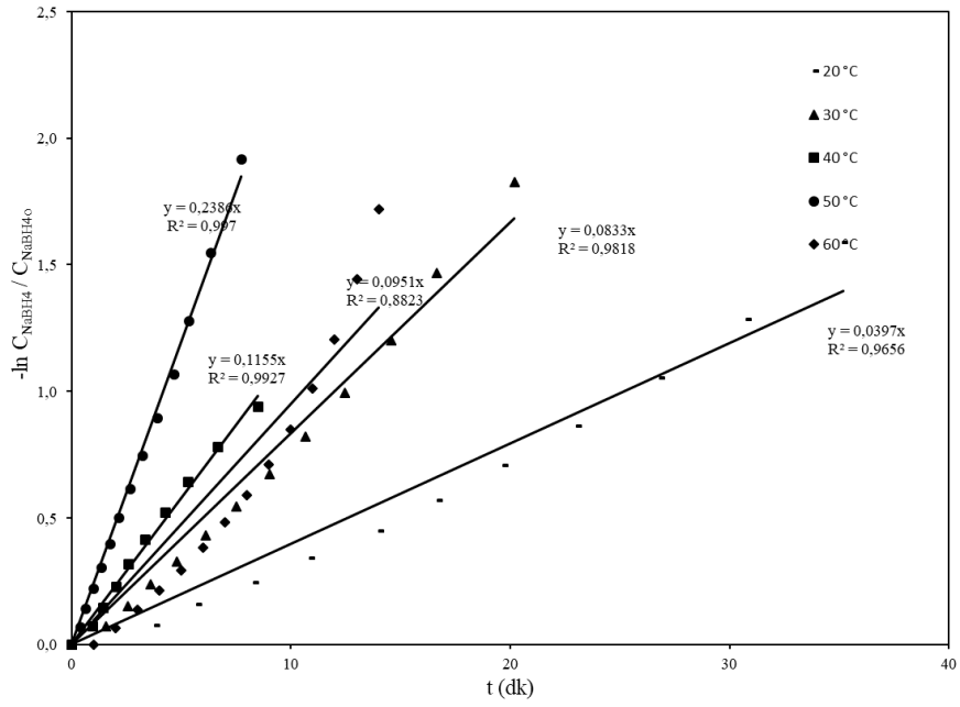
Şekil 6.8. CoB/MA katalizörünün birinci derece tepkime grafiği
