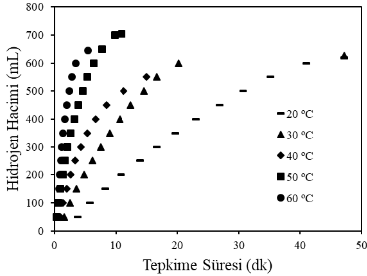
Şekil 6.6. CoB/MA katalizörü ile sodyum borhidrür hidrolizinde tepkime sıcaklığının hidrojen üretim hacmine etkisi (indirgeme oranı: 3:1 \text{BH}_4^-/\text{Co} , metal yükleme oranı: %15, sodyum hidroksit derişimi: %2,5, katalizör miktarı: 0,05 g, sodyum borhidrür derişimi: %2,5)
