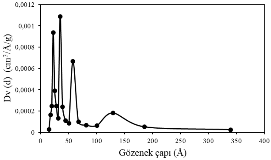
Şekil 6.33. %15 CoO/MA (500°C, 60 dk) katalizörünün gözenek boyut dağılımı
