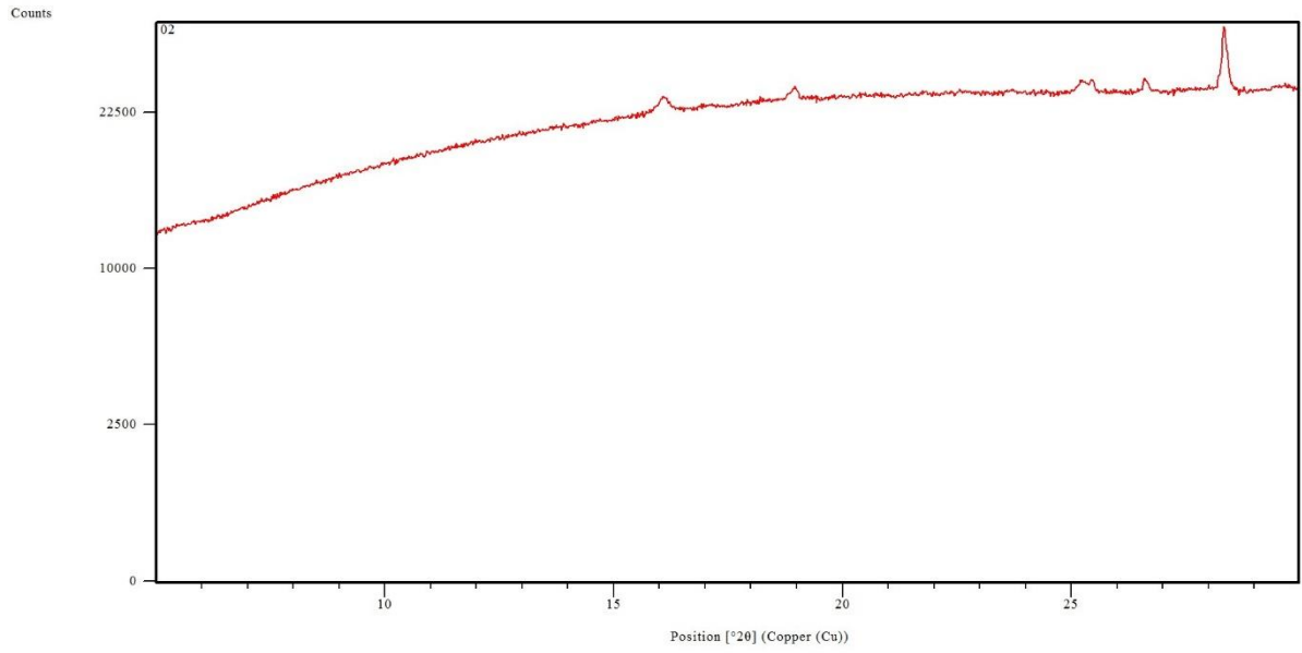
Şekil 6.26. %15 CoO / MA (600°C, 60 dk) katalizörünün XRD kırınım deseni
