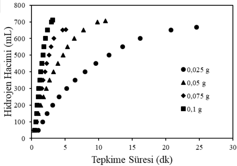
Şekil 6.4. CoB/MA katalizörü ile sodyum borhidrür hidrolizinde katalizör miktarının hidrojen üretim hacmine etkisi (indirgeme oranı: 3:1 BH 4 - /Co, metal yükleme oranı: %15, sodyum hidroksit derişimi: %2,5, sodyum borhidrür derişimi: %2,5, tepkime sıcaklığı: 50°C)
