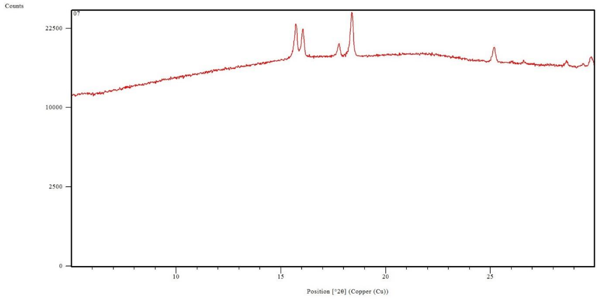
Şekil 6.24. %15 CoB / MA katalizörünün XRD kırınım deseni
