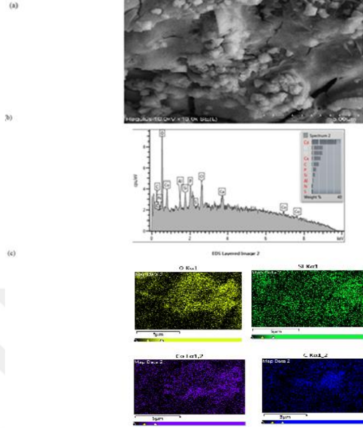
Şekil 6.42. %15 CoO/MA (600°C, 60 dk) katalizörünün a)SEM görüntüsü b) EDS sonucu c) elementel haritası
