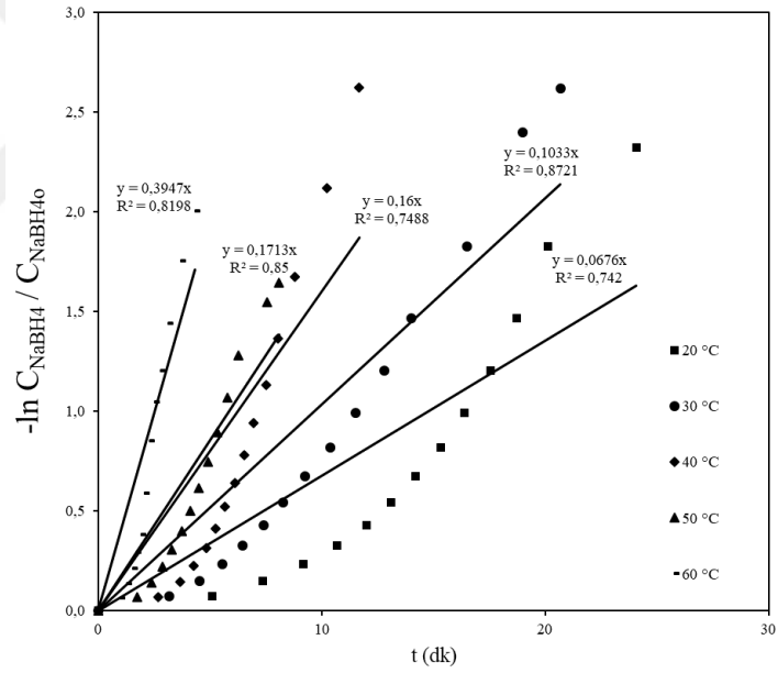
Şekil 6.19. CoO /MA katalizörünün birinci derece tepkime grafiği
