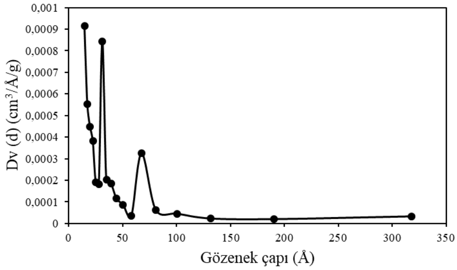
Şekil 6.35. %15 CoO/MA (600°C, 60 dk) katalizörünün gözenek boyut dağılımı
