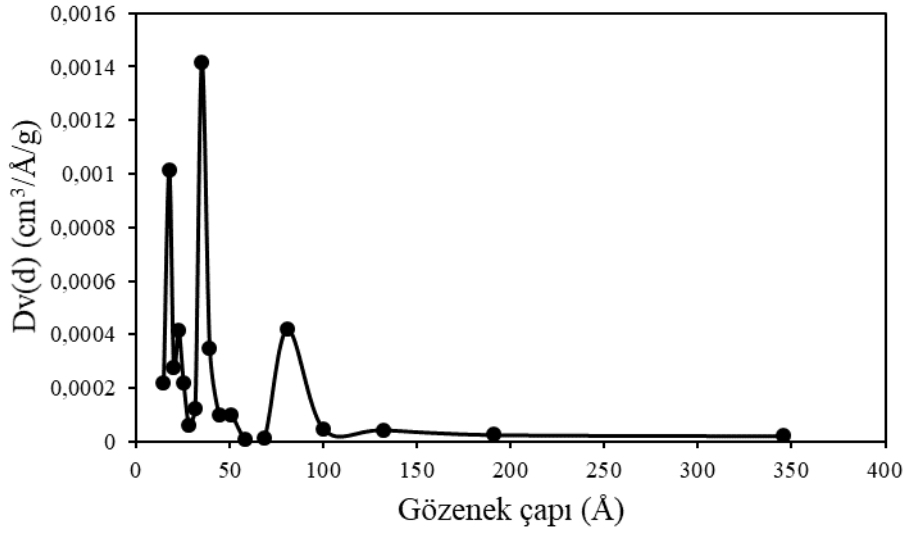
Şekil 6.37. %15 CoO/MA (700°C, 60 dk) katalizörünün gözenek boyut dağılımı
