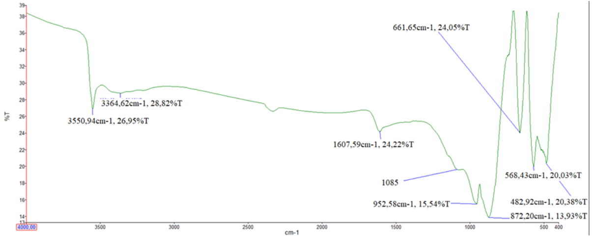
Şekil 6.51. %20 CoO/MA (600°C, 60 dk) katalizörünün FTIR spektrumu
