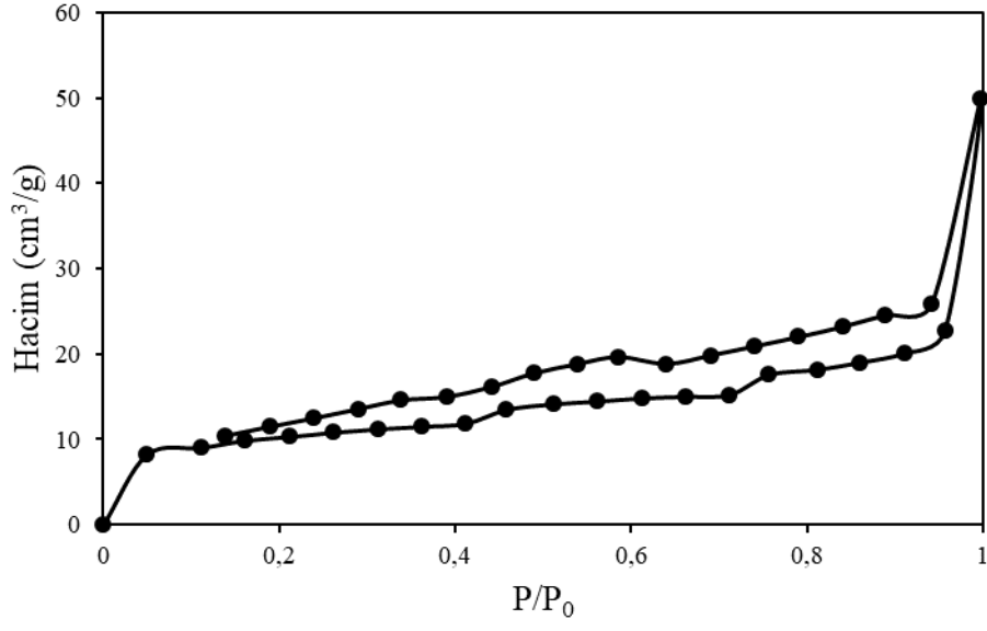
Şekil 6.36. %15 CoO/MA (700°C, 60 dk) katalizörünün azot adsorpsiyon-desorpsiyon izotermi
