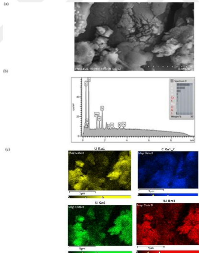
Şekil 6.38. MA destek maddesinin a)SEM görüntüsü b) EDS sonucu c) elementel haritası
