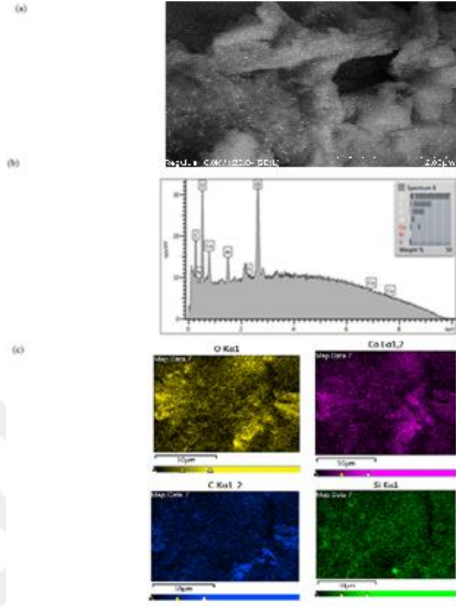
Şekil 6.39. %15 Co/MA örneğinin a)SEM görüntüsü b) EDS sonucu c) elementel haritası
