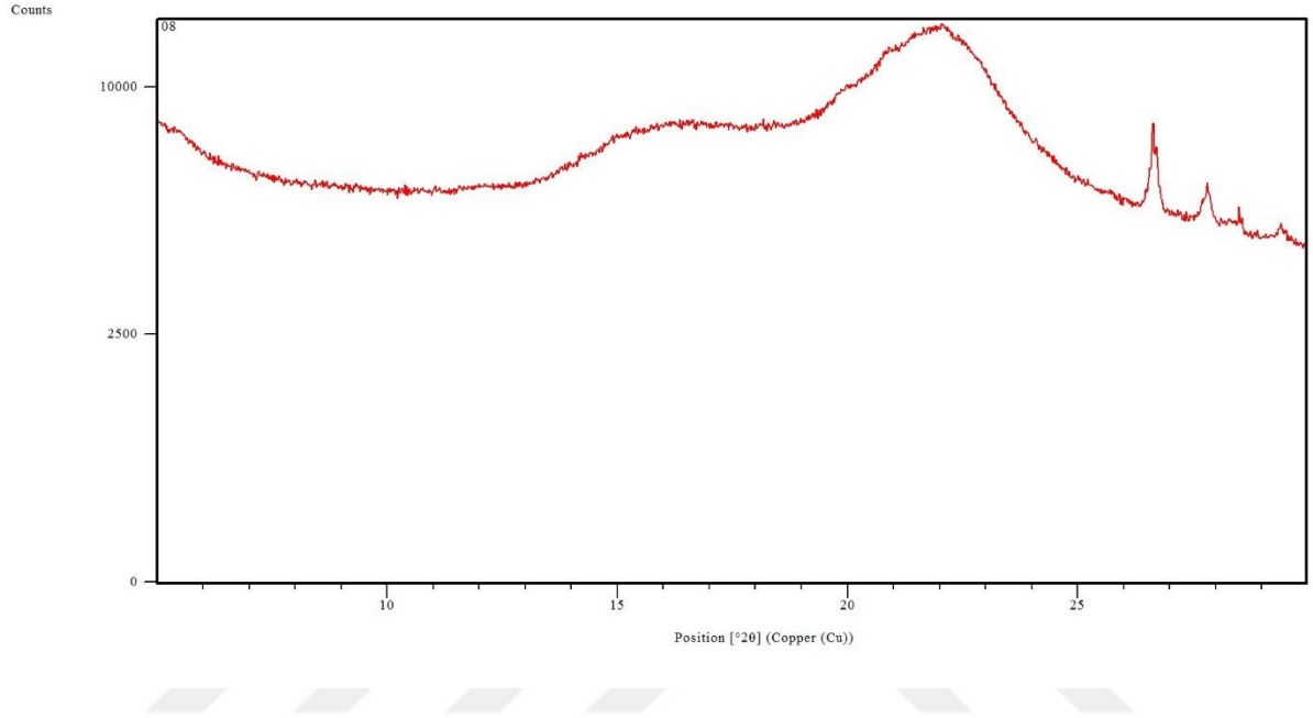
Şekil 6.22. MA destek maddesinin XRD kırınım deseni
