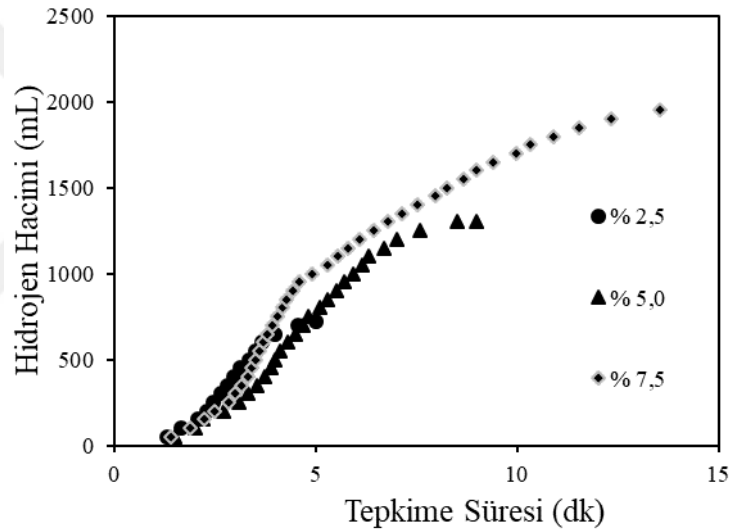
Şekil 6.16. CoO/MA katalizörü ile sodyum borhidrür hidrolizinde sodyum borhidrür derişiminin hidrojen üretim hacmine etkisi (kalsinasyon sıcaklığı: 600°C, kalsinasyon süresi: 60 dk, sodyum hidroksit derişimi: %2,5, katalizör miktarı: 0,05 g, tepkime sıcaklığı: 50°C)
