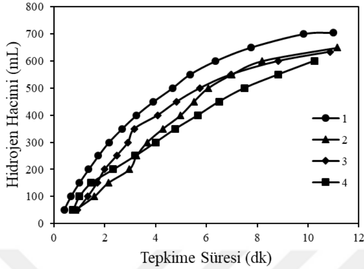
Şekil 6.10. CoB/MA katalizörü ile sodyum borhidrür hidrolizinde katalizörün tekrar kullanım sayısının hidrojen üretim hacmine etkisi (indirgeme oranı: 3:1 \text{BH}_4^-/\text{Co} , metal yükleme oranı: %15, sodyum hidroksit derişimi: %2,5, katalizör miktarı: 0,05 g, sodyum borhidrür derişimi: %2,5, tepkime sıcaklığı: 50°C)
