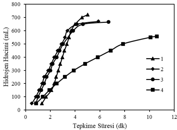
Şekil 6.21. CoO/MA katalizörü ile sodyum borhidrür hidrolizinde katalizörün tekrar kullanım sayısının hidrojen üretim hacmine etkisi (kalsinasyon sıcaklığı: 600°C, kalsinasyon süresi: 60 dk, sodyum hidroksit derişimi: %2,5, katalizör miktarı: 0,05 g, sodyum borhidrür derişimi: %2,5, tepkime sıcaklığı: 50°C)
