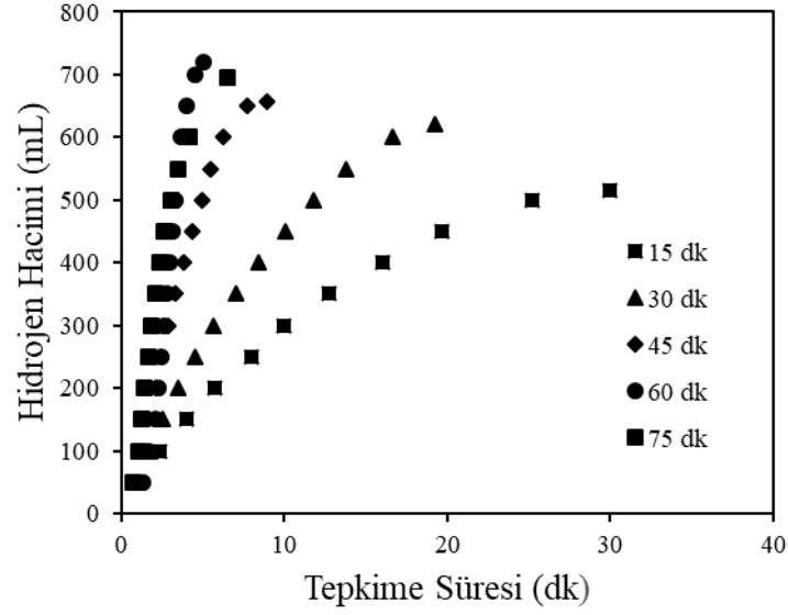
Şekil 6.13. CoO/MA katalizörü ile sodyum borhidrür hidrolizinde kalsinasyon süresinin hidrojen üretim hacmine etkisi (kalsinasyon sıcaklığı: 600°C, sodyum hidroksit derişimi: %2,5, katalizör miktarı: 0,05 g, sodyum borhidrür derişimi: %2,5, tepkime sıcaklığı: 50°C)
