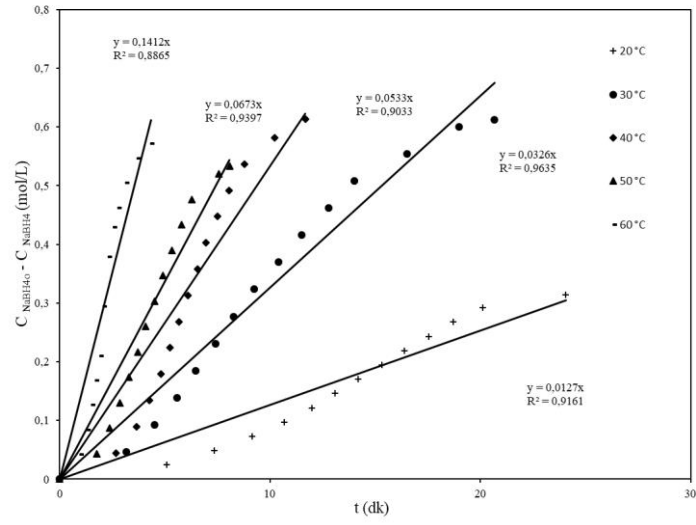
Şekil 6.18. CoO /MA katalizörünün sıfırıncı derece tepkime grafiği
