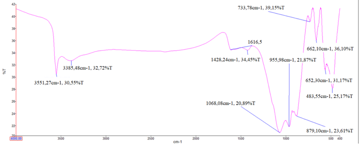
Şekil 6.50. %10 CoO/MA (600°C, 60 dk) katalizörünün FTIR spektrumu
