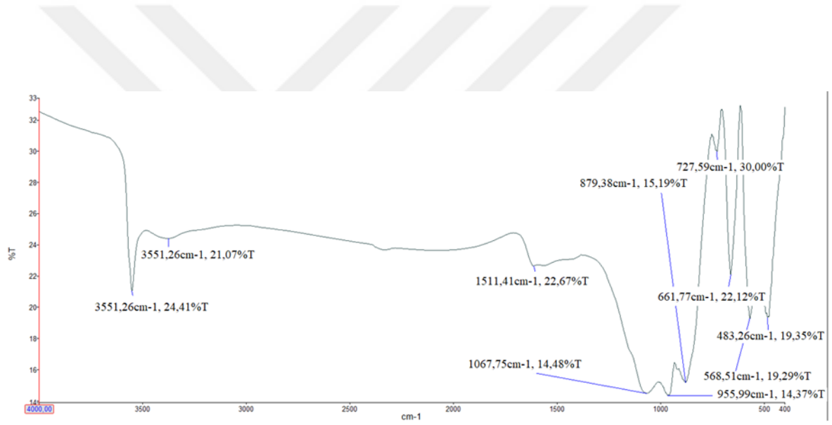
Şekil 6.48. %15 CoO/MA (600°C, 60 dk) katalizörünün FTIR spektrumu
