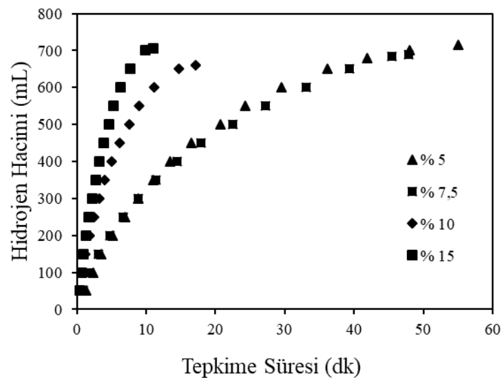
Şekil 6.2. CoB/MA katalizörü ile sodyum borhidrür hidrolizinde metal yükleme oranının hidrojen üretim hacmine etkisi (indirgeme oranı: 3:1 \text{BH}_4^-/\text{Co} , sodyum hidroksit derişimi: %2,5, katalizör miktarı: 0,05 g, sodyum borhidrür derişimi: %2,5, tepkime sıcaklığı: 50°C)
