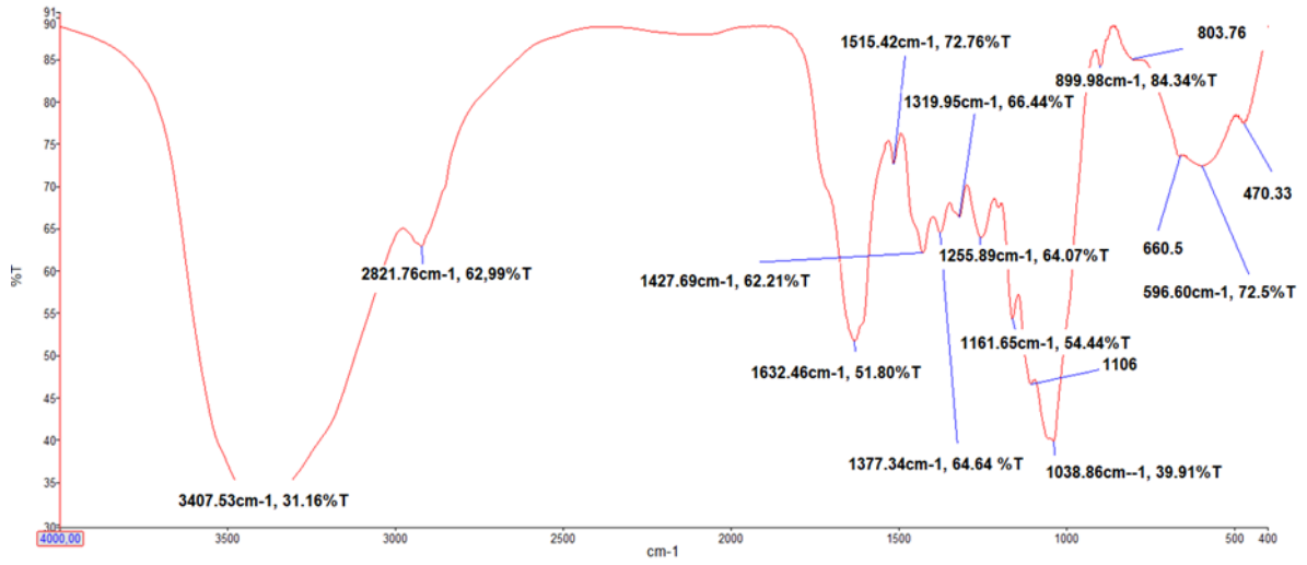
Şekil 6.45. %15 Co/MA örneğinin FTIR spektrumu
