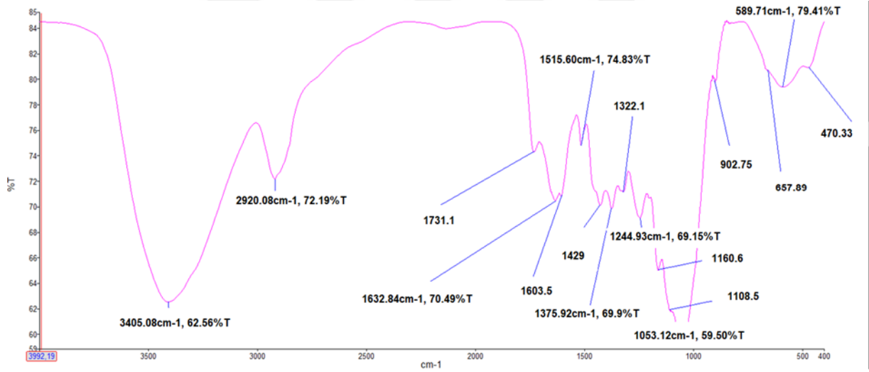
Şekil 6.44. MA destek maddesinin FTIR spektrumu
