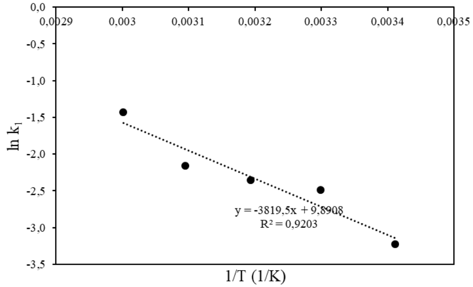
Şekil 6.9. CoB/MA katalizörünün 1/T - \ln k_1 grafiği
