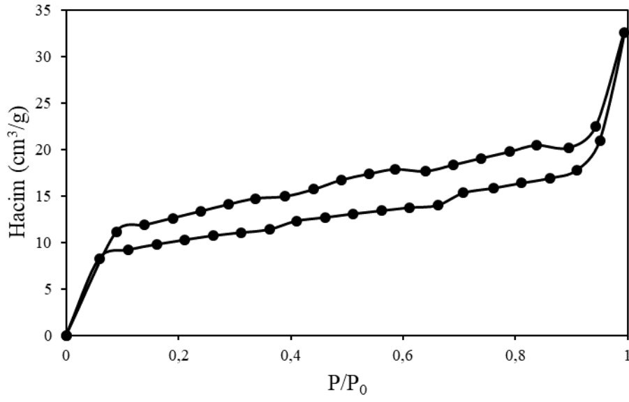
Şekil 6.34. %15 CoO/MA (600°C, 60 dk) katalizörünün azot adsorpsiyon-desorpsiyon izotermi
