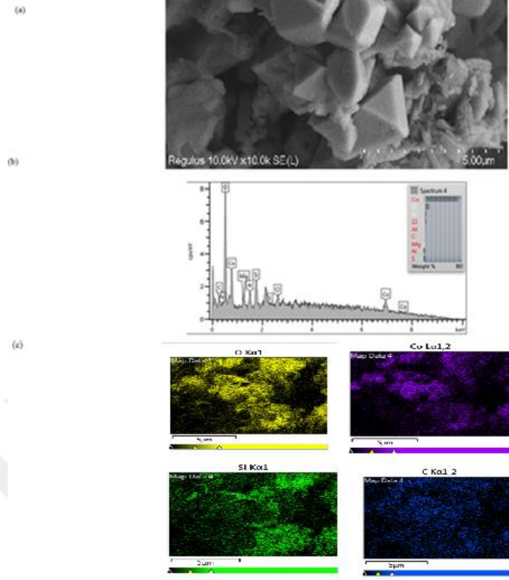
Şekil 6.43. %15 CoO/MA (700°C, 60 dk) katalizörünün a)SEM görüntüsü b) EDS sonucu c) elementel haritası
