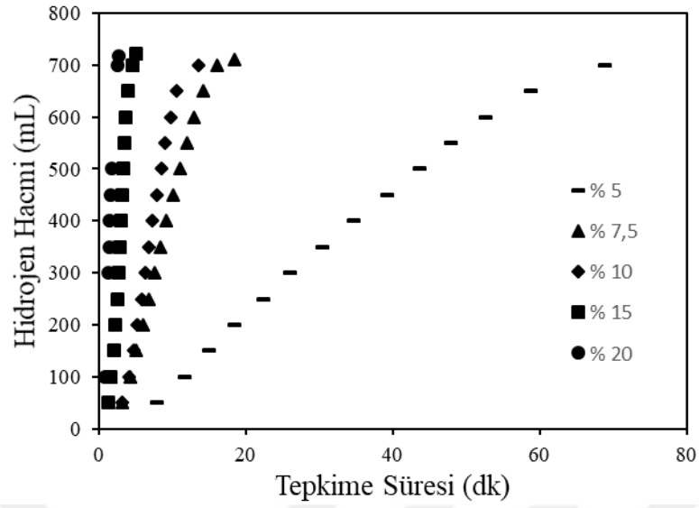
Şekil 6.11. CoO/MA katalizörü ile sodyum borhidrür hidrolizinde kobalt yükleme oranının hidrojen üretim hacmine etkisi (kalsinasyon sıcaklığı: 600°C, kalsinasyon süresi: 60 dk, sodyum hidroksit derişimi: %2,5, katalizör miktarı: 0,05 g, sodyum borhidrür derişimi: %2,5, tepkime sıcaklığı: 50°C)
