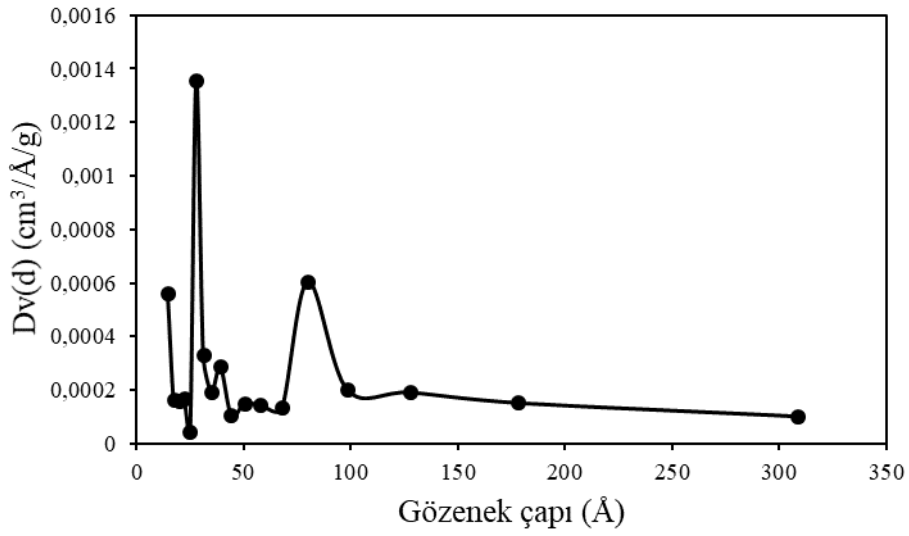
Şekil 6.31. %15 CoB/MA (3:1 BH 4 - / Co) katalizörünün gözenek boyut dağılımı
