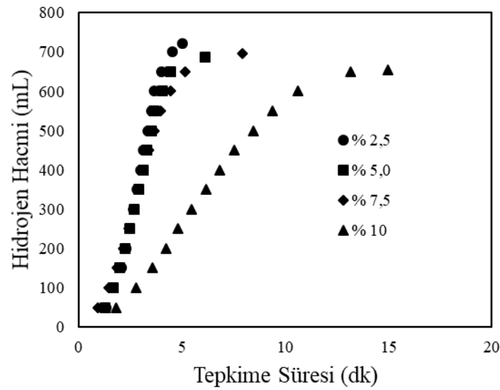
Şekil 6.14. CoO/MA katalizörü ile sodyum borhidrür hidrolizinde sodyum hidroksit derişiminin hidrojen üretim hacmine etkisi (kalsinasyon sıcaklığı: 600°C, kalsinasyon süresi: 60 dk, katalizör miktarı: 0,05 g, sodyum borhidrür derişimi: %2,5, tepkime sıcaklığı: 50°C)
