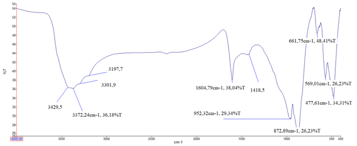
Şekil 6.47. %15 CoO/MA (500°C, 60 dk) katalizörünün FTIR spektrumu
