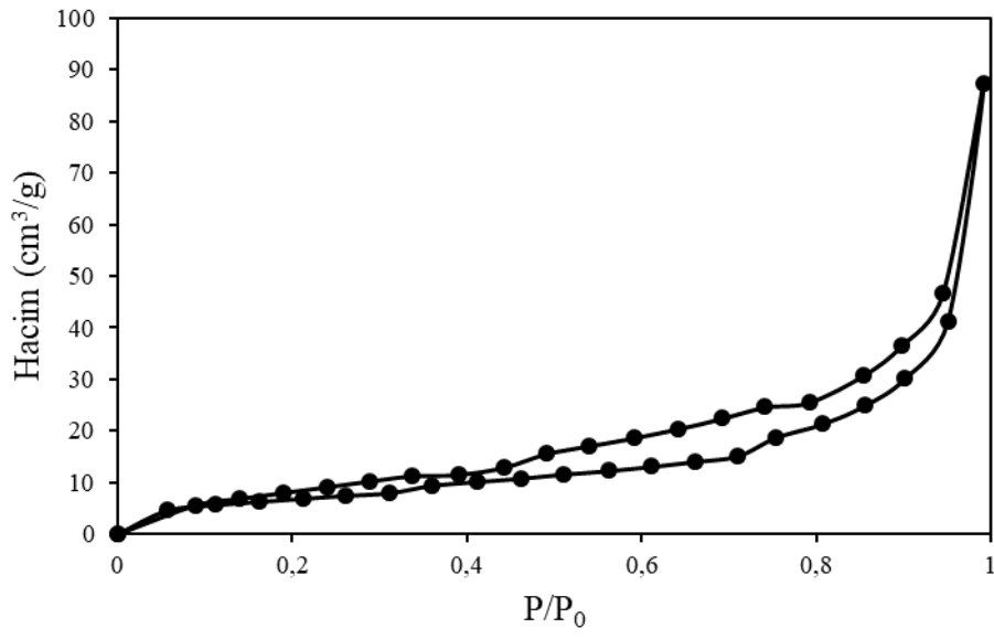
Şekil 6.30. %15 CoB/MA (3:1 BH 4 - / Co) katalizörünün azot adsorpsiyon-desorpsiyon izotermi
