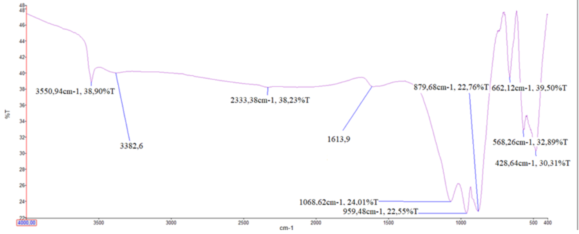
Şekil 6.49. %15 CoO/MA (700°C, 60 dk) katalizörünün FTIR spektrumu
