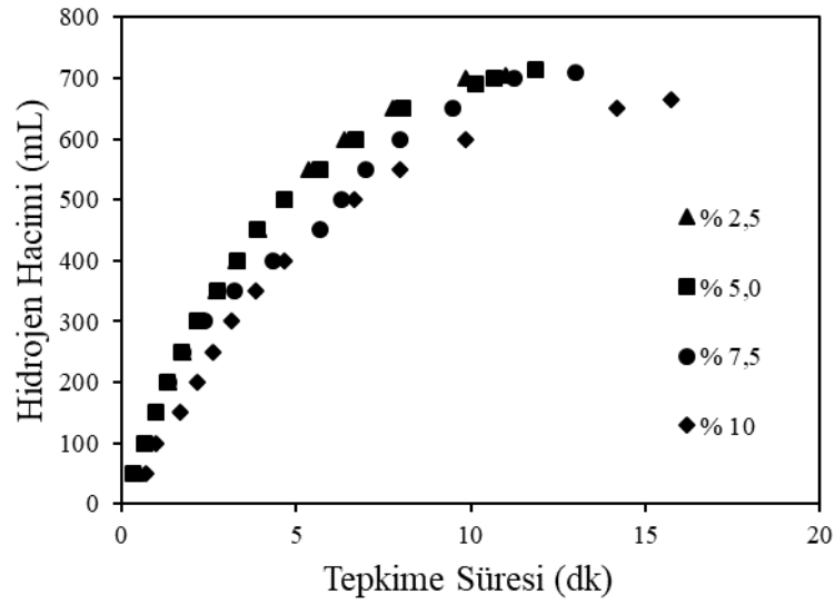
Şekil 6.3. CoB/MA katalizörü ile sodyum borhidrür hidrolizinde sodyum hidroksit derişiminin hidrojen üretim hacmine etkisi (indirgeme oranı: 3:1 BH_4^-/Co , metal yükleme oranı: %15, katalizör miktarı: 0,05 g, sodyum borhidrür derişimi: %2,5, tepkime sıcaklığı: 50°C)
