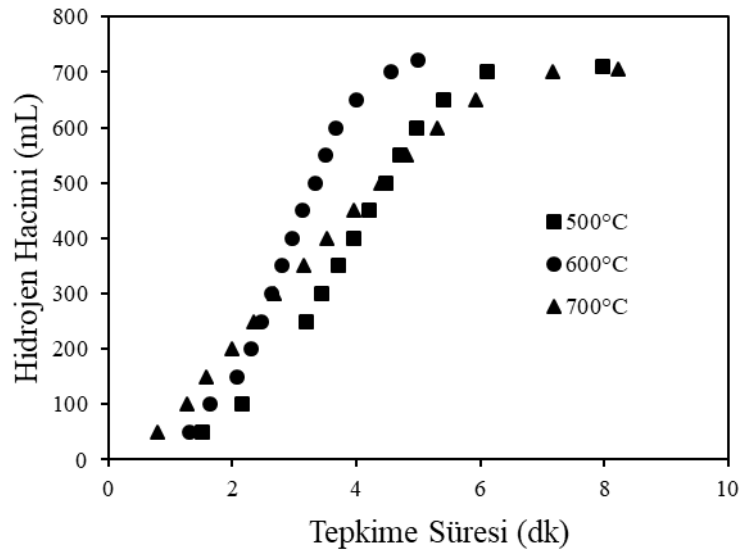
Şekil 6.12. CoO/MA katalizörü ile sodyum borhidrür hidrolizinde kalsinasyon sıcaklığının hidrojen üretim hacmine etkisi (kalsinasyon süresi: 60 dk, sodyum hidroksit derişimi: %2,5, katalizör miktarı: 0,05 g, sodyum borhidrür derişimi: %2,5, tepkime sıcaklığı: 50°C)
