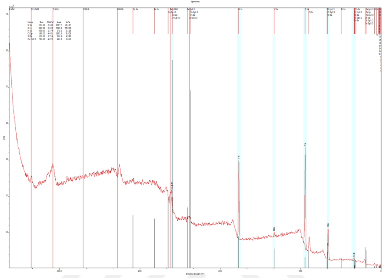
Şekil 6.53. %15 Co/MA örneğinin XPS analiz sonuçları
