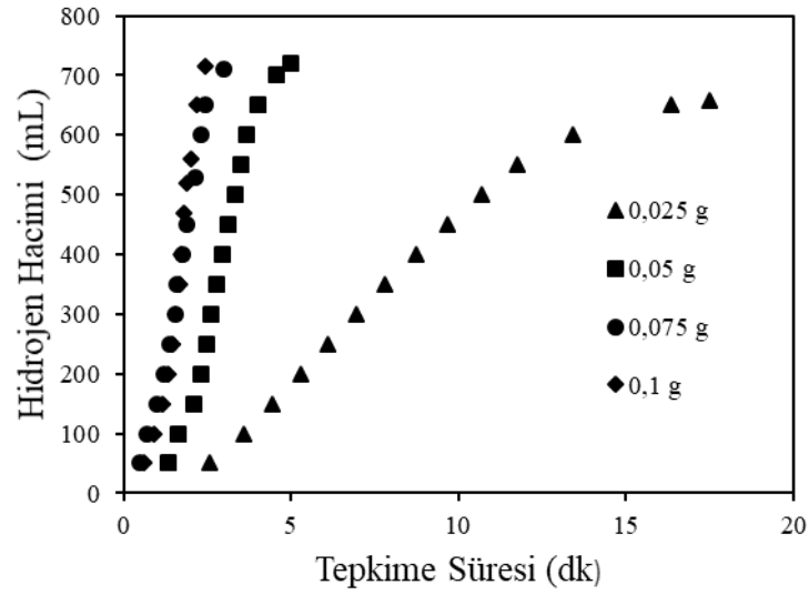
Şekil 6.15. CoO/MA katalizörü ile sodyum borhidrür hidrolizinde katalizör miktarının hidrojen üretim hacmine etkisi (kalsinasyon sıcaklığı: 600°C, kalsinasyon süresi: 60 dk, sodyum hidroksit derişimi: %2,5, sodyum borhidrür derişimi: %2,5, tepkime sıcaklığı: 50°C)
