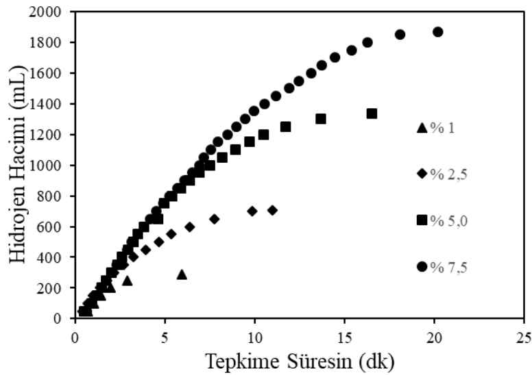
Şekil 6.5. CoB/MA katalizörü ile sodyum borhidrür hidrolizinde NaBH 4 sodyum borhidrür derişiminin hidrojen üretim hacmine etkisi (indirgeme oranı: 3:1 BH 4 - /Co, metal yükleme oranı: %15, sodyum hidroksit derişimi: %2,5, katalizör miktarı: 0,05 g, tepkime sıcaklığı: 50°C)
