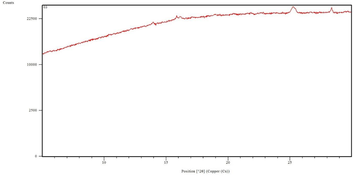
Şekil 6.23. %15 CoB/MA katalizörünün XRD kırınım deseni
