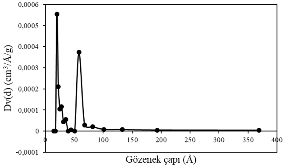
Şekil 6.29. MA destek maddesinin gözenek boyut dağılımı
