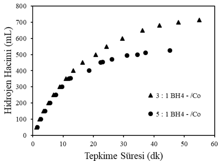
Şekil 6.1. CoB/MA katalizörü ile sodyum borhidrür hidrolizinde indirgeme oranının hidrojen üretim hacmine etkisi (metal yükleme oranı: %5, sodyum hidroksit derişimi: %2,5, katalizör miktarı: 0,05 g, sodyum borhidrür derişimi: %2,5, tepkime sıcaklığı: 50°C)
