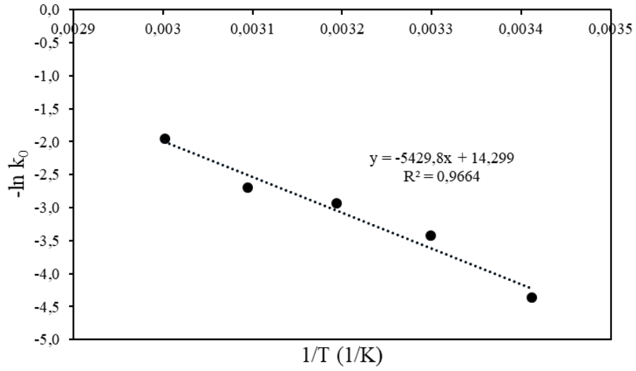
Şekil 6.20. CoO /MA katalizörünün 1/T-ln k 0 grafiği
