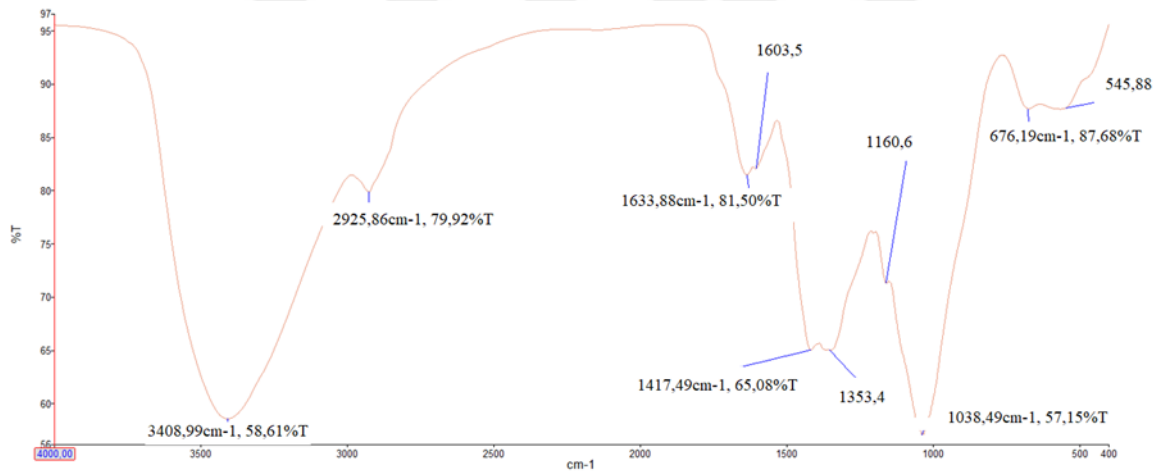
Şekil 6.46. %15 CoB/MA (3:1 \text{BH}_4^- / Co) katalizörünün FTIR spektrumu
