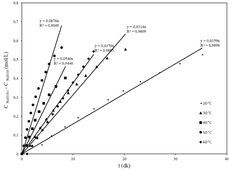
Şekil 6.7. CoB/MA katalizörünün sıfırıncı derece tepkime grafiği
