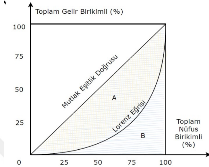
Şekil 1. Lorenz diyagramı 206
