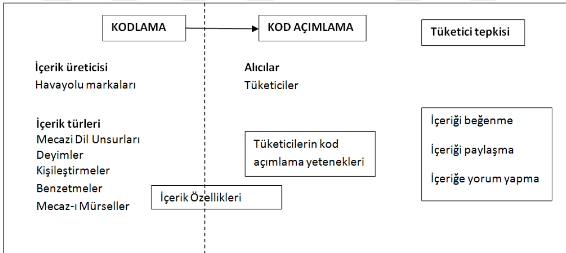
Şekil 3.1. Araştırmanın teorik çerçevesine uyarlanan kodlama-kod açıklama teorisi
