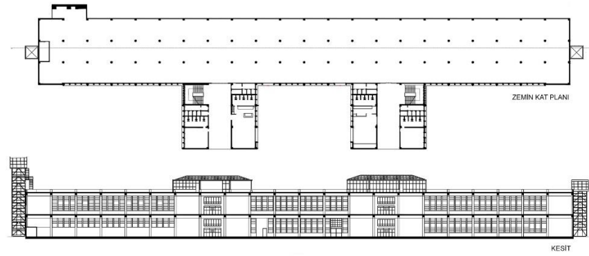
Şekil 3.4. Yeni Kundura Binası plan-kesit (Beykoz Kundura Mekân Kataloğu,2022)
