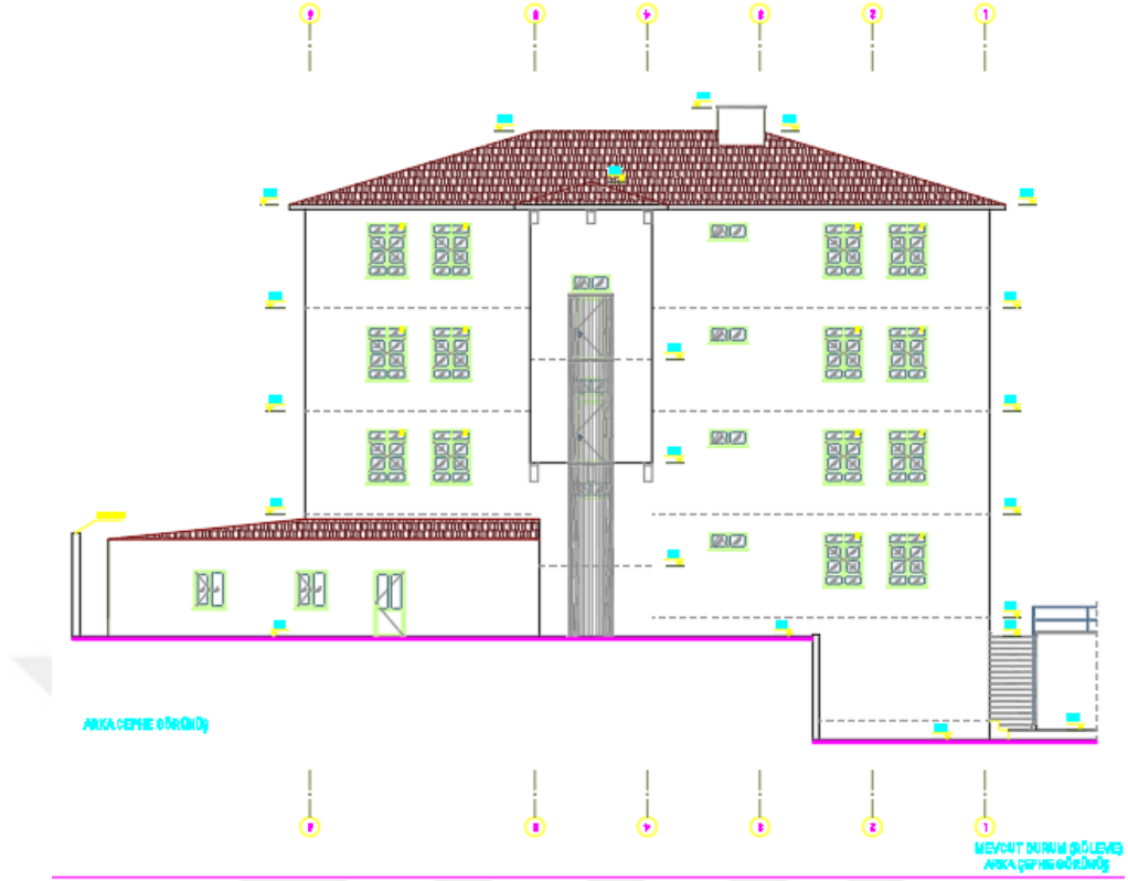
Şekil 4.4. Betonarme yapı arka cephe görünüş
