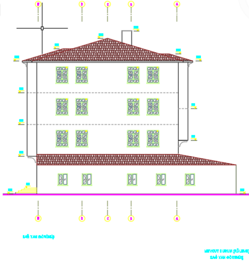
Şekil 4.5. Betonarme yapı sağ yan görünüş
