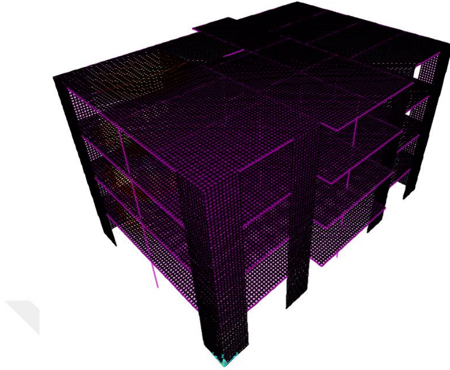
Şekil 4.20. Betonarme yapının yıkım-söküm işlemleri öncesi 2.Mod şekli
