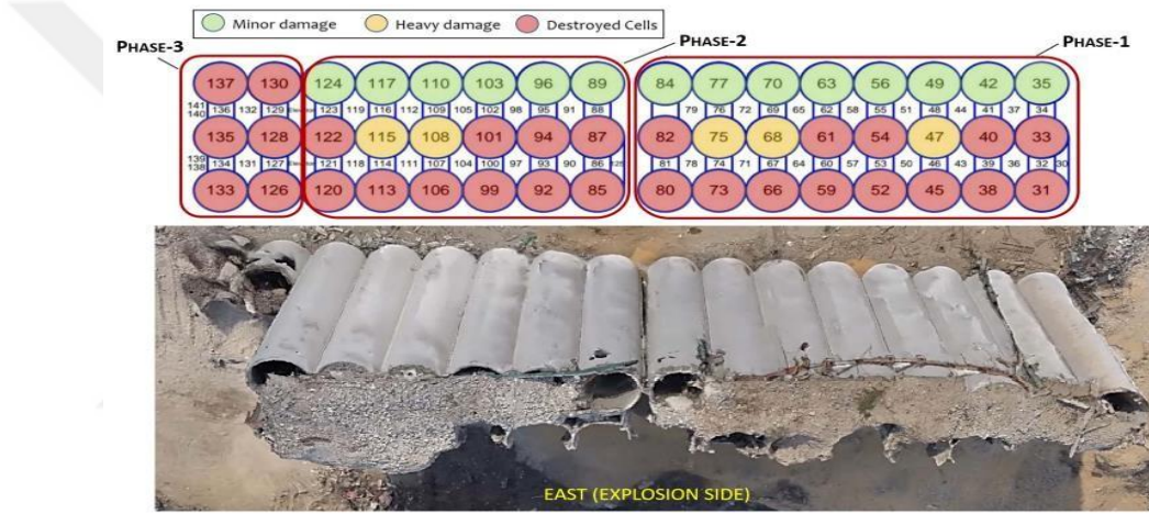
Şekil 3. 15. Tahıl silosu kompleksinin konfigürasyonunu gösteren plan görünümü. Silo gölgelendirmesi, patlama hasar seviyelerini gösterir. [47]
