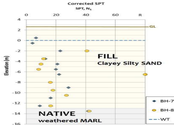
Şekil 3. 16. Yeraltı profili; Faz-1 silolarının ayak izi altındaki sondaj kuyularından alınan veriler. [48]
