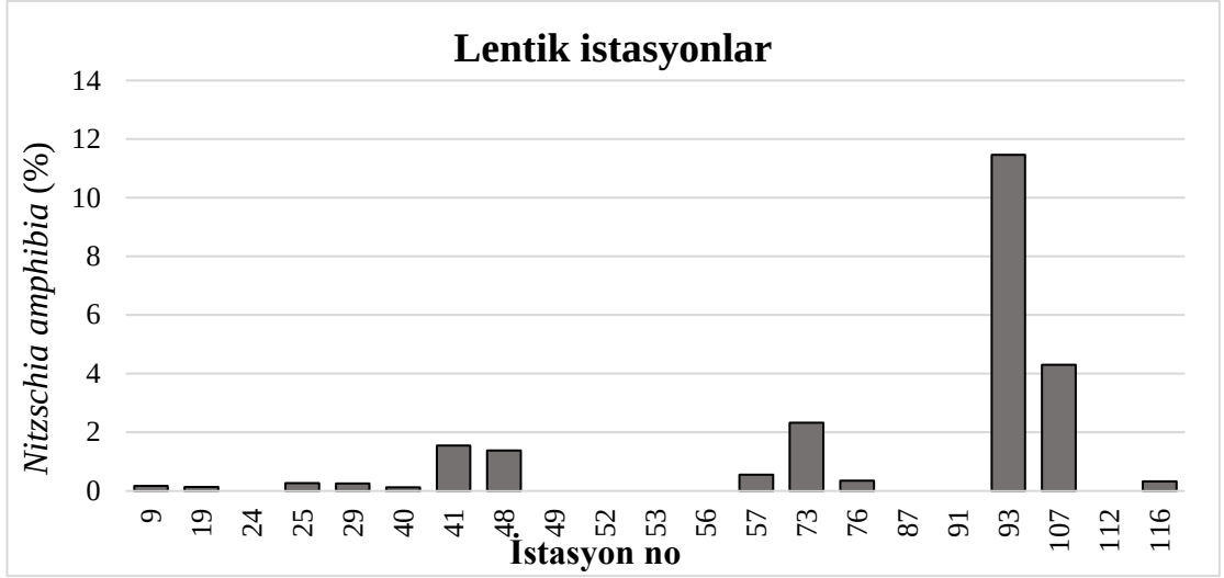
Şekil 4.61. Nitzschia amphibia 'nin lentik istasyonlardaki nispi bolluk değişimi
