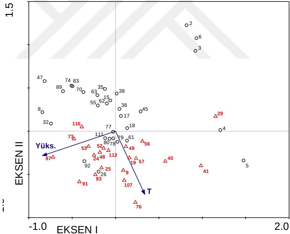
Şekil 4.68. İstasyonların çevresel değişkenler ile birlikte ordınasyon grafiği (Daire lotik, üçgen lentik istasyonlar).
