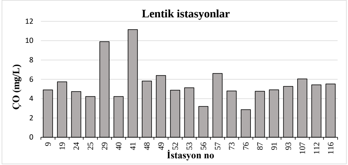
Şekil 4.11. Lentik istasyonların çözünmüş oksijen değerleri
