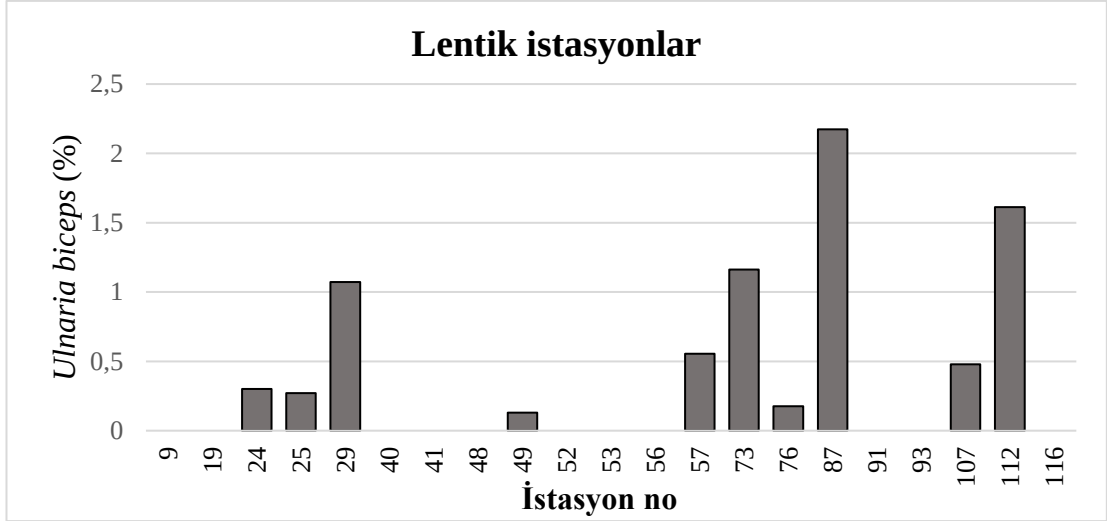
Şekil 4.51. Ulnaria biceps 'in lentik istasyonlardaki nispi bolluk değışimi
