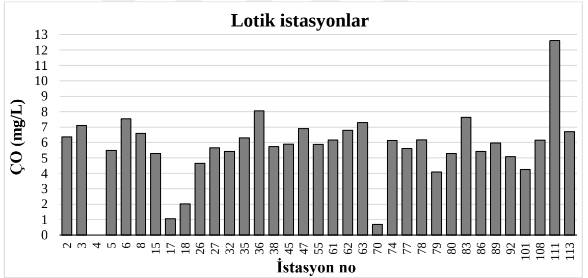
Şekil 4.10. Lotik istasyonların çözünmüş oksijen değerleri
