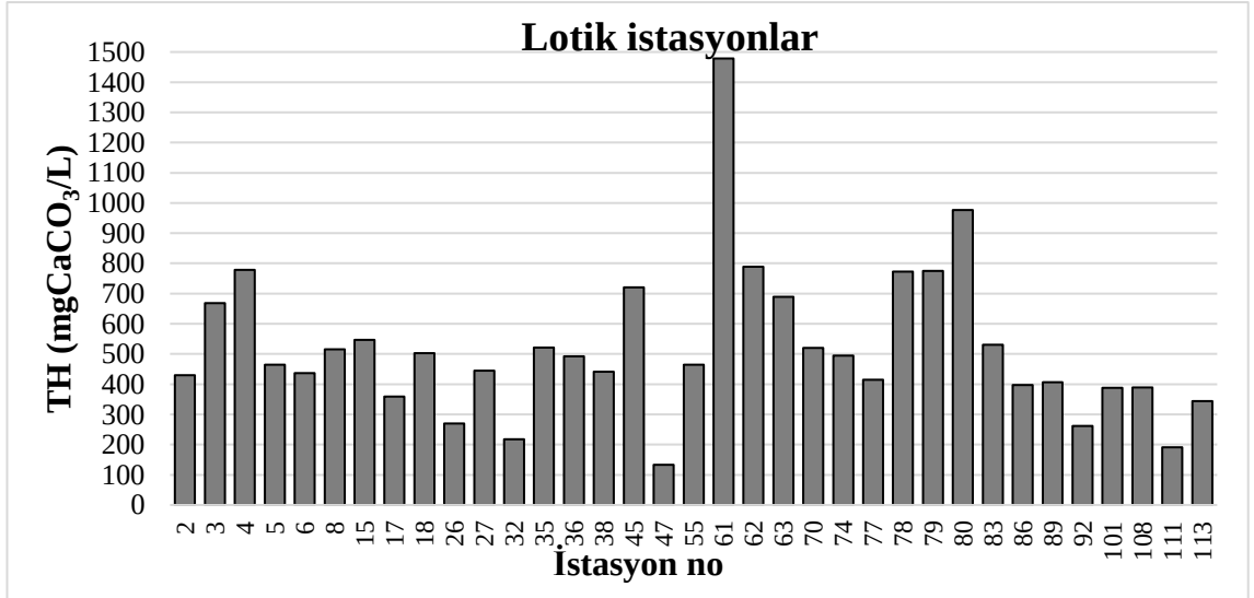
Şekil 4.19. Lotik istasyonların toplam sertlik değerleri
