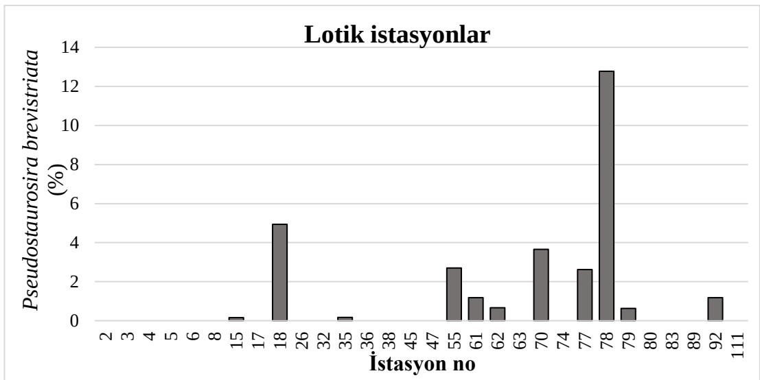
Şekil 4.52. Pseudostaurosira brevistriata 'nın lotik istasyonlardaki nispi bolluk değışimi
