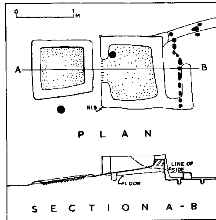
Plan 30: Hacilar GN/IIA ocak/fırın planları (Mellaart 1970b).
