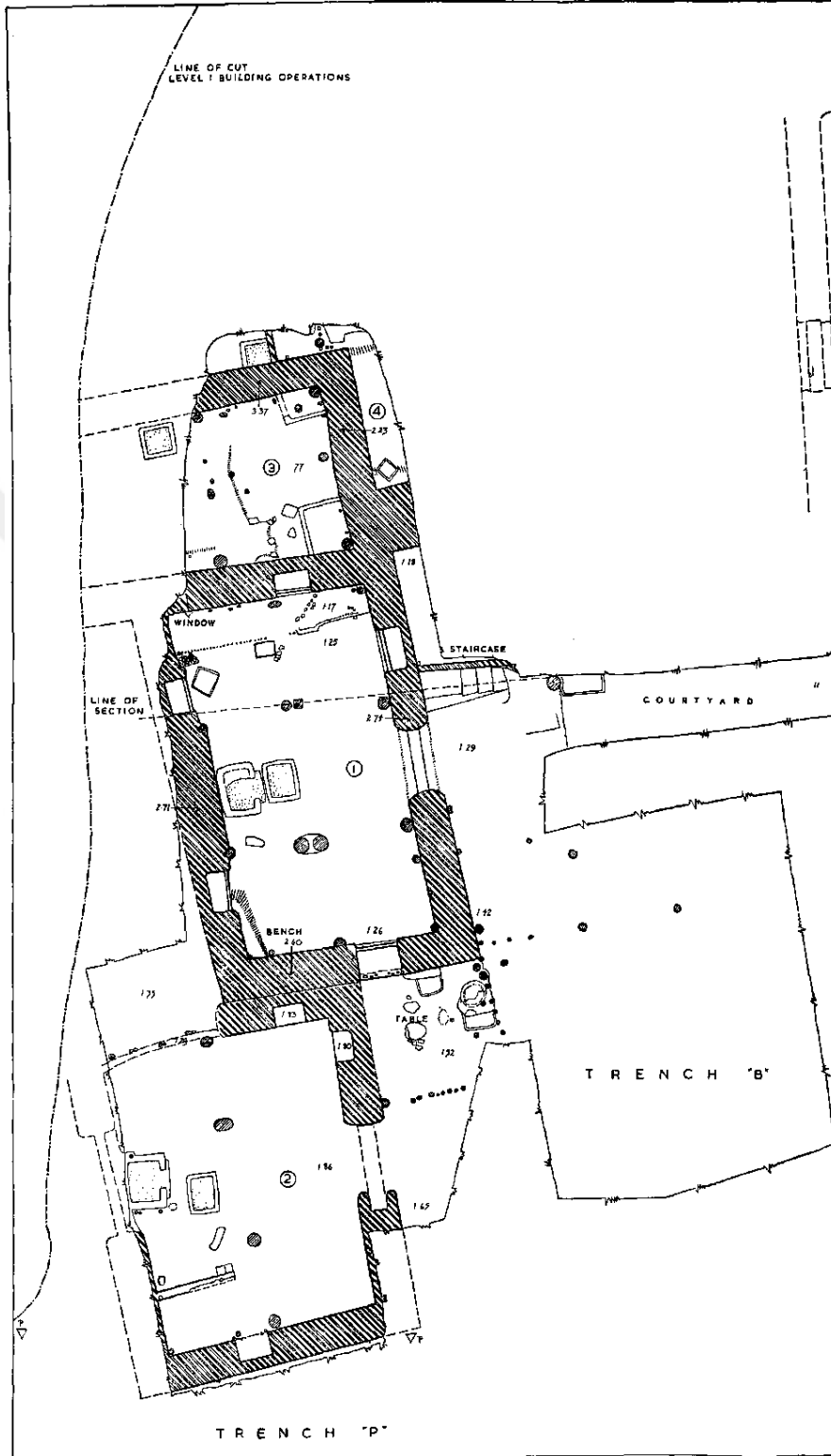
Plan 20: Hacilar EN II/VI yerleşim planı (Mellaart 1970b).
