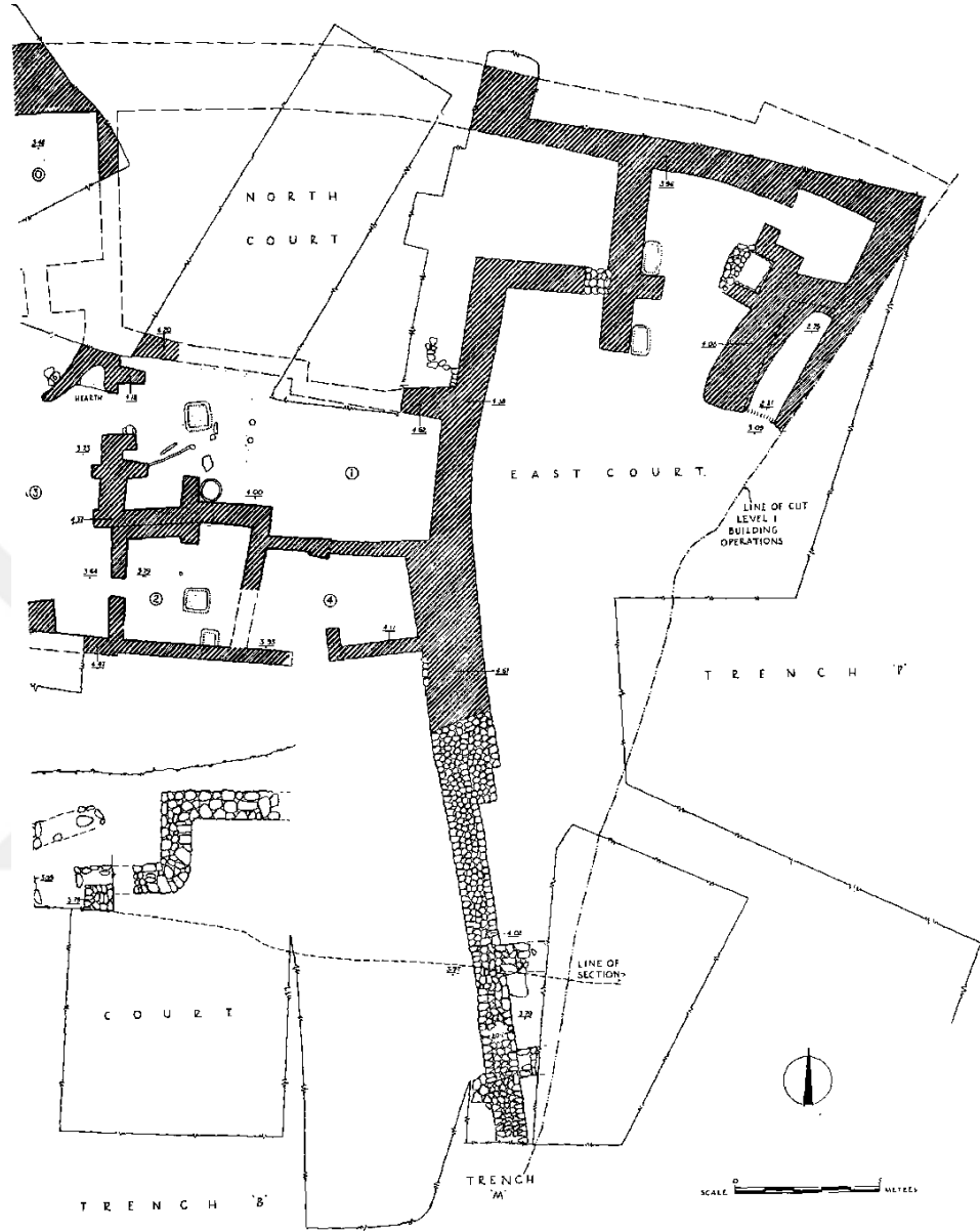
Plan 27: Hacilar GN/IIB yerleşim planı (Mellaart 1970b).
