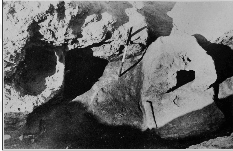
Resim 51: Hacılar EN II/VI tabakası Q.6 evinde bulunan dörtgen planlı fırın ve depolama ünitesi (Mellaart 1970b).
