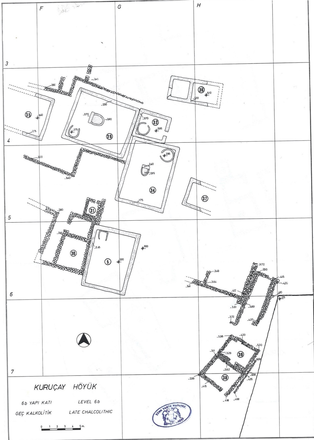
Plan 12: Kuruçay GKÇ/6b yerleşim planı (Duru 1996).
