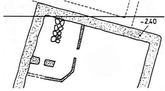
Çizim 4: Kuruçay GKÇ/6a Paravanalar (Duru, 1996).
