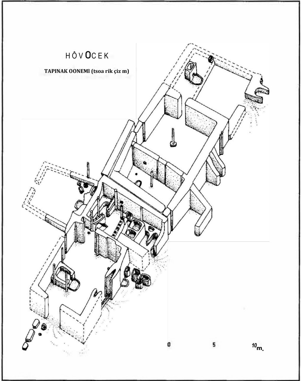
Plan 6: Höyücek Tapınak Dönemi yapılarının izometrik çizimi. (Duru Umurtak 2005).
