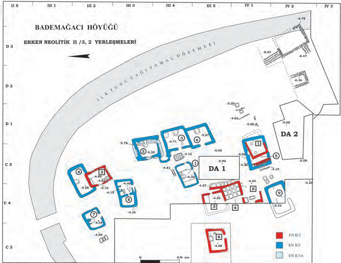
Plan 2: Bademağacı EN II/2-3 yerleşim planı (Duru Umurtak 2019).
