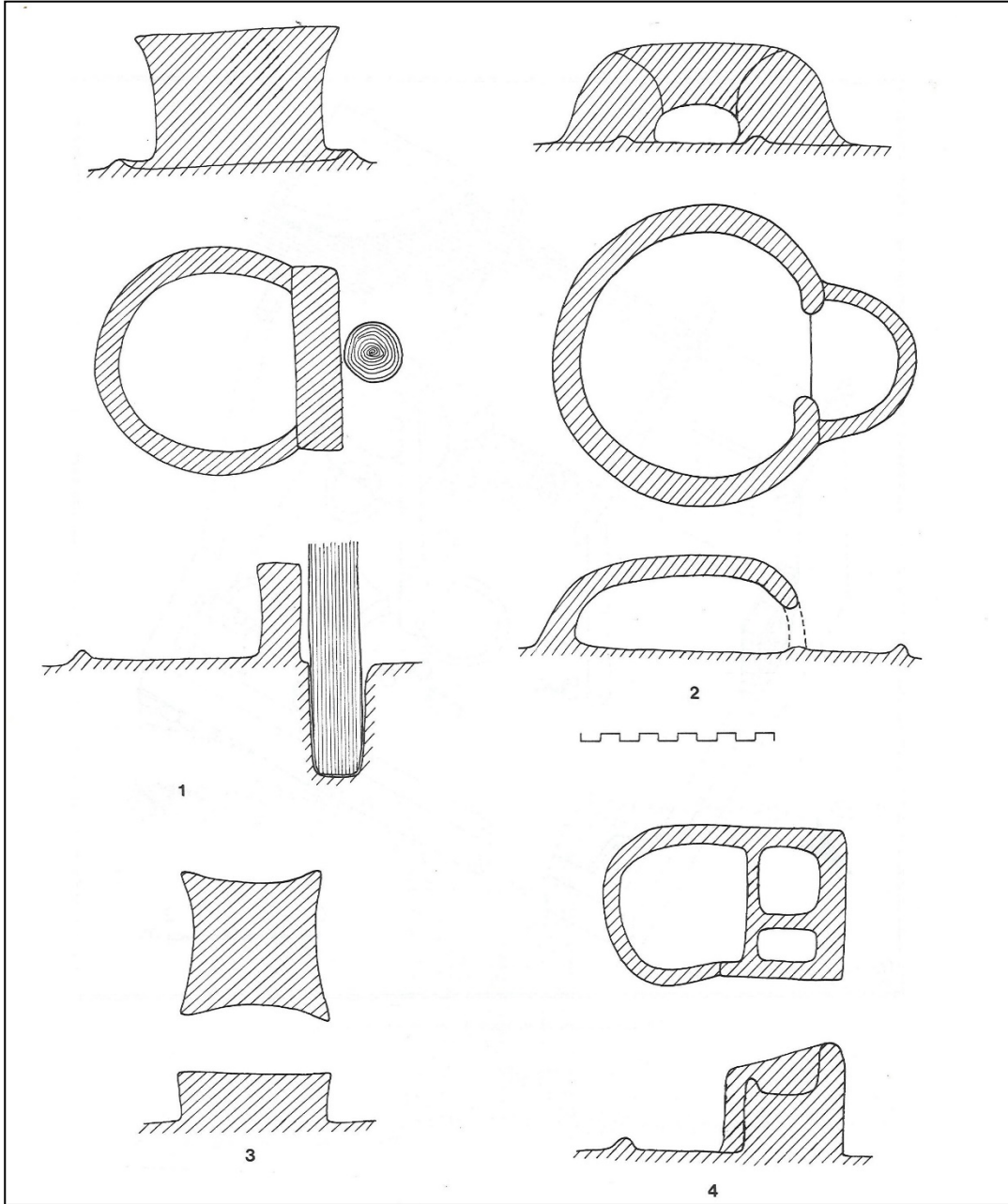
Resim 43: Kuruçay GKÇ/3 56 numaralı tapınak yapısı içerisinde bulunan taşınmazlara ait çizimler; 1. Kerpiç stelli ocak/sunak, 2. Yarım daire planlı kül yalıklı fırın, 3. İç bükey kenarlı masif kil masa, 4. Dörtgen planlı kül yalıklı ocak (Duru 1994)
