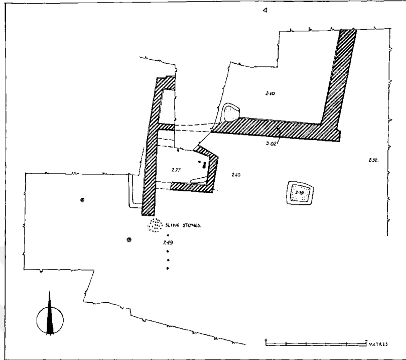
Plan 22: Hacilar GN/IV yerleşim planı (Mellaart 197b).
