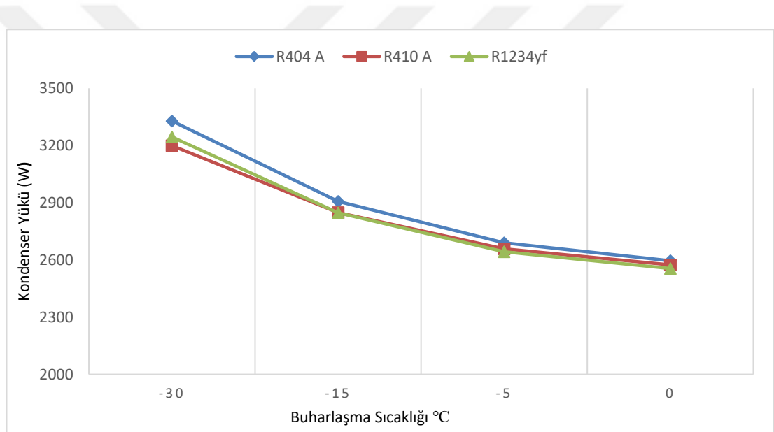
Şekil 5.3. Sistemin farklı akışkanlara göre kondenser yükleri
