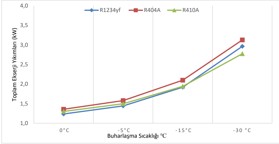
Şekil 5.4. Sistemlerin ekserji yıkımları
