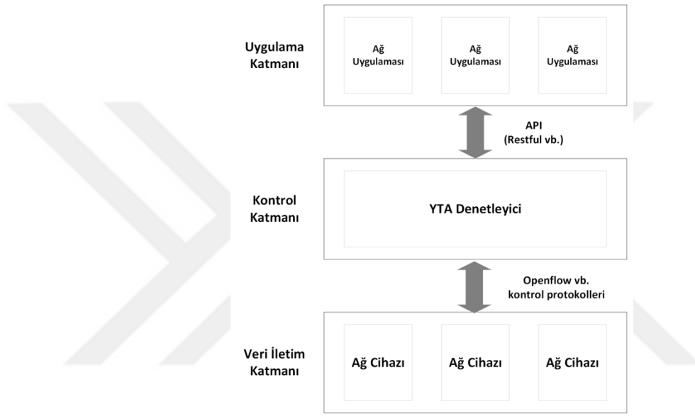
Şekil 1.4. YTA mimarisi
