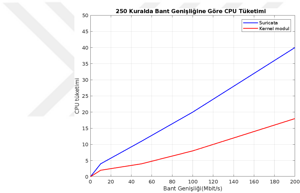
Şekil 4.3. Sabit kural sayısında bant genişliği artırılarak CPU tüketimi
