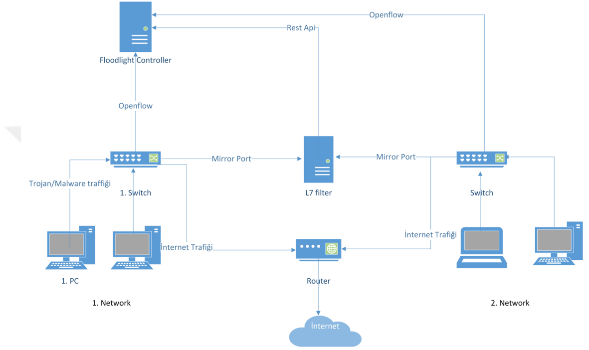
Şekil 4.4. Katman 7 filtrelemenin YTA mimarisine uygulanması
