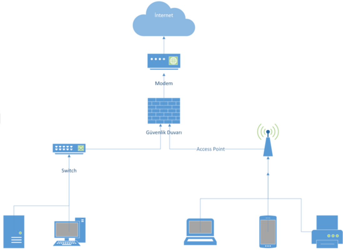
Şekil 1.1. Güvenlik Duvarı
