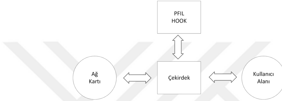
Şekil 3.2. PFIL Hook
