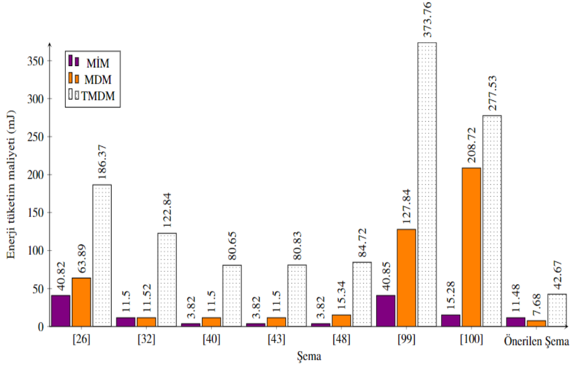
Şekil 5.3. Önerilen şema ve diğer şemaların enerji tüketim maliyetlerinin karşılaştırılması
