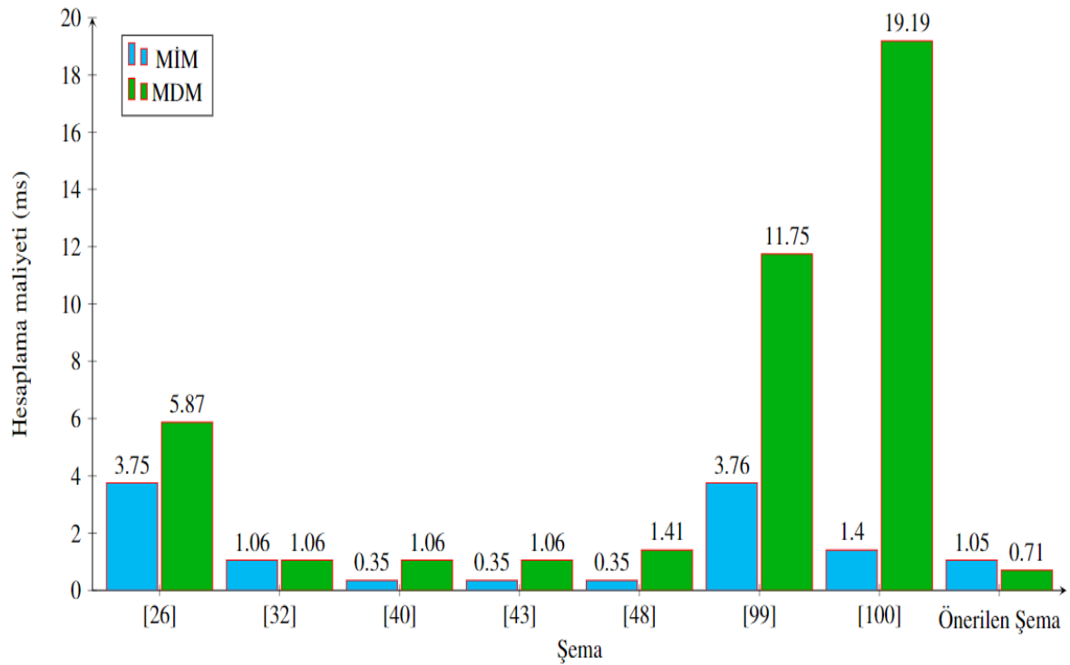
Şekil 5.2. Önerilen şemanın ve mevcut şemaların hesaplama maliyetinin karşılaştırılması
