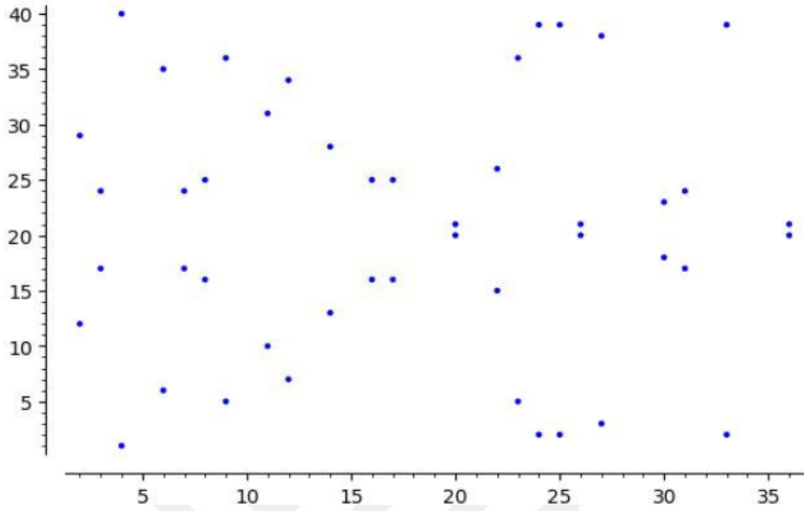
Şekil 3.2. E / \mathbb{F}_{41} : y^2 = x^3 + 3x + 7 eliptik eğrisinin noktalarının gösterimi
