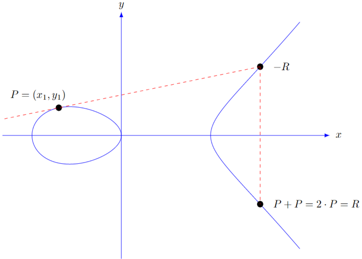
Şekil 3.6. Eliptik eğri üzerinde nokta çiftleme ( P + P = 2 \cdot P = R )
