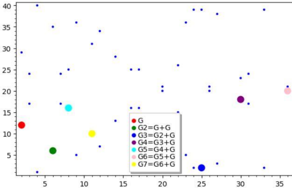
Şekil 3.8. Eliptik eğri üzerindeki noktalar arasında bağlantı
