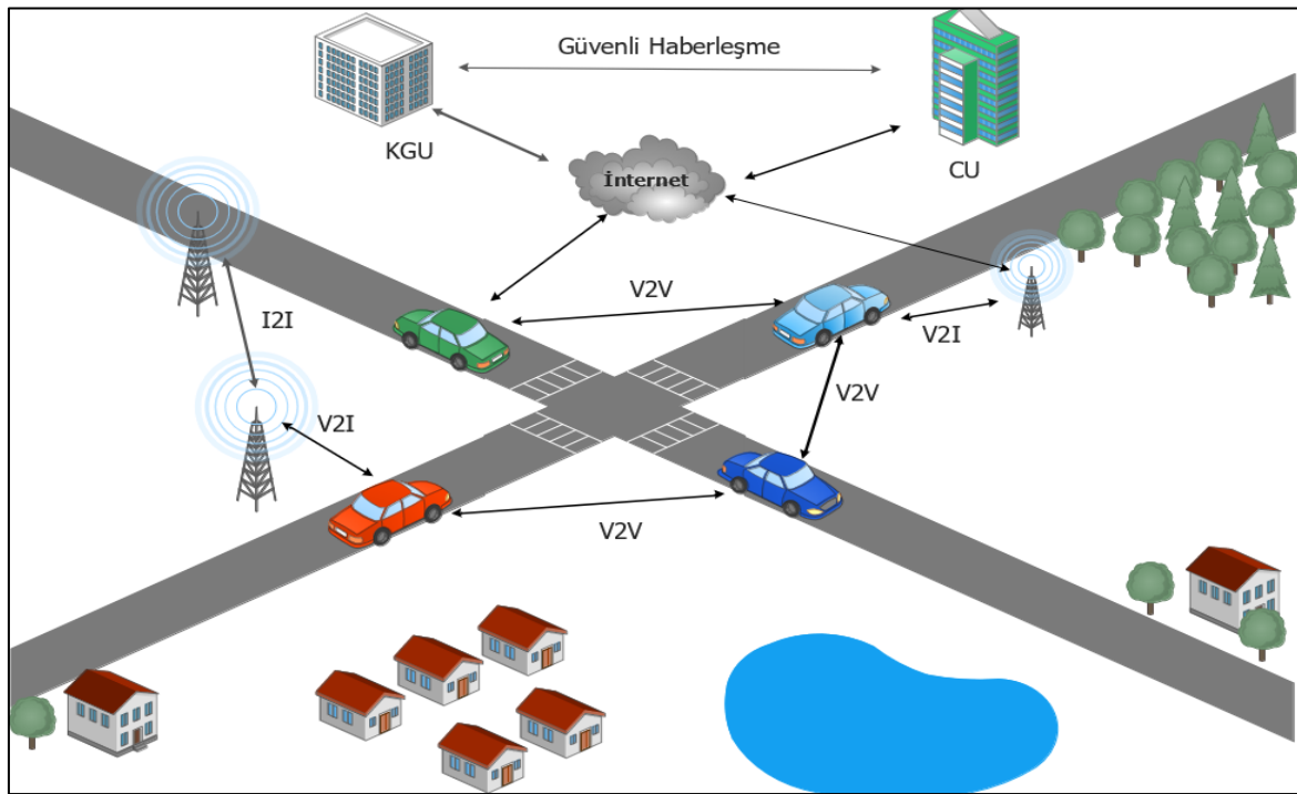
Şekil 5.1. IoV ağ mimarisi
