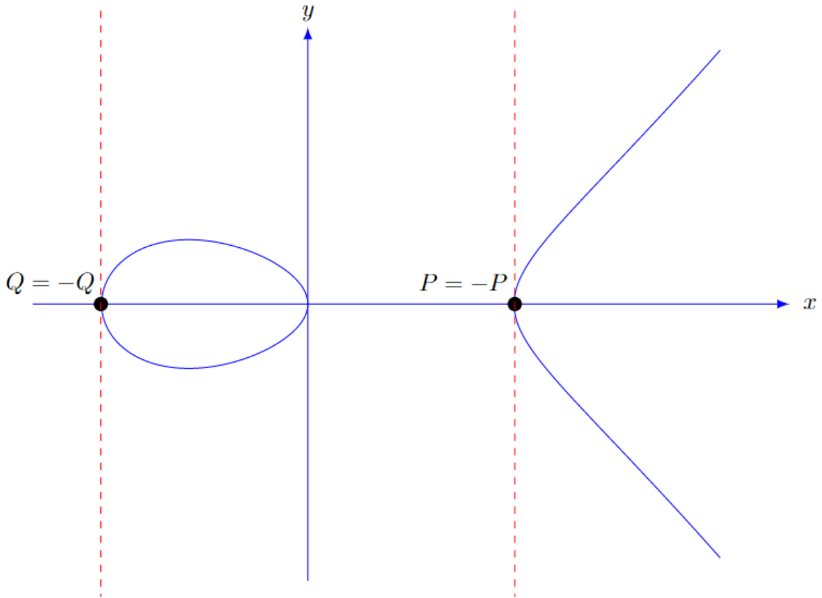
Şekil 3. 7. P = -P olması durumunda nokta çiftleme ( P + P = 2 \cdot P = \mathcal{O} )
