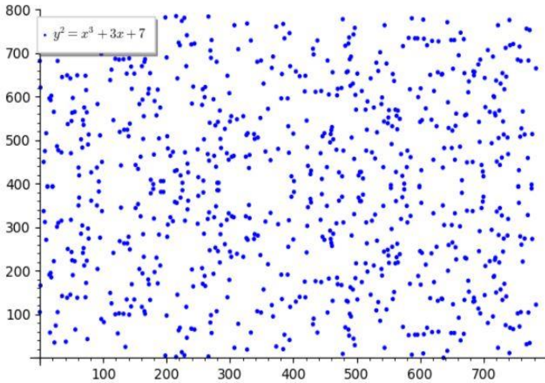
Şekil 3.3. E / \mathbb{F}_{787} eliptik eğrisi üzerindeki noktaların gösterimi
