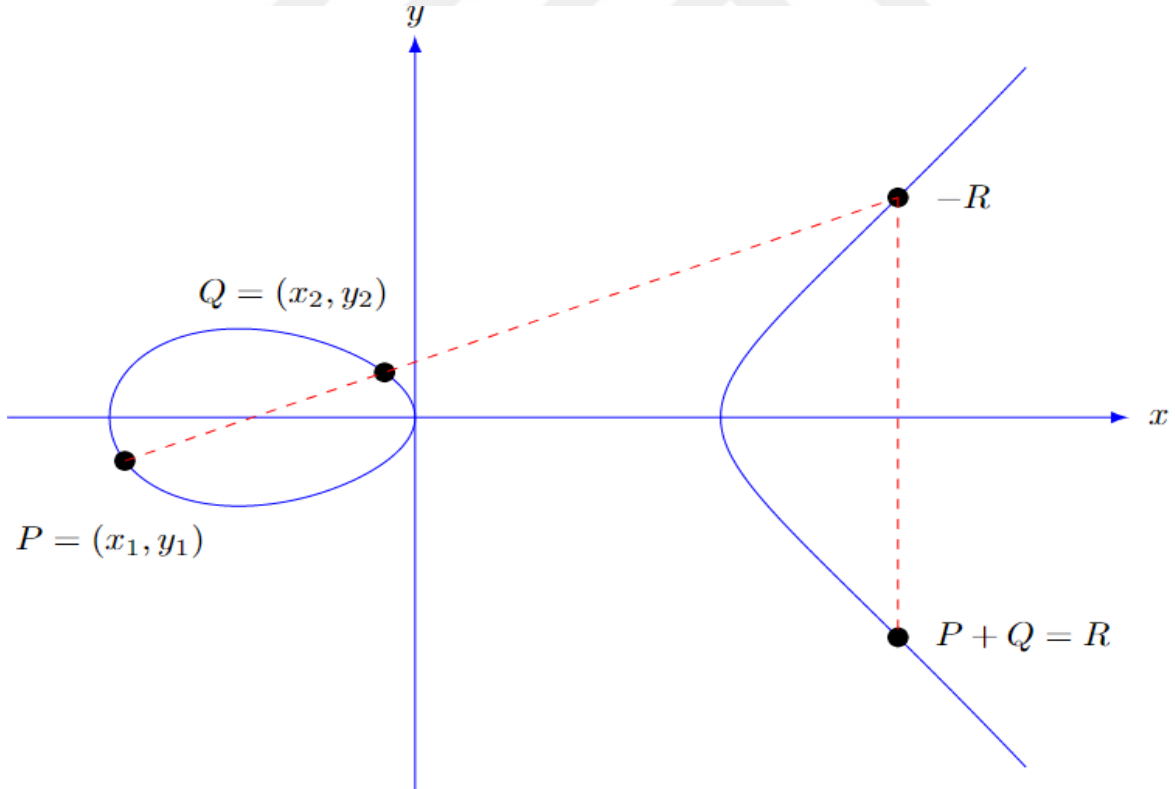
Şekil 3.5. Eliptik eğri üzerinde toplama işlemi ( P + Q = R )
