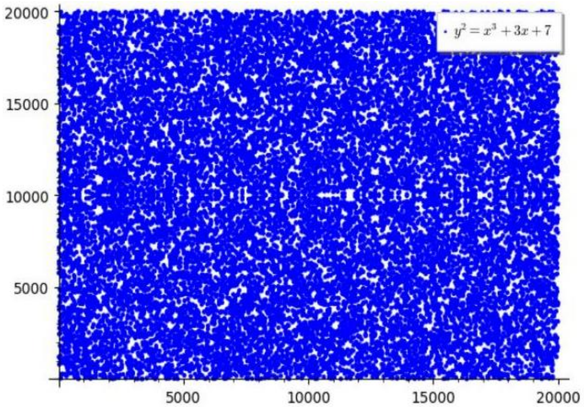
Şekil 3.4. E / \mathbb{F}_{20011} eliptik eğrisi üzerindeki noktaların gösterimi
