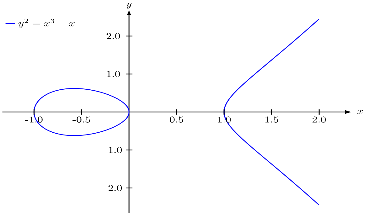
Şekil 3.1. y^2 = x^3 - x eliptik eğrisi
