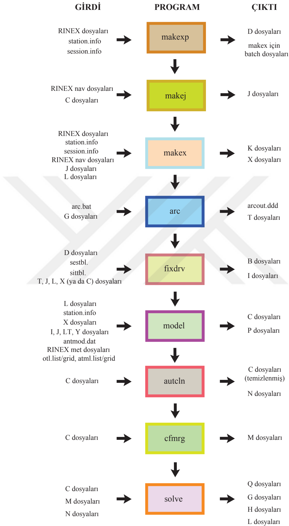
Şekil 2.9 GAMIT işlem adımları ([98]'den yararlanılmıştır)
