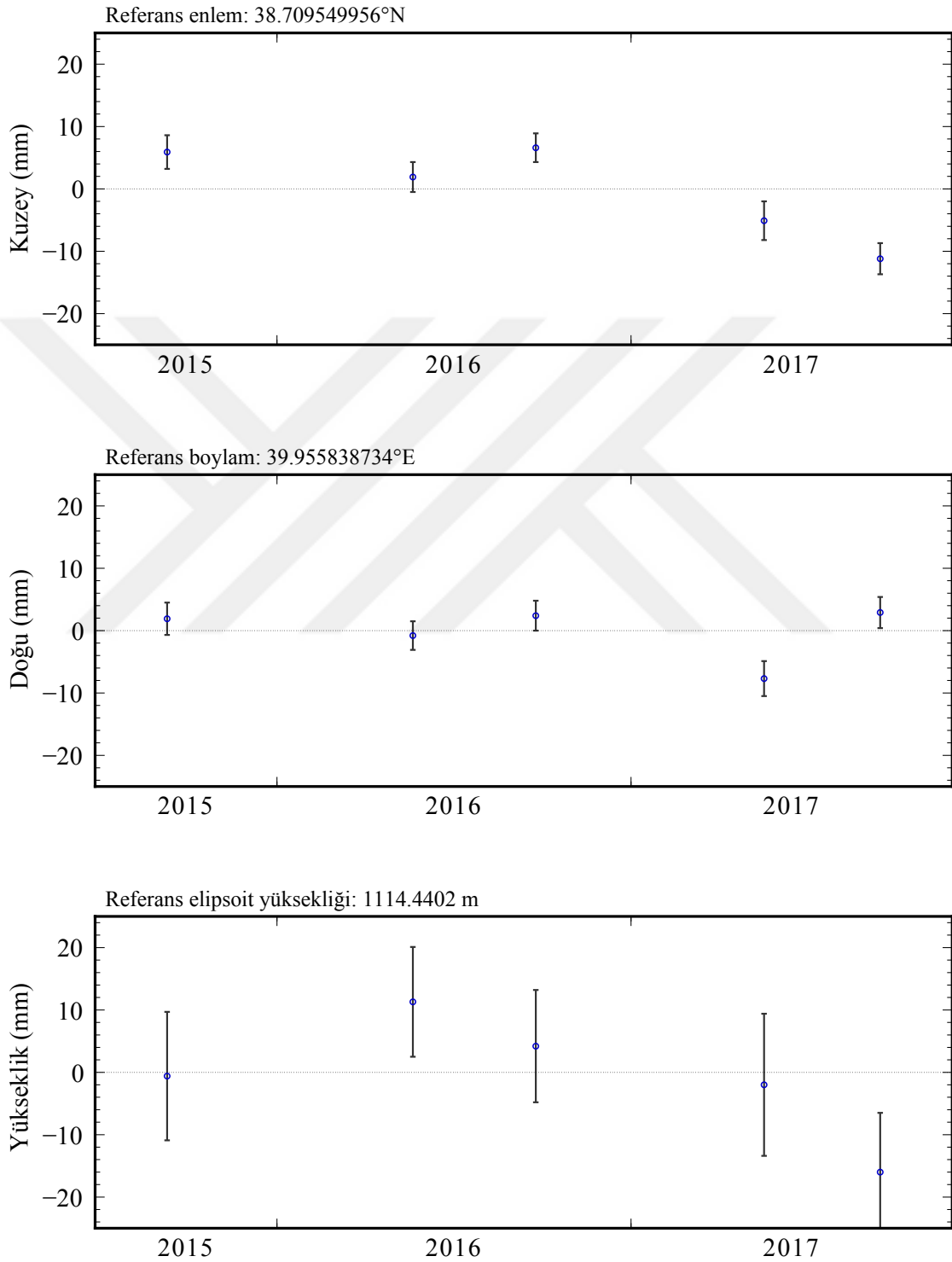
Şekil 4.14 EL06 kampanya GPS noktasına ait zaman serisi
