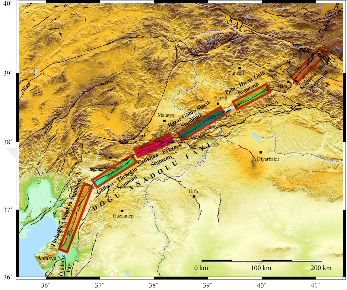
Şekil 4.1 DAF segmentleri ([151]'dan yararlanılarak çizilmiştir)
