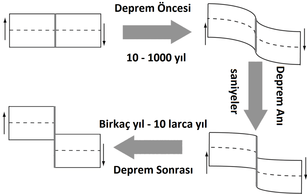
Şekil 2.1 Deprem döngüsünün doğrultu atımlı faylarda klasik gösterimi [50]
