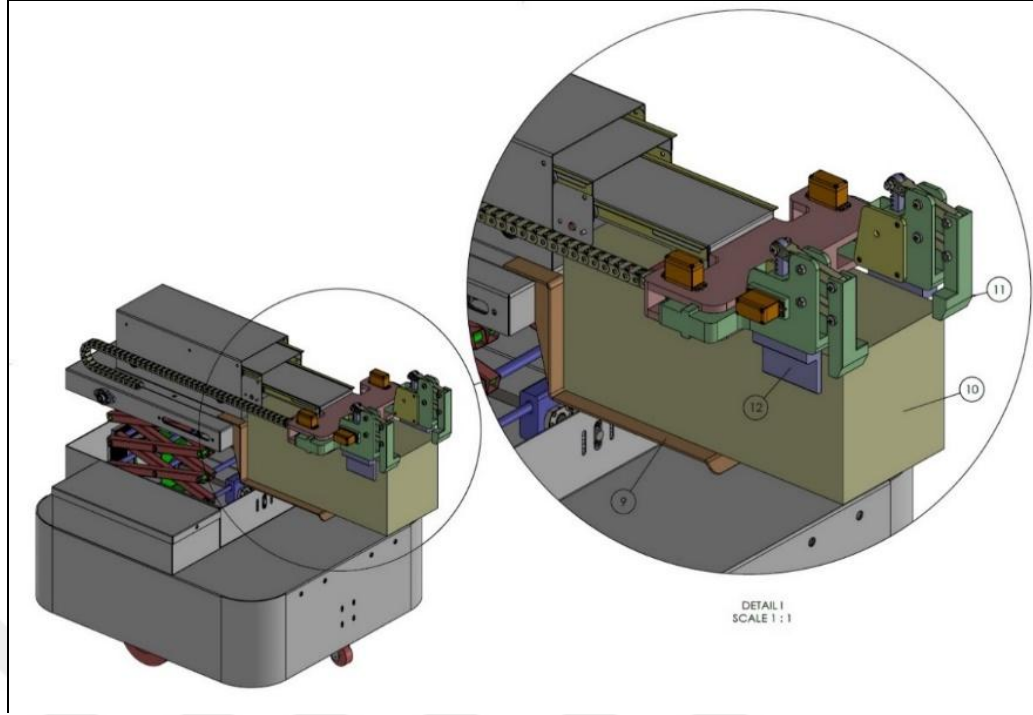
Şekil 3.24: Paralel Çeneli Robotik Tutucunun Hedef Nesneyi Kavrama Uygulaması (9. Ürün tepsisi, 12. Paralel çene, 10. Nesne, 11. Dikey ön çene)
