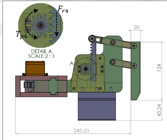
Şekil 3.33: İkinci Robotik Tutucu Tasarımı Dikey Yönde Etkiyen Kuvvetler
