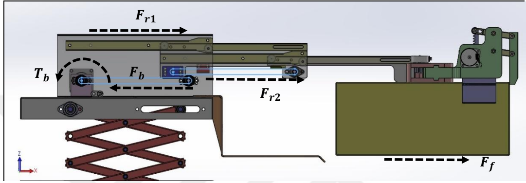
Şekil 3.21: Teleskobik Mekanizmaya Etkiyen Kuvvetler
