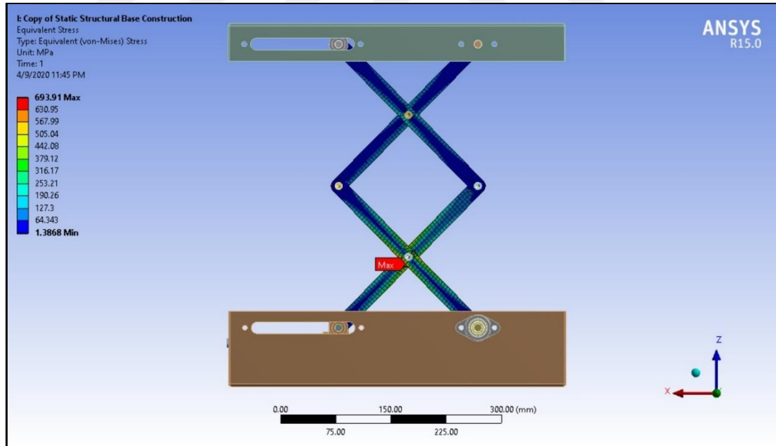
Şekil 5.7: Birinci Makas Tasarımı Statik Yapısal Analizi Sonucu Gerilme Dağılımı
