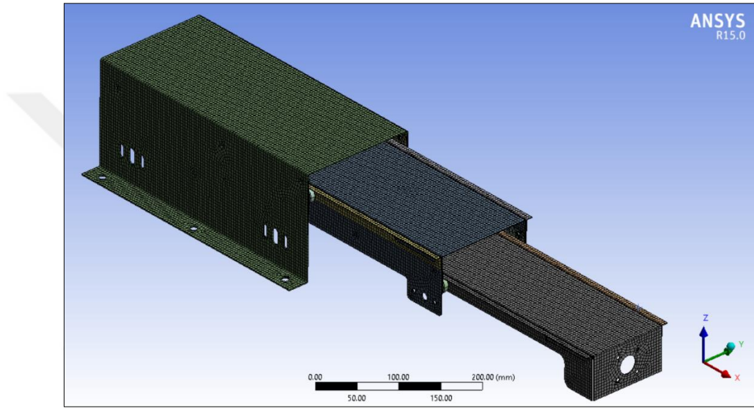
Şekil 5.22: Teleskobik Mekanizmanın Hesaplama Ağı Modeli
