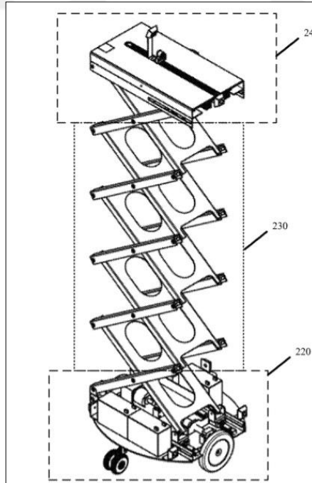
Şekil 2.5: “INVIA” Firmasının Geliştirdiği Mobil Depo Robotunun Genel Mekanik Tasarım Bölümleri [16]
