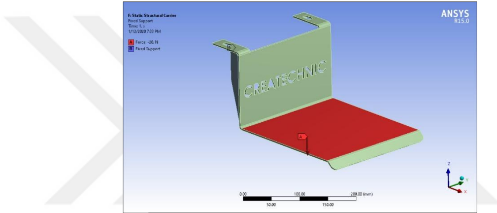
Şekil 5.11: Taşıyıcı Plaka Tasarımının Statik Yapısal Analiz Modeli
