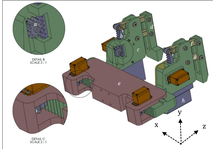
Şekil 3.30: İkinci Robotik Tutucu Tasarımının Alt Komponentleri (a. Çene-1 pinyon dişli, b. Kremayer Dişli, c. Çene-1, d. Çene-2, e. Kılavuz Parça, f. Uzuv-2, g. Uzuv-1, h. Paralel Çene)
