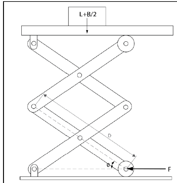
Şekil 3.15: Makaslı Kaldırma Sistemi Serbest Cisim Diyagramı [19]
