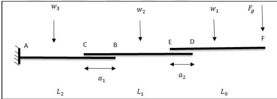
Şekil 5.13: Teleskobik Mekanizma Kesme Kuvveti Diyagramı
