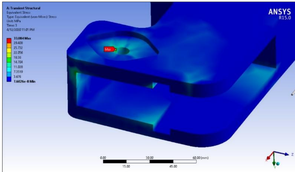
Şekil 5.29: Kılavuzlama Bölgesi Gerilme Dağılımı
