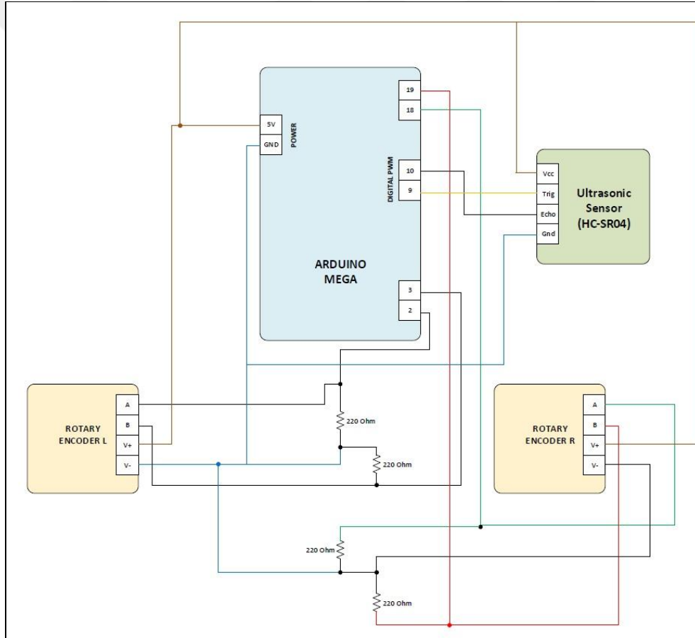
Şekil 3.40: Kontrolcü Kartı Sensör Girişleri Devre Şeması
