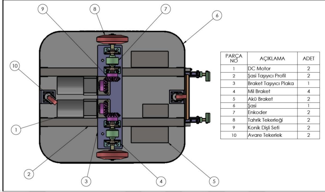
Şekil 3.10: Mekanik Şasi Altan Görünüş
