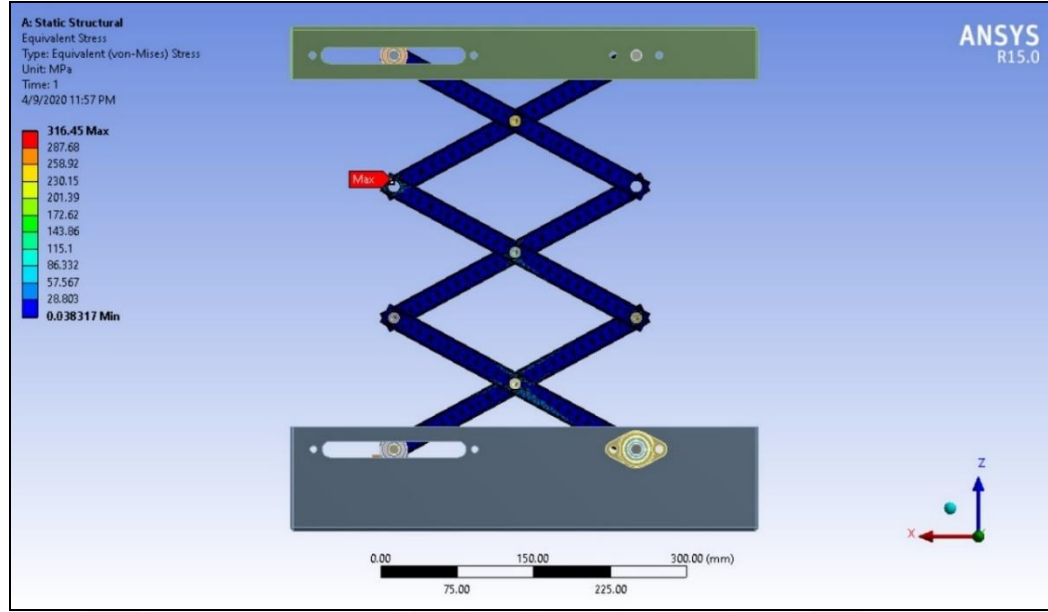
Şekil 5.6: İkinci Makas Tasarımı Statik Yapısal Analizi Sonucu Gerilme Dağılımı
