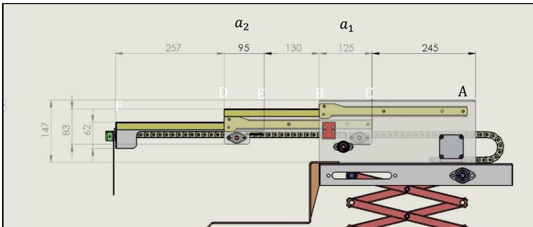
Şekil 5.14: Teleskobik Mekanizma Yandan Görünüş Teknik Resmi
