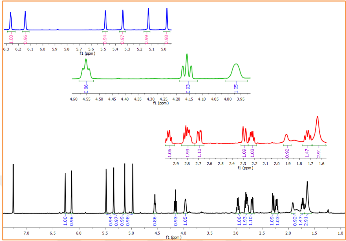
Şekil 4.90 CPGY-11 bileşiğinin (deasilsinaropikrin) 1 H NMR spektrumu (CDCl 3 -d 1 )
