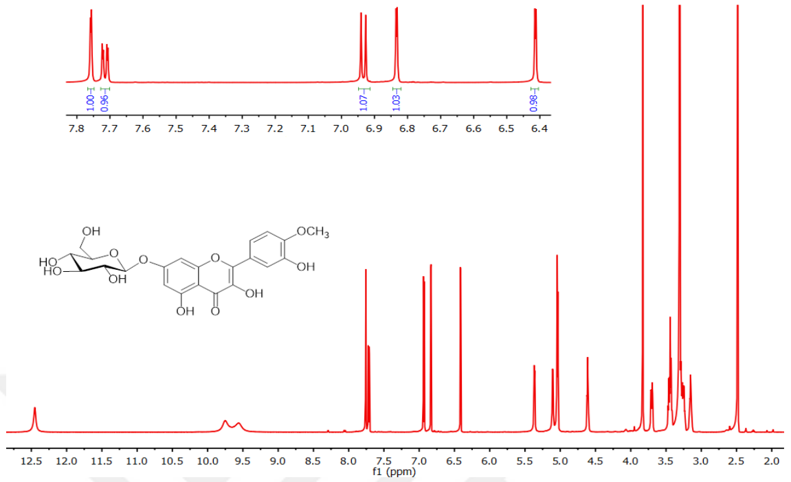
Şekil 4.59 CPC-9 bileşiğinin (Tamariksetin 7-O-β-D glukopiranozit) ^1\text{H} NMR spektrumu ( \text{DMSO-d}_6 )
