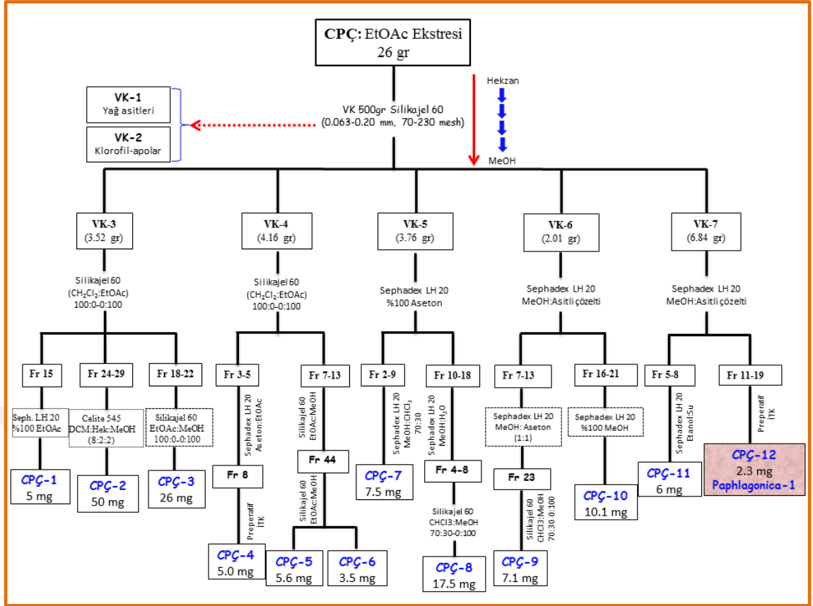
Şekil 3.6 CPÇ (EtOAc ekstresi) izolasyon şeması
