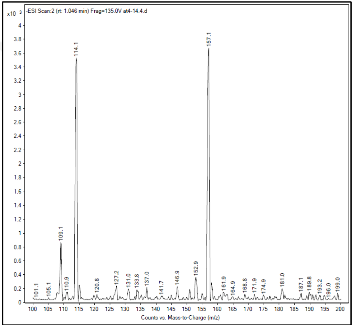
Şekil 4.50 CPC-12 bileşiğinin (Paphlagonica-1) MS spektrumu
