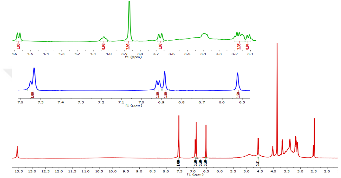
Şekil 3.19 Diosmetin 6-C-β glikozit (CPGY-6) bileşiğinin 1 H NMR spektrumu (DMSO-d 6 )
