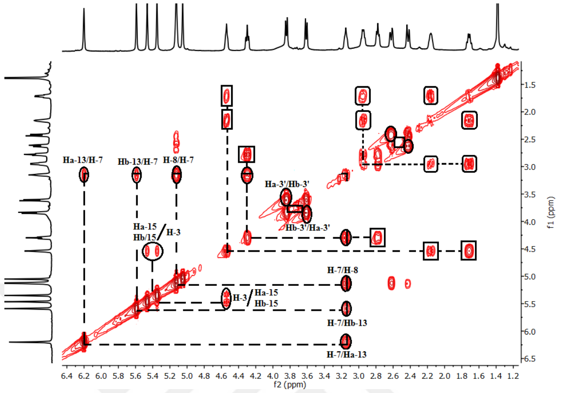
Şekil 4.105 CPGY-12 bileşiğinin [8 \alpha -O-(2',3'-dihidroksiizobutiril) desasiklinaropikrin] ^1\text{H} - ^1\text{H} COSY NMR spektrumu ( \text{CDCl}_3\text{-d}_1 )
