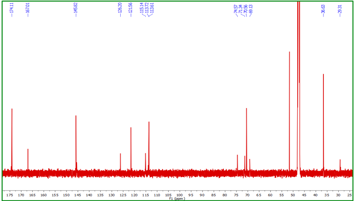
Şekil 2.37 Klorojenik asit metil ester (CPC-6) bileşığının ^{13}\text{C} NMR spektrumu (MeOD- \text{d}_4 )
