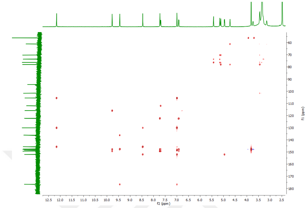
Şekil 3.29 Kuersetagetin-4'-metileter-7-O- \beta glikozit (CPGY-7) bileşiğinin HMBC NMR spektrumu (DMSO-d 6 )
