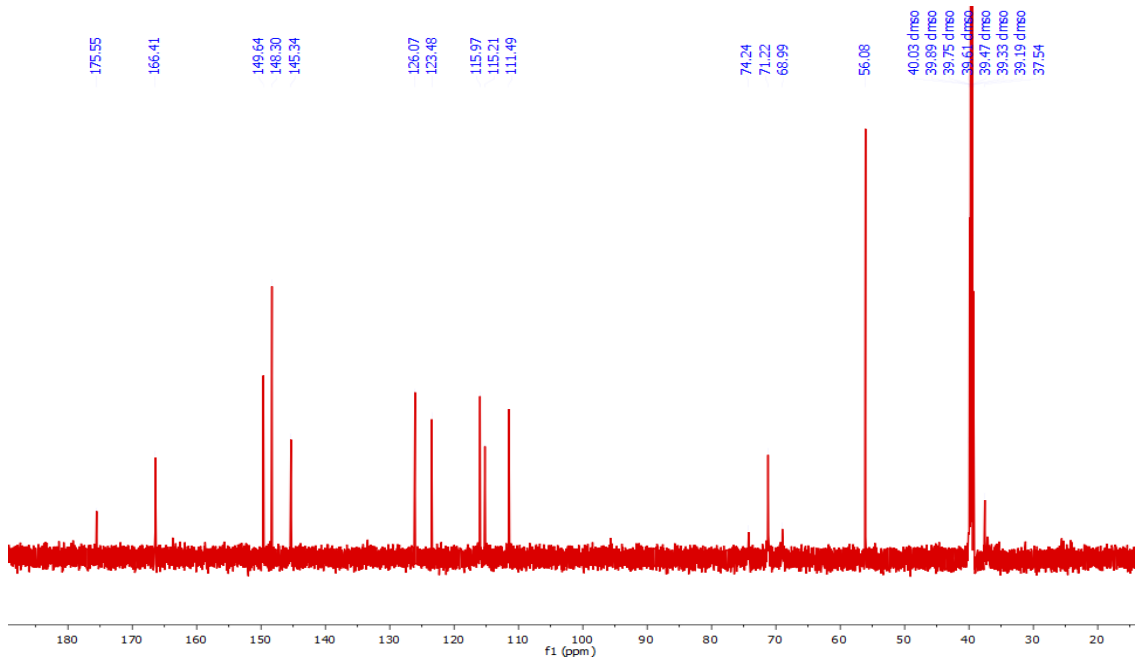
Şekil 3.8 3-O-feruloilkuinik asit (CPGY-4) bileşığının ^{13}\text{C} NMR spektrumu (DMSO- \text{d}_6 )
