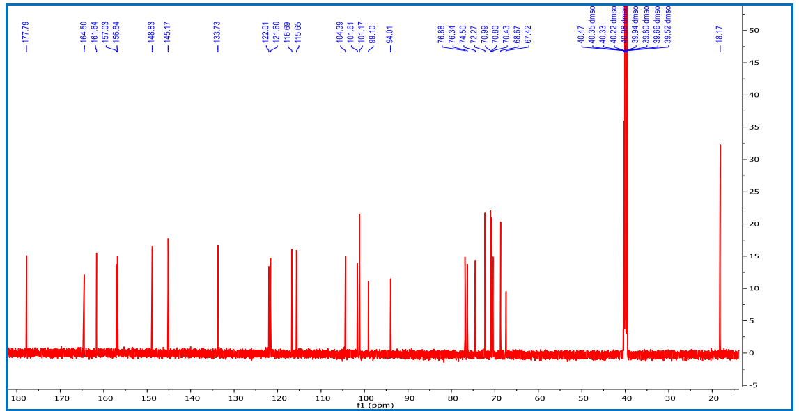
Şekil 2.29 Rutin (CPC-14) molekülünün 13 C NMR spektrumu (DMSO-d 6 )
