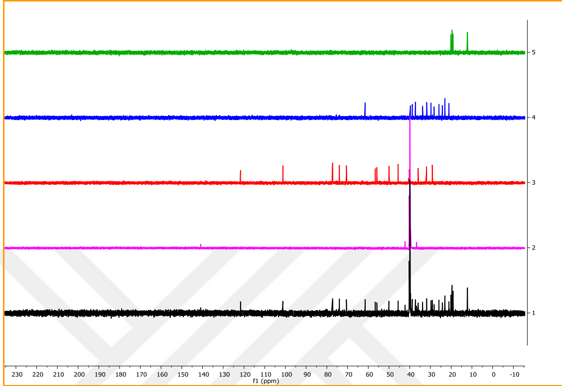
Şekil 2.3 Daucosterin (CPÇ-11) molekülüne ait ^{13}\text{C} DEPT NMR spektrumu (DMSO- \text{d}_6 )
