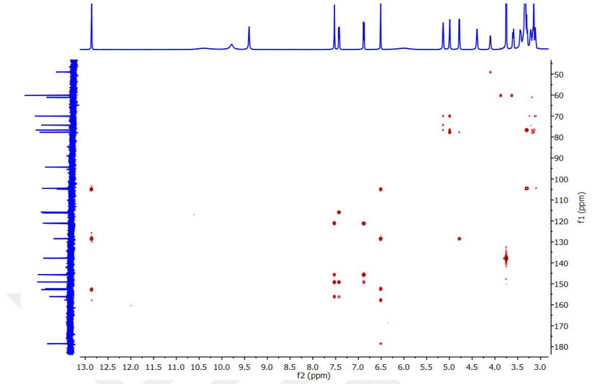
Şekil 3.17 Kuersetagetin-3-metileter-6-O-β-glikopiranozit (CPGY-5) bileşiğinin HMBC NMR spektrumu (DMSO-d 6 )
