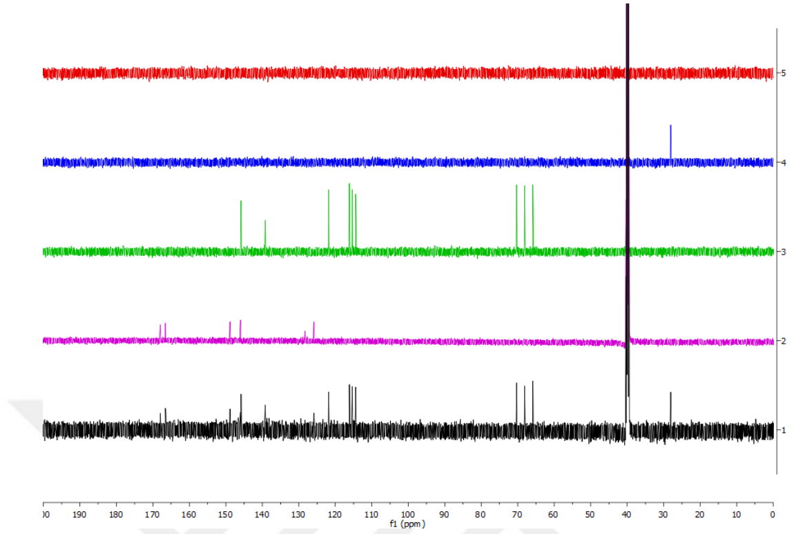
Şekil 2.32 5-O-kafeoil şikimik asit (CPC-4) bileşiğinin ^{13}\text{C} DEPT NMR spektrumu (DMSO- \text{d}_6 )
