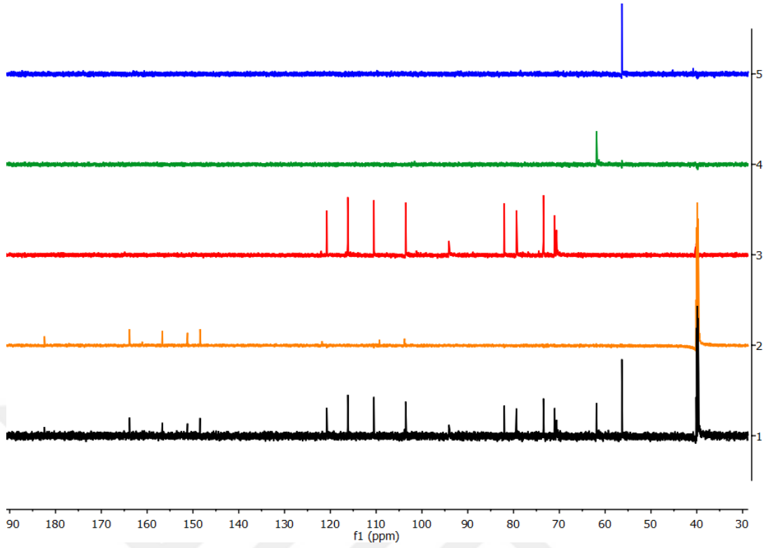
Şekil 3.21 Diosmetin 6-C- \beta glikozit (CPGY-6) bileşiğinin ^{13}\text{C} DEPT NMR spektrumu (DMSO- \text{d}_6 )
