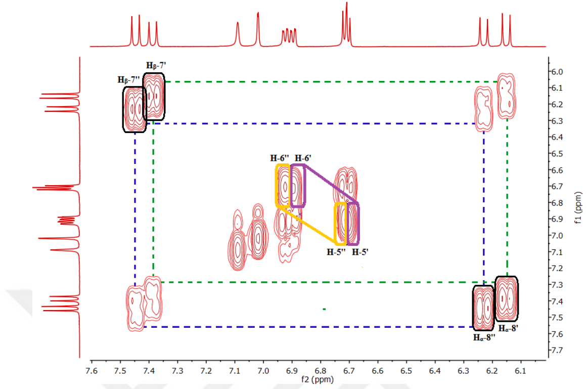
Şekil 4.76 CPC-8 bileşiğinin (1,3-dikafeoilkuinik asit) COSY NMR spektrumu (devam)
