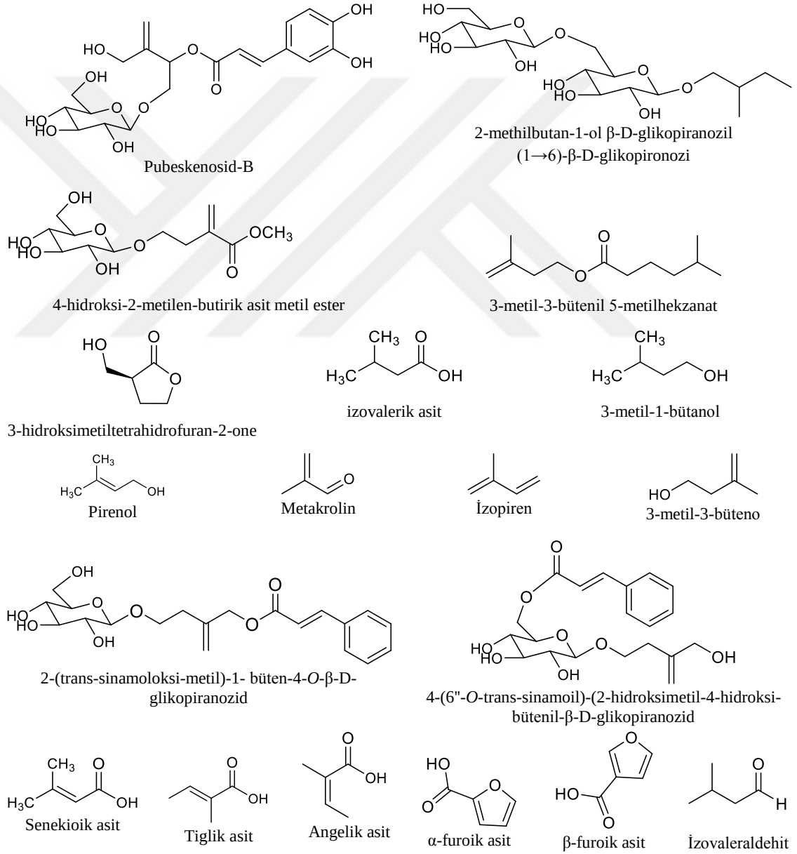
Şekil 2.8 Bazı bitki türlerinden izole edilen hemiterpenoidler
