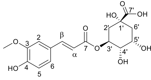
3-O-feruloilkuinik asit (CPGY-4) bileşığının kimyasal yapısı
