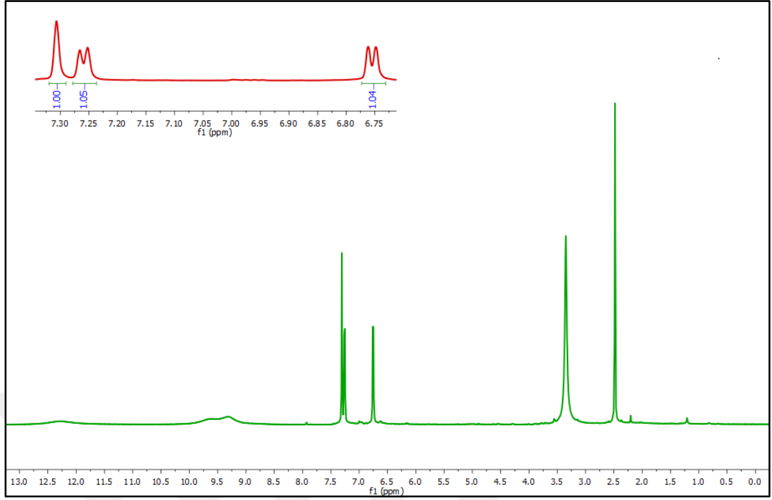
Şekil 1.2 Klorojenik asit (CCGY-2) molekülünün ^1\text{H} -NMR spektrumu ( \text{DMSO-d}_6 )
