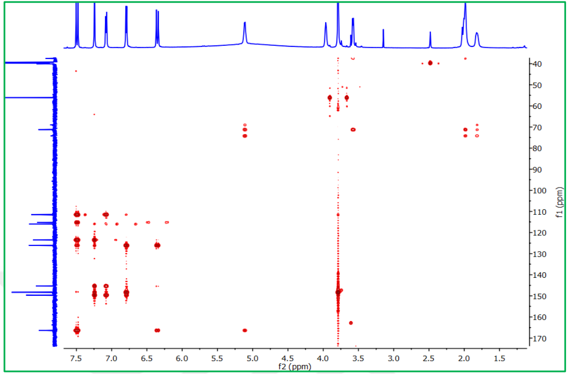
Şekil 3.11 3-O-feruloilkuinik asit (CPGY-4) bileşiğinin HMBC NMR spektrumu (DMSO-d 6 )
