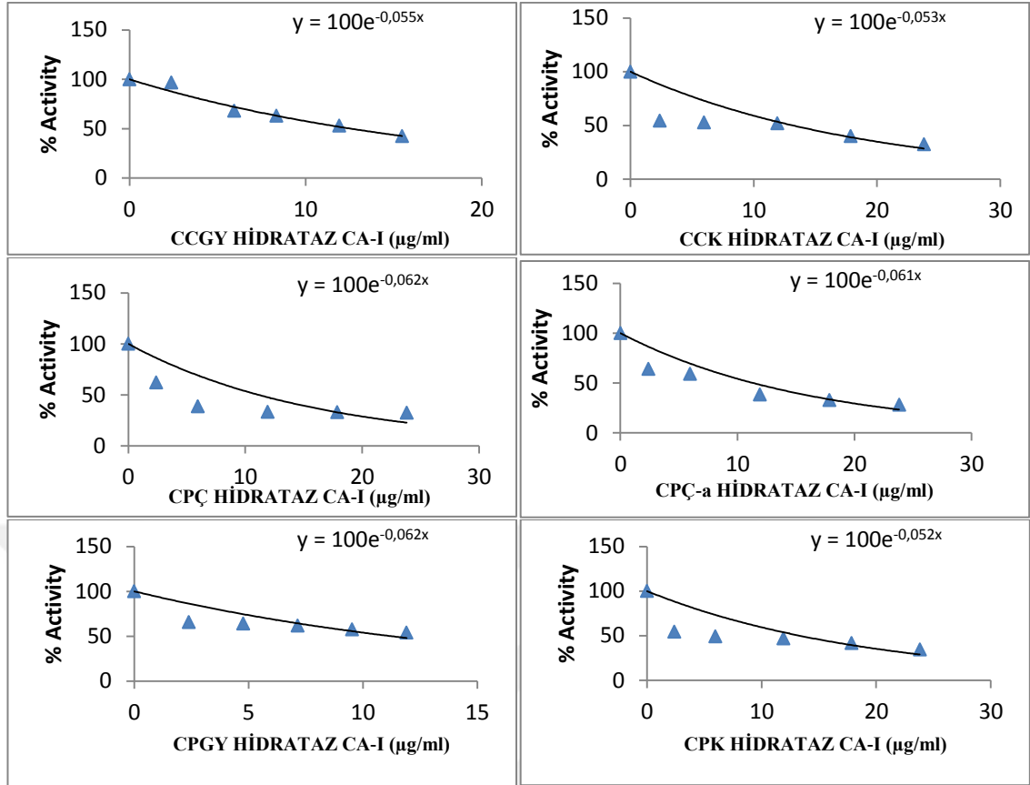
Şekil 4.7 C. paphlagonica ve C. cankiriense bitki ekstralarının CA-I izoenzimine karşı hidrataz aktivitesi grafikleri
