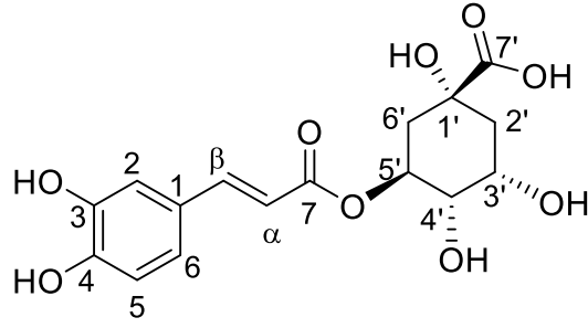
Şekil 4.35 CCGY-2 bileşiğinin (Klorojenik asit) yapısı
