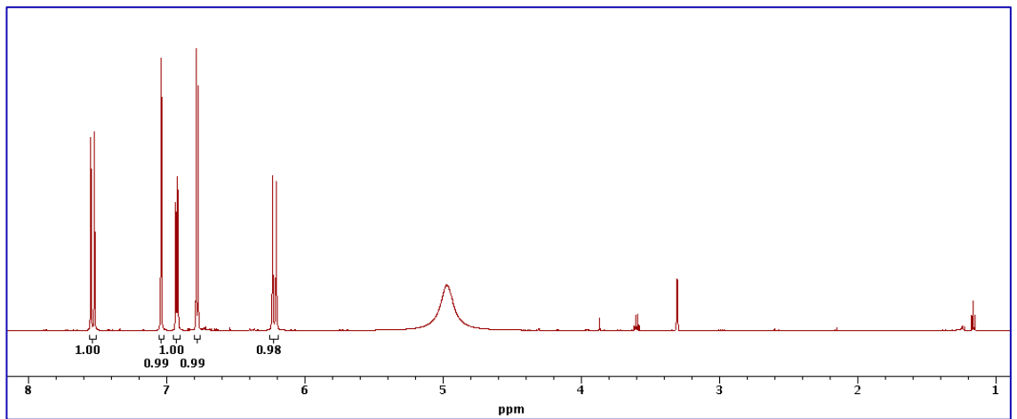
Şekil 4.42 CCGY-4 bileşiğinin (Kafeik asit) ^1\text{H} NMR spektrumu (MeOD- d_4 )
