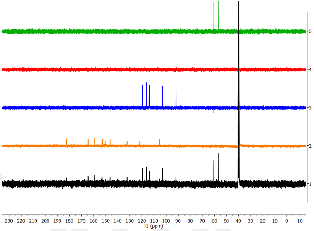
Şekil 3.32 Cirsiliol (CPGY-10) bileşiğinin ^{13}\text{C} DEPT NMR spektrumu (DMSO- \text{d}_6 )
