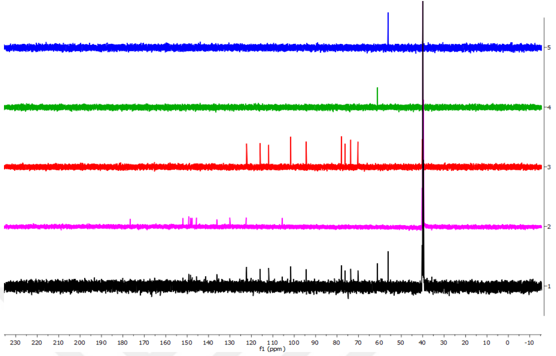
Şekil 3.27 Kuersetagetin-4'-metileter-7-O-β glikozit (CPGY-7) bileşiğinin ^{13}\text{C} DEPT NMR spektrumu (DMSO- \text{d}_6 )
