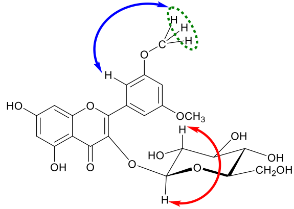
Şekil 4.25 CCGY-5 (Cankiriense-1) bileşiğine ait COSY etkileşimi
