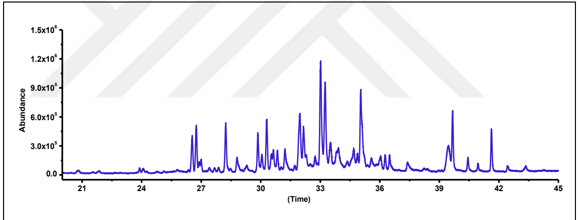
Şekil 4.9 CPÇ bitkisinin uçucu yağ bileşenlerine ait GC-MS kromatogramı
