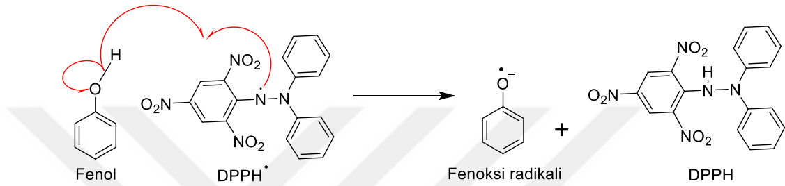
Şekil 3.15 DPPH • radikalinin yapısı ve antioksidan ile verdiği reaksiyon
