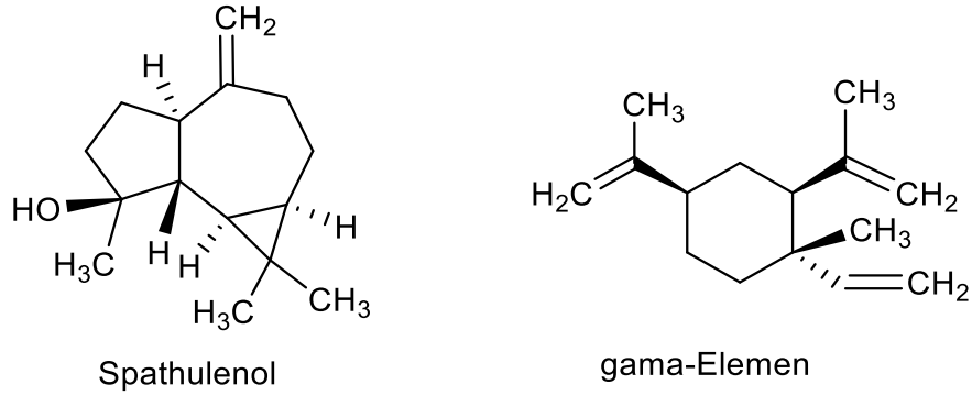
Şekil 4.10 CPÇ bitkisinin uçucu yağ içerisindeki ana bileşenler
