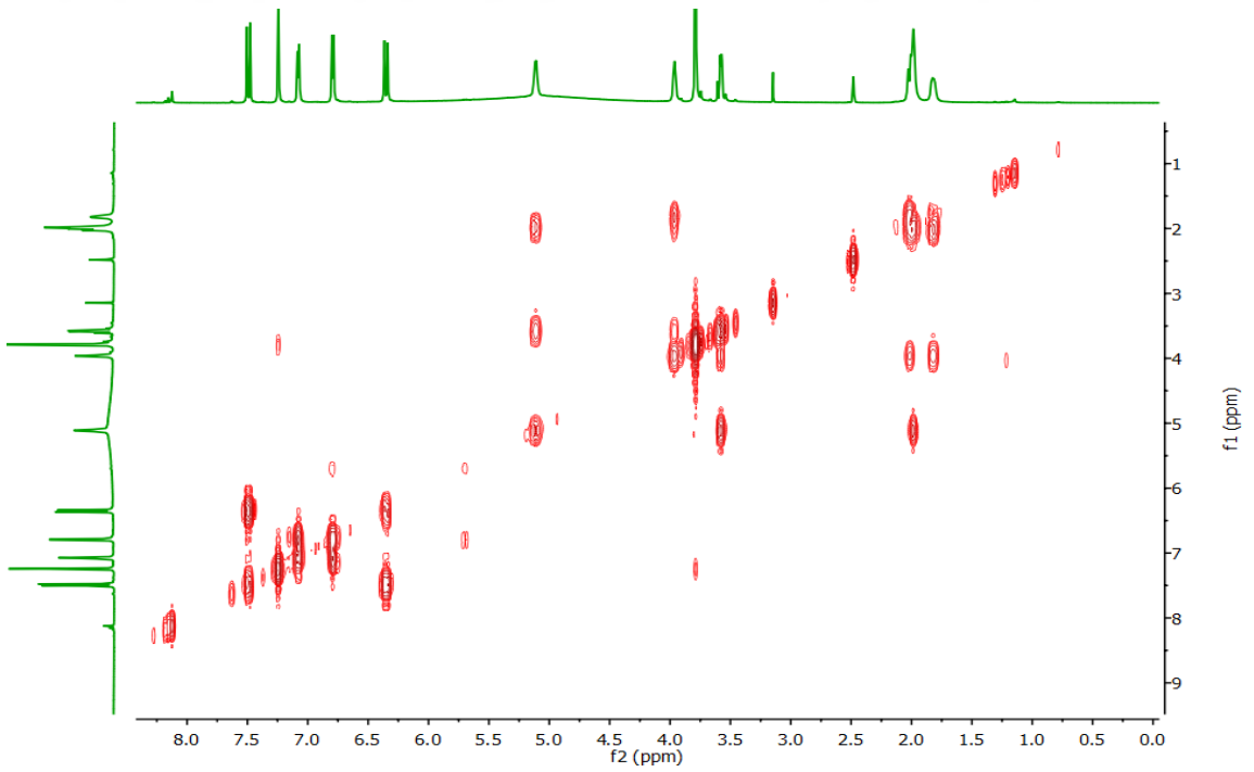
Şekil 3.12 3-O-feruloilkuinik asit (CPGY-4) bileşiğinin COSY NMR spektrumu (DMSO-d 6 )
