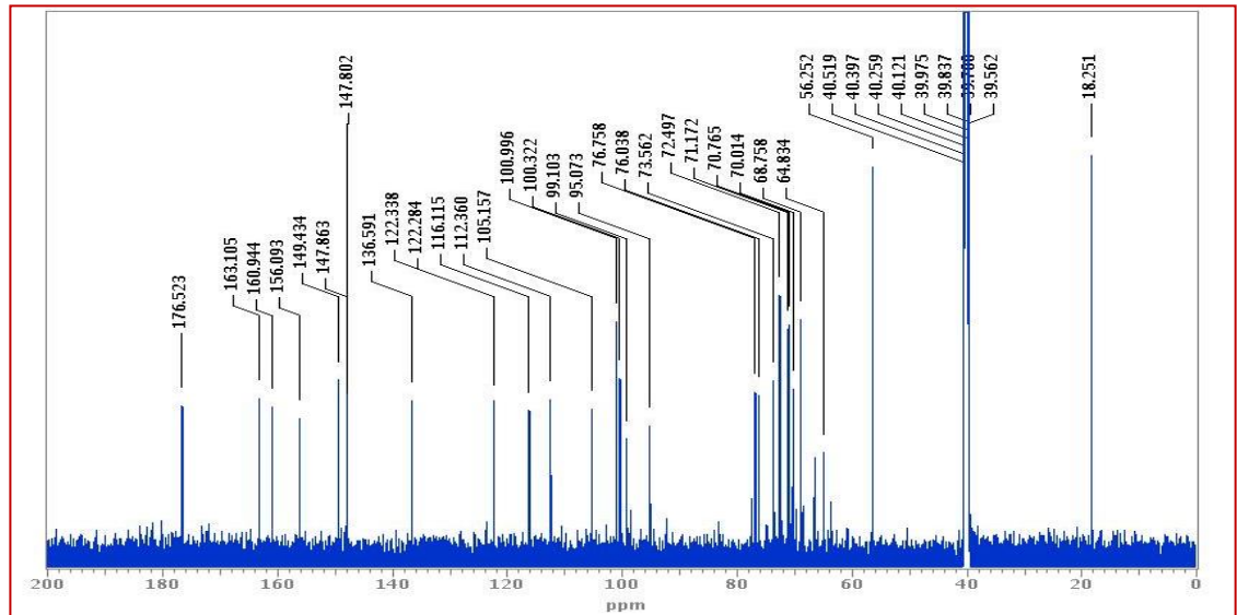
Şekil 2.24 Tamariksetin 7-O-β rutinozid (CPÇ-13) molekülünün ^{13}\text{C} NMR spektrumu (DMSO- \text{d}_6 )
