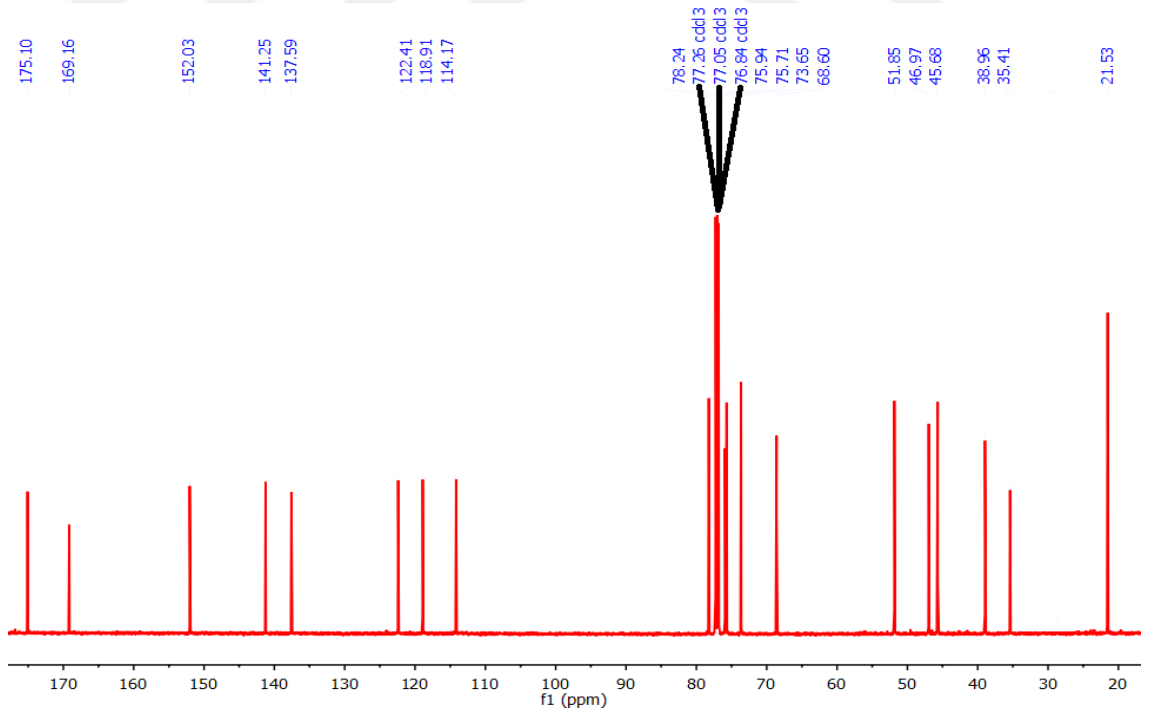
Şekil 4.100 CPGY-12 bileşiğinin [8 \alpha -O-(2',3'-dihidroksiizobutiril) desasiklinaropikrin] 13 C NMR spektrumu (CDCl 3 -d 1 )
