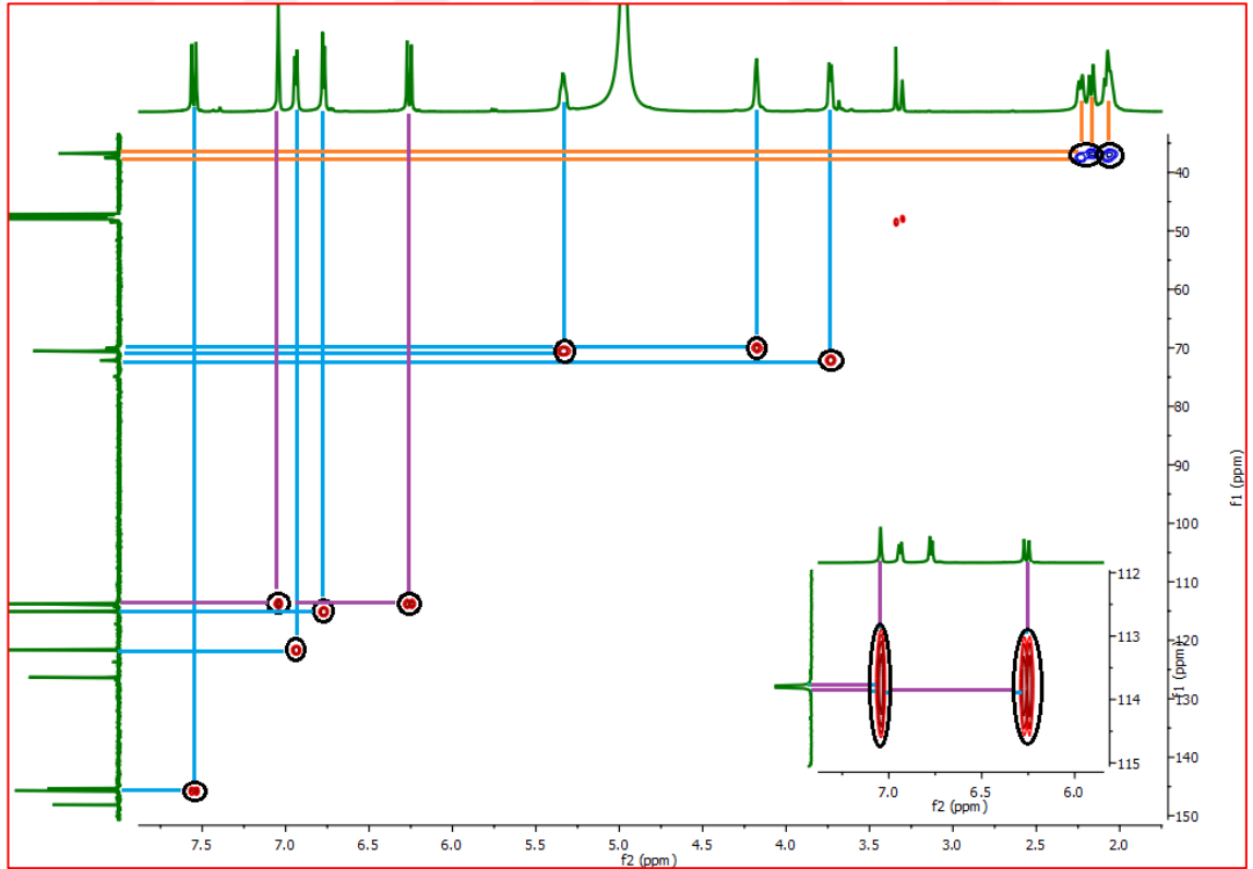
Şekil 4.39 CCGY-2 bileşiğinin (Klorojenik asit) HSQC NMR spektrumu (MeOD- d_4 )
