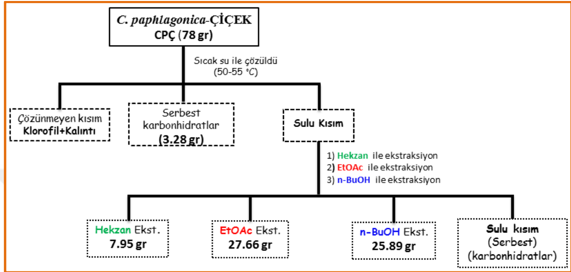
Şekil 3.3 CPÇ ekstraktlarının elde edilme şeması
