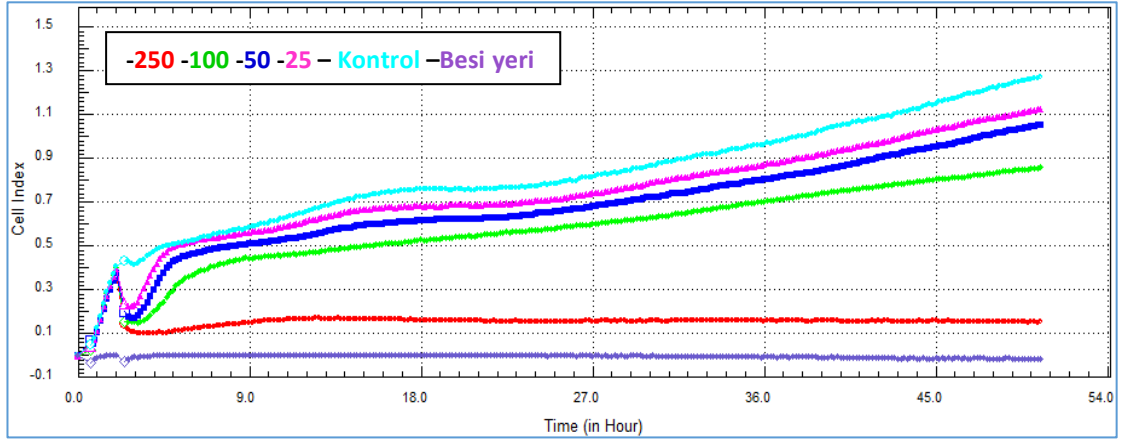
Şekil 4.1 CCÇ ekstresinin HeLa hücrelerine karşı antiproliferatif aktivite grafiği
