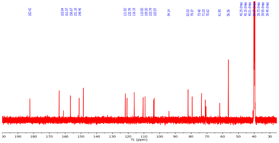
Şekil 3.20 Diosmetin 6-C-β glikozit (CPGY-6) bileşiğinin 13 C NMR spektrumu (DMSO-d 6 )
