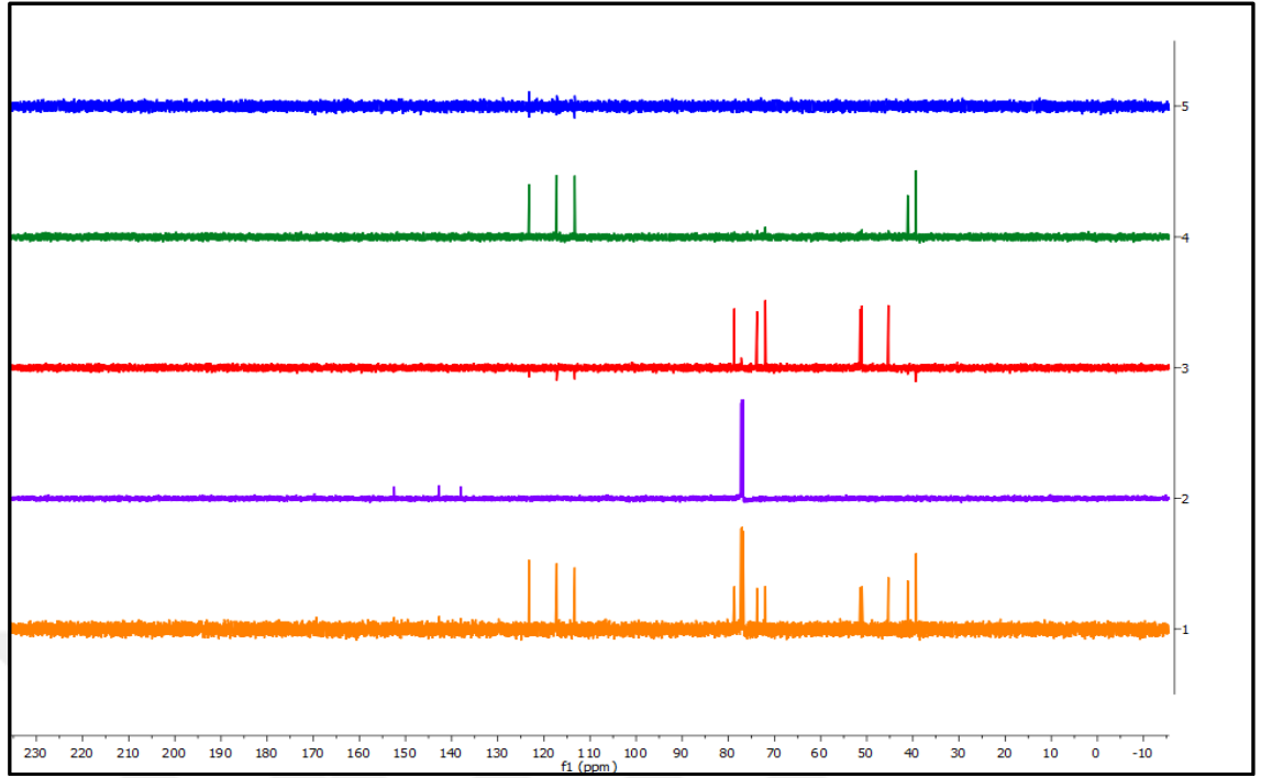
Şekil 4.92 CPGY-11 bileşiğinin (deasilsinaropikrin) ^{13}\text{C} DEPT NMR spektrumu ( \text{CDCl}_3 )
