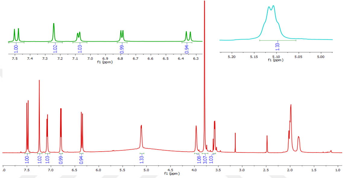
Şekil 3.7 3-O-feruloilkuinik asit (CPGY-4) bileşığının ^1\text{H} NMR spektrumu (DMSO- \text{d}_6 )
