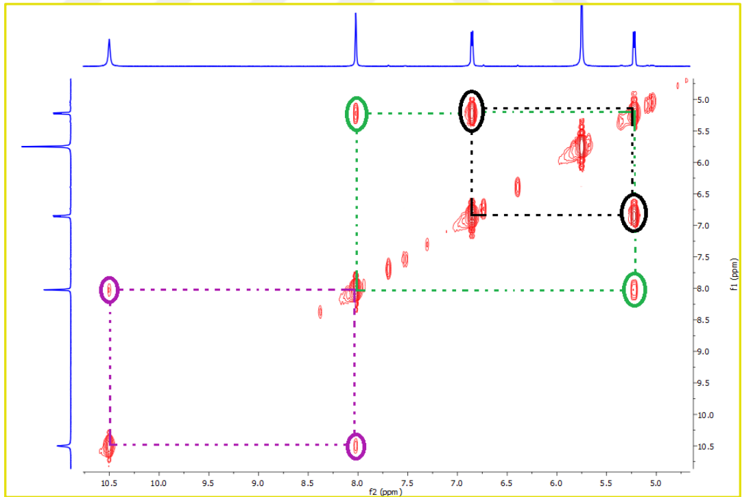
Şekil 4.57 CPC-12 bileşiğinin (5-amino-1-diazenil-3,4-dihidroksi-1,5-dihidro-2H-pirol-2-on) COSY NMR spektrumu (DMSO-d 6 )
