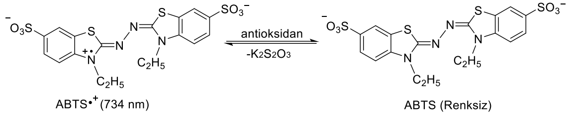
Şekil 3.16 \text{ABTS}^{\bullet+} radikalinin yapısı ve antioksidan ile verdiği reaksiyon
