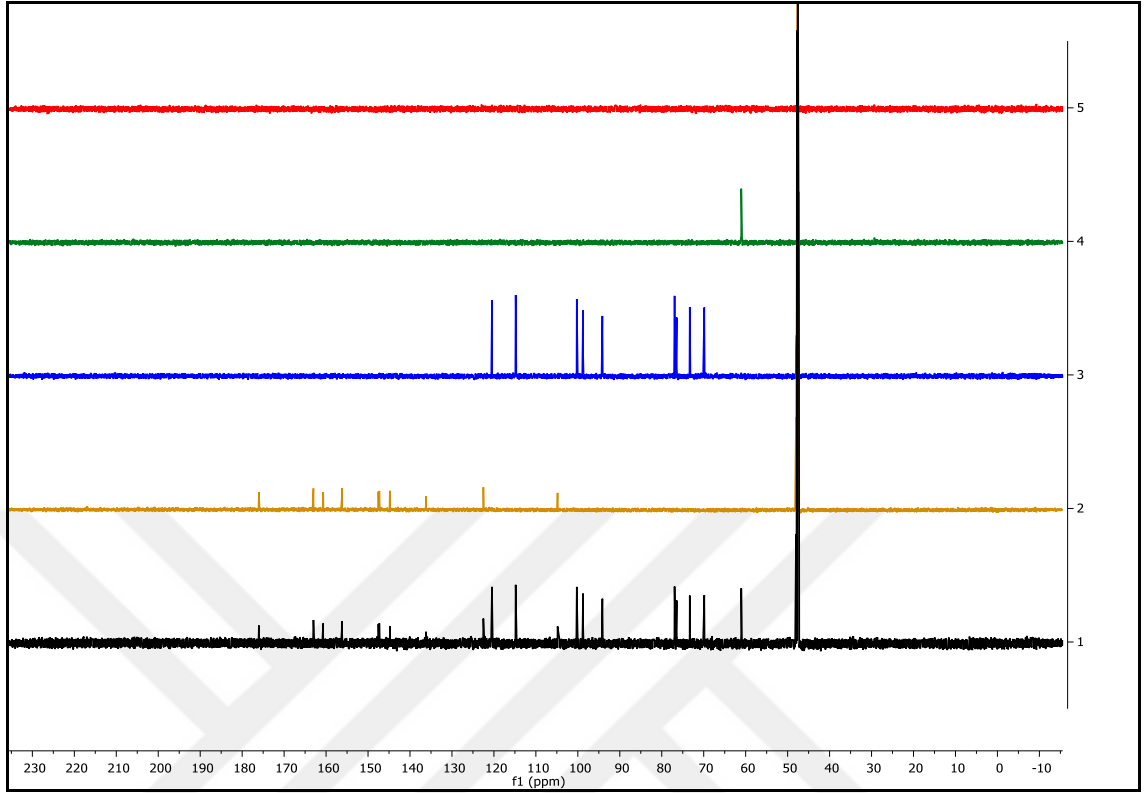
Şekil 2.7 Kuersimetrin (CPÇ-10) molekülüne ait ^{13}\text{C} DEPT NMR spektrumu (MeOD- \text{d}_4 )
