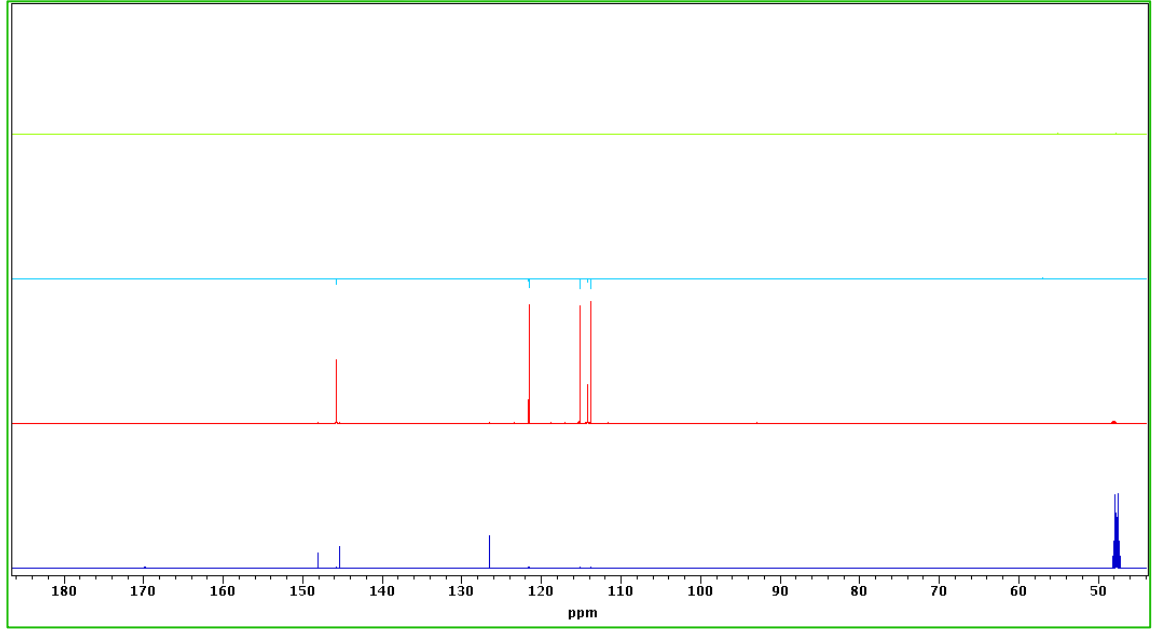
Şekil 4.44 CCGY-4 bileşiğinin (Kafeik asit) DEPT NMR spektrumu (MeOD- d_4 )
