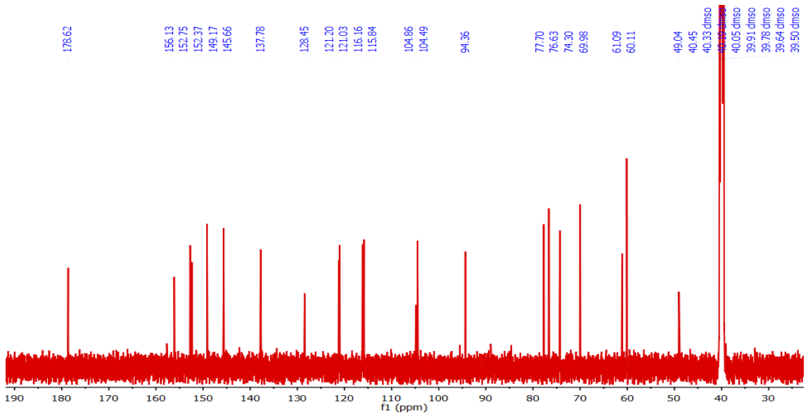
Şekil 3.14 Kuersetagetin-3-metileter-6-O-β-glikopiranozit (CPGY-5) bileşiğinin 13 C NMR spektrumu (DMSO-d 6 )
