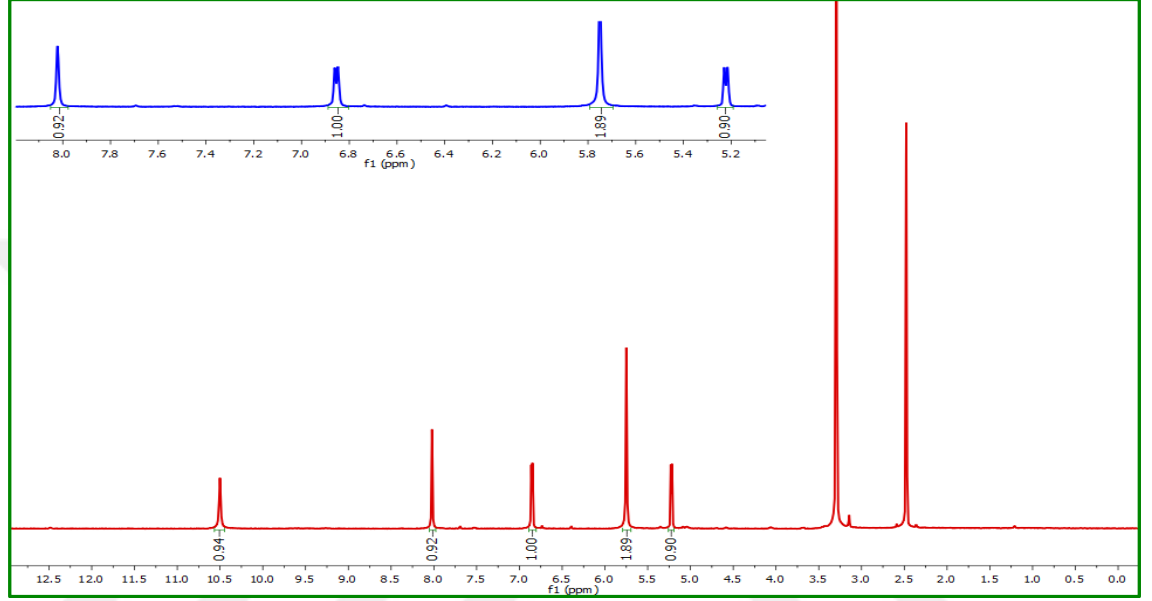
Şekil 4.52 CPC-12 bileşiğinin (5-amino-1-diazenil-3,4-dihidroksi-1,5-dihidro-2H-pirol-2-on) 1 H NMR spektrumu (DMSO-d 6 )
