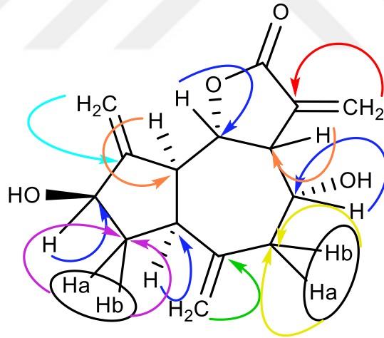
Şekil 4.93 CPGY-11 bileşiğinin HSQC etkileşimleri
