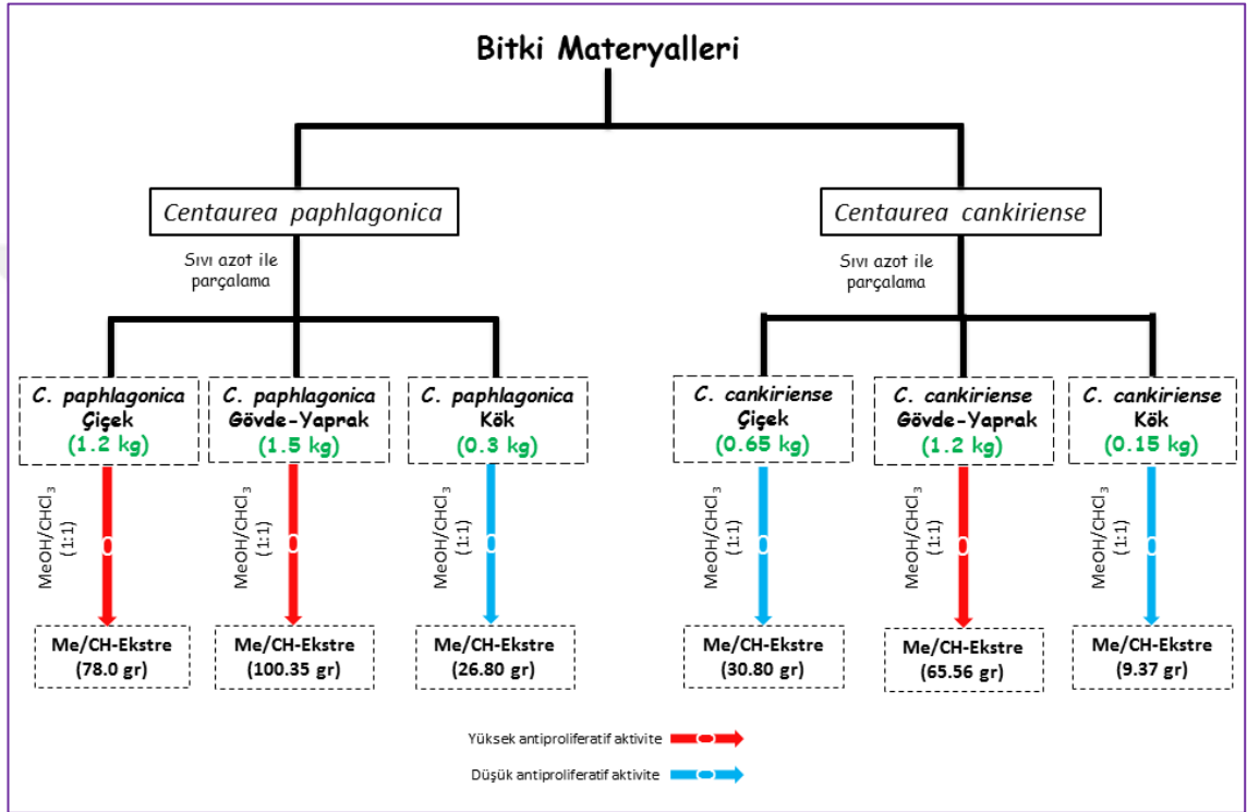
Şekil 3.2 Bitki materyallerinden ham ekstrelerin elde edilme şeması
