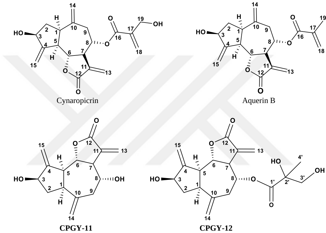
Şekil 5.1 İzole edilen bazı seskiterpen laktonların
