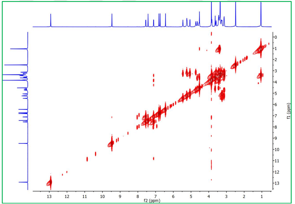
Şekil 1.29 Diosmin (CCGY-8) molekülüne ait COSY NMR spektrumu (DMSO-d 6 )
