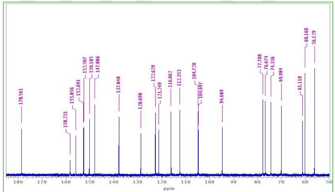
Şekil 4.82 CPGY-8 bileşiğinin (Paphlagonica-2) 13 C NMR spektrumu (DMSO-d 6 )
