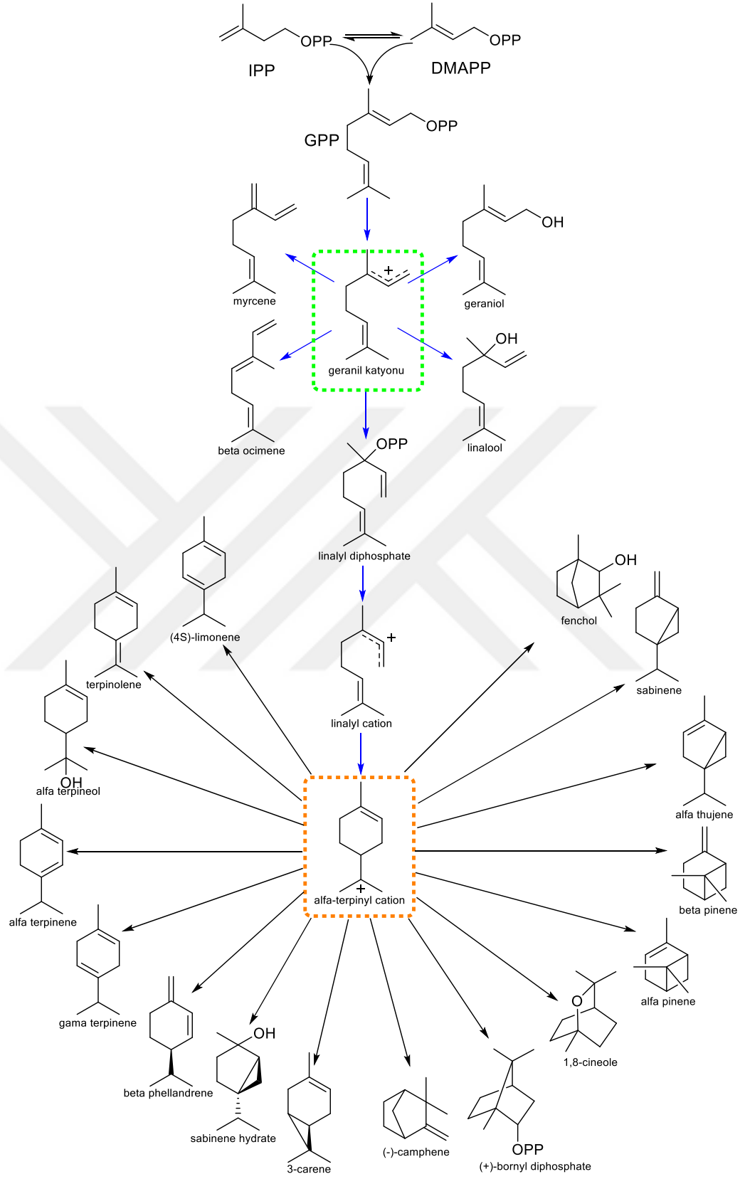
Şekil 2.9 Monoterpenlerin (monoterpenoid) biyosentezi ve bazı monoterpenler (Ignea et al. 2019, Ramak et al. 2014, Zebec et al. 2016)
