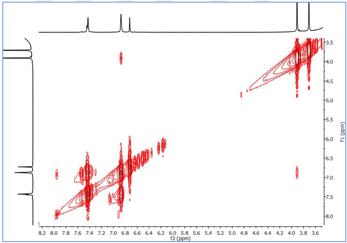
Şekil 3.35 Cirsiliol (CPGY-10) bileşiğinin COSY NMR spektrumu (DMSO-d 6 )
