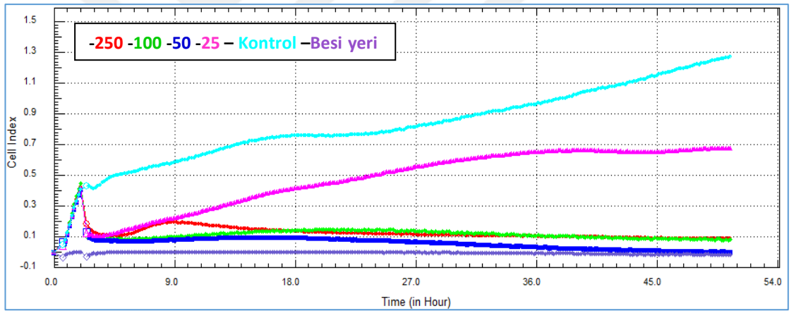
Şekil 4.2 CCGY ekstresinin HeLa hücrelerine karşı antiproliferatif aktivite grafiği
