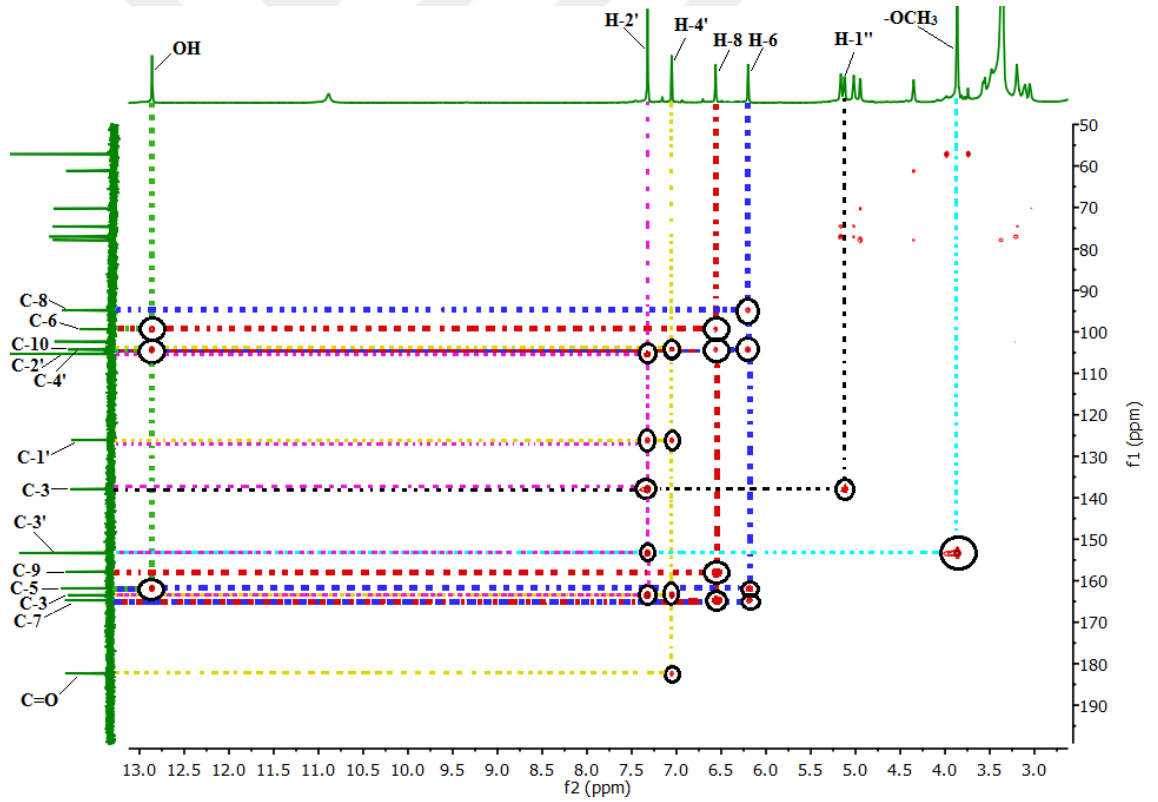
Şekil 4.24 CCGY-5 (Cankiriense-1) bileşiğinin HMBC NMR spektrumu (DMSO- d_6 )
