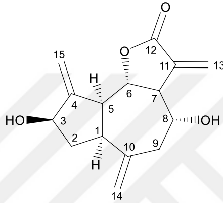
Şekil 4.89 CPGY-11 bileşiđinin (deasilsinaropikrin) kimyasal yapısı
