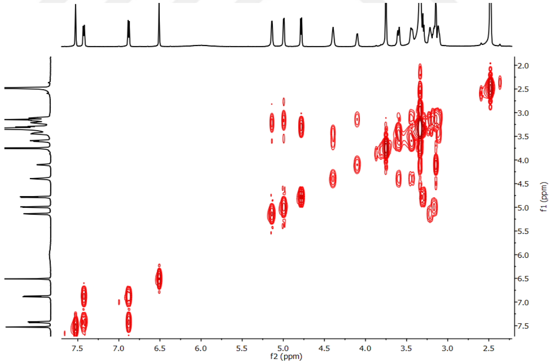
Şekil 3.18 Kuersetagetin-3-metileter-6-O-β-glikopiranozit (CPGY-5) bileşiğinin COSY NMR spektrumu (DMSO-d 6 )
