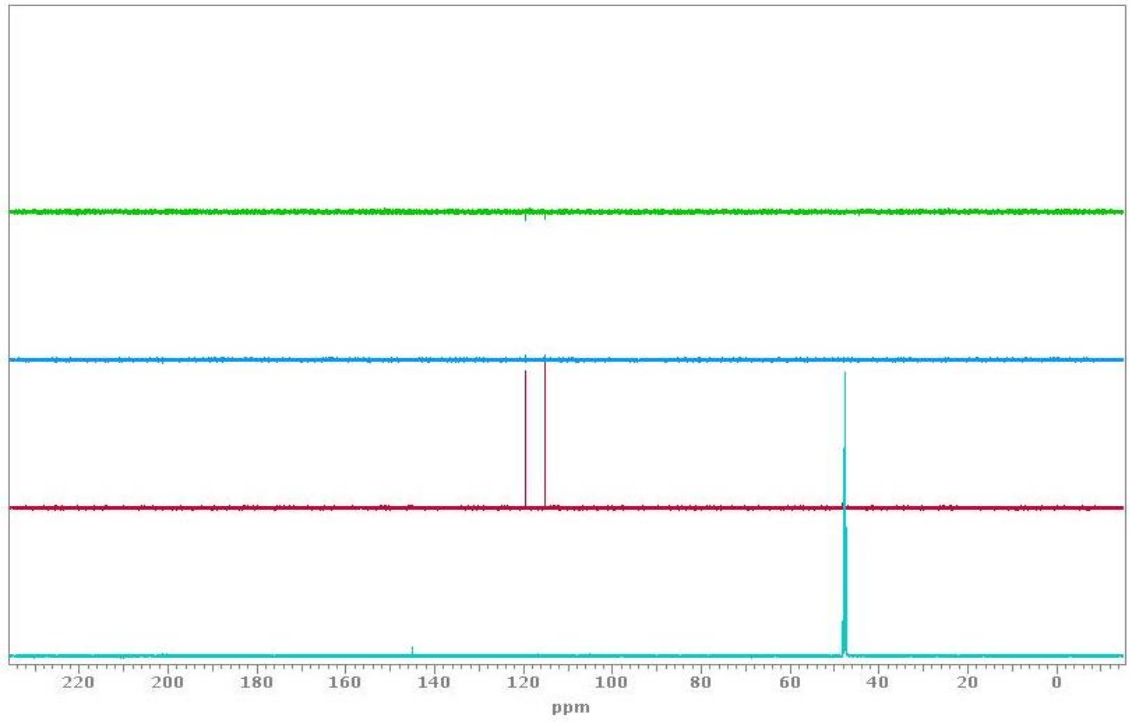
Şekil 2.40 Pirokateşol (CPÇ-1) bileşiğinin ^{13}\text{C} DEPT NMR spektrumu (MeOD- \text{d}_4 )
