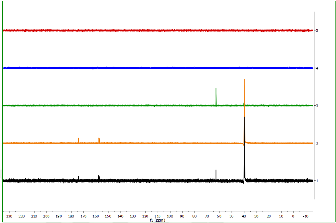
Şekil 4.54 CPC-12 bileşiğinin (5-amino-1-diazenil-3,4-dihidroksi-1,5-dihidro-2H-pirol-2-on) ^{13}\text{C} DEPT NMR spektrumu (DMSO- \text{d}_6 )
