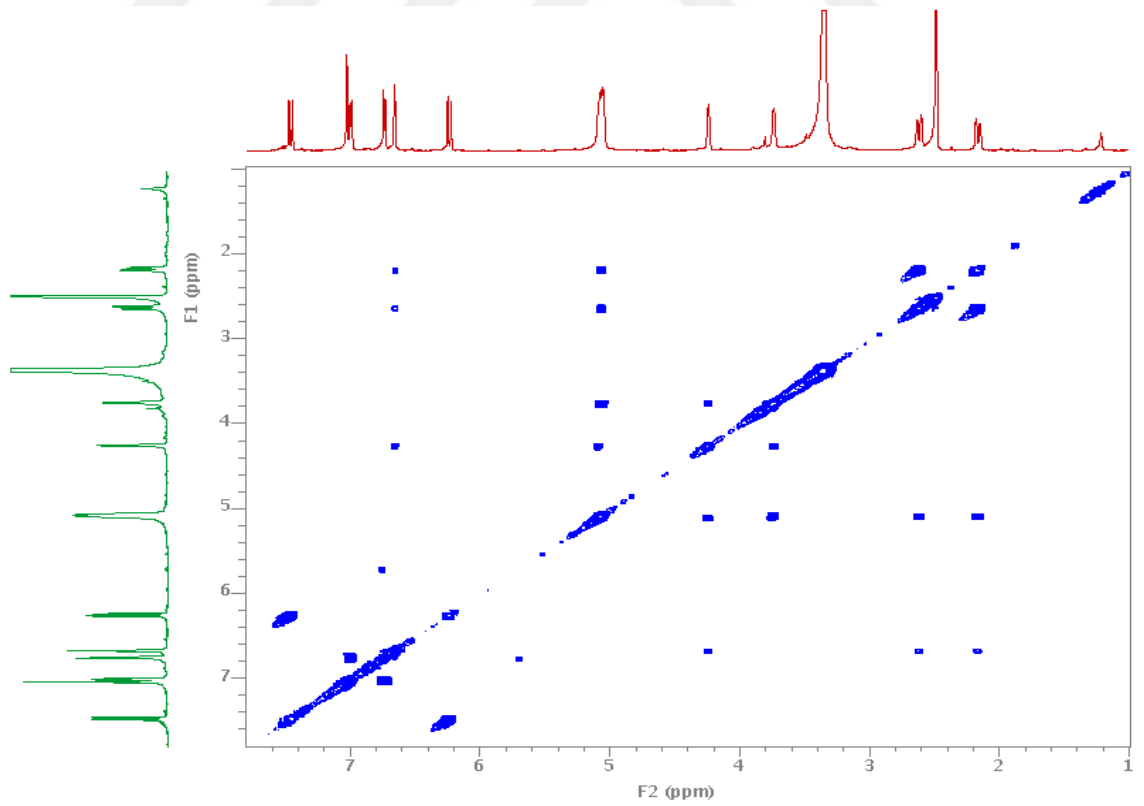
Şekil 2.35 5-O-kafeoil şikimik asit (CPC-4) bileşiğinin COSY NMR spektrumu (DMSO-d 6 )
