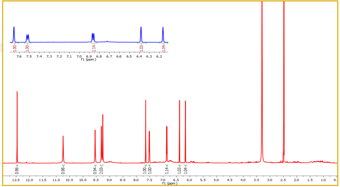
Şekil 2.11 Kuersetin (CPC-7) molekülüne ait ^1\text{H} NMR spektrumu
