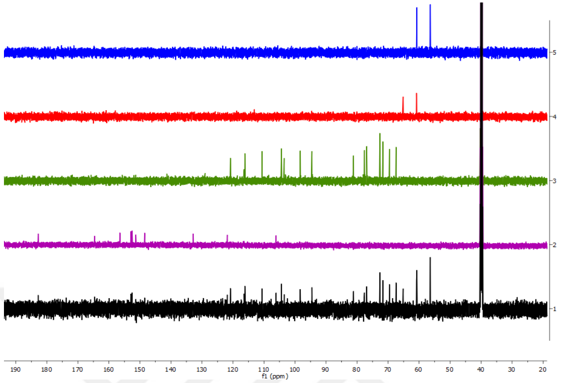
Şekil 4.32 CCGY-9 bileşiğinin (Cankiriense-2) ^{13}\text{C} DEPT NMR spektrumu ( \text{DMSO}-d_6 )
