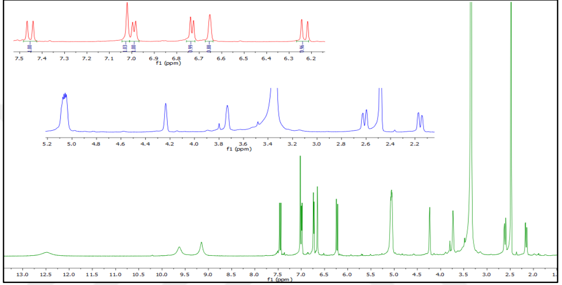
Şekil 2.30 5-O-kafeoil şikimik asit (CPC-4) bileşığının 1 H NMR spektrumu (DMSO-d 6 )
