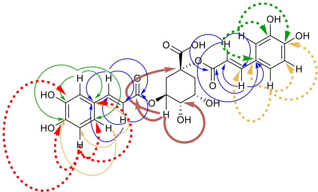
Şekil 4.73 CPC-8 bileşiğinin (1,3-dikafeoilkuinik asit) HMBC etkileşimi
