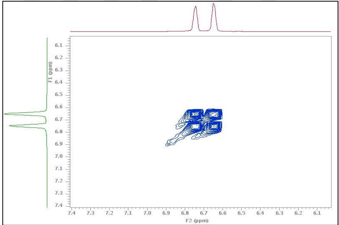
Şekil 2.43 Pirokateşol (CPC-1) bileşiğinin COSY NMR spektrumu (MeOD-d 4 )
