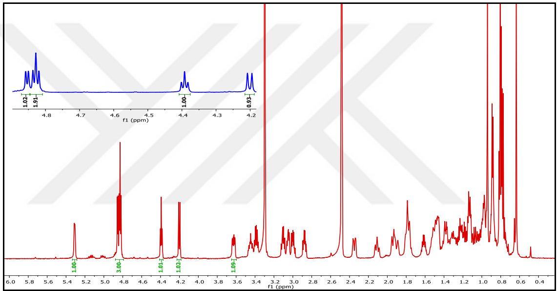
Şekil 2.1 Daucosterin (CPC-11) molekülüne ait ^1\text{H} NMR spektrumu (DMSO- d_6 )
