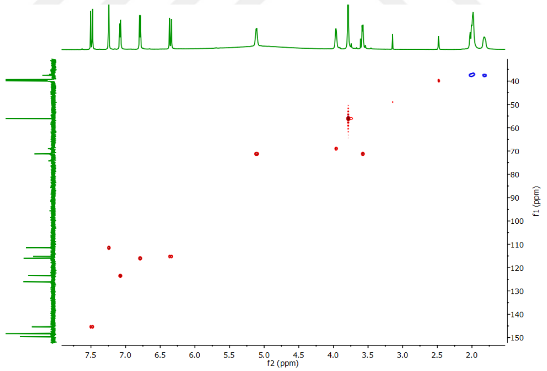
Şekil 3.10 3-O-feruloilkuinik asit (CPGY-4) bileşiğinin HSQC NMR spektrumu (DMSO- \text{d}_6 )
