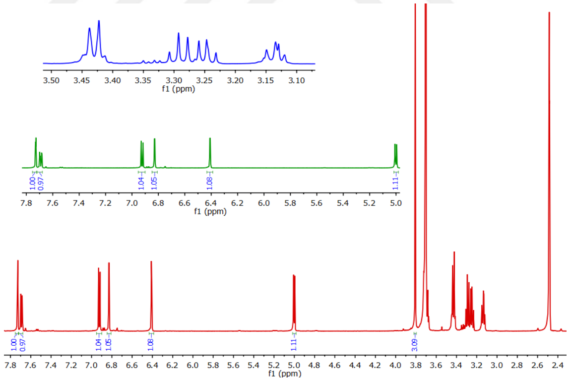
Şekil 4.60 CPC-9 bileşiğinin (Tamariksetin 7-O-β-D glukopiranozit) ^1\text{H} NMR spektrumu ( \text{D}_2\text{O} ilavesi ile)
