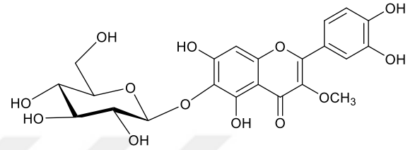
CPGY-5 Kuersetagetin-3-metileter-6-O- \beta -glikopiranozit
