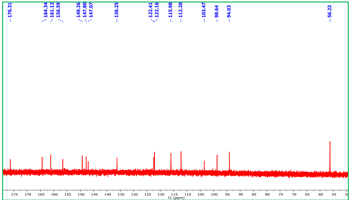
Şekil 2.18 Tamariksetin (CPÇ-5) molekülüne ait ^{13}\text{C} NMR spektrumu (DMSO- \text{d}_6 )
