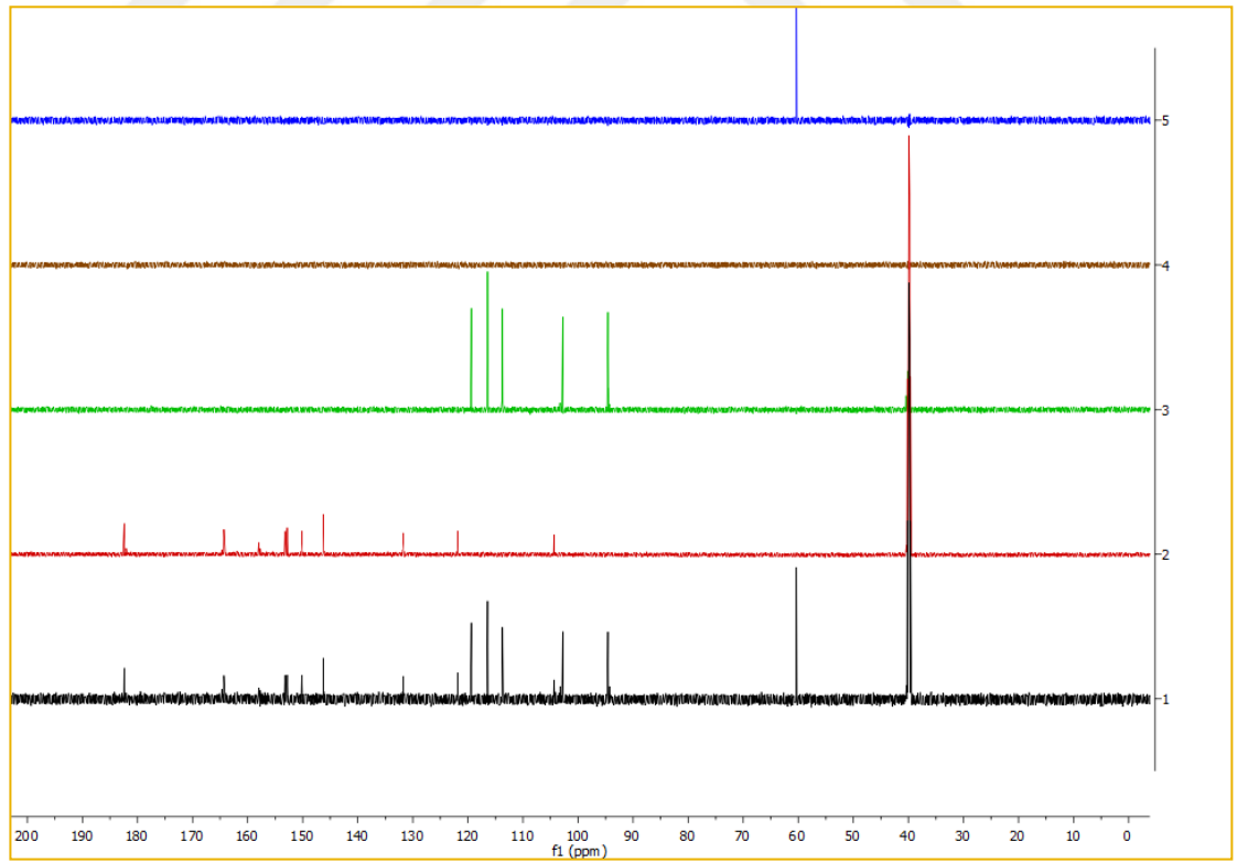
Şekil 1.19 Nepetin (CCGY-7) molekülüne ait ^{13}\text{C} DEPT NMR spektrumu (DMSO- \text{d}_6 )
