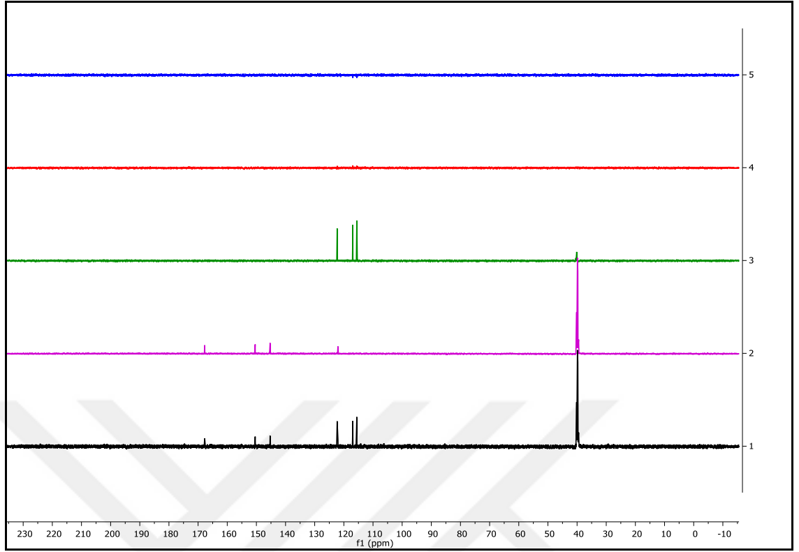
Şekil 1.6 Klorojenik asit (CCGY-2) molekülünün DEPT spektrumu (DMSO-d 6 )
