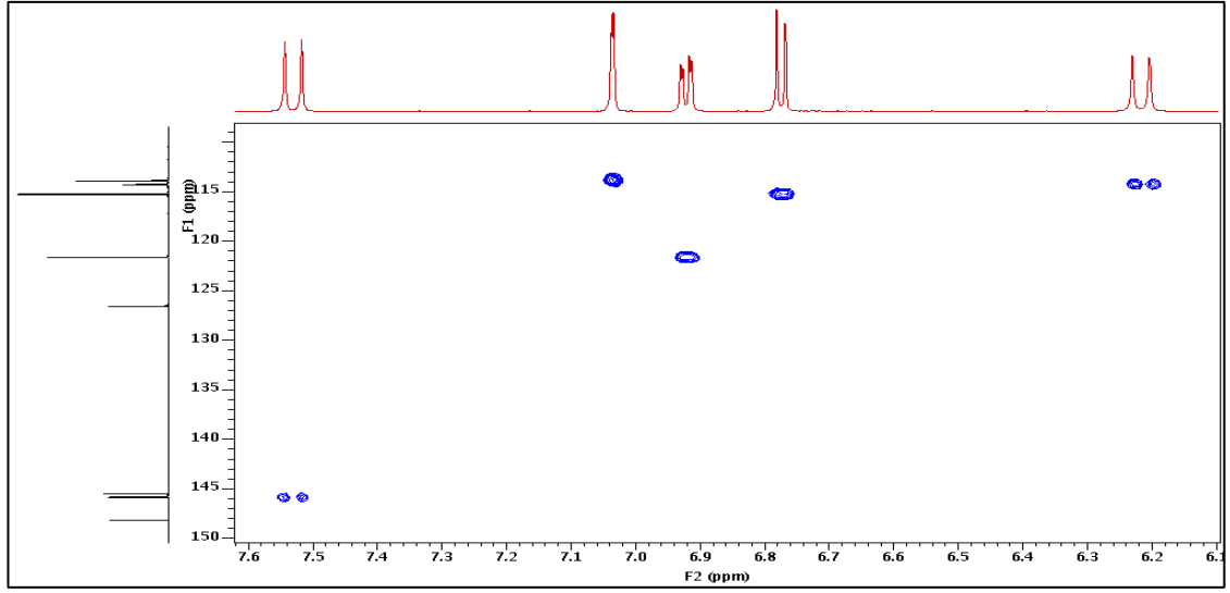
Şekil 4.45 CCGY-4 bileşiğinin (Kafeik asit) HSQC NMR spektrumu (MeOD- d_4 )
