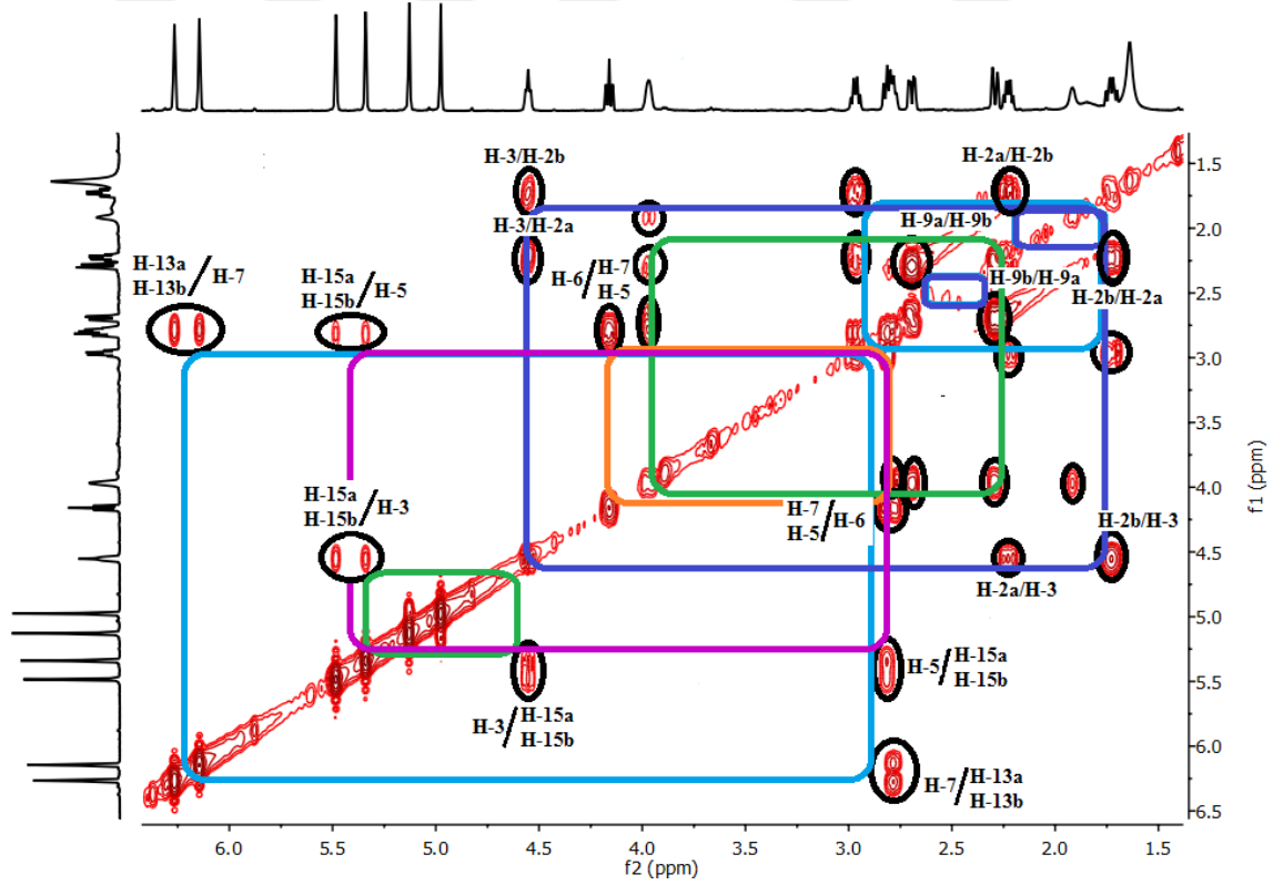
Şekil 4.97 CPGY-11 bileşiğinin (deasilinaropikrin) COSY NMR spektrumu ( \text{CDCl}_3\text{-d}_1 )
