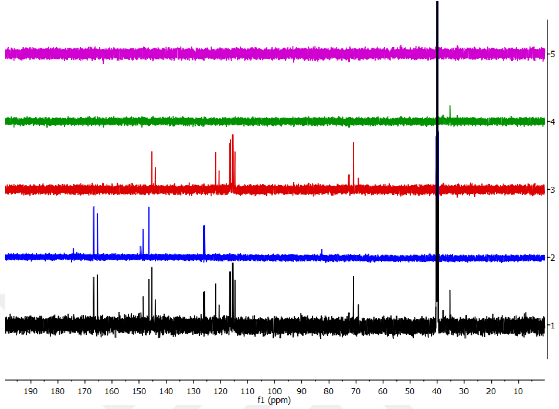
Şekil 4.70 CPC-8 bileşiğinin (1,3-dikafeoilkuinik asit) ^{13}\text{C} DEPT NMR spektrumu (DMSO- \text{d}_6 )
