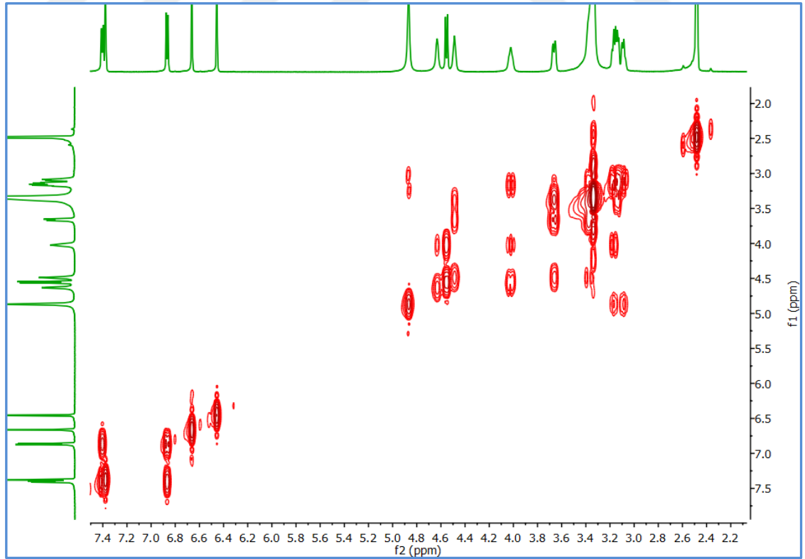
Şekil 3.6 İsoorientin (CPGY-2) bileşiğinin COSY NMR spektrumu (DMSO-d 6 )
