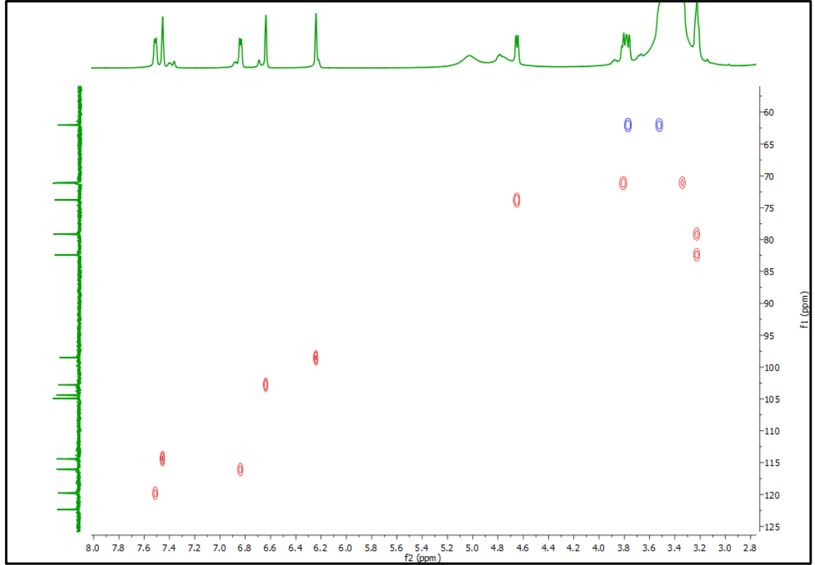
Şekil 1.10 Orientin (CCGY-3) molekülünün HSQC NMR spektrumu (DMSO- \text{d}_6 )
