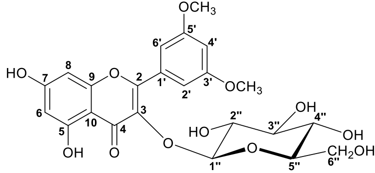
Şekil 4.17 CCGY-5 bileşiğinin (Cankiriense-1) yapısı
