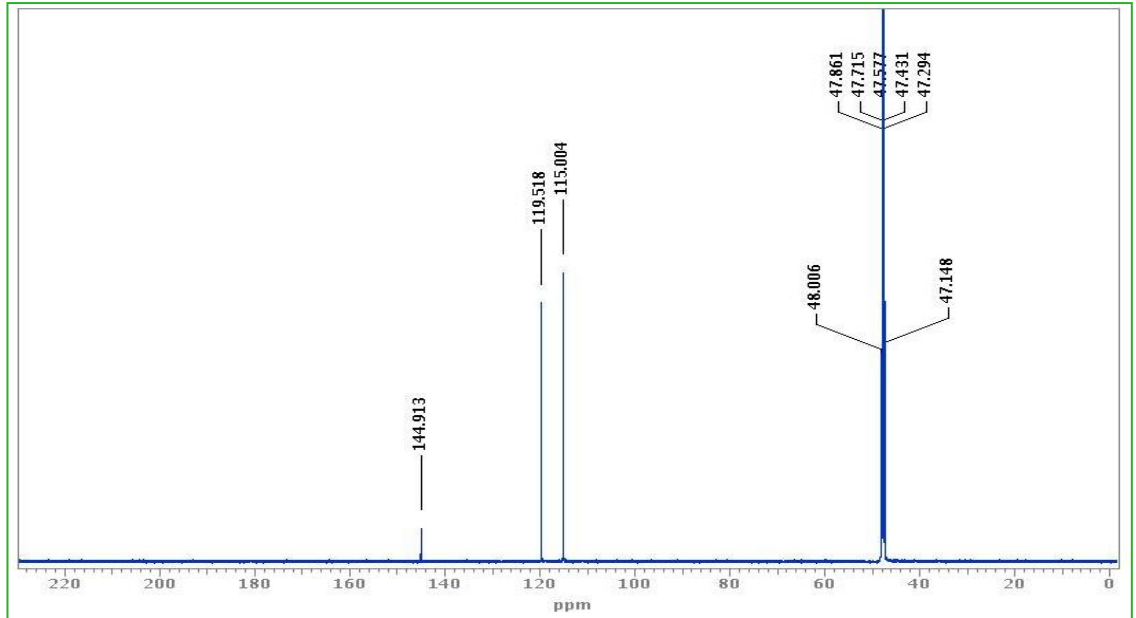
Şekil 2.39 Pirokeşol (CPÇ-1) bileşğinin ^{13}\text{C} NMR spektrumu (MeOD- \text{d}_4 )
