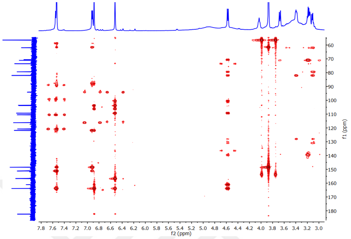
Şekil 3.23 Diosmetin 6-C- \beta glikozit (CPGY-6) bileşiğinin HMBC NMR spektrumu (DMSO- d_6 )
