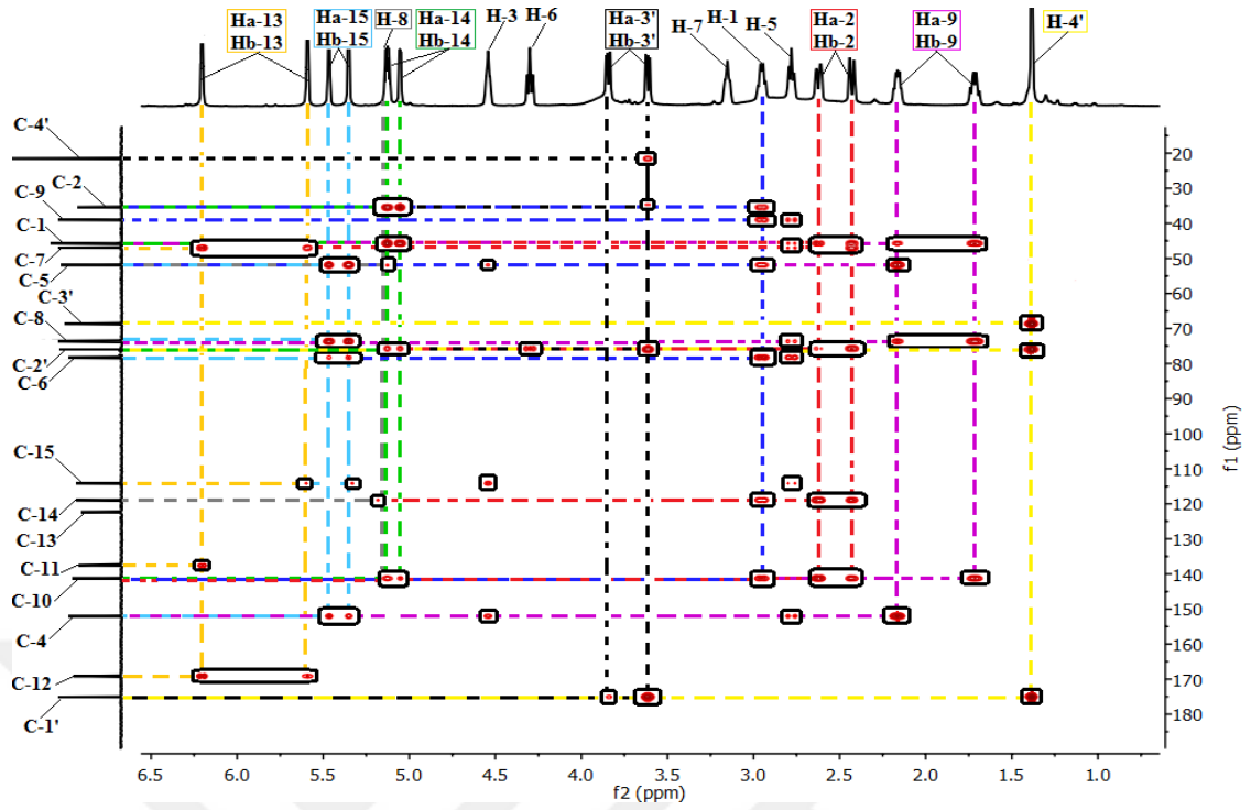
Şekil 4.103 CPGY-12 bileşiğinin [8 \alpha -O-(2',3'-dihidroksiizobutiril) desasiklinaropikrin] HMBC NMR spektrumu (CDCl 3 -d 1 )
