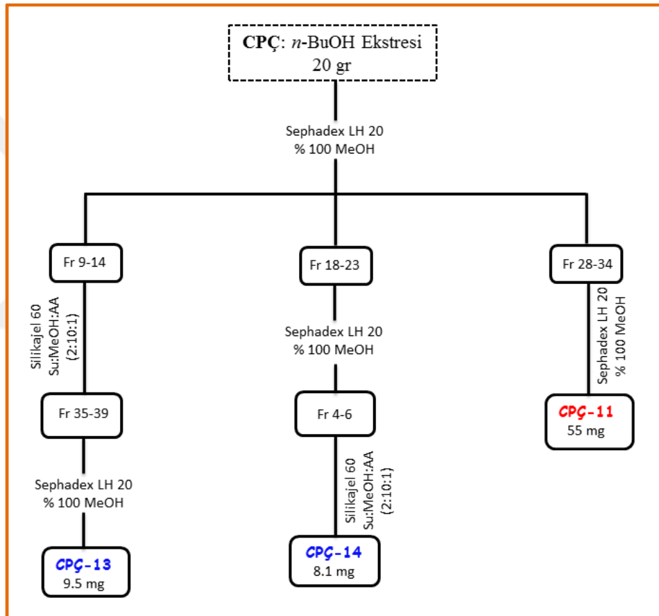
Şekil 3.7 CPÇ (n-BuOH ekstresi) izolasyon şeması
