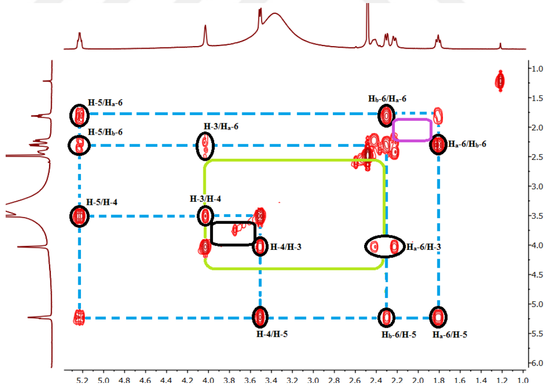
Şekil 4.75 CPC-8 bileşiğinin (1,3-dikafeoilkuinik asit) COSY NMR spektrumu (DMSO-d 6 )
