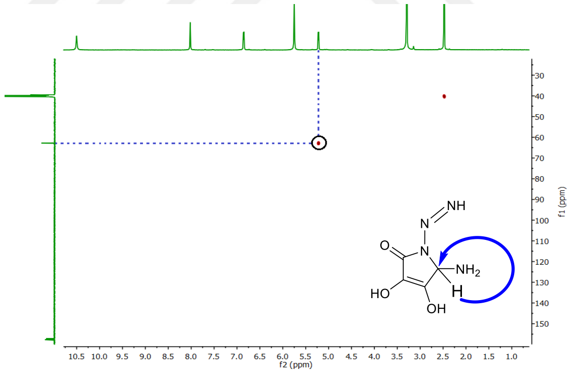
Şekil 4.55 CPC-12 bileşiğinin (5-amino-1-diazenil-3,4-dihidroksi-1,5-dihidro-2H-pirol-2-on) HSQC NMR spektrumu (DMSO- \text{d}_6 )
