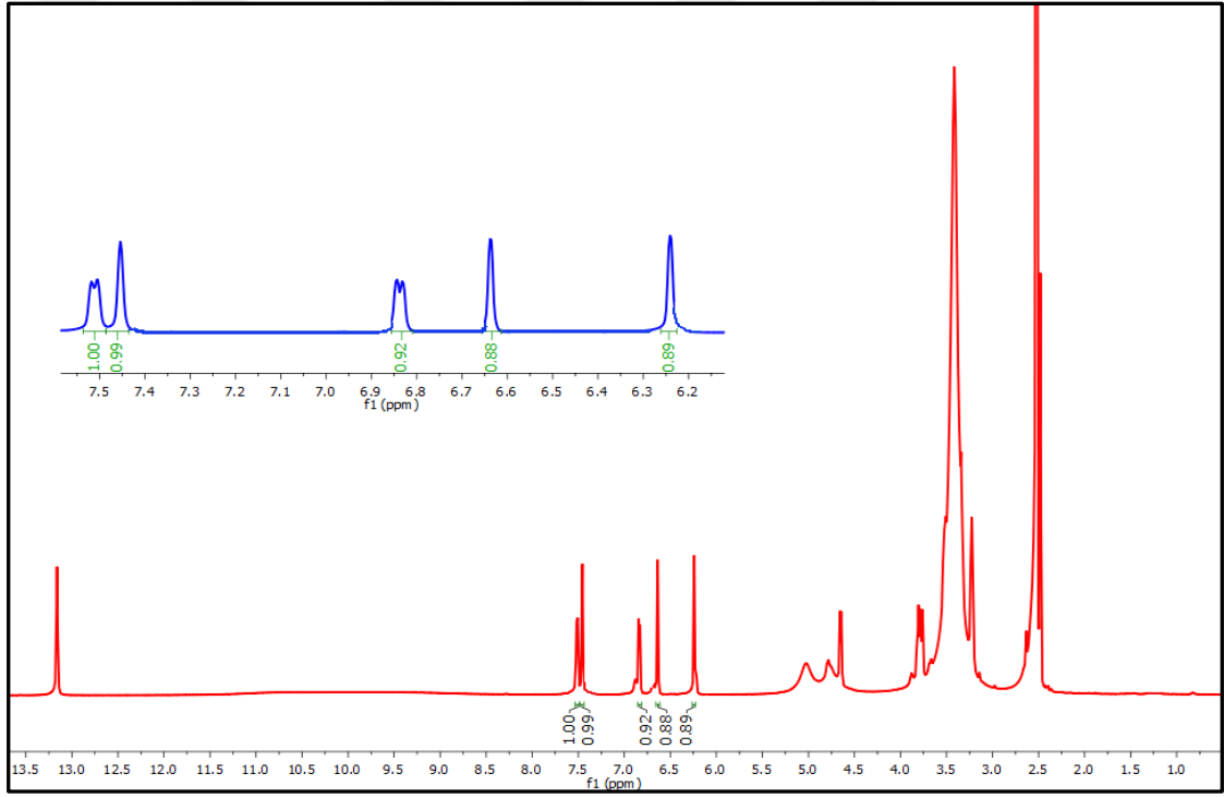
Şekil 1.8 Orientin (CCGY-3) molekülünün ^1\text{H} -NMR spektrumu ( \text{DMSO-d}_6 )
