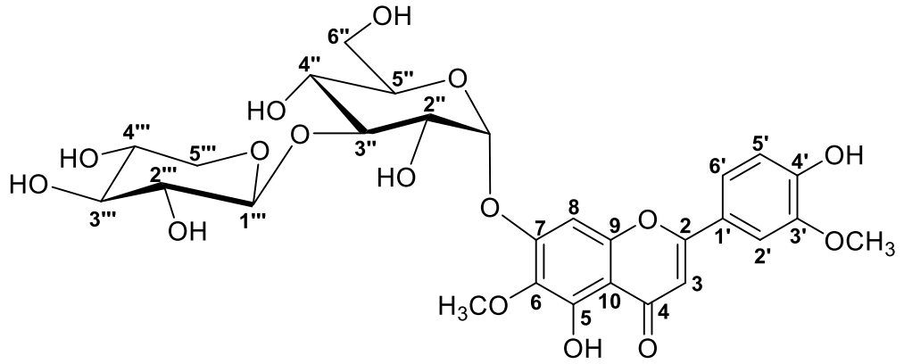
Şekil 4.29 CCGY-9 bileşiğinin (Cankiriense-2) kimyasal yapısı
