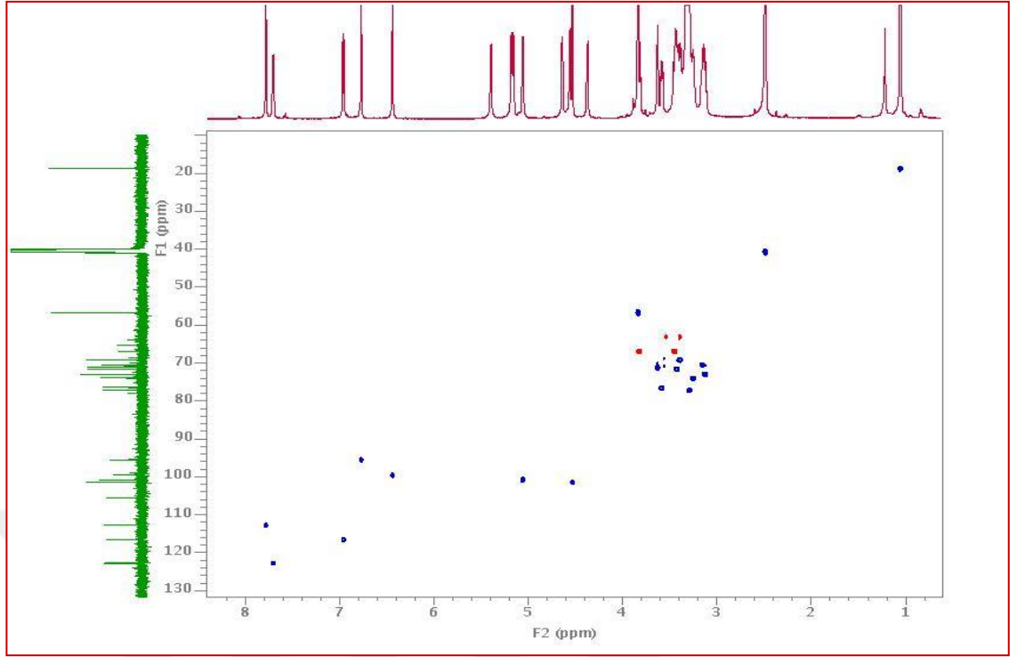
Şekil 2.25 Tamariksetin 7-O- \beta rutinozit (CPC-13) molekülünün HSQC NMR spektrumu (DMSO- d_6 )
