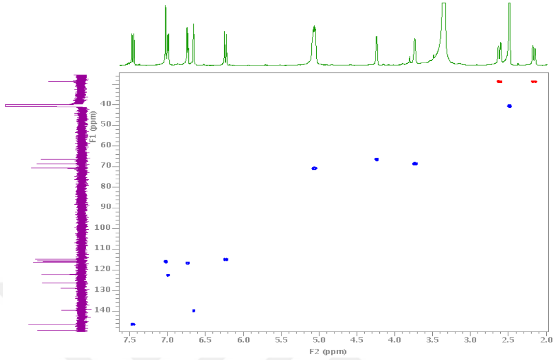
Şekil 2.34 5-O-kafeoil şikimik asit (CPC-4) bileşiğinin HSQC NMR spektrumu (DMSO-d 6 )
