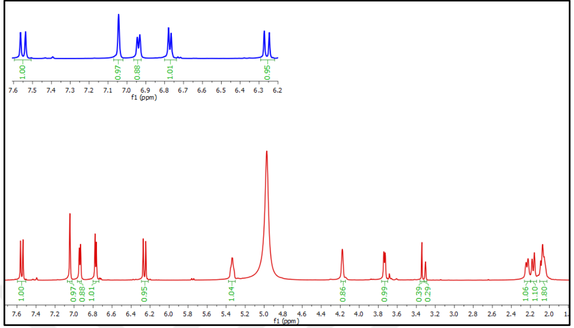
Şekil 4.36 CCGY-2 bileşiğinin (Klorojenik asit) 1 H NMR spektrumu (MeOD-d 4 )
