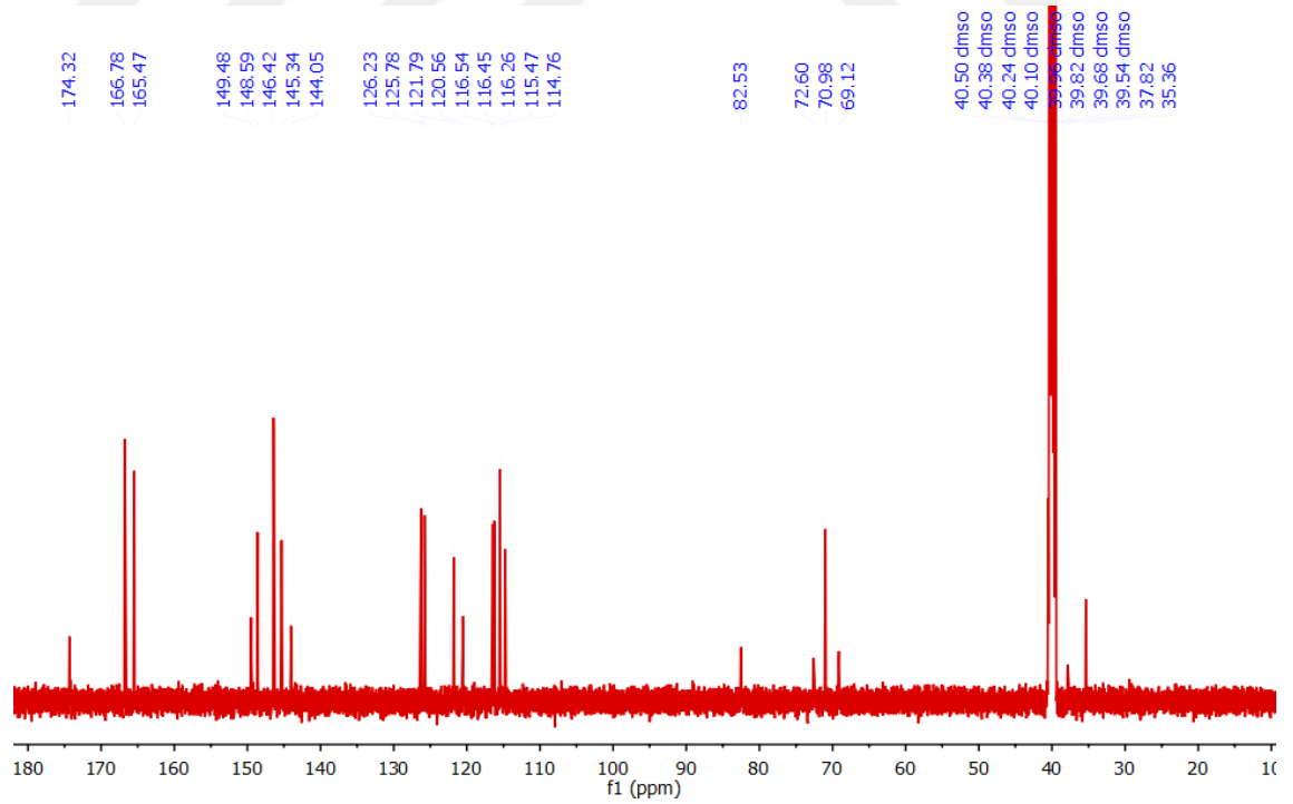
Şekil 4.69 CPC-8 bileşiğinin (1,3-dikafeoilkuinik asit) ^{13}\text{C} NMR spektrumu (DMSO- \text{d}_6 )
