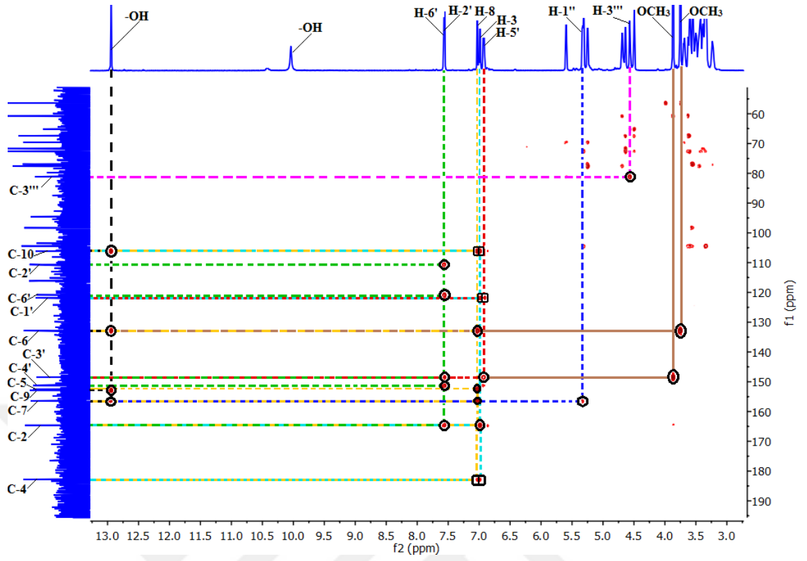
Şekil 4.34 CCGY-9 bileşiğinin (Cankiriense-2) HMBC NMR spektrumu (DMSO- d_6 )
