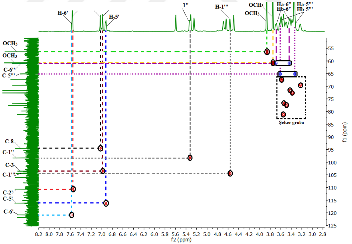
Şekil 4.33 CCGY-9 bileşiğinin (Cankiriense-2) HSQC NMR spektrumu ( \text{DMSO}-d_6 )
