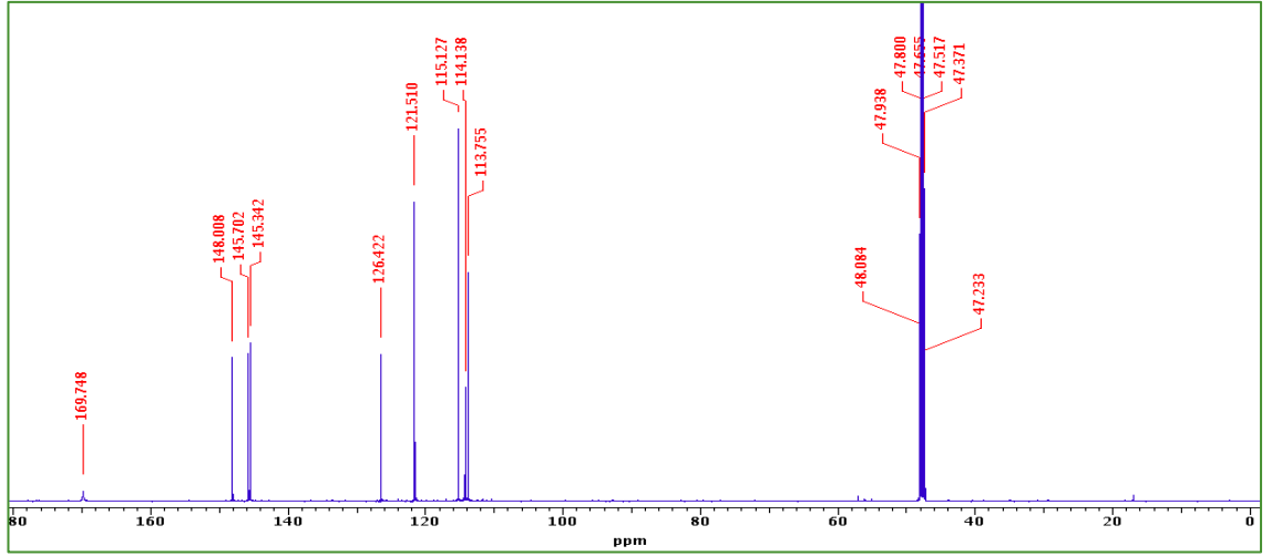
Şekil 4.43 CCGY-4 bileşiğinin (Kafeik asit) ^{13}\text{C} NMR spektrumu (MeOD- d_4 )
