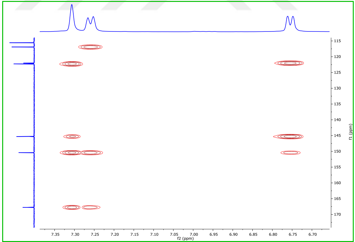
Şekil 1.5 Klorojenik asit (CCGY-2) molekülünün HMBC spektrumu (DMSO-d 6 )
