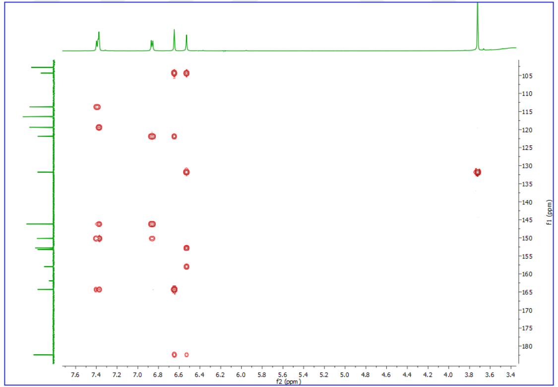
Şekil 1.21 Nepetin (CCGY-7) molekülüne ait HMBC NMR spektrumu (DMSO-d 6 )
