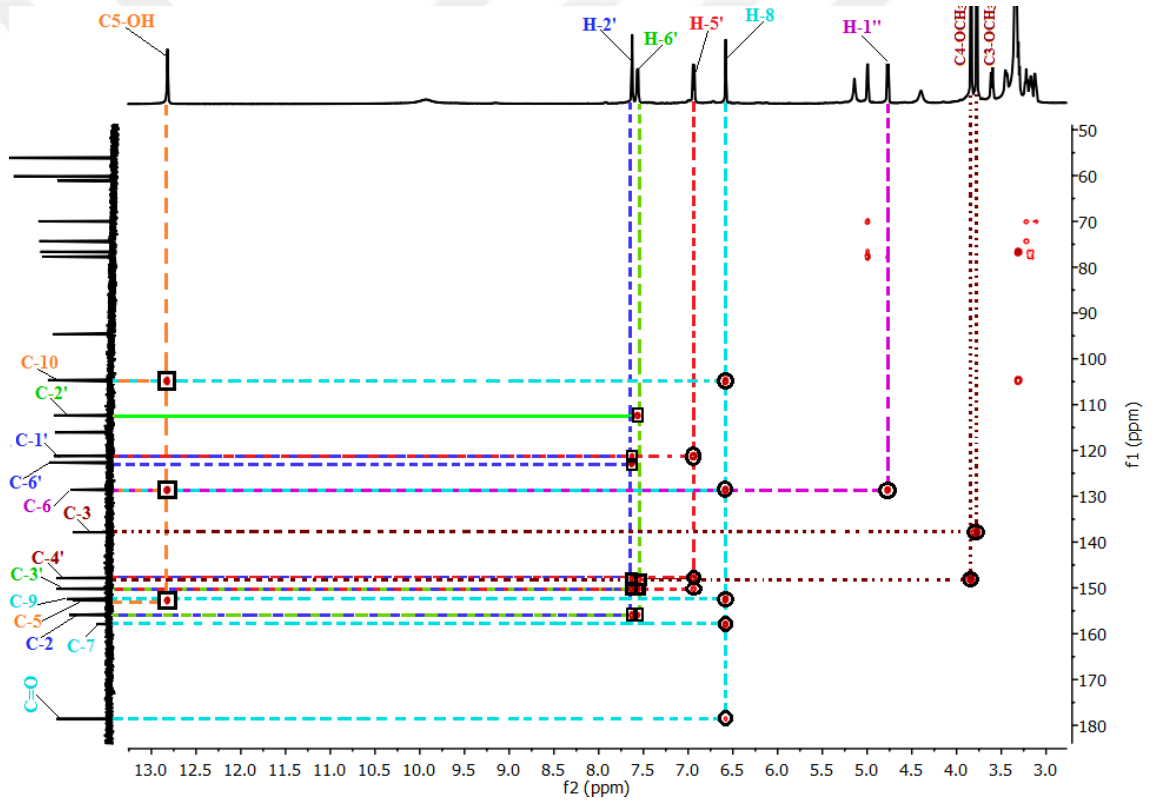
Şekil 4.86 CPGY-8 bileşiğinin (Paphlagonica-2) HMBC NMR spektrumu (DMSO-d 6 )
