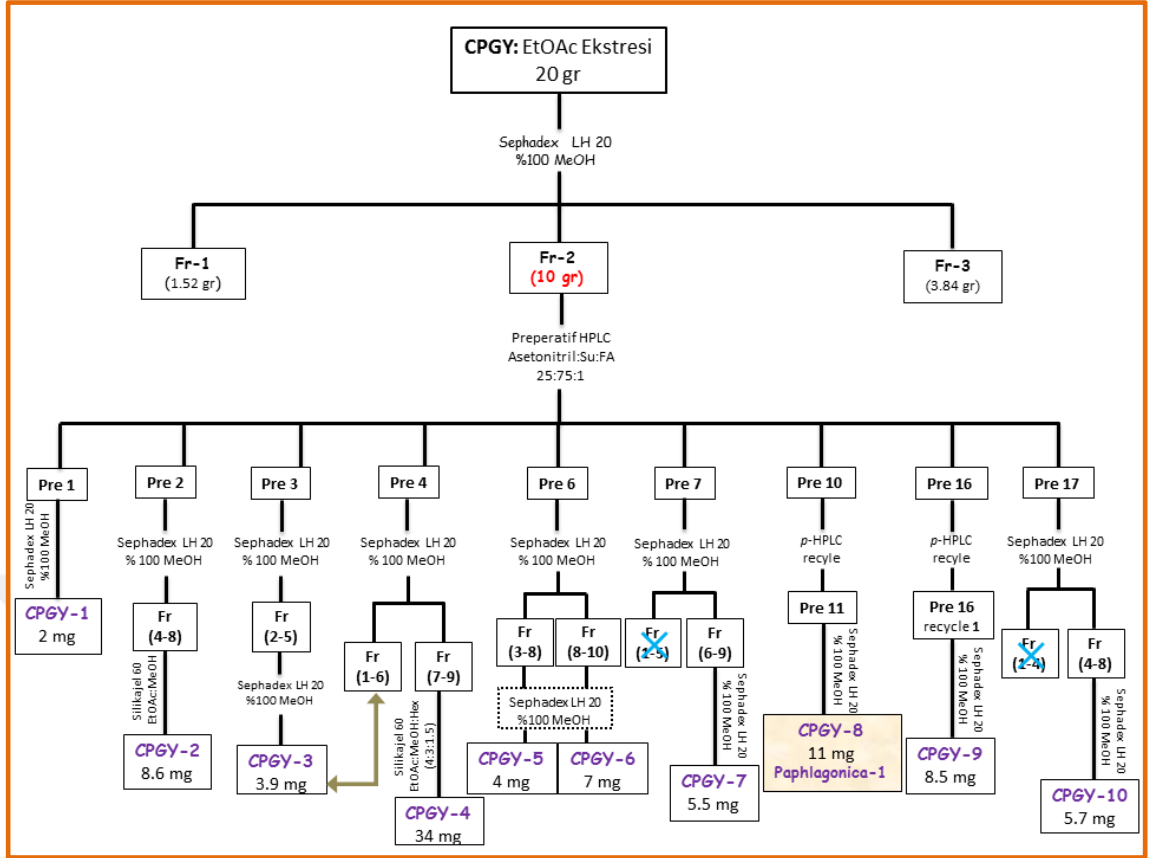
Şekil 3.8 CPGY (EtOAc ekstresi) izolasyon şeması
