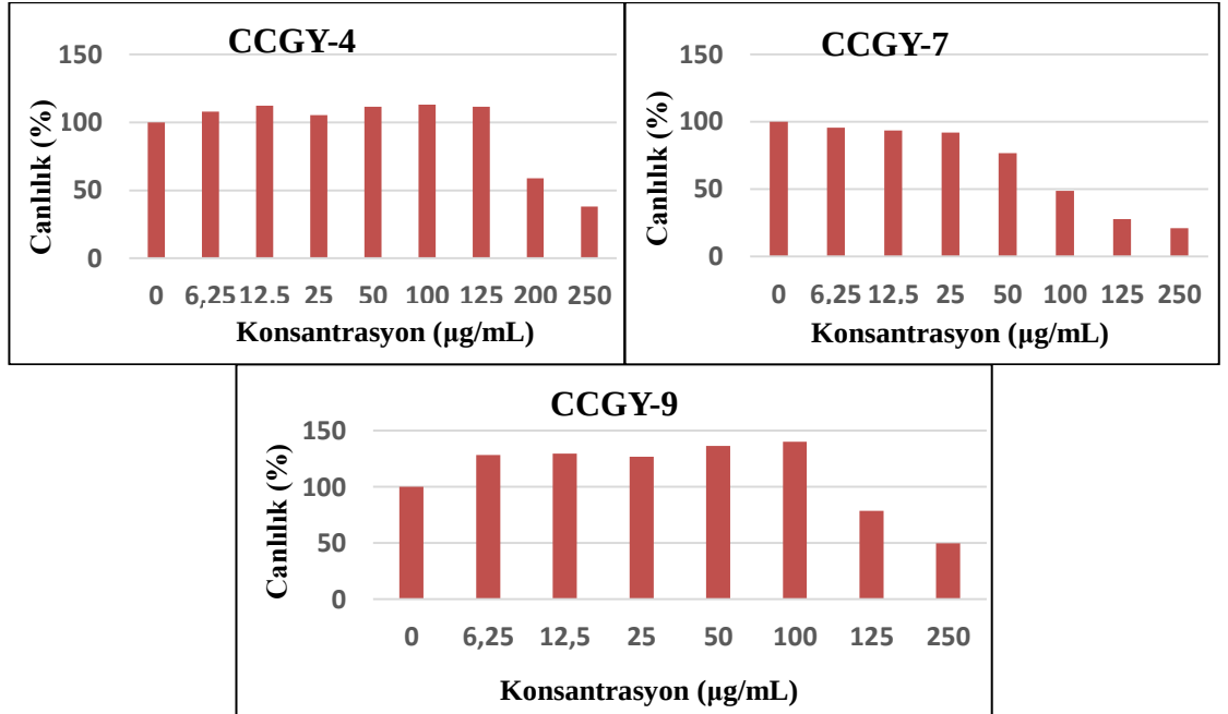
Şekil 4.107 C. cankiriense gövde-yaprak (CCGY) kısımlarından izole edilen bileşiklerin HeLa hücrelerine karşı antikanser aktivite grafikleri
