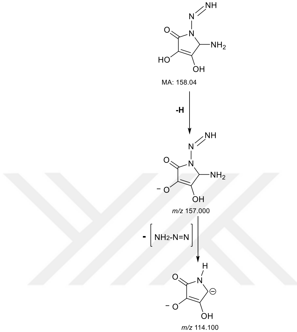
Şekil 4.51 CPÇ-12 bileşiğinin (Paphlagonica-1) MS-MS parçalanma ürünleri
