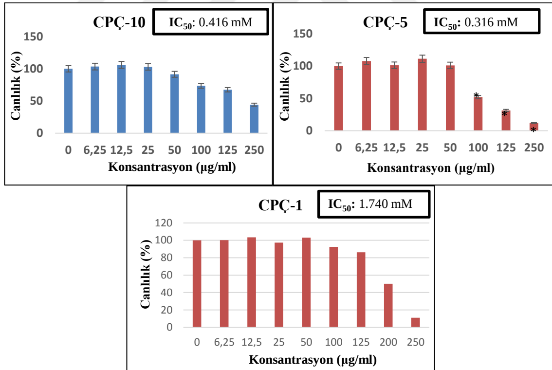
Şekil 4.108 C. paphlagonica çiçek (CPÇ) ekstresinden izole edilen bileşiklerin HeLa hücresine karşı antiproliferatif aktivite grafikleri
