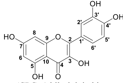
Kuersetin (CPC-7) bileşığının kimyasal yapısı
