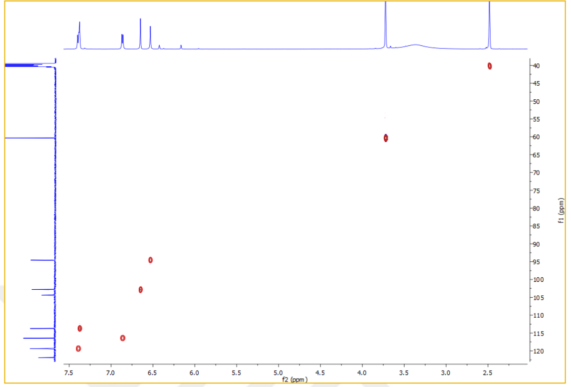
Şekil 1.20 Nepetin (CCGY-7) molekülüne ait HSQC NMR spektrumu (DMSO-d 6 )
