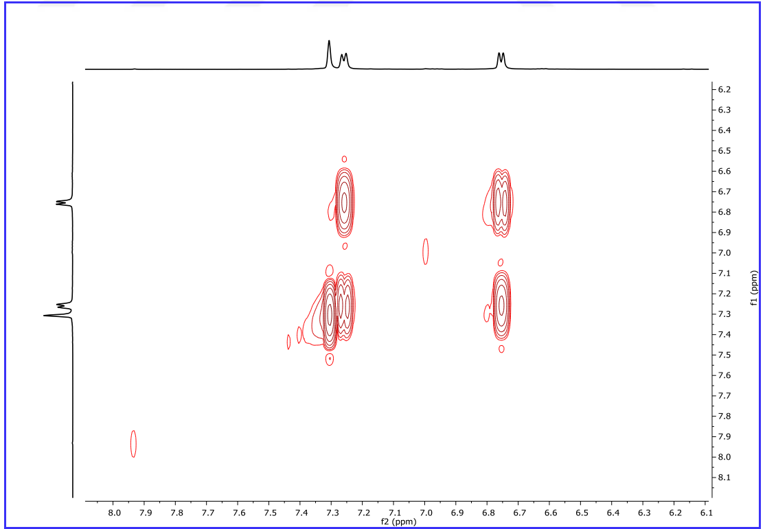
Şekil 1.7 Klorojenik asit (CCGY-2) molekülünün COSY spektrumu (DMSO-d 6 )
