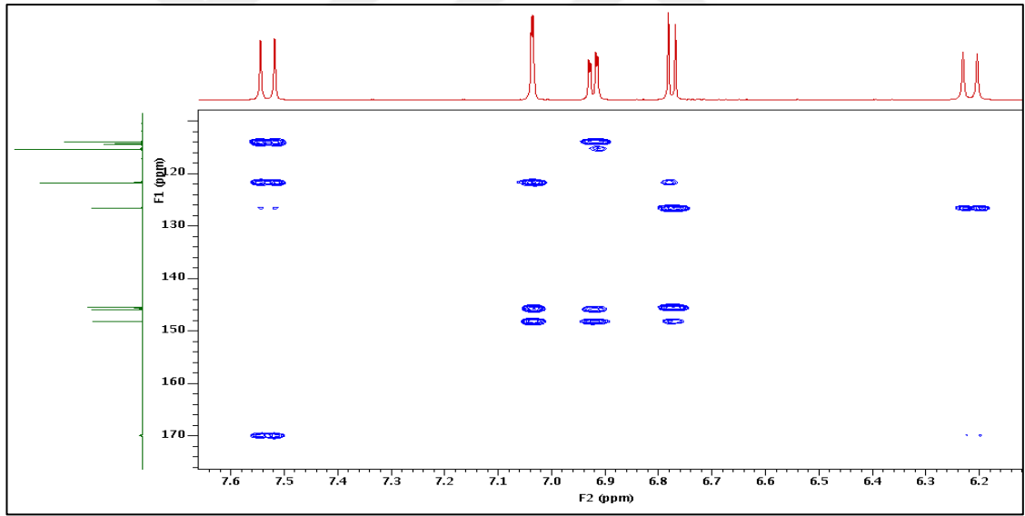
Şekil 4.46 CCGY-4 bileşiğinin (Kafeik asit) HMBC NMR spektrumu (MeOD- d_4 )
