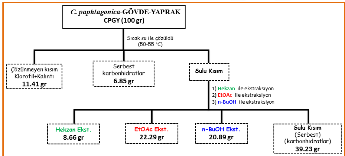
Şekil 3.4 CPGY ekstraktlarının elde edilme şeması
