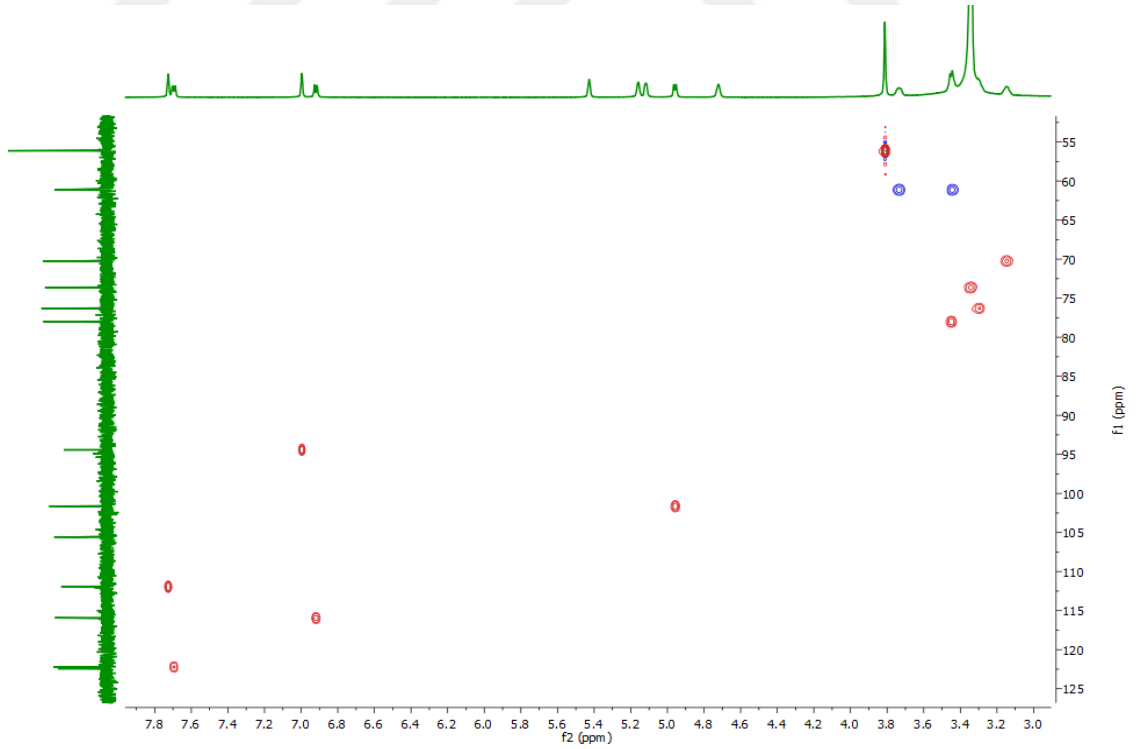
Şekil 3.28 Kuersetagetin-4'-metileter-7-O-β glikozit (CPGY-7) bileşiğinin HSQC NMR spektrumu (DMSO- \text{d}_6 )
