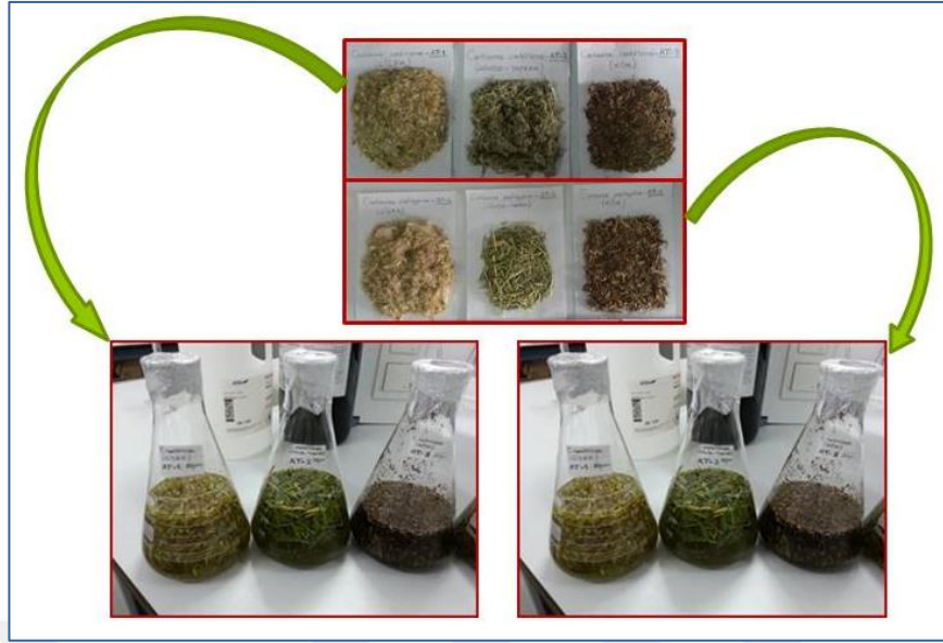
Şekil 3.1 Biyolojik aktivite için parçalanmış bitkilerin ekstraksiyon işlemi
