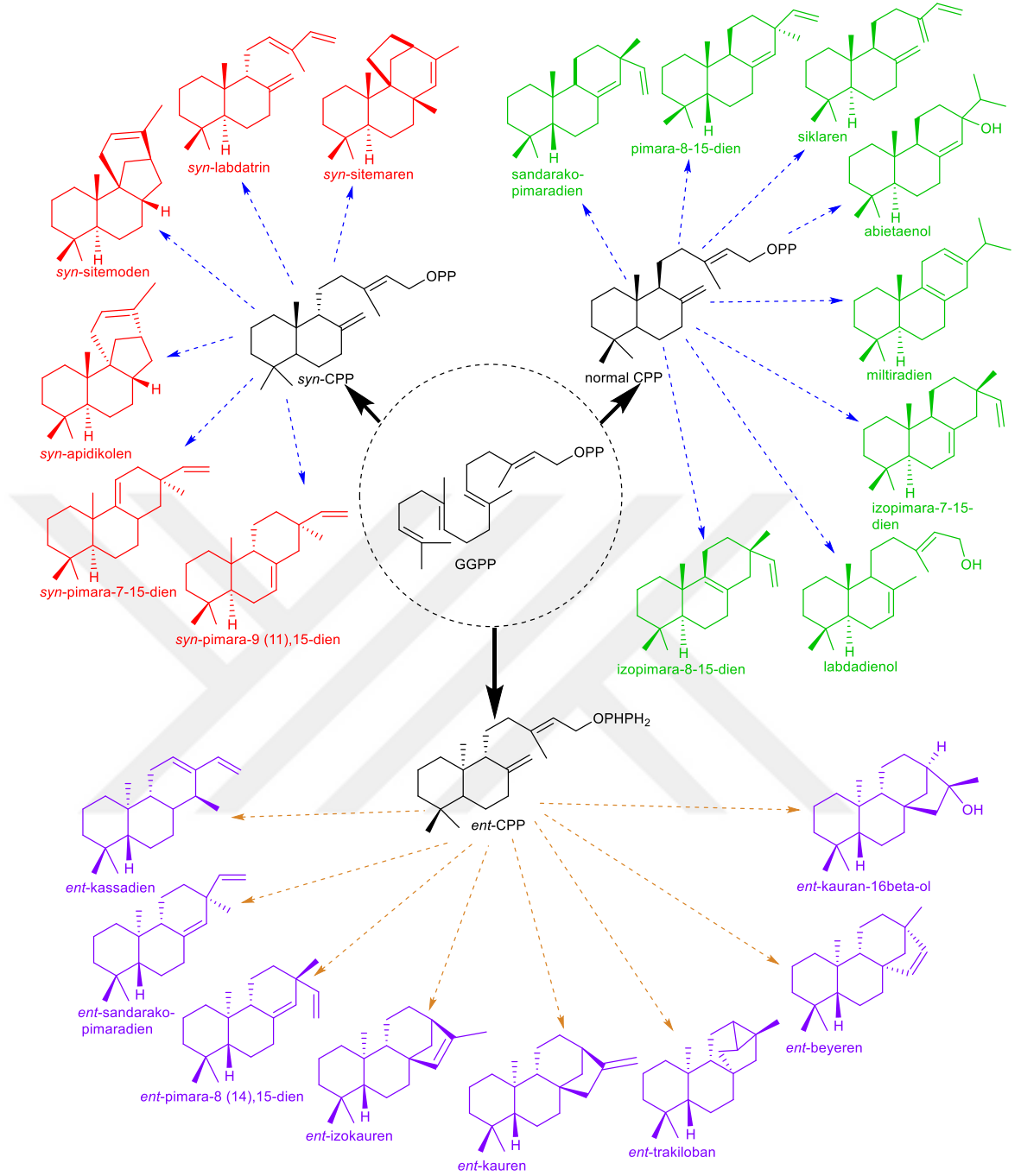
Şekil 2.14 Diterpenlerin biyo-sentezi ve bazı diterpenler (Andersen-Ranberg et al. 2016, Smanski et al. 2012, Vattekkatte and Boland 2020)
