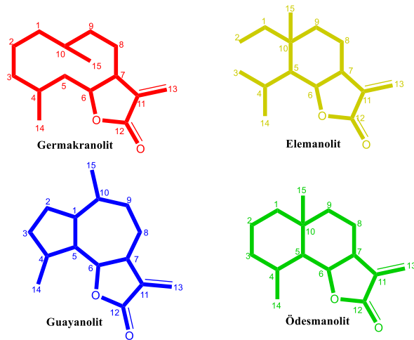
Şekil 2.12 Bazı seskiterpen lakton grupları
