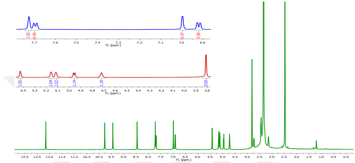
Şekil 3.25 Kuersetagetin-4'-metileter-7-O-β glikozit (CPGY-7) bileşiğinin 1 H NMR spektrumu (DMSO-d 6 )
