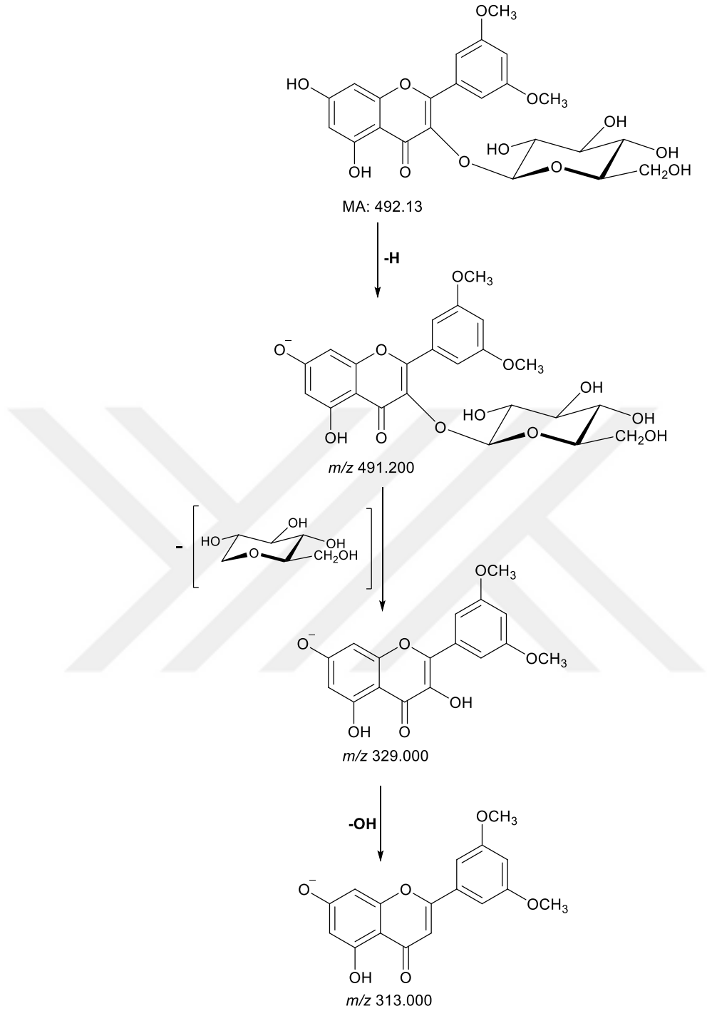
Şekil 4.16 CCGY-5 bileşiğinin (Cankiriense-1) MS-MS parçalanma ürünleri
