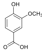
CPÇ-2 Vanilik asit
