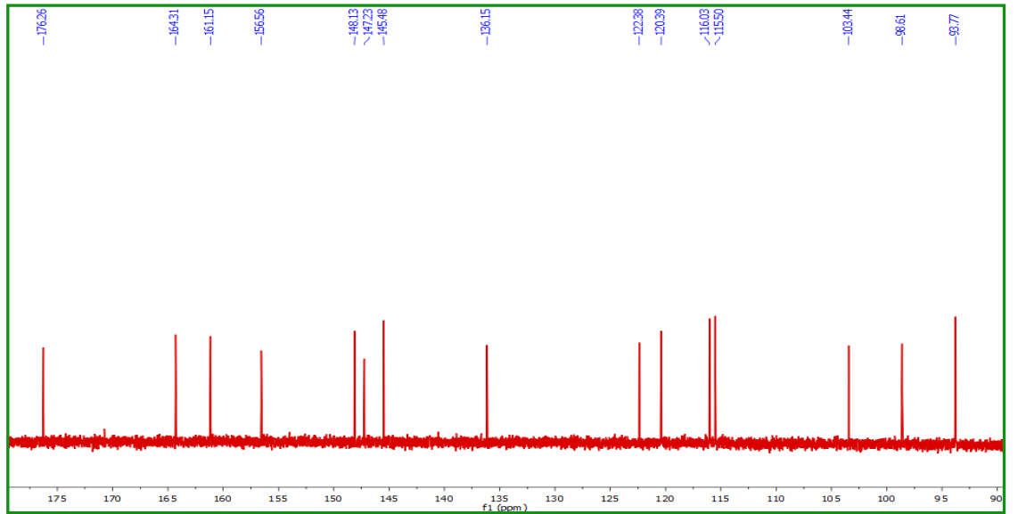
Şekil 2.11 Kuersetin (CPC-7) molekülüne ait ^1\text{H} NMR spektrumu
