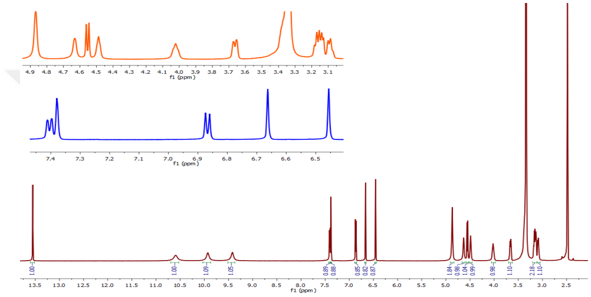
Şekil 3.1 İsoorientin (CPGY-2) bileşiğinin 1 H NMR spektrumu (DMSO-d 6 )
