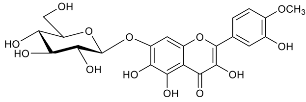
Kuersetagetin-4'-metileter-7-O-β glikozit (CPGY-7) bileşiğinin kimyasal yapısı
