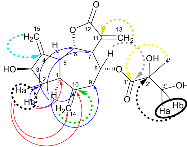
Şekil 4.102 CPGY-12 bileşiğine ait [8 \alpha -O-(2',3'-dihidroksiizobutiril) desasiklinaropikrin] HMBC etkileşimleri
