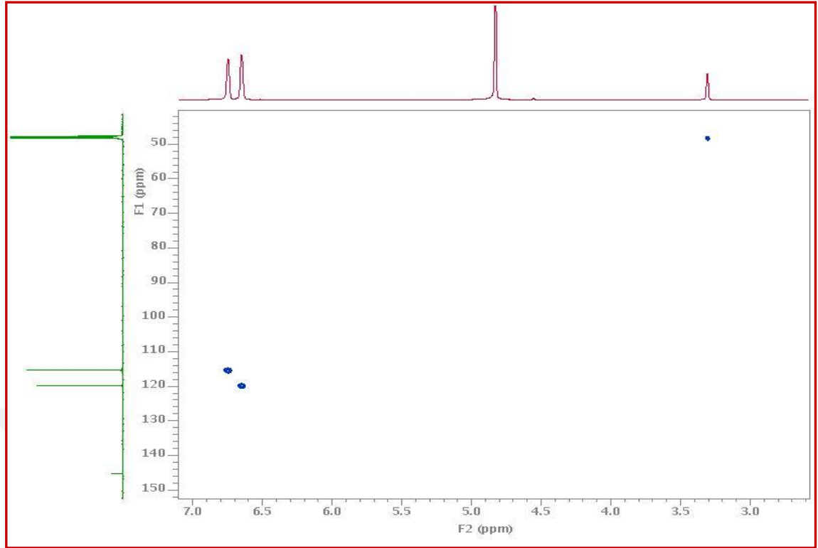
Şekil 2.42 Pirokateşol (CPC-1) bileşiğinin HSQC NMR spektrumu (MeOD-d 4 )
