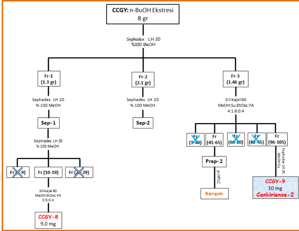
Şekil 3.11 CCGY ( n -BuOH ekstresi) izolasyon şeması
