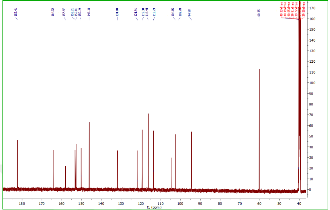
Şekil 1.18 Nepetin (CCGY-7) molekülüne ait ^{13}\text{C} NMR spektrumu (DMSO- \text{d}_6 )
