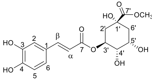
Klorojenik asit metil ester (CPC-6) bileşığının kimyasal yapısı
