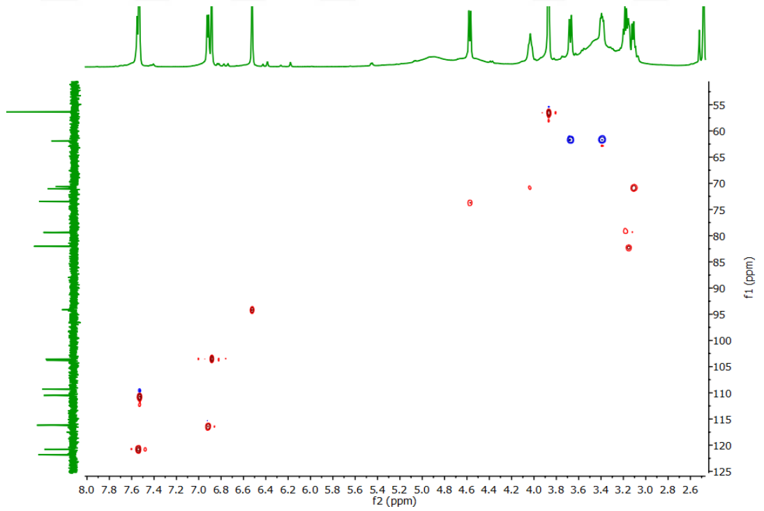
Şekil 3.22 Diosmetin 6-C- \beta glikozit (CPGY-6) bileşiğinin HSQC NMR spektrumu (DMSO- \text{d}_6 )
