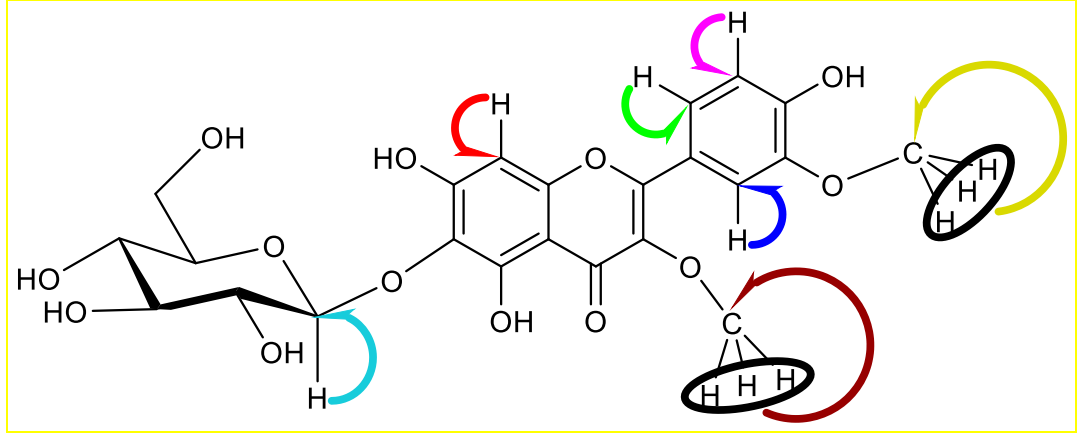
Şekil 4.85 CPGY-8 bileşiğinin (Paphlagonica-2) HSQC etkileşimi
