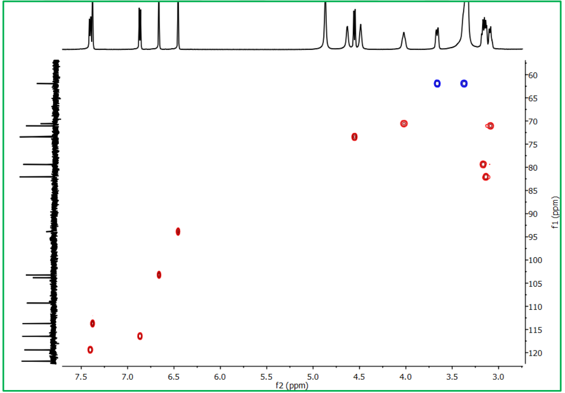
Şekil 3.4 İsoorientin (CPGY-2) bileşiğinin HSQC NMR spektrumu ( \text{DMSO-d}_6 )
