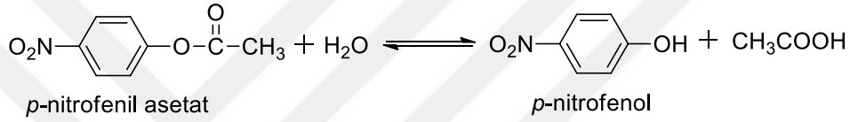
Şekil 3.18 p -nitrofenilasetatın, p -nitrofenole dönüşüm mekanizması
