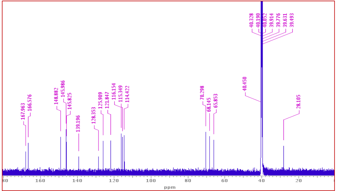
Şekil 2.31 5-O-kafeoil şikimik asit (CPC-4) bileşığının 13 C NMR spektrumu (DMSO-d 6 )
