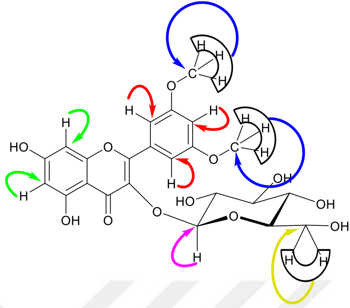
Şekil 4.21 CCGY-5 (Cankiriense-1) bileşiğinin HSQC etkileşimi
