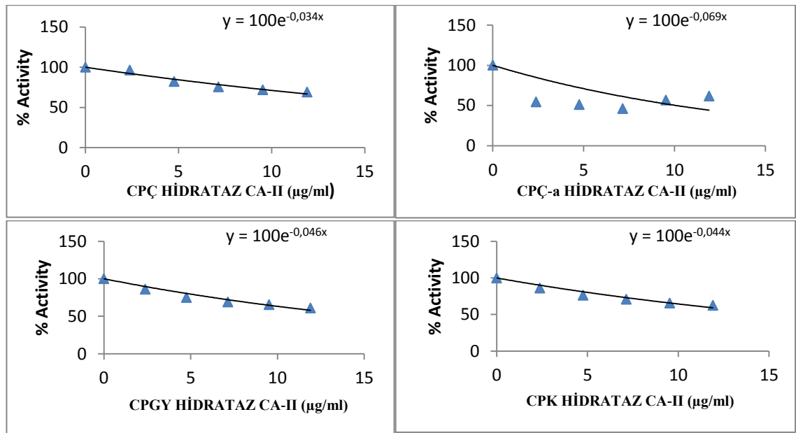
Şekil 4.8 C. paphlagonica ve C. cankiriense bitki ekstralarının CA-II izoenzimine karşı hidrataz aktivitesi grafikleri
