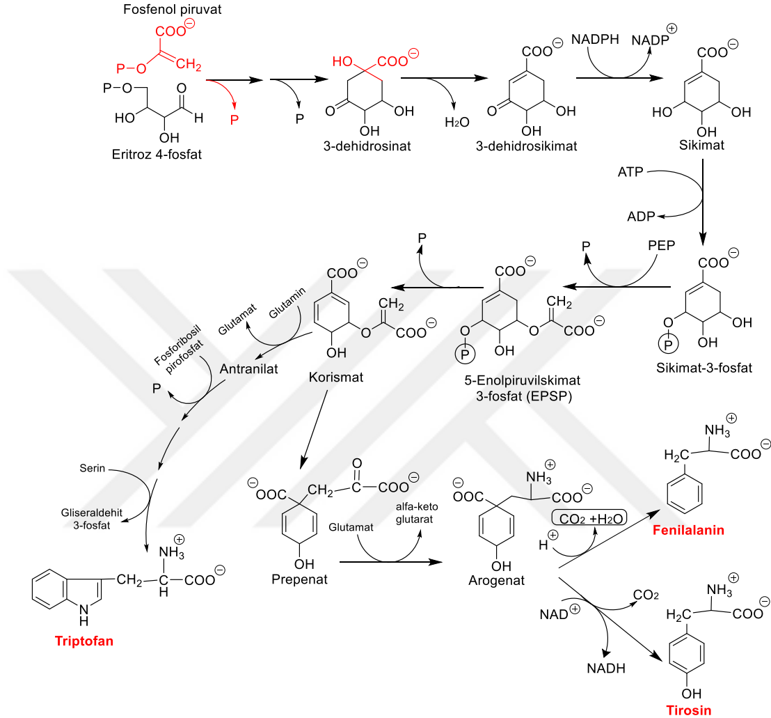
Şekil 2.16 Alkaloidlerin temel olarak türedikleri biyosentez basamakları (Diaz et al. 2015, Funayama and Cordell 2014)
