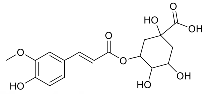
CPGY-4 3-O-feruloilkuinik asit
