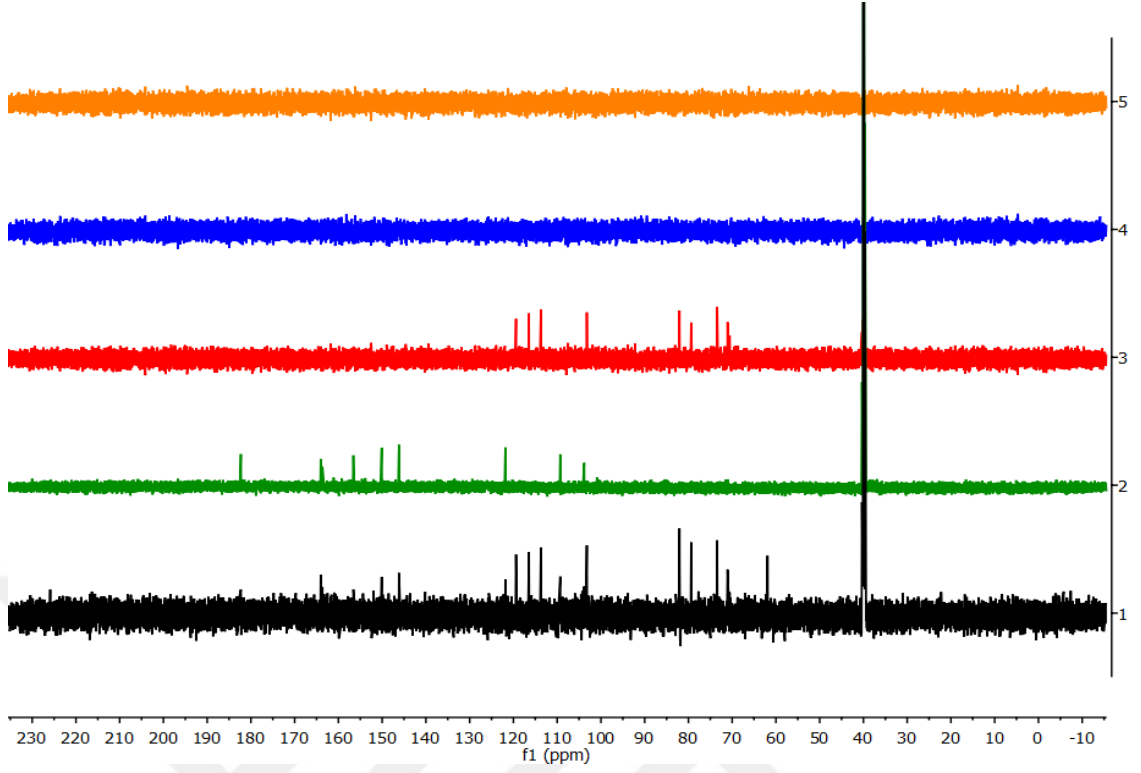
Şekil 3.3 İsoorientin (CPGY-2) bileşiğinin ^{13}\text{C} DEPT NMR spektrumu ( \text{DMSO-d}_6 )
