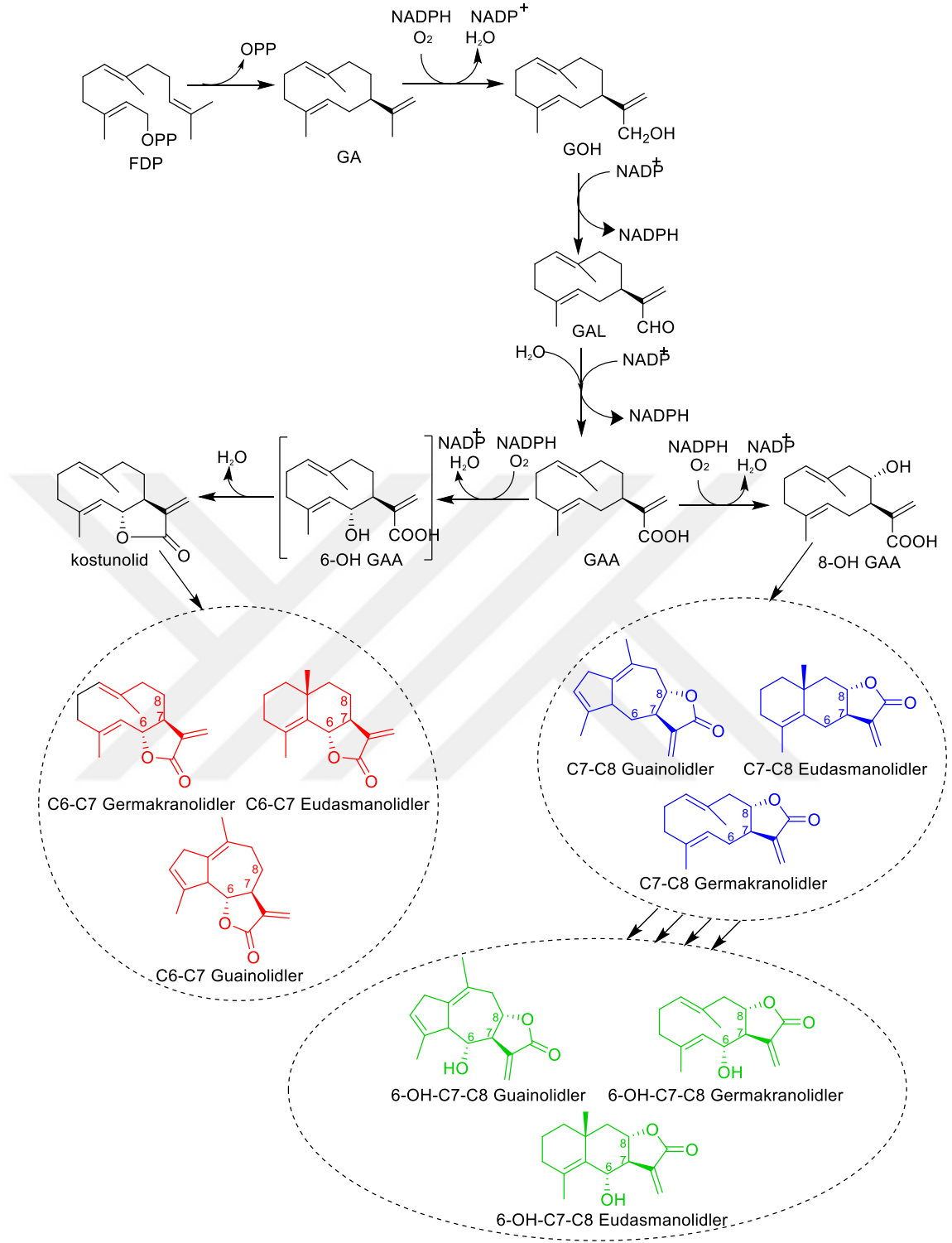
Şekil 2.13 Seskiterpen laktonların biyosentezi ve bazı seskiterpen laktonlar (De Kraker et al. 2002, Ramirez et al. 2013)
