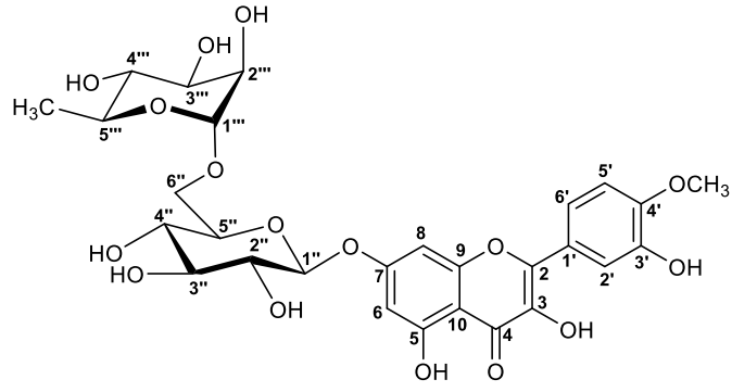
Tamariksetin 7-O-β rutinozid (CPÇ-13) bileşiğinin kimyasal yapısı
