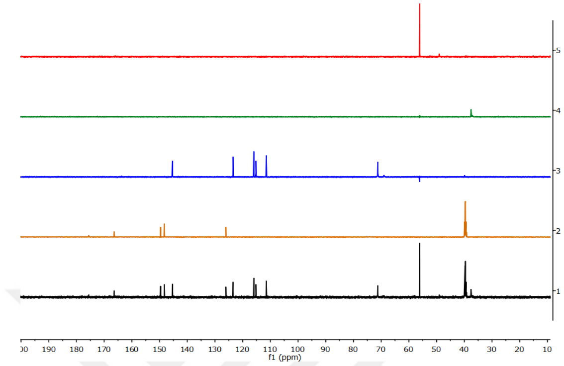
Şekil 3.9 3-O-feruloilkuinik asit (CPGY-4) bileşiğinin ^{13}\text{C} DEPT NMR spektrumu (DMSO- \text{d}_6 )
