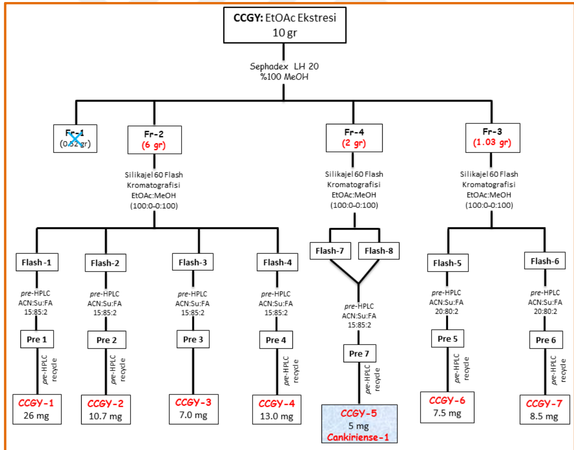
Şekil 3.10 CCGY (EtOAc ekstresi) izolasyon şeması
