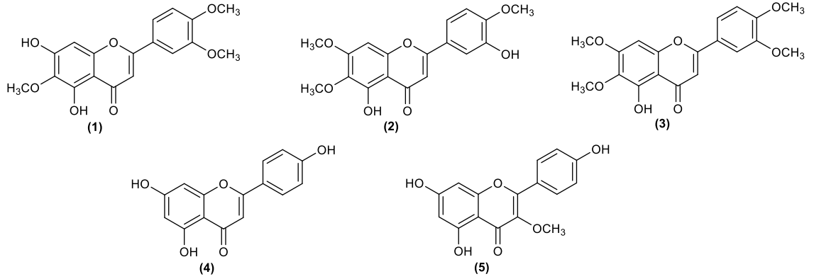
Şekil 5.3 Centaurea arenaria bitkisinden izole edilen bazı flavonoidler
