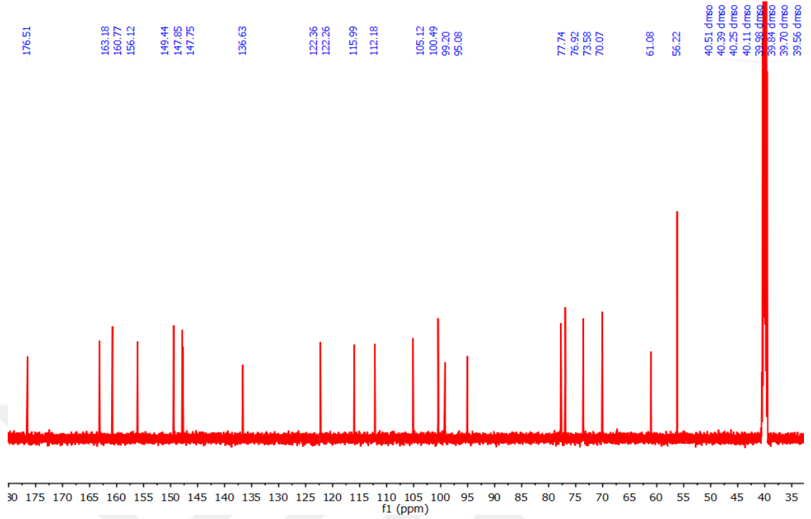
Şekil 4.61 CPC-9 bileşiğinin (Tamariksetin 7-O- \beta -D glukopiranozit) ^{13}\text{C} NMR spektrumu (DMSO- \text{d}_6 )
