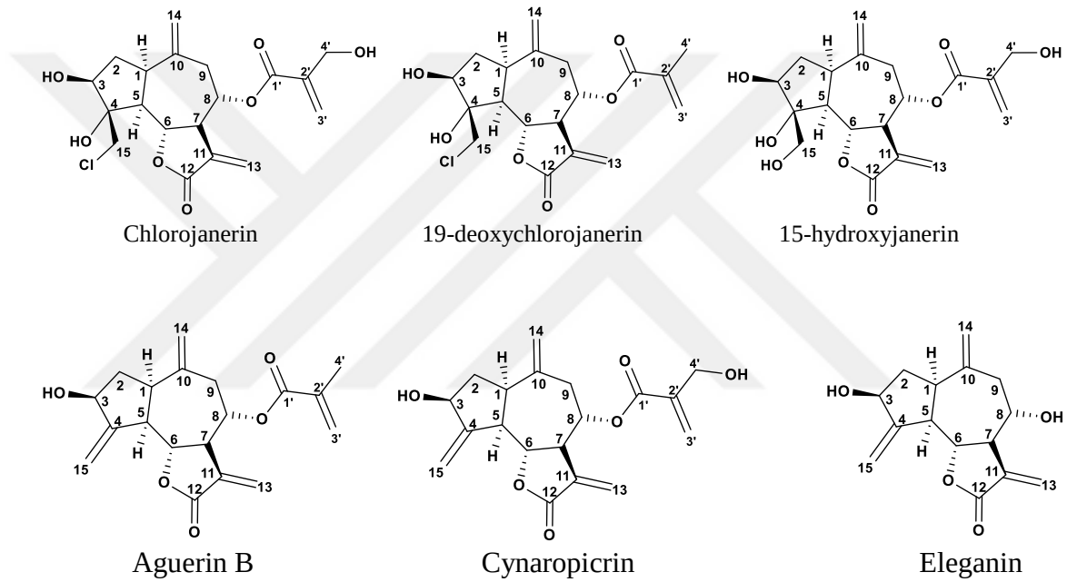
Şekil 5.2 Psephellus pyrrhoblepharus bitkisinden izole edilen seskiterpen laktonlar
