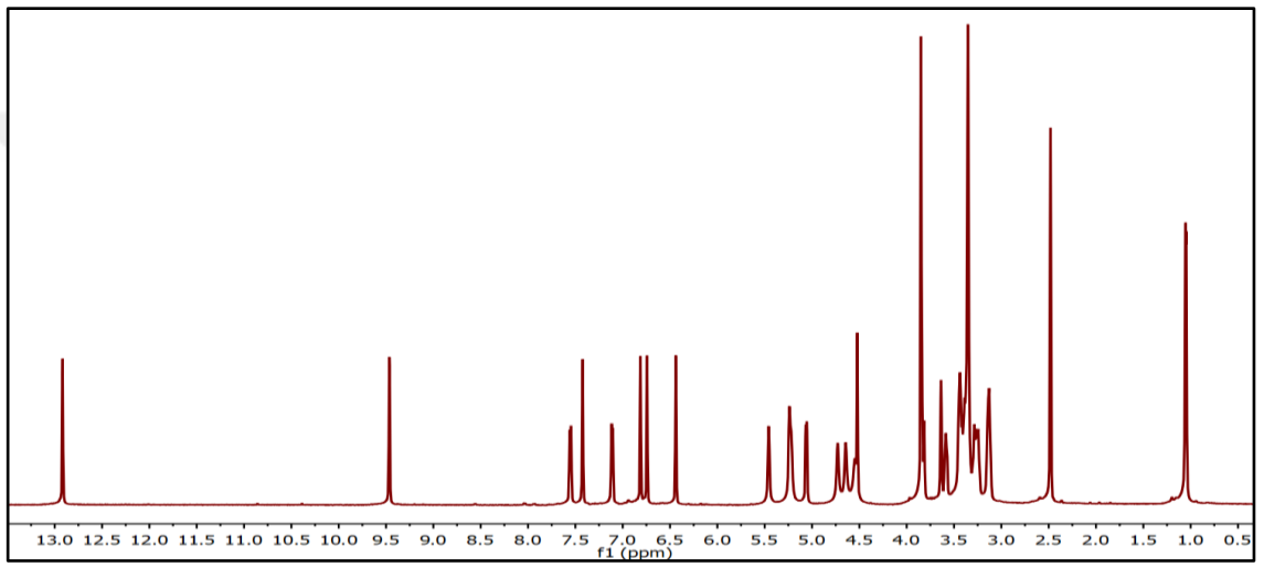
Şekil 1.22 Diosmin (CCGY-8) molekülüne ait 1 H NMR spektrumu (DMSO-d 6 )
