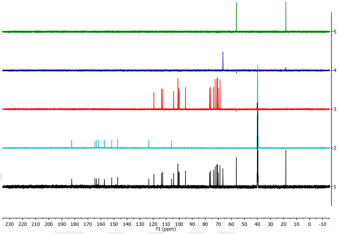
Şekil 1.24 Diosmin (CCGY-8) molekülüne ait ^{13}\text{C} DEPT NMR spektrumu (DMSO- \text{d}_6 )
