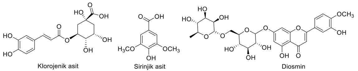
Şekil 4.11 HPLC-TOF/MS analizine göre C. cankiriense ekstralarında ana bileşenler
