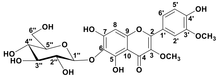
Şekil 4.80 CPGY-8 bileşiğinin (Paphlagonica-2) yapısı
