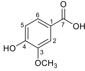
Vanilik asit (CCGY-6) bileşığının kimyasal yapısı
