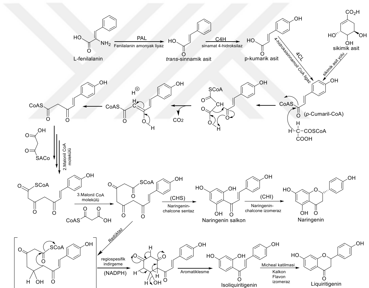
Şekil 2.5 Flavonoidlerin biyosentez yolakları (Austin and Noel 2003, Luhata and Luhata 2017)
