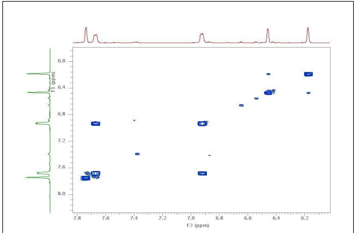
Şekil 2.22 Tamariksetin (CPÇ-5) molekülüne ait COSY NMR spektrumu (DMSO-d 6 )
